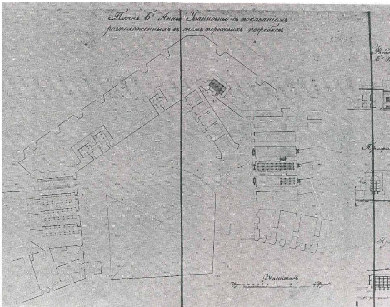
12. План бастиона Анны Иоанновны с показанием расположения пороховых погребков. РГА ВМФ, ф.3/л,оп.34, д.3758. I 843 г. Архив ИЛПР, нег. 68183а.
