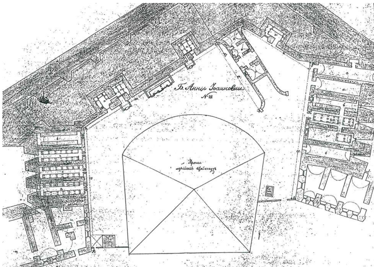
13. Чертеж бастиона Анны Иоанновны. Фрагмент. РГА ВМФ, ф.3/л, оп.34, д.3797а. 1844г.
