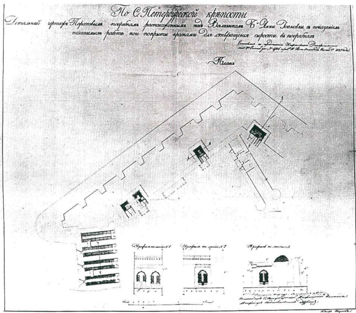
11. Детальный чертеж пороховым погребкам в фасах бастиона Анны Иоанновны. РГА ВМФ, ф.3/л,оп.34, д.3741. 1842 г. Архив ИЛПР, нег. 68182а.
