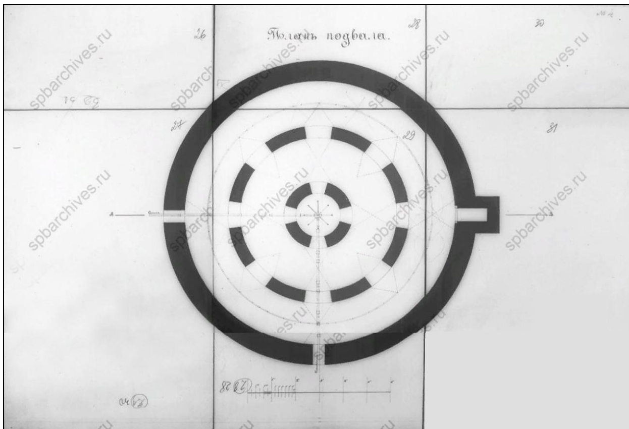
14. Фонтан в Александровском саду. План подвала. 1877 г. Арх. А. Р. Гешвенд. ЦГИА СПб. Ф. 513. Оп. 118. Д. 321. Л. 26–31.
