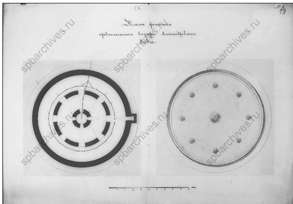
12. План фонтана, предполагаемого внутри Александровского сада. 1877 г. Арх. А. Р. Гешвенд. ЦГИА СПб. Ф. 513. Оп. 118. Д. 321. Л. 18–19.
