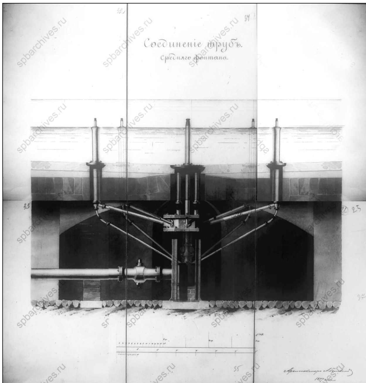
15. Фонтан в Александровском саду. Соединение труб среднего фонтана. 1877 г. Арх. А. Р. Гешвенд. ЦГИА СПб. Ф. 513. Оп. 118. Д. 321. Л. 32–37.
