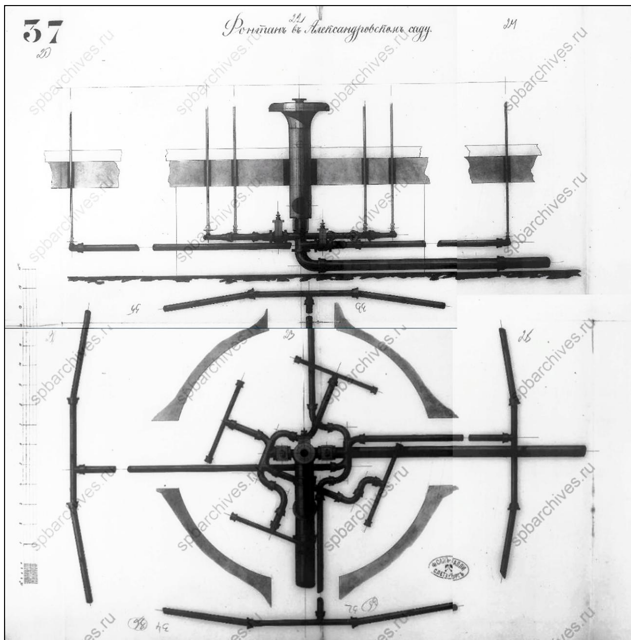
13. Фонтан в Александровском саду. 1877 г. Арх. А. Р. Гешвенд. ЦГИА СПб. Ф. 513. Оп. 118. Д. 321. Л. 20–35.
