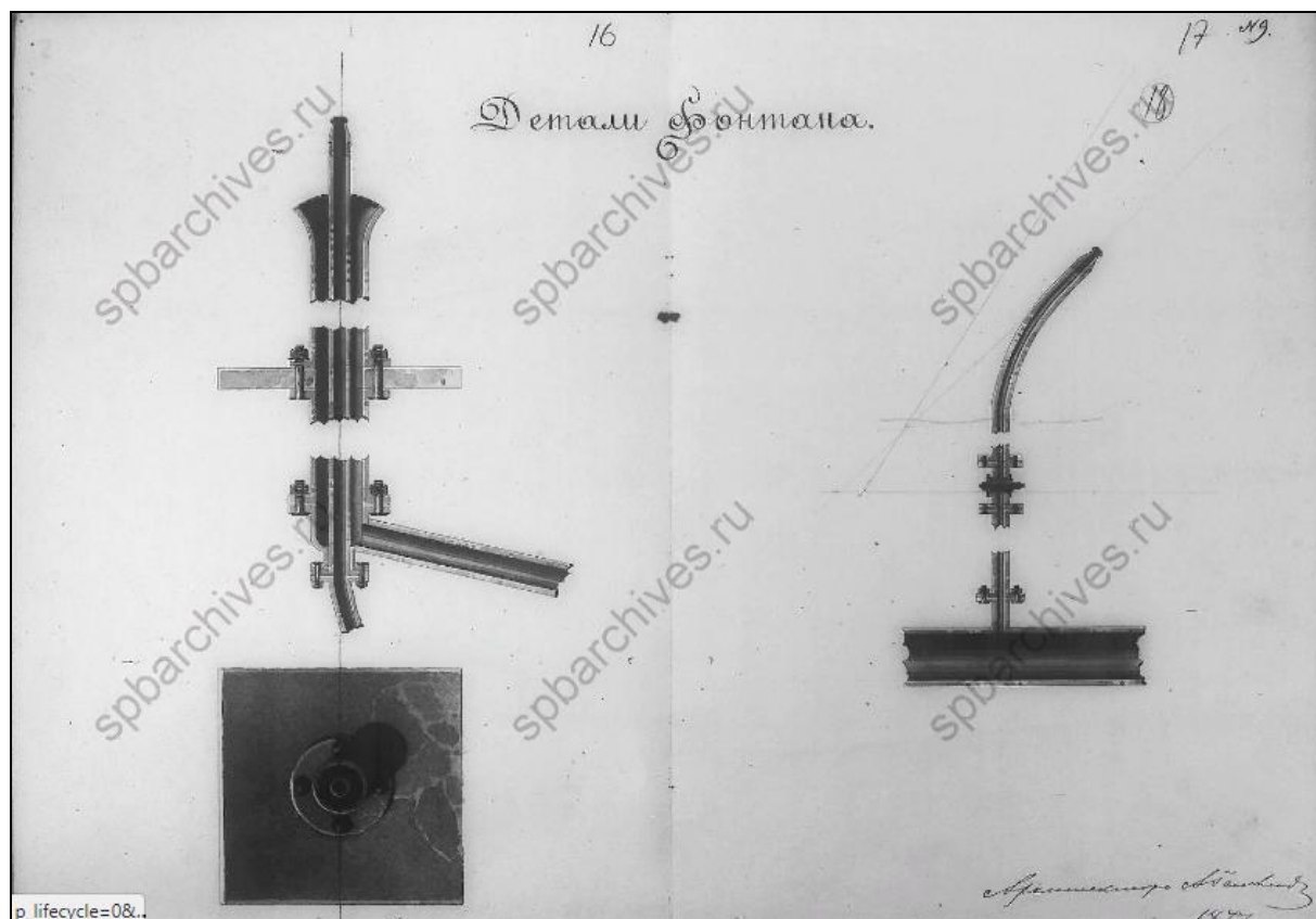
11. Детали фонтана. 1877 г. Арх. А. Р. Гешвенд. ЦГИА СПб. Ф. 513. Оп. 118. Д. 321. Л. 16–17.
