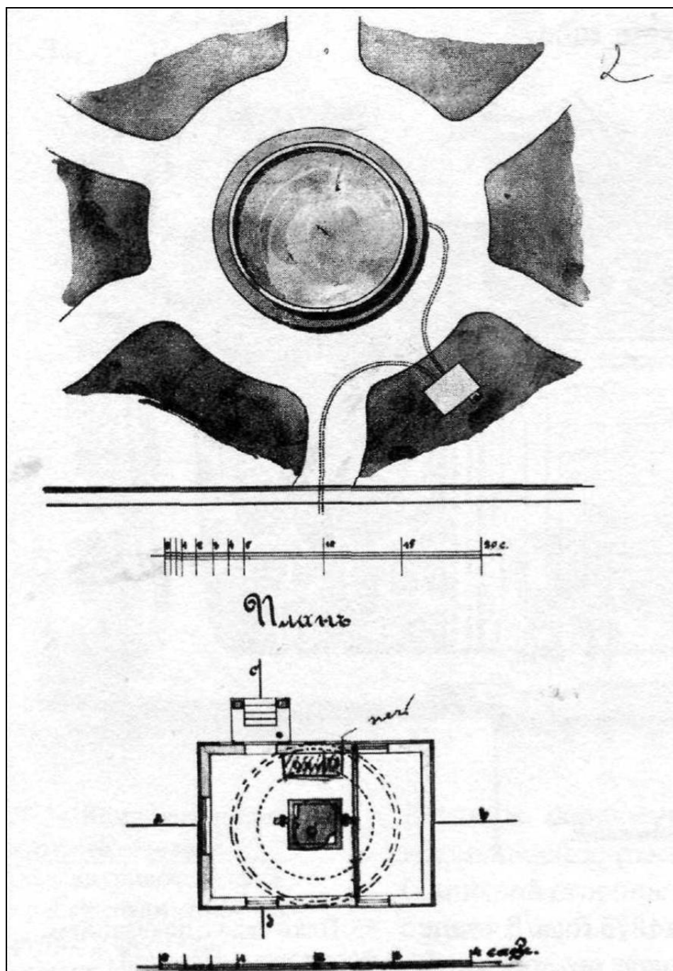
17. Фрагмент Александровского сада с показанием места постройки сторожевого домика с водомером и план домика. 1881 г. Из книги: Веснина Н. Н. Сады Невского проспекта. СПб., 2008. С. 48.
