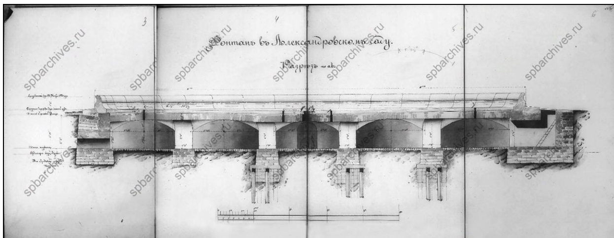
8. Фонтан в Александровском саду. Разрез по аб. 1876 г. Арх. А. Р. Гешвенд. ЦГИА СПб. Ф. 513. Оп. 118. Д. 321. Л. 3–5.
