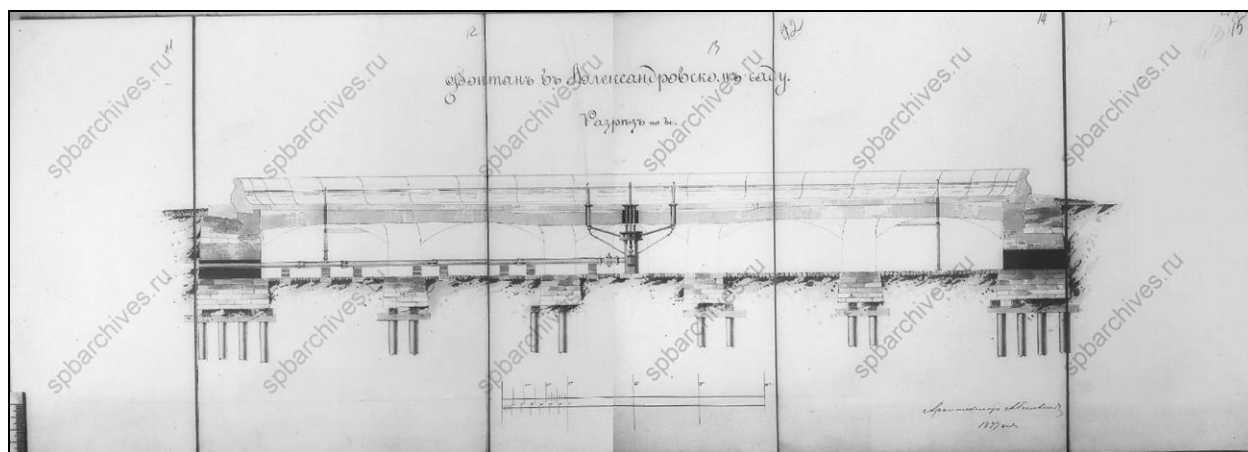
10. Фонтан в Александровском саду. Разрез по в. 1877 г. Арх. А. Р. Гешвенд. ЦГИА СПб. Ф. 513. Оп. 118. Д. 321. Л. 11–15.
