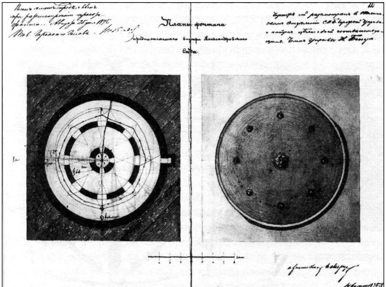
6. План предполагаемого фонтана Александровского сада, одобренный Техническим отделением Горуправы. 1875 г. И. А. Мерц. Из книги: Веснина Н. Н. Сады Невского проспекта. СПб., 2008. С. 45.
