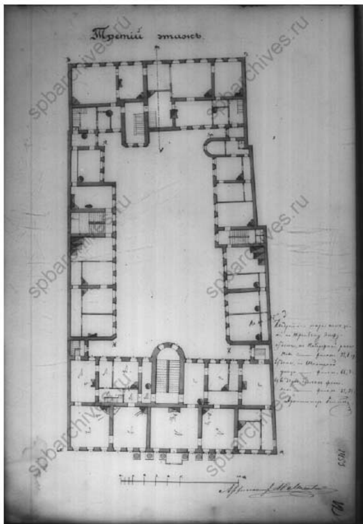
Илл. 29. План 3-го этажа. 1866 г. (источник: ЦГИА СПб. Ф. 515 Оп. 4. Д. 394-1).
