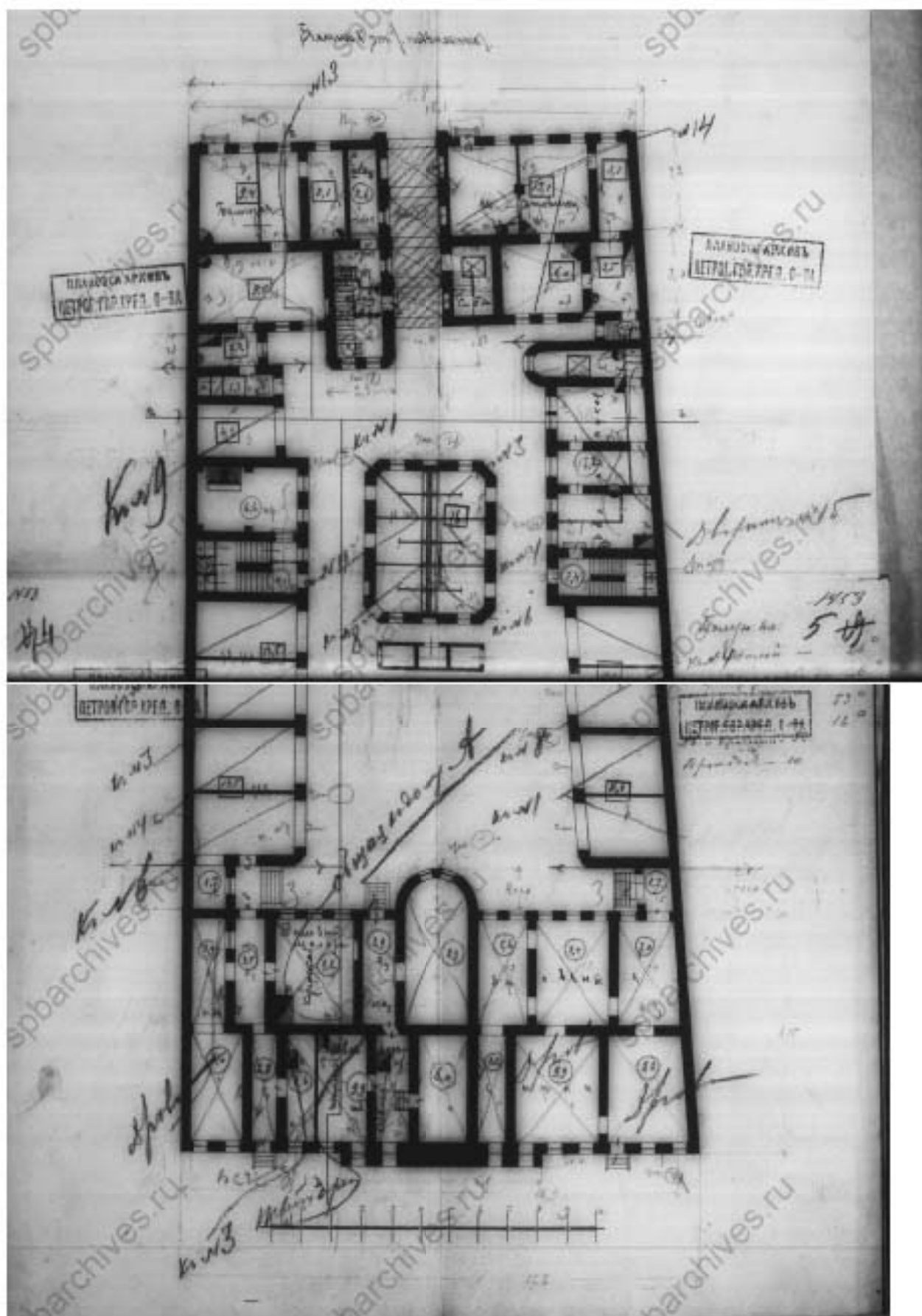
Илл. 38. План 1-го этажа (подвального). 1915 г. (источник: ЦГИА СПб. Ф. 515 Оп. 4. Д. 394-2).
