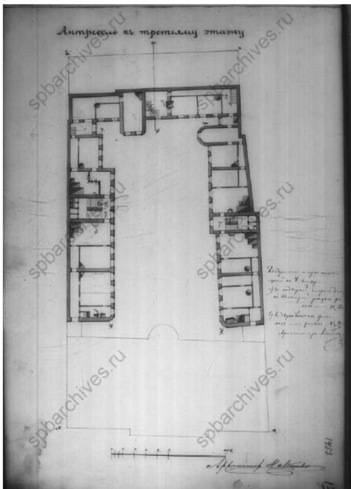
Илл. 30. План антресоли к 3-му этажу. 1866 г. (источник: ЦГИА СПб. Ф. 515 Оп. 4. Д. 394-1).
