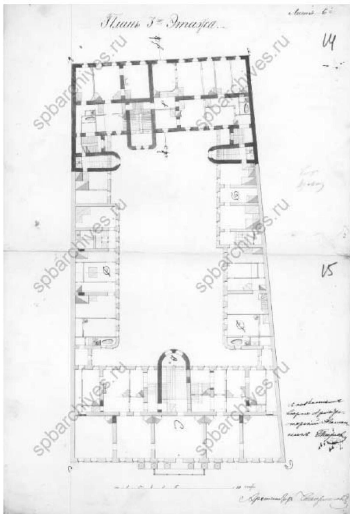
Илл. 9. Проектный план 3-го этажа. 1855 г. (источник: ЦГИА СПб. Ф. 513. Оп. 102. Д. 4558).
