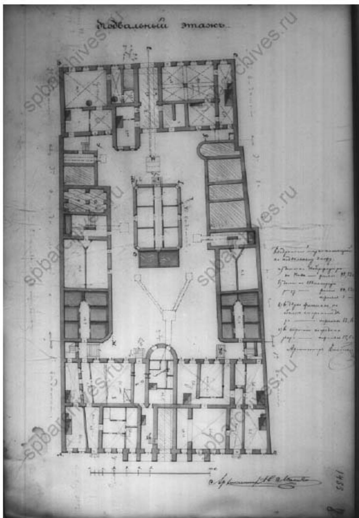
Илл. 25. План подвального этажа. 1866 г. (источник: ЦГИА СПб. Ф. 515 Оп. 4. Д. 394-1).
