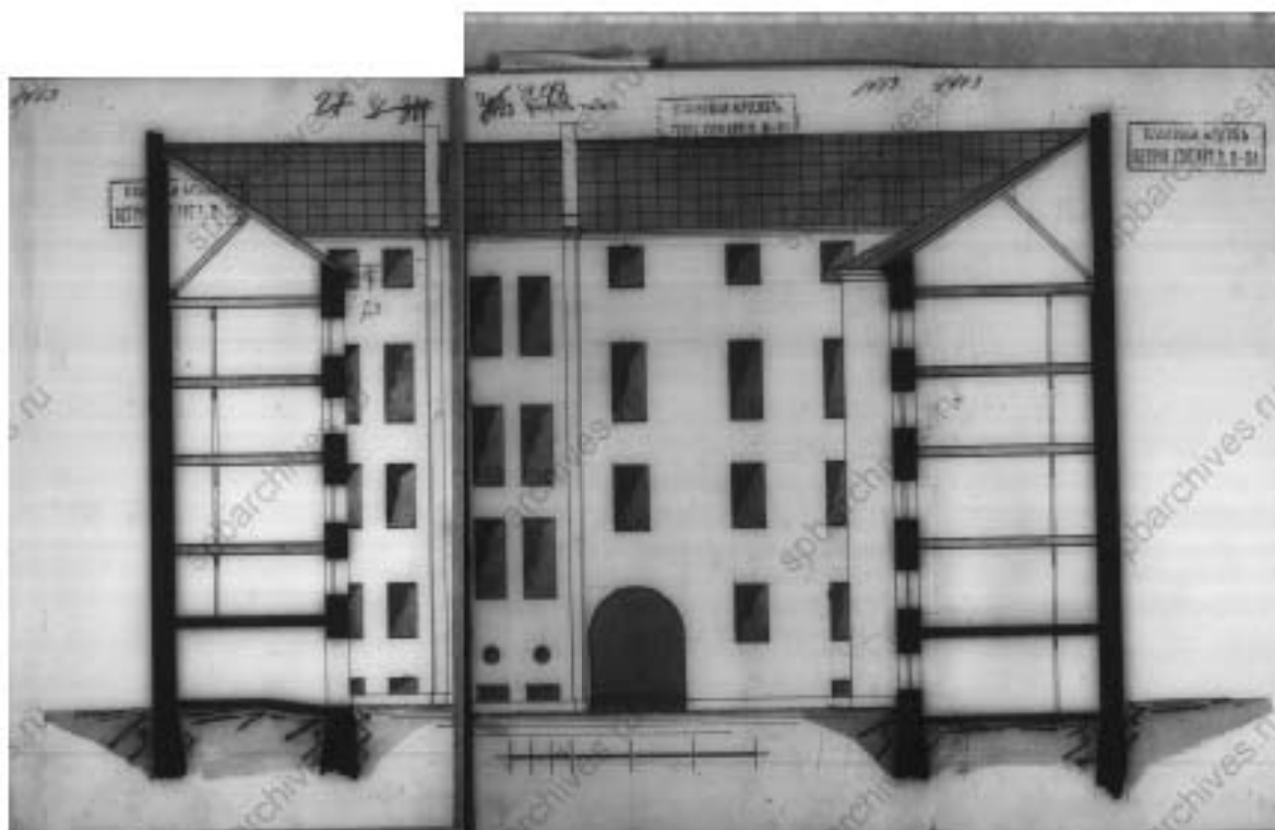
Илл. 36. Фасад лицевого корпуса по Шпалерной улицы со стороны двора. 1915 г. (источник: ЦГИА СПб. Ф. 515 Оп. 4. Д. 394-2).
