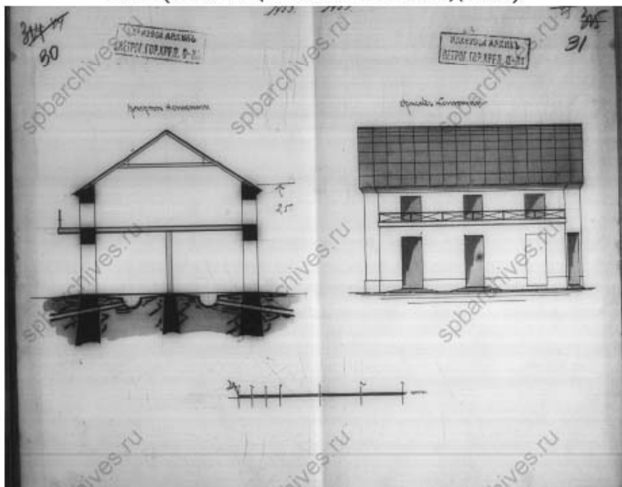
Илл. 37. Фасад и разрез конюшни. 1915 г. (источник: ЦГИА СПб. Ф. 515 Оп. 4. Д. 394-2).
