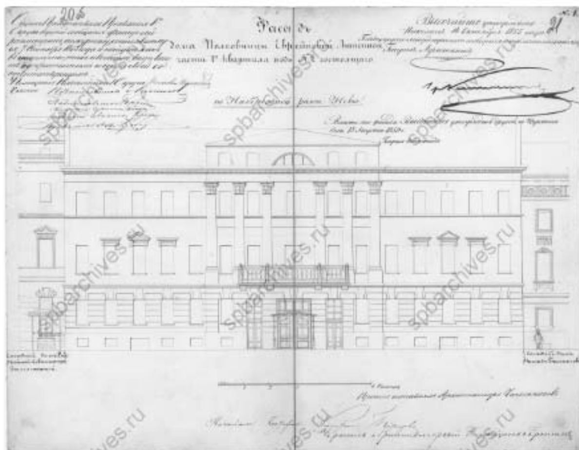
Илл. 15. Фасад дома Полковницы Евреиновой Литейной части 1-го квартала под № 15/7 по набережной реки Невы. 1855 г. (источник: ЦГИА СПб. Ф. 513. Оп. 102. Д. 4558).
