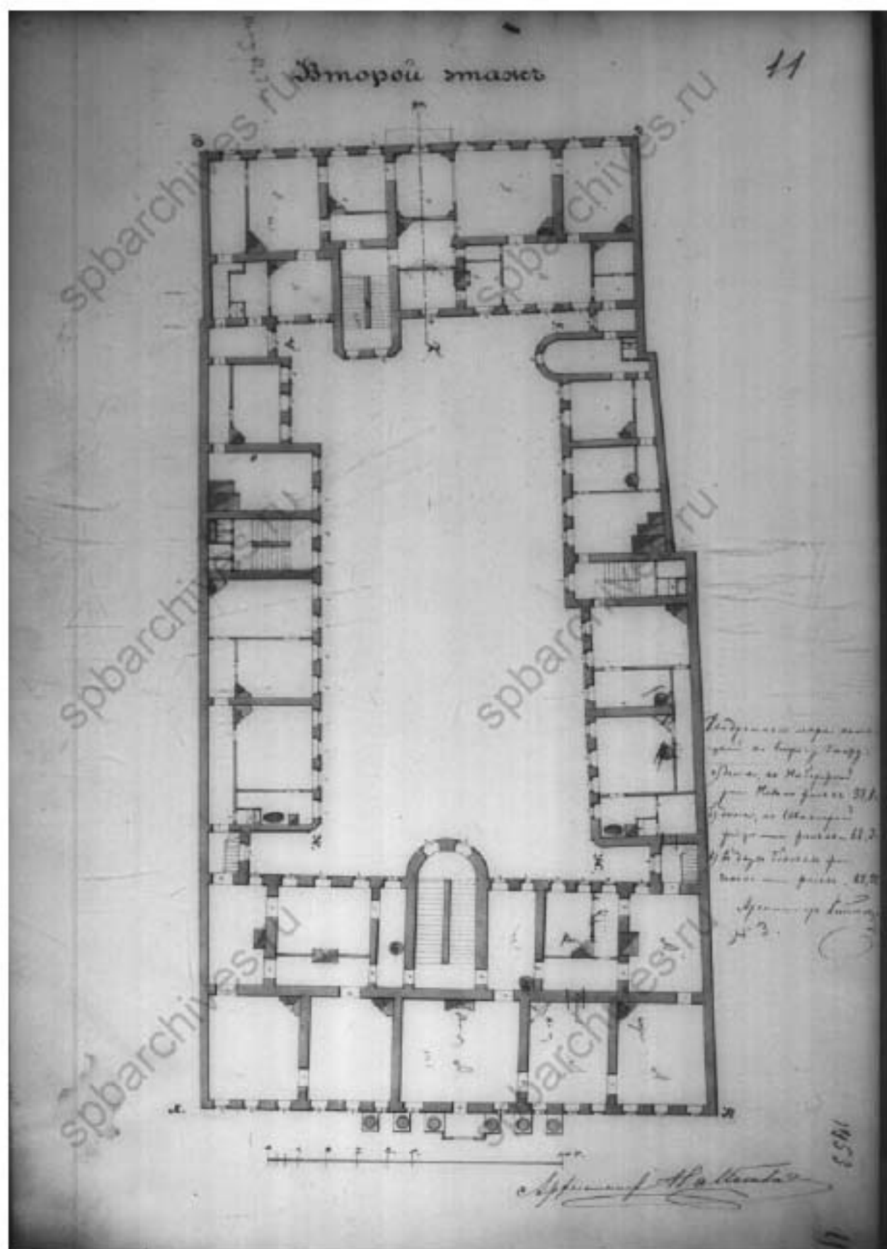
Илл. 28. План 2-го этажа. 1866 г. (источник: ЦГИА СПб. Ф. 515 Оп. 4. Д. 394-1).
