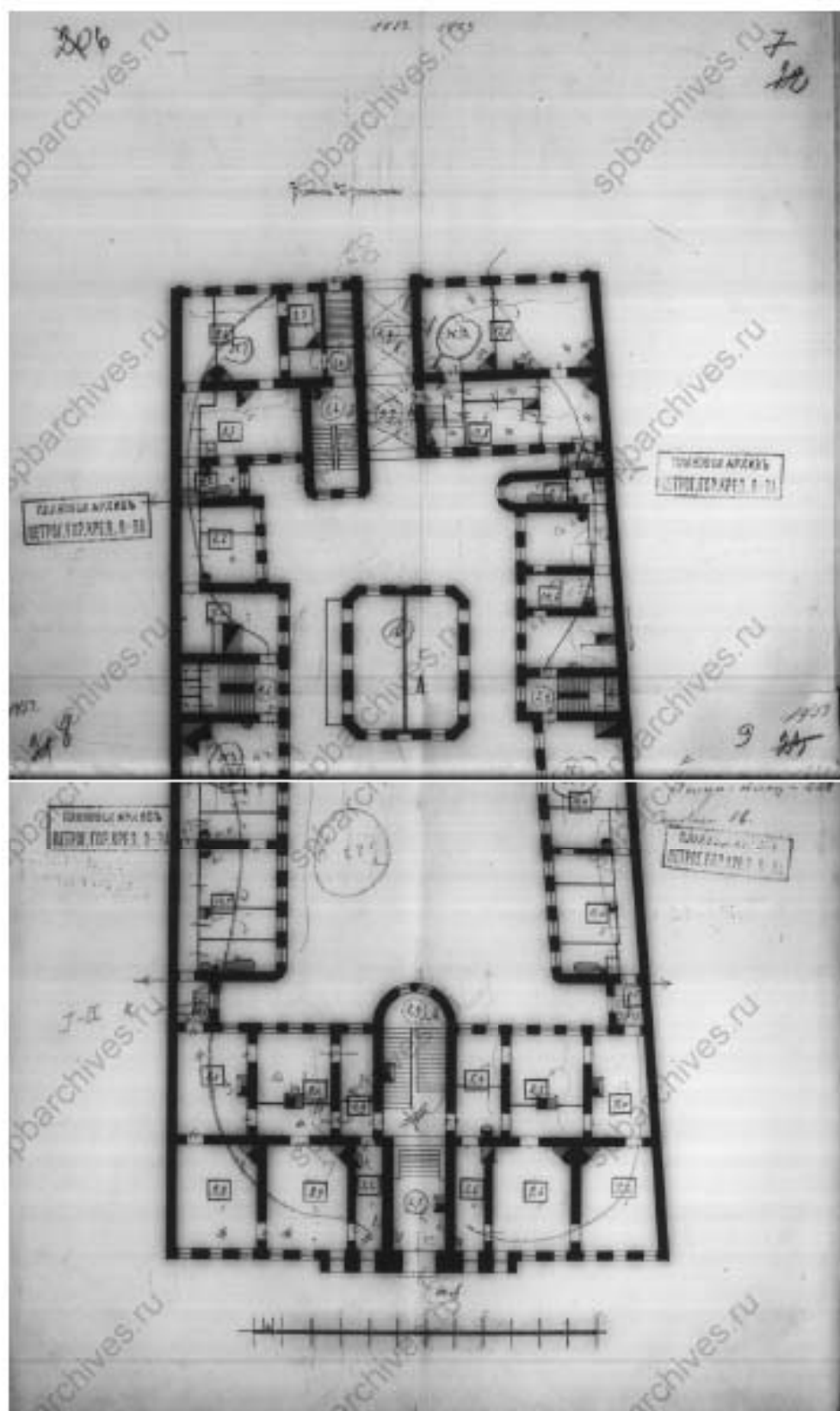
Илл. 39. План 2-го этажа. 1915 г. (источник: ЦГИА СПб. Ф. 515 Оп. 4. Д. 394-2).
