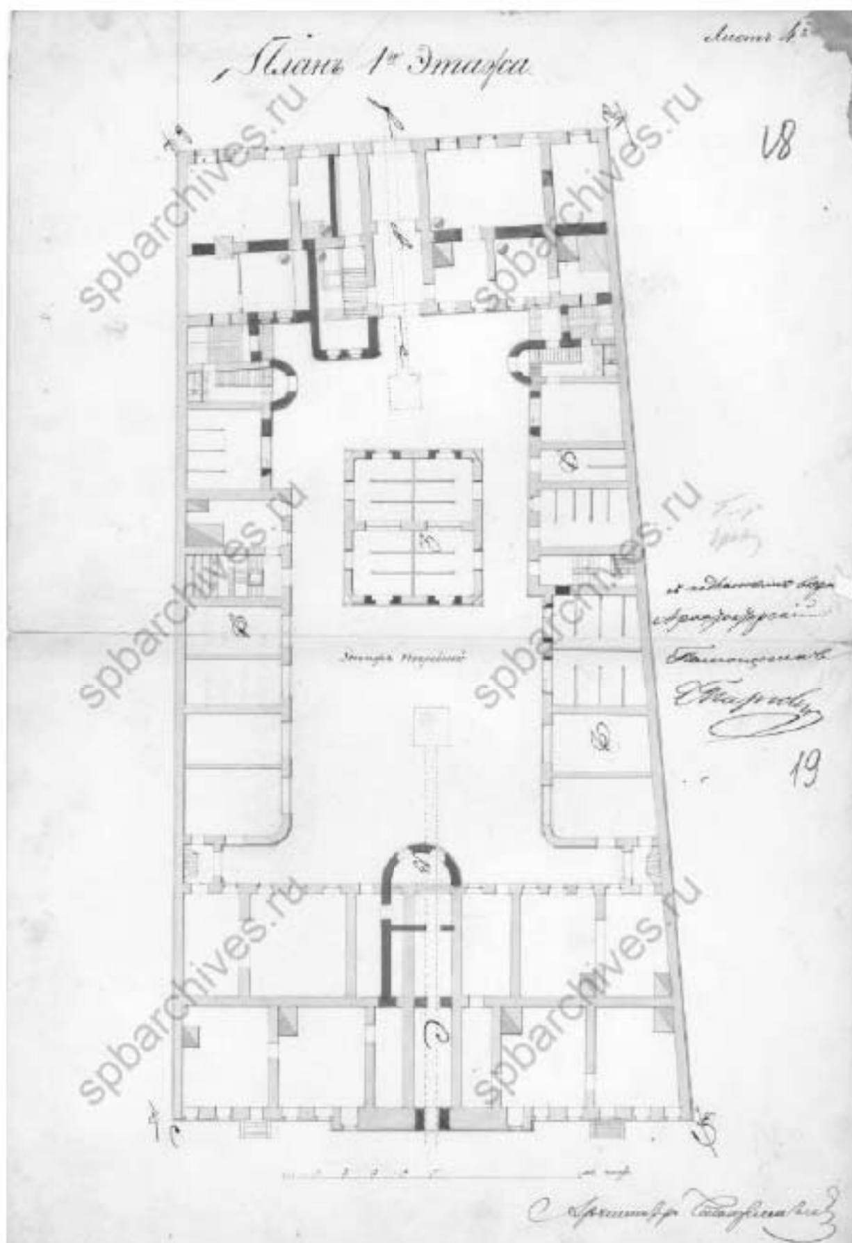
Илл. 7. Проектный план 1-го этажа. 1855 г. (источник: ЦГИА СПб. Ф. 513. Оп. 102. Д. 4558).
