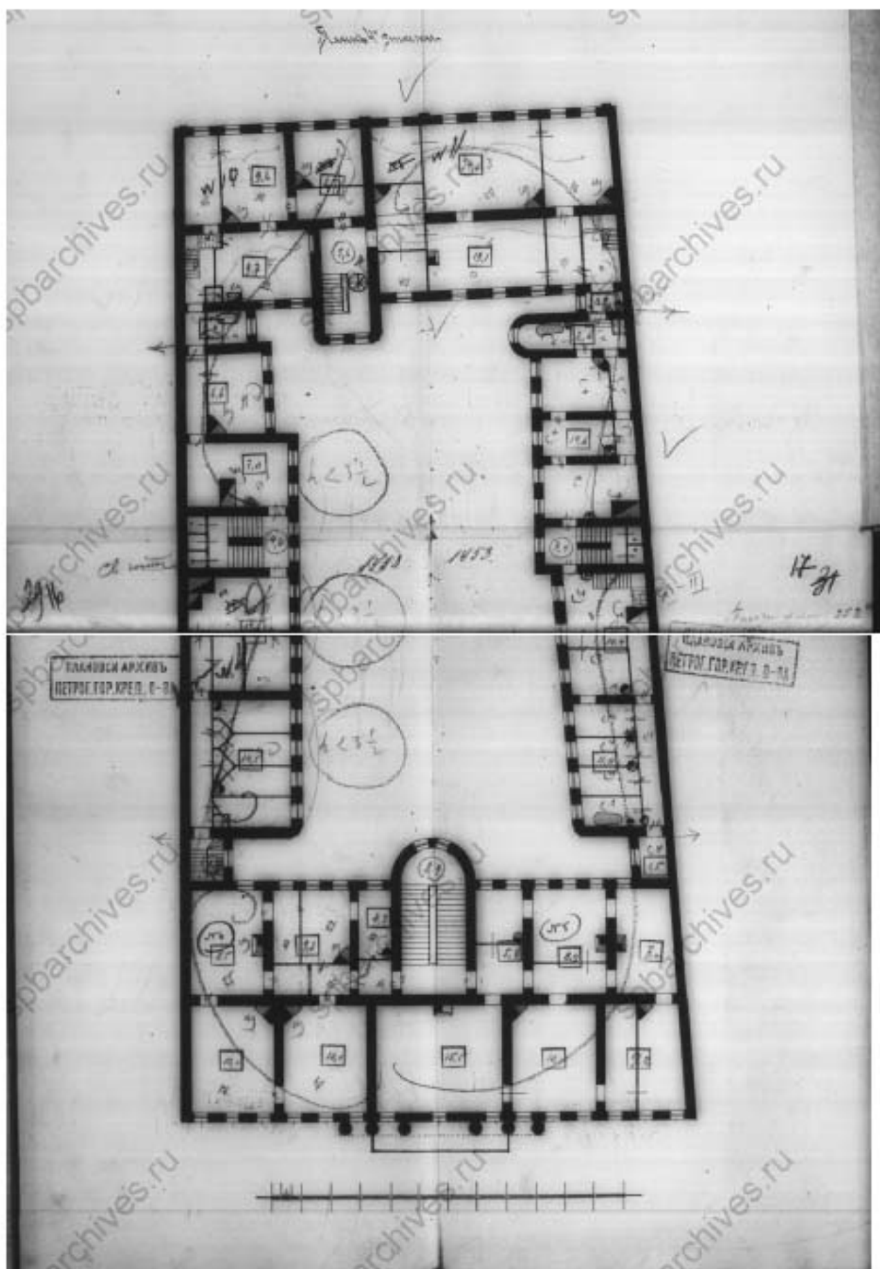
Илл. 41. План 4-го этажа. 1915 г. (источник: ЦГИА СПб. Ф. 515 Оп. 4. Д. 394-2).
