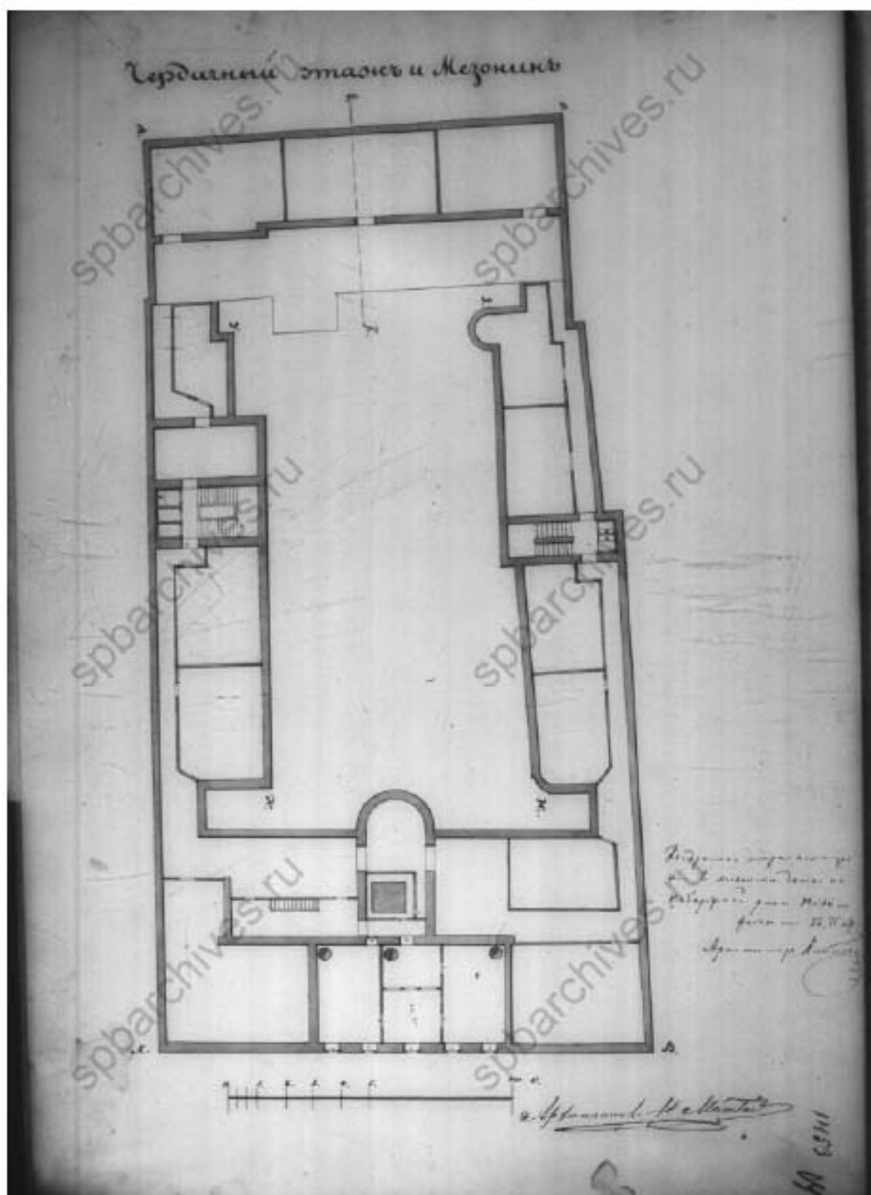
Илл. 31. План чердачного этажа и мезонина. 1866 г. (источник: ЦГИА СПб. Ф. 515 Оп. 4. Д. 394-1).
