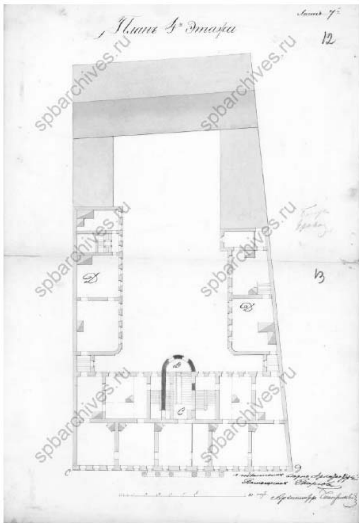
Илл. 10. Проектный план 4-го этажа. 1855 г. (источник: ЦГИА СПб. Ф. 513. Оп. 102. Д. 4558).
