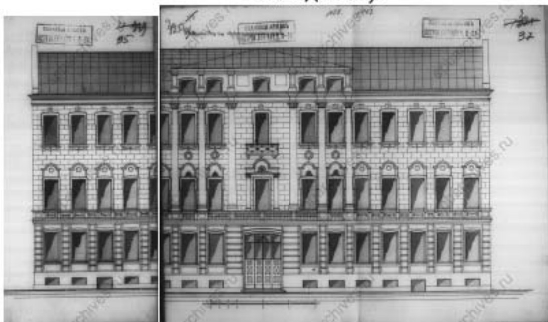
Илл. 34. Фасад по Французской набережной. 1915 г. (источник: ЦГИА СПб. Ф. 515 Оп. 4. Д. 394-2).
