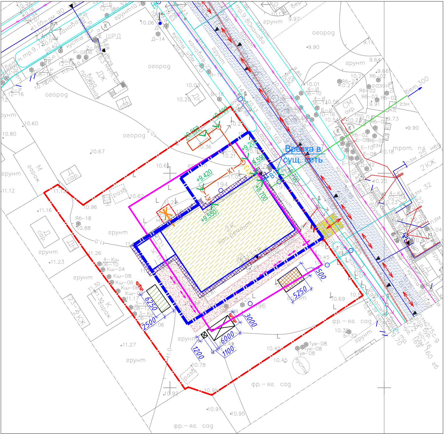
Стройгенплан. М 1:500
