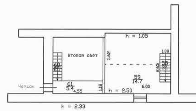
План антресоли
