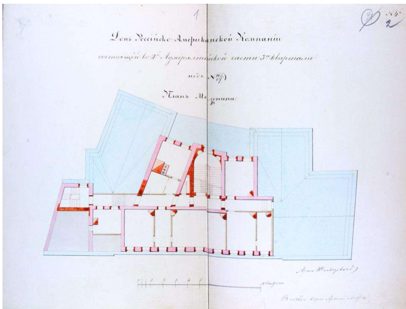
17. Проект перестройки лицевого и дворового флигеля, благоустройства двора. План мезонина. 1853г. Архитектор Р.А. Желязевич. ЦГИА СПб. Ф. 513. Оп. 102. Д. 3383. Л. 1–2.
