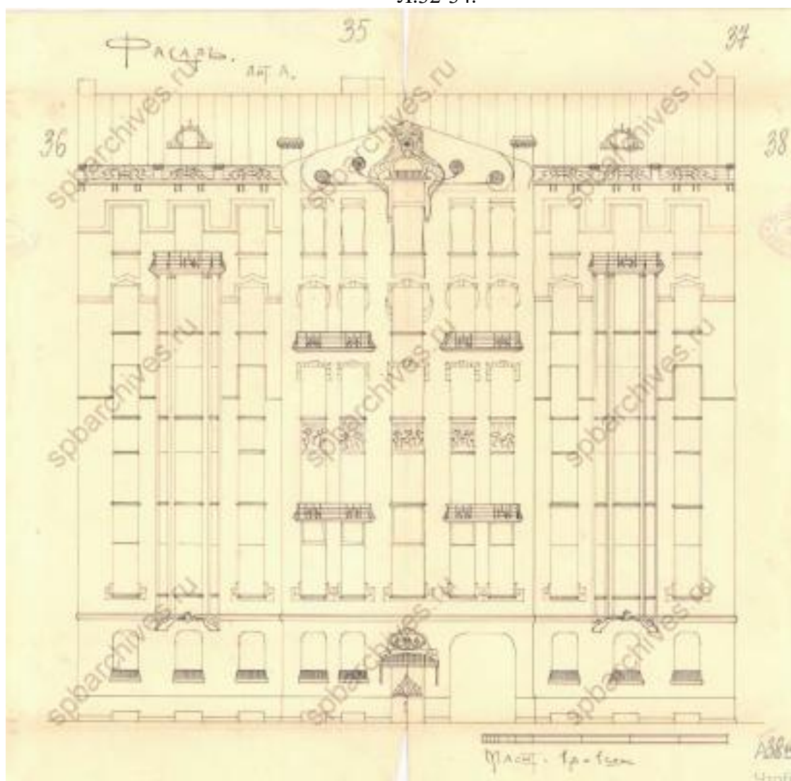
12. План лицевого фасада вновь возводимого здания на участке 70 15-й линии В.О. по проекту, утв. 15 апреля 1910 г. ЦГИА СПб. Ф.513. Оп.102. Д.1928. Л.35-38.
