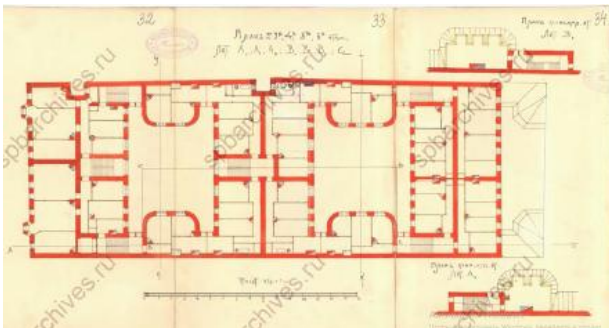
11. План 2, 3, 4, 5, 6 этажей и мансрды вновь возводимого здания на участке 70 15-й линии В.О. по проекту, утв. 15 апреля 1910 г. ЦГИА СПб. Ф.513. Оп.102. Д.1928. Л.32-34.
