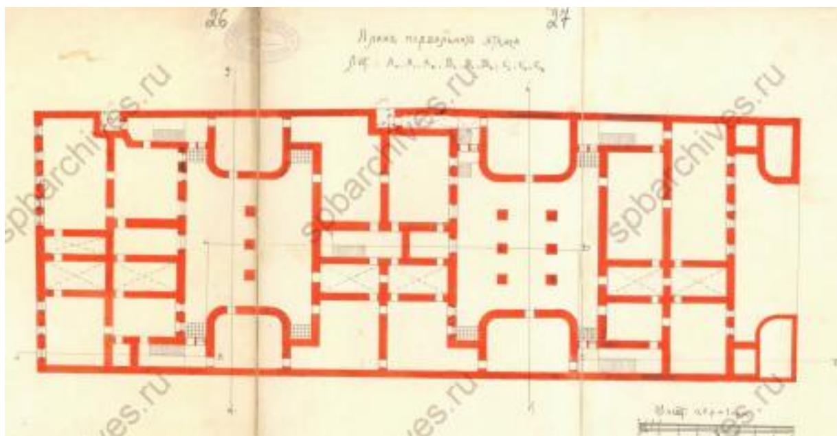
9. План подвала вновь возводимого здания на участке 70 15-й линии В.О. по проекту, утв. 15 апреля 1910 г. // ЦГИА СПб. Ф.513. Оп.102. Д.1928. Л.26-28.
