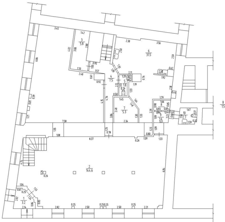
План 1-го этажа
