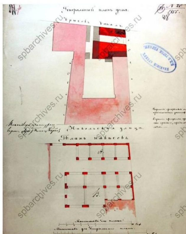
Илл. 12. Генеральный план дома почтенного Гражданина Игнатия Лесникова, состоящий во 2-й Адмиралтейской части 4-го кв., под № 180. 1855 г. ЦГИА СПб. Ф. 513. Оп. 102. Д. 3352. Л. 48.
