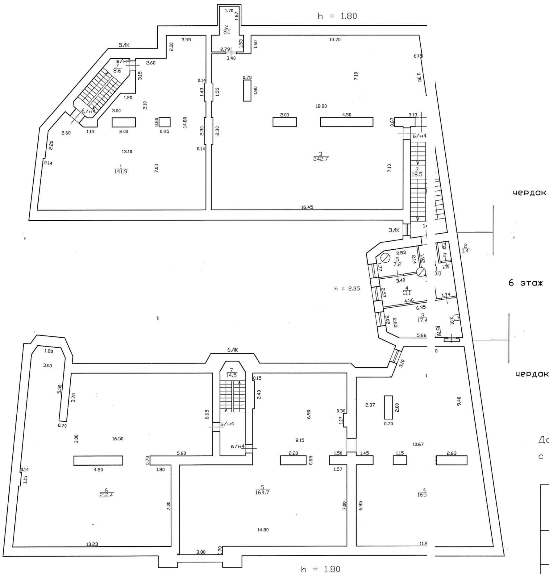
План 6 этажа и чердака
