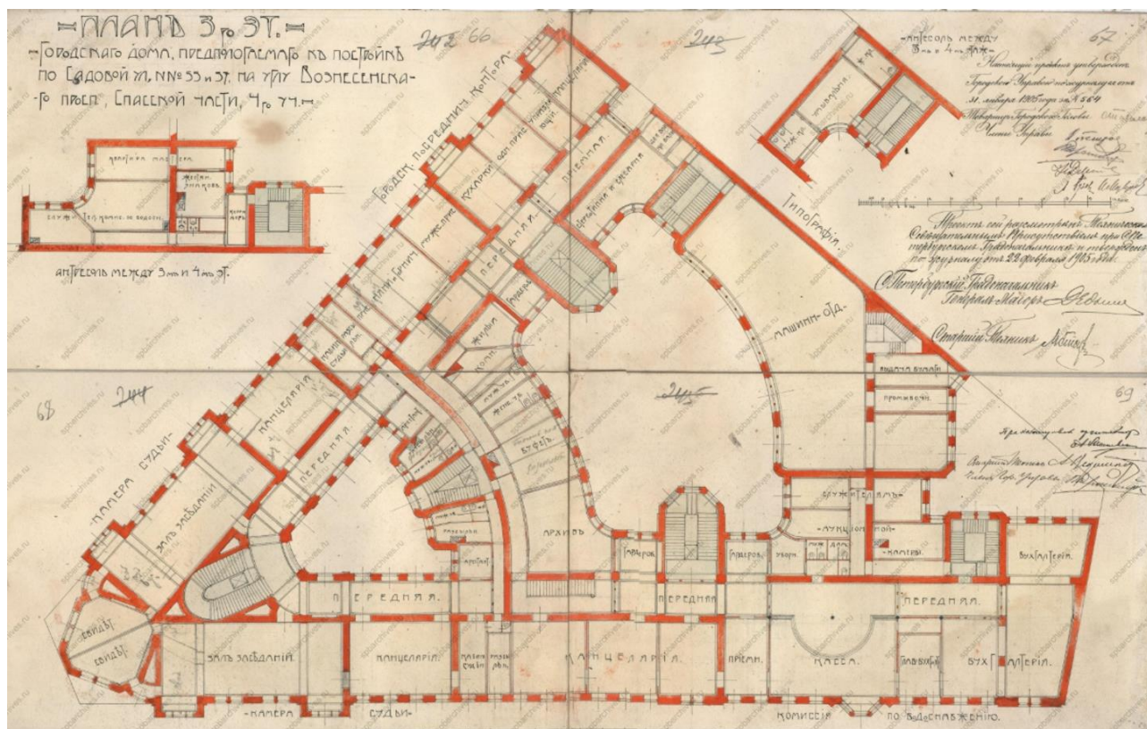
9. План 3-го этажа Городского дома. 22.02.1905. Проект арх. Лишневого. ЦГИА СПб. Ф.503. Оп.101. Д.587. Л.66-67
