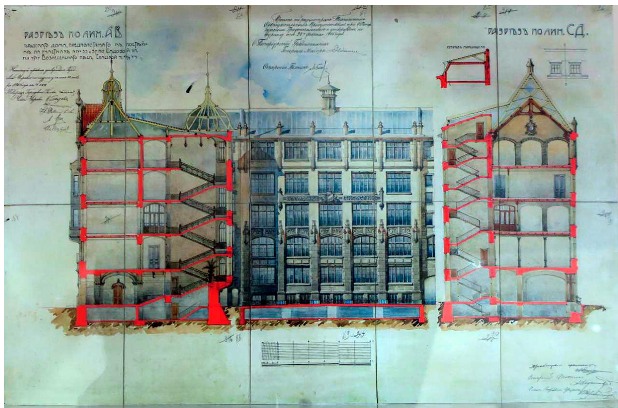
7. Фасад и разрез по Вознесенскому пр. 22.02.1905. Проект арх. Лишневаго. ЦГИА СПб. Ф.503. Оп.101. Д.587. Л.82-91.
