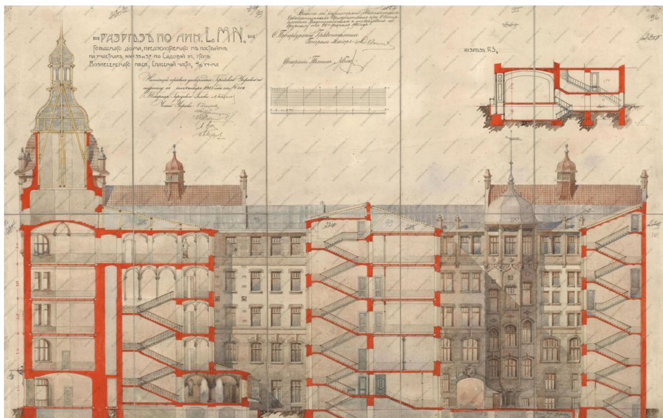
8. Разрез по линии LMN. 22.02.1905. Проект арх. Лишневаго. ЦГИА СПб. Ф.503. Оп.101. Д.587. Л.93-96.
