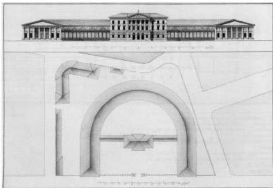
Илл. 1. Фасад по Садовой улице и генеральный план Ассигнационного банка. / Джакомо Кваренги. Архитектурная графика. - СПб: Март, 1998. С. 26.
