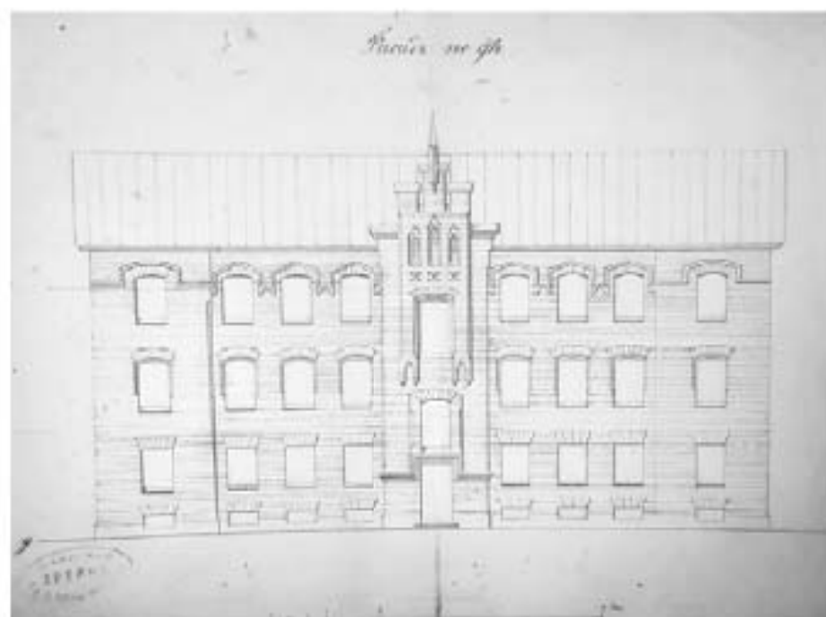
28. Проект фасада здания на участке, принадлежащем Алексею Ивановичу Глинкову, состоящей наб. Обводного канала Нарвской части 3 участка № 134. 1872 г.
