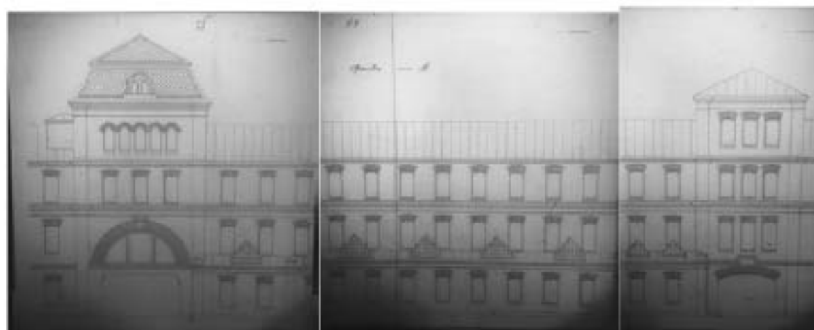
32. Проект одноэтажной пристройки к существующему корпусу лит. Е (совр. корп. 63). Дворовый фасад. 1902 г. Е. Гельман. ЦГИА СПб. Ф. 513. Оп. 102. Д. 5647 1. Лл. 79-81
