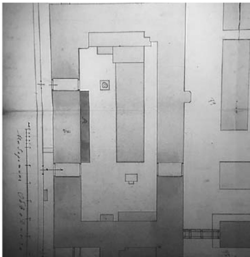
31. Проект одноэтажной пристройки к существующему корпусу лит. Е (совр. корп. 63). 1902 г. Е. Гельман. ЦГИА СПб. Ф. 513. Оп. 102. Д. 5647 1. Лл. 74-75
