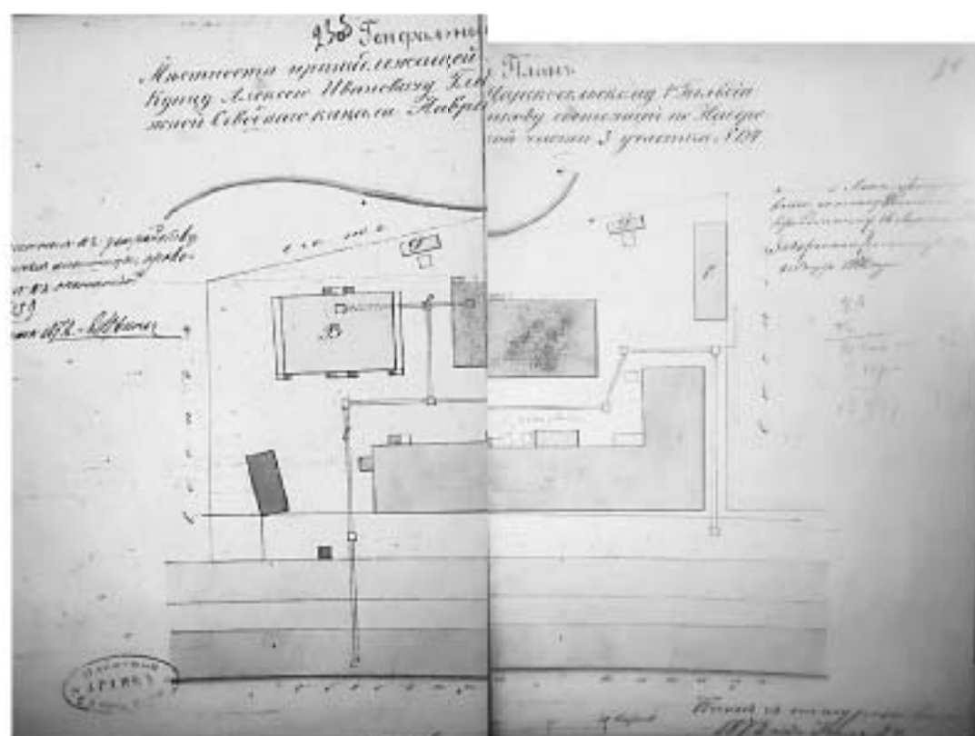
27. Генеральный план местности, принадлежащий царскосельской гильдии купцу Алексею Ивановичу Глинкову, состоящей наб. Обводного канала Нарвской части 3 участка № 134. 1872 г. Под лит. А – современный корпус поликлиники, расположенный в дворовой части.
