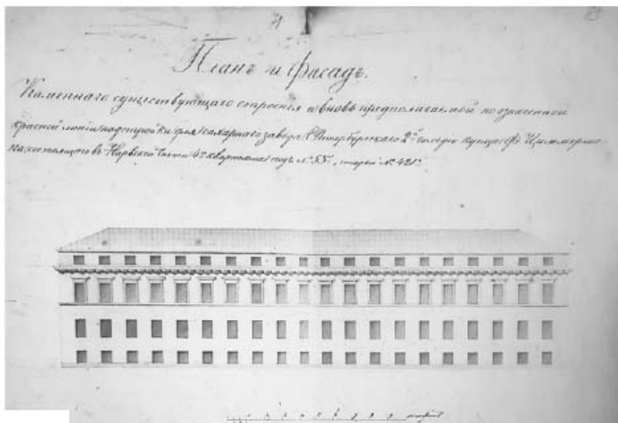
25. Проект надстройки здания. Чертеж лицевого фасада. 1840 г. Архитектор Г. Цолликофер. ЦГИА СПб. Ф. 513. Оп. 102. Д. 5684.
