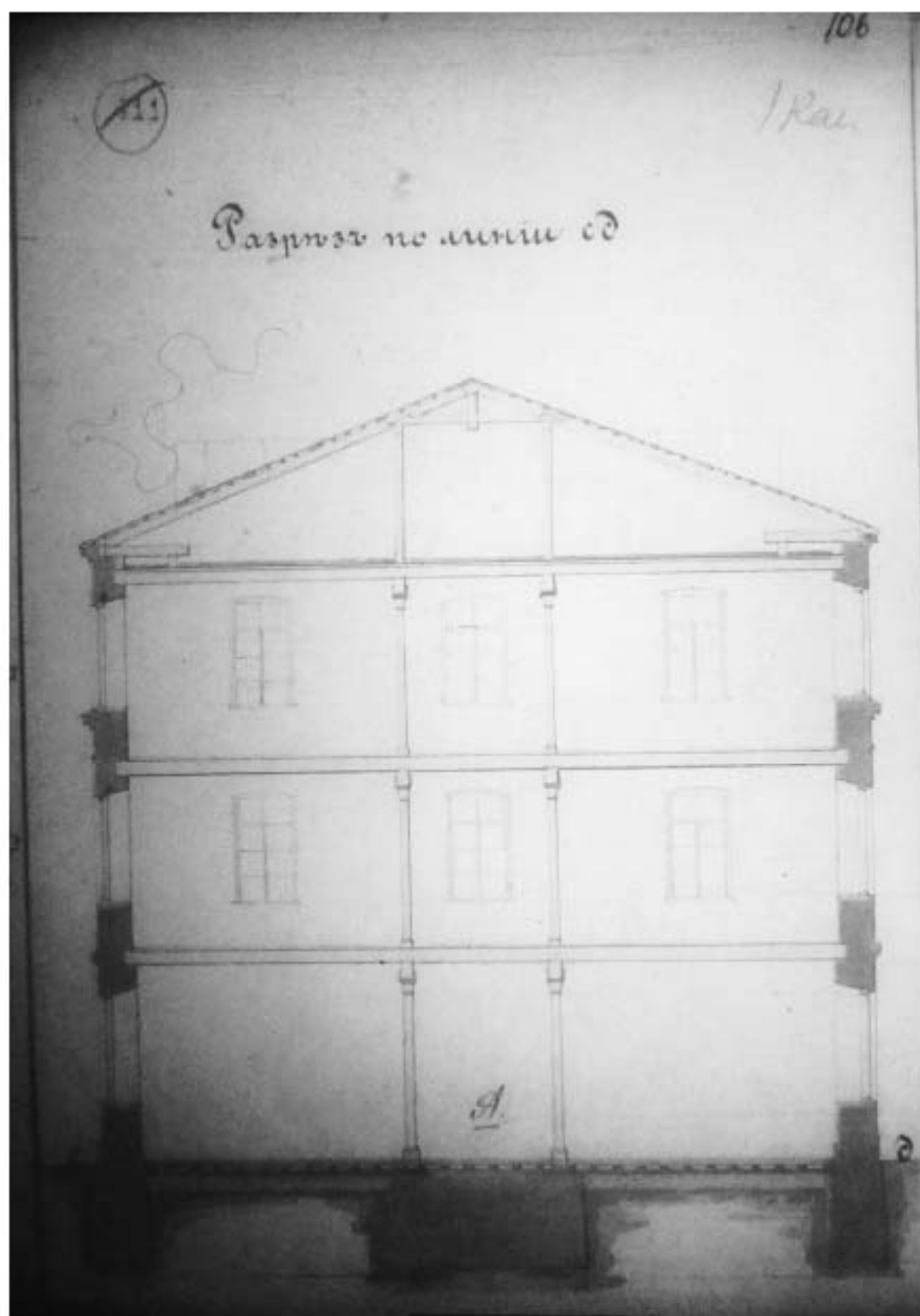
30. Проект перестройки корпуса Лит А 1 – совр. корпус 54, лит. А- совр. корпус 63. Разрез. Архитектор Р.Р. Генрихсен. 1868 г. ЦГИА СПб. Ф. 513. Оп. 102. Д. 5645. Л. 106
