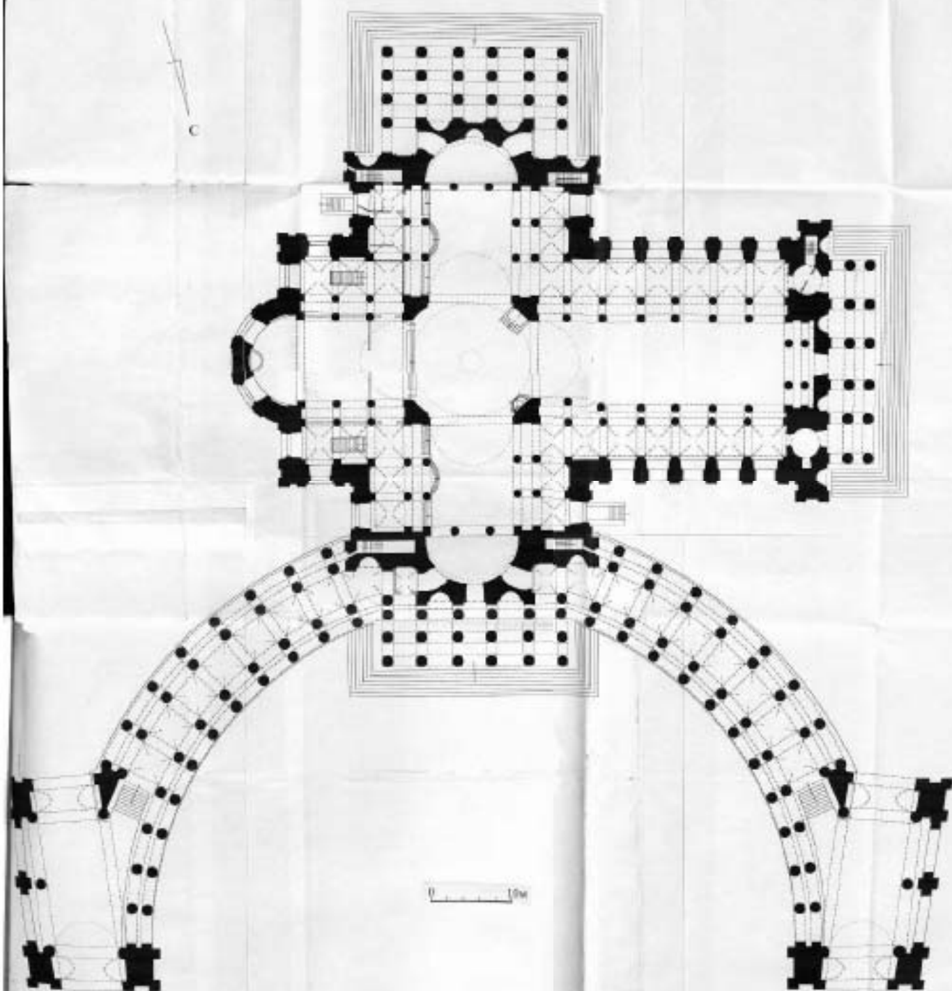
Санкт-Петербург, Центральный район, Коллежский вл. 2 Собор Казанской иконы Божией Матери (Жоакимов) 1801-1811 гг. План верхнего этажа
