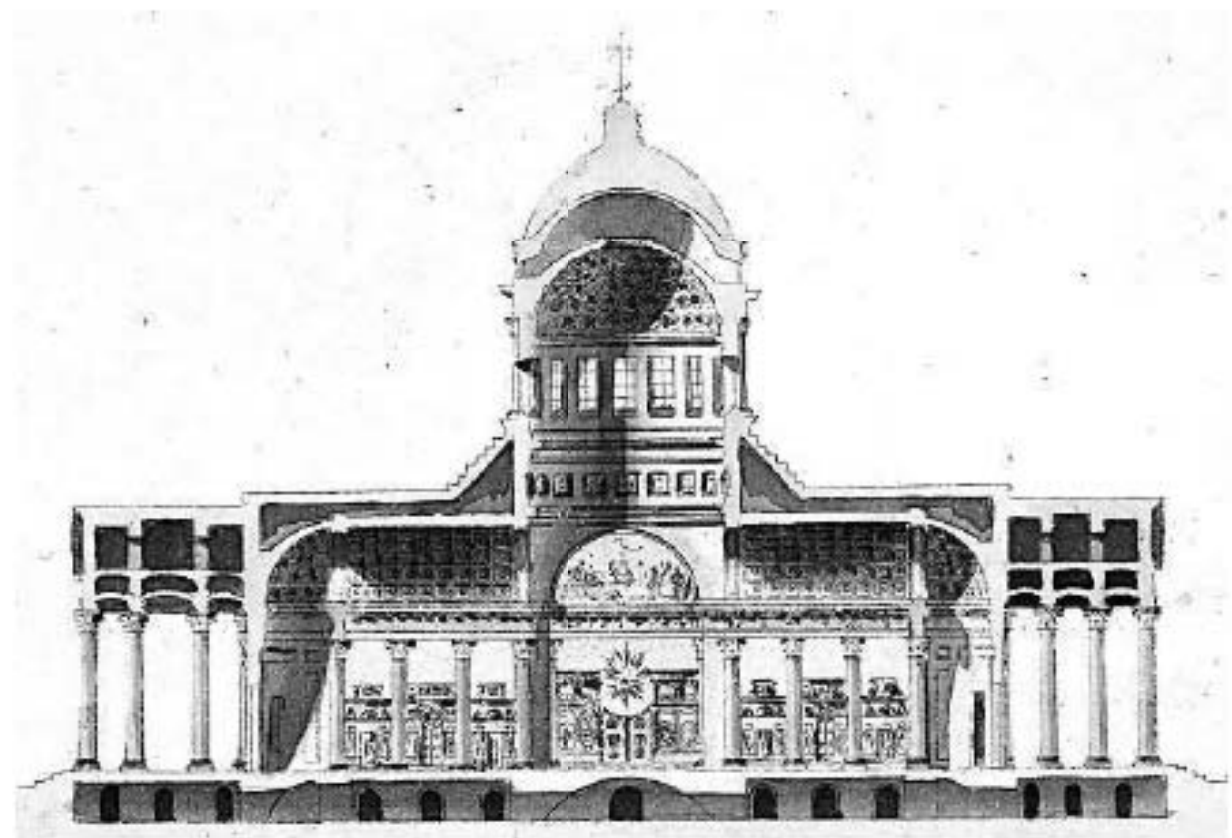
Илл. 6. Воронихин А. Н. Проект Казанского собора в Санкт-Петербурге. Поперечный разрез. 1800 г. Фрагмент. Государственный музей архитектуры им. А. В. Щусева. Инв. номер РІ-8337/3.
