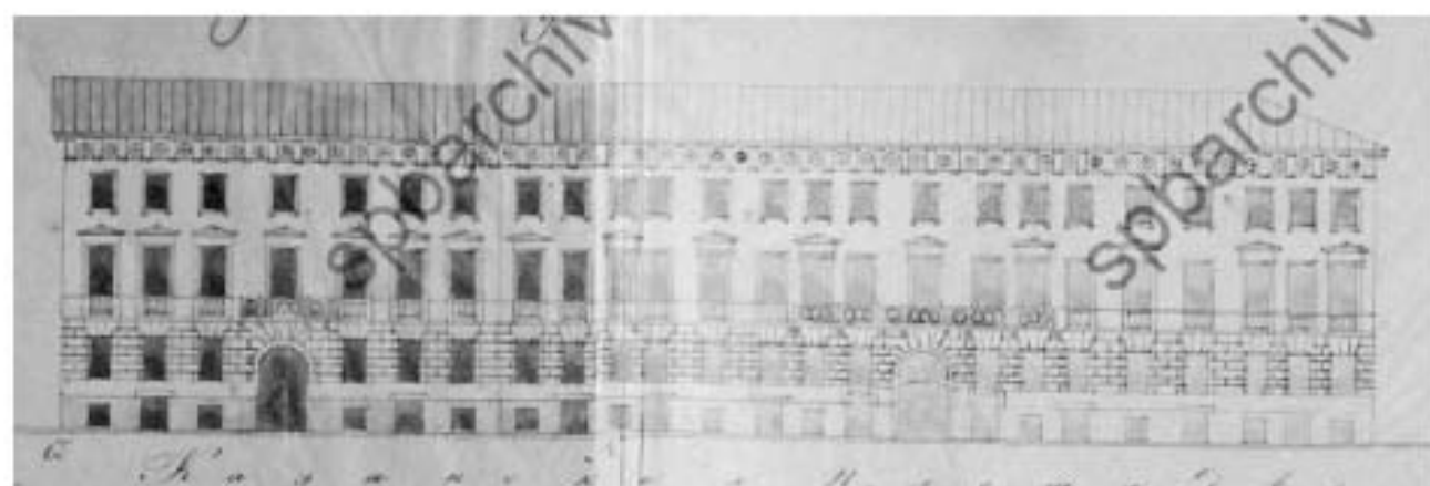
Илл. 25. Фасад и разрез флигеля (ЦГИА СПб ф.513 оп.102 д.3377А, л.41-44)
