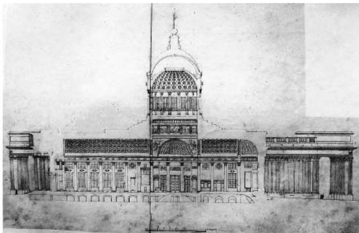
Илл. 15. Санкт-Петербург. Казанский собор. Обмерный чертеж продольного разреза. 1837 г. КТИОП СПб, А-873, ф. 38768.
