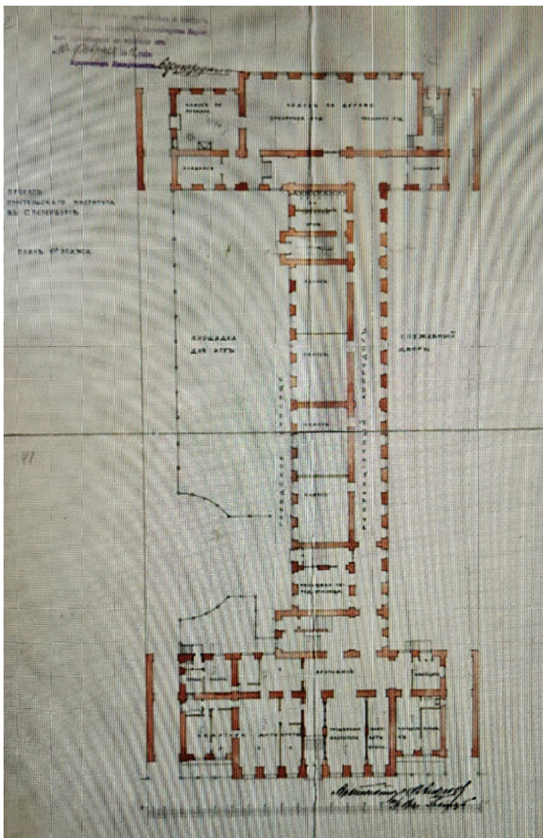
3. В.М. Андросов. Проект Санкт-Петербургского Учительского института. План первого этажа главного здания. 1912 г. (РГИА. Ф. 733. Оп. 178. Д. 45)
