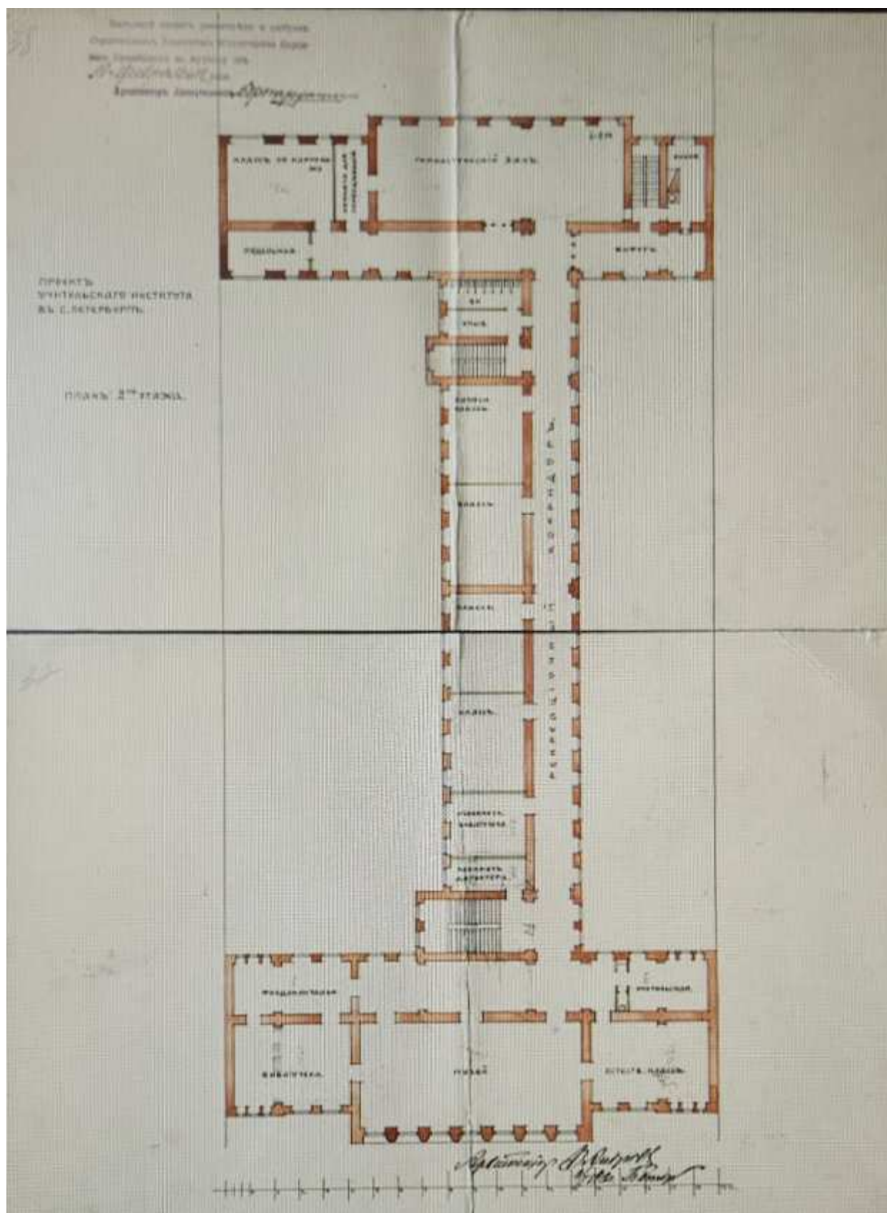
4. В.М. Андросов. Проект Санкт-Петербургского Учительского института. План второго этажа главного здания. 1912 г. (РГИА. Ф. 733. Оп. 178. Д. 45)
