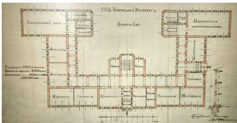
12. Л.П. Шишко. Проект Санкт-Петербургского Учительского института (нереализованный). План первого этажа главного здания. 1913 г. (РГИА. Ф. 733. Оп. 178. Д. 45)
