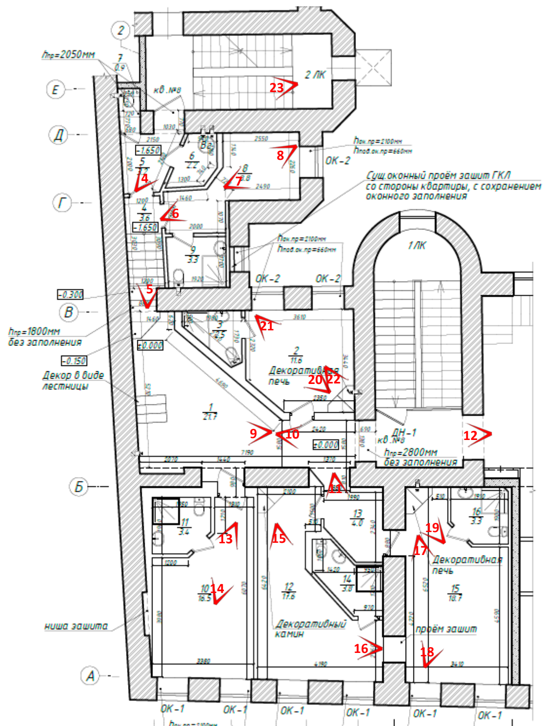
Рисунок 2. Схема фотофиксации на фрагменте плана 5 этажа
