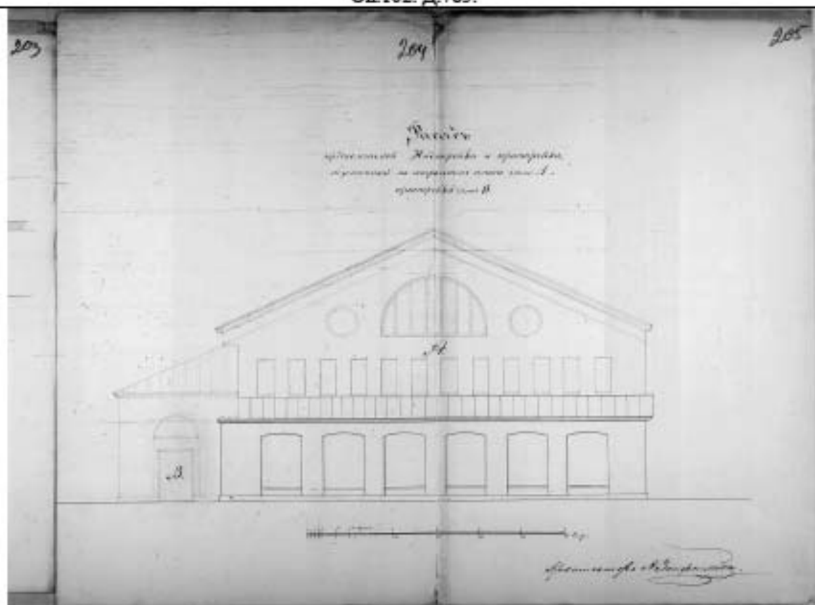
1875 г. Проект перестройки кочегарки. Торцевой фасад. 1-й вариант. Архитектор А. Ф.
