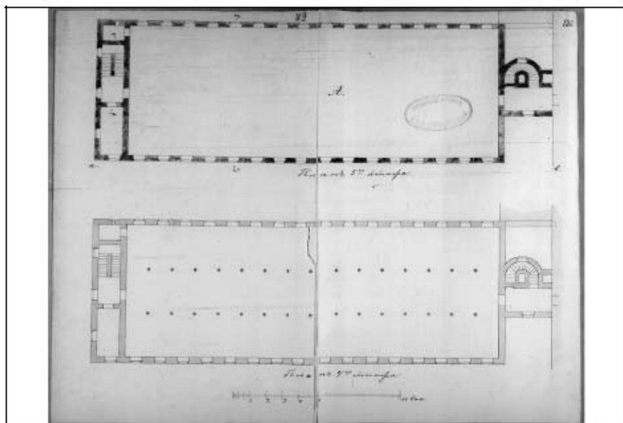
1888 г. Западный флигель. Проект надстройки 5-го этажа. Архитектор Н.А.Гаккель. ЦГИА СПб. Ф.513. Оп.102. Д.786.
