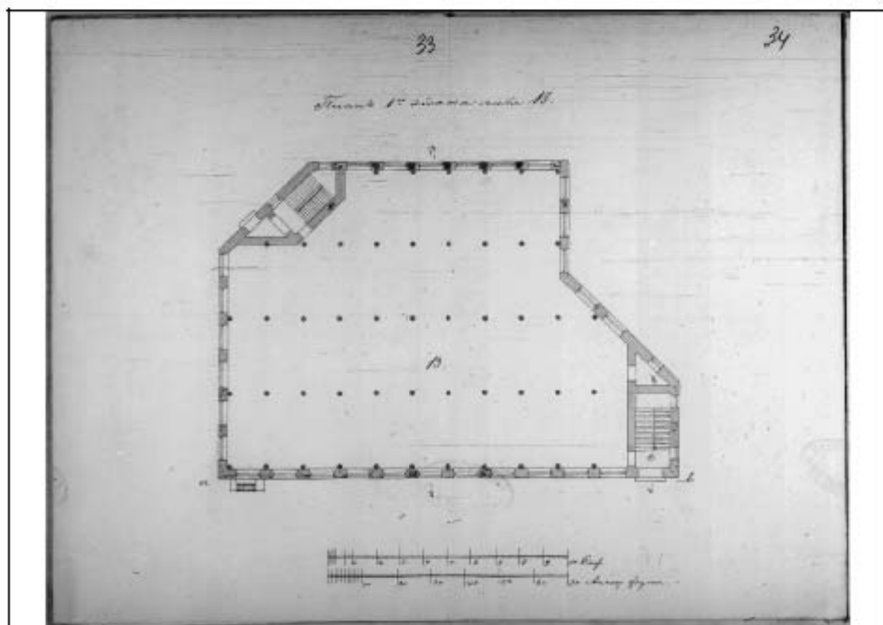
1899 г. План нового прядильного корпуса на месте газгольдера в каре основных корпусов. Не осуществлен. Архитектор Н.А.Гаккель. ЦГИА СПб. Ф.513. Оп.102. Д.786.
