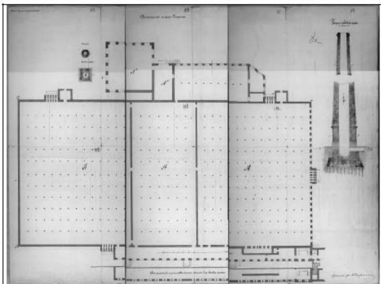
1869. План ткацкого корпуса. (север справа). Архитектор А. Ф. Занфтлебен. ЦГИА СПб. Ф. 513. Оп. 102. Д. 784.
