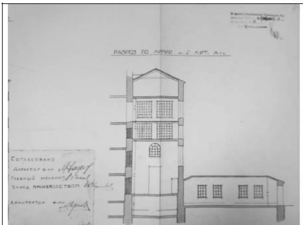
1927 г. Разрез по линии а-б корпусов А9 и А10 (утрачены). Архитектор А.М.Арнольд. ЦГАНТД. Ф. Р-192. Оп. 1-3. Д.2227.
