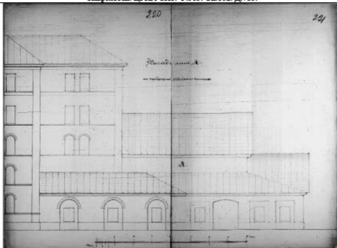
1875 г. Проект перестройки кочегарки. Лицевой фасад со стороны Обводного канала. Архитектор А.Ф. Занфтлебен. ЦГИА СПб. Ф.513. Оп.102. Д.785.
