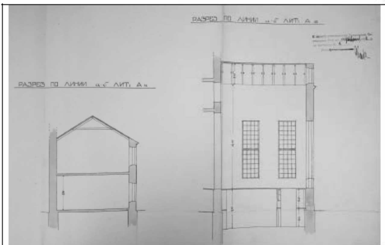
1927 г. Разрезы корпусов А16 и А15 (сохранились). Архитектор А.М.Арнольд. ЦГАНТД. Ф. Р-192. Оп. 1-3. Д.2227.
