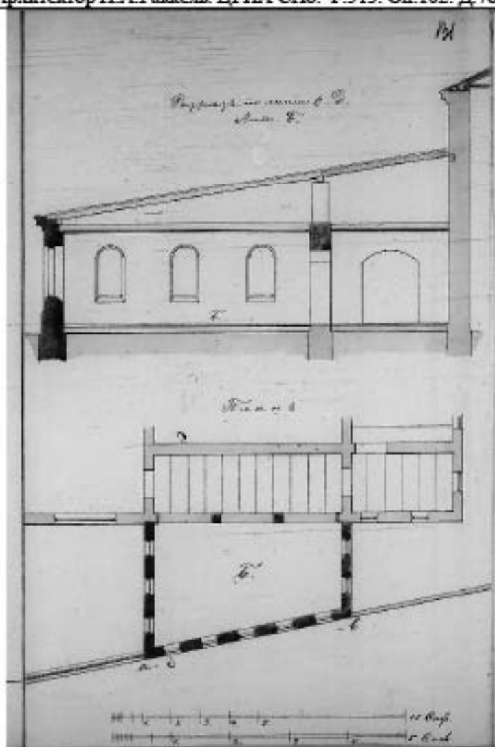
1888 г. Пристройка выступающей части Б, фасад а-б. План и разрез. Архитектор Н.А.Гаккель. ЦГИА СПб. Ф.513. Оп.102. Д.786.
