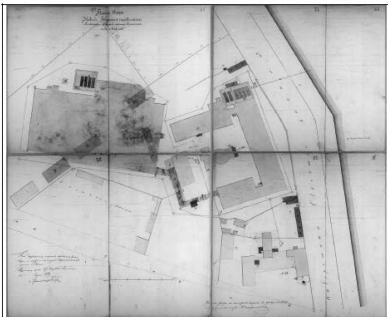
1869 г. План территории бумагопрядильни с приобретенным участком по Боровой улице и показанием его благоустройства и канализации и строительством нового ткацкого корпуса. Архитектор А. Ф. Занфтлебен. ЦГИА СПб. Ф. 513. Оп. 102. Д. 784.
