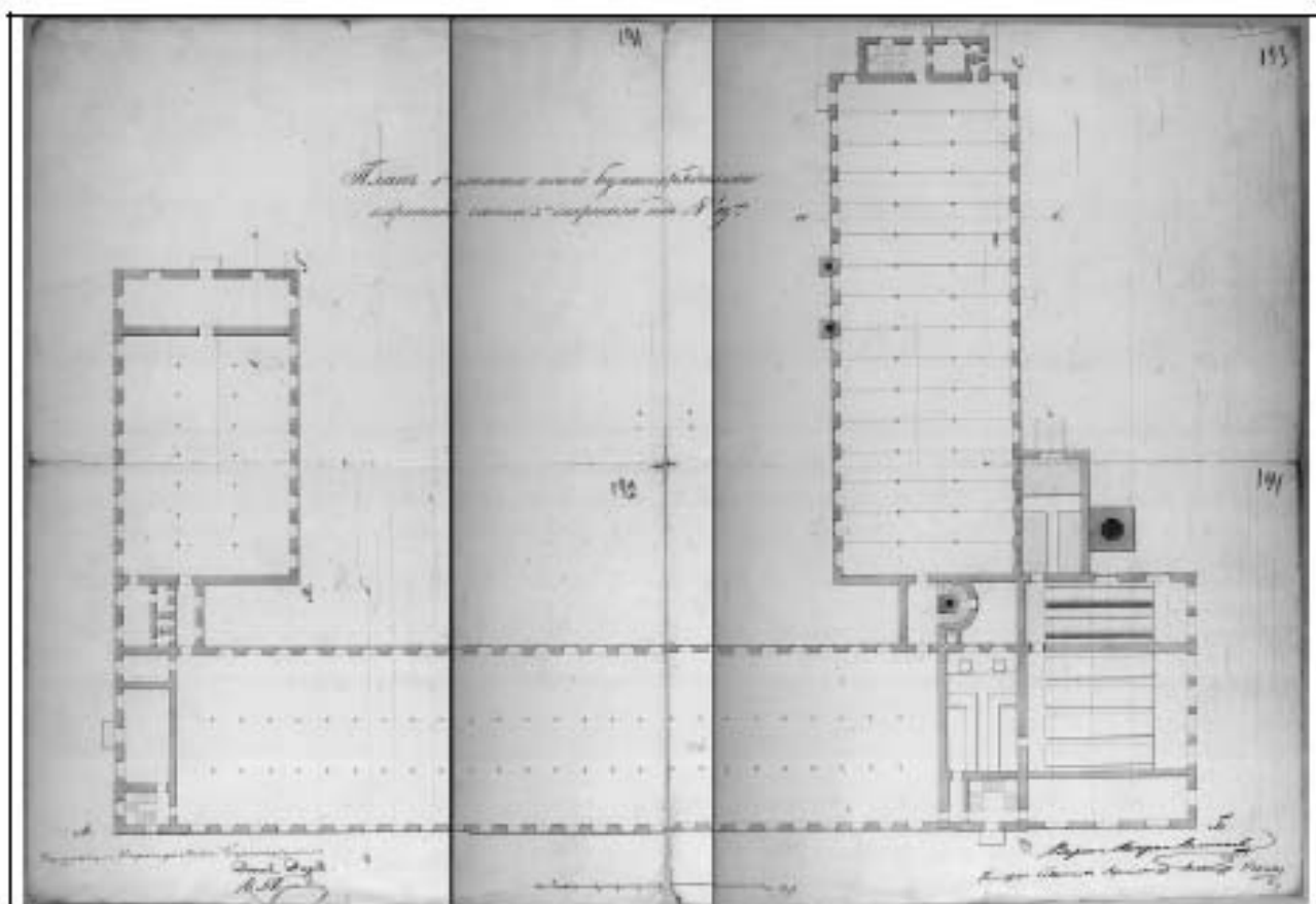
1845-1850 гг. План 1-го этажа. Архитектор А.Н.Роков. ЦИИА СПб. Ф.513. Оп.102. Д.784.
