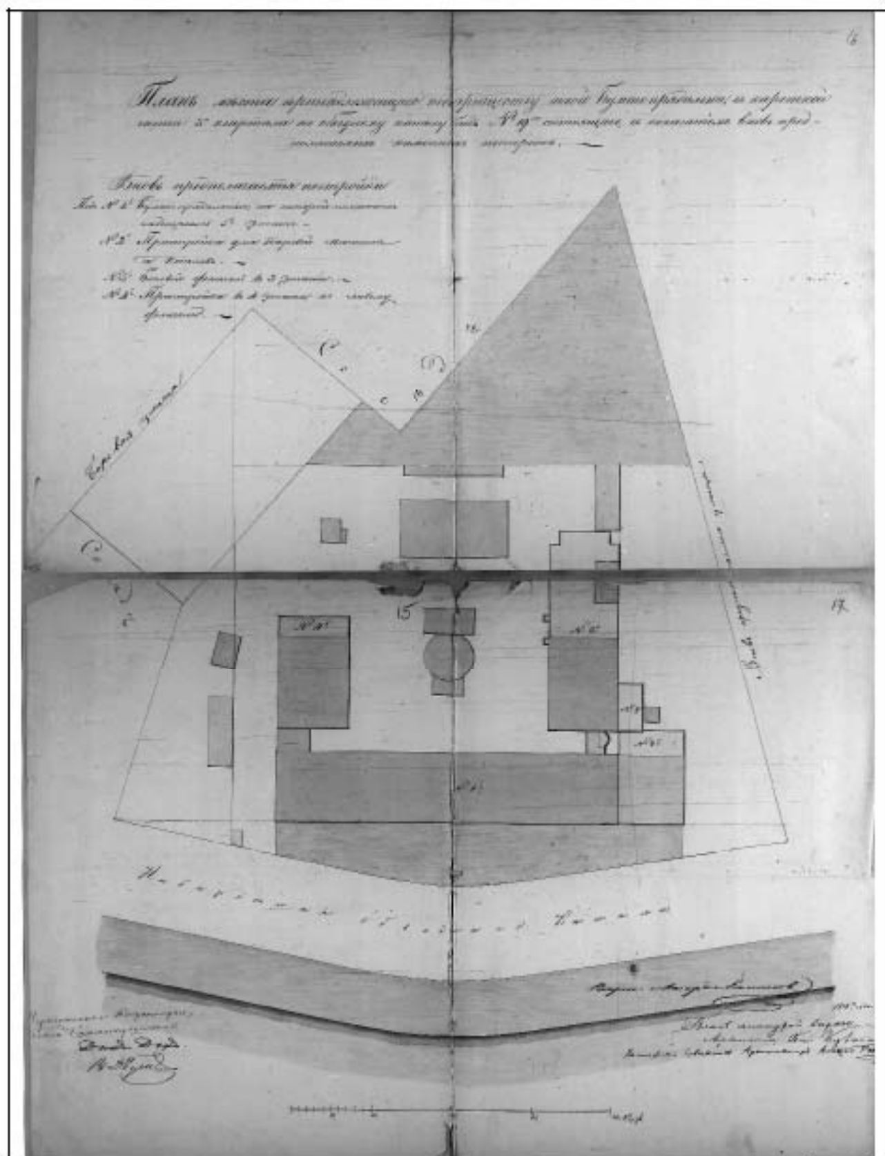
1850 г. План построек на участке Новой Бумагопрядильни. Архитектор А.Н.Роков. СПб. Ф.513. Оп.102. Д.784.
