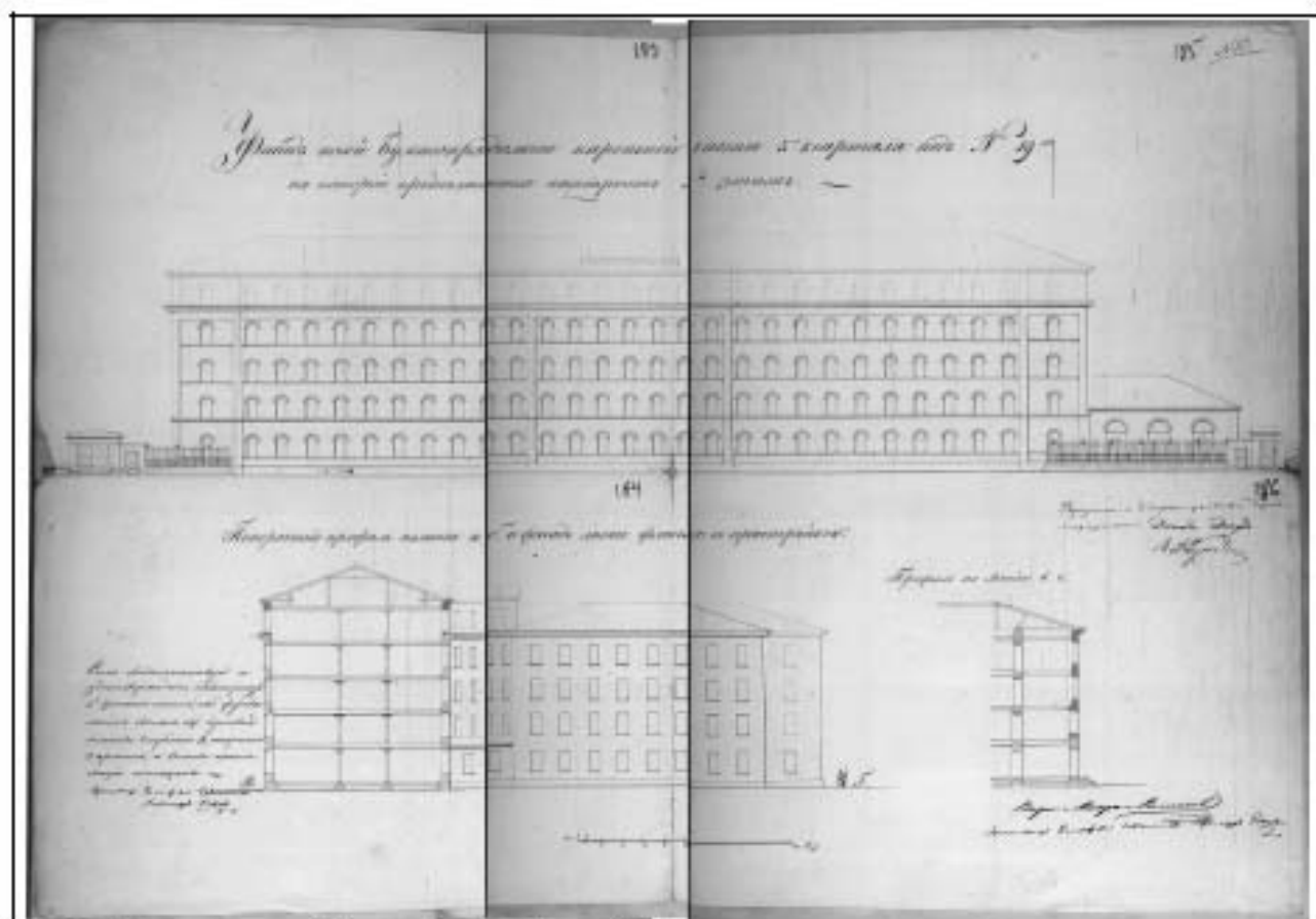
1850 г. Проект надстройки 5-го этажа. Лицевой фасад главного корпуса. Разрез главного корпуса и фасад восточного флигеля. Архитектор А.Н.Роков. ЦГИА СПб. Ф.513. Оп.102. Д.784.
