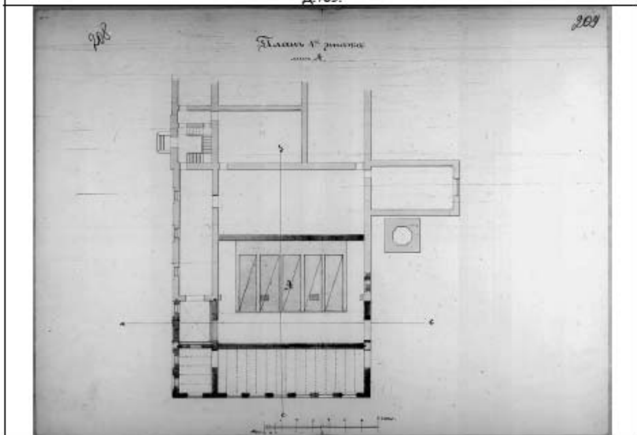
1875 г. Проект перестройки кочегарки. План 1 этажа. Архитектор А. Ф. Занфтлебен. ЦГИА СПб.
