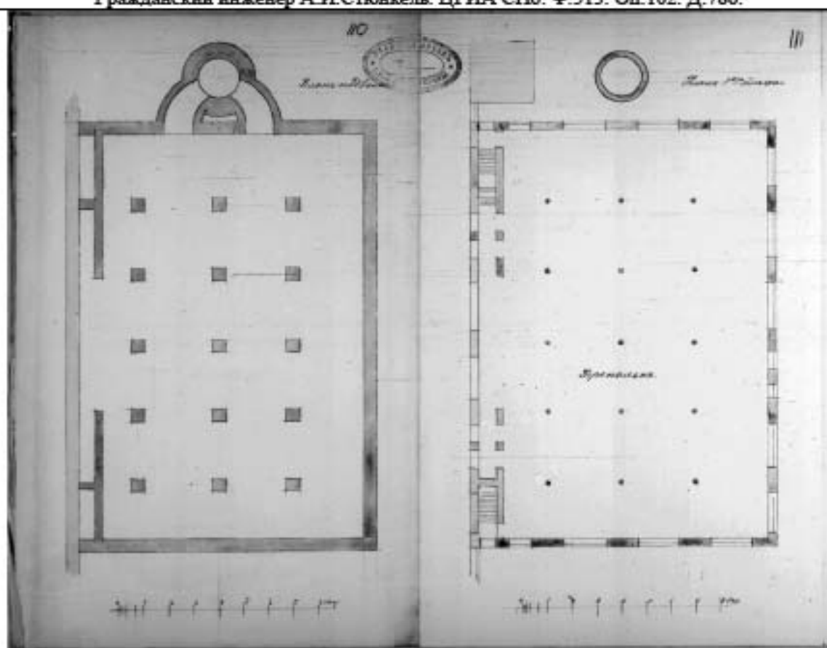
1913 г. Проект перестройки прядильного корпуса в каре основных корпусов. Гражданский инженер А.И.Стюнкель. ЦГИА СПб. Ф.513. Оп.102. Д.786.
