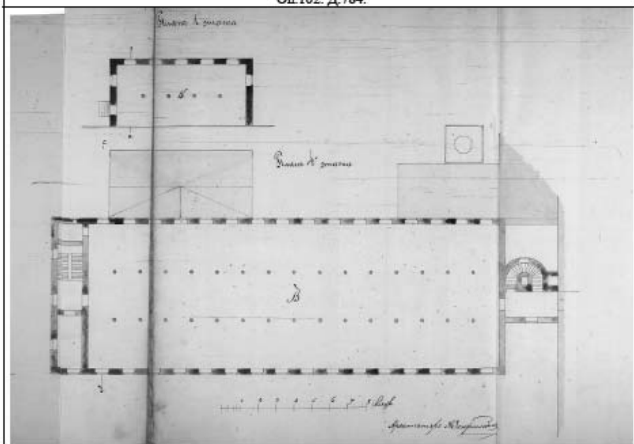
1872 г. Проект перестройки 4-го этажа восточного флигеля. Архитектор А. Ф. Занфглеб. ЦГИА СПб. Ф. 513. Оп. 102. Д. 784.
