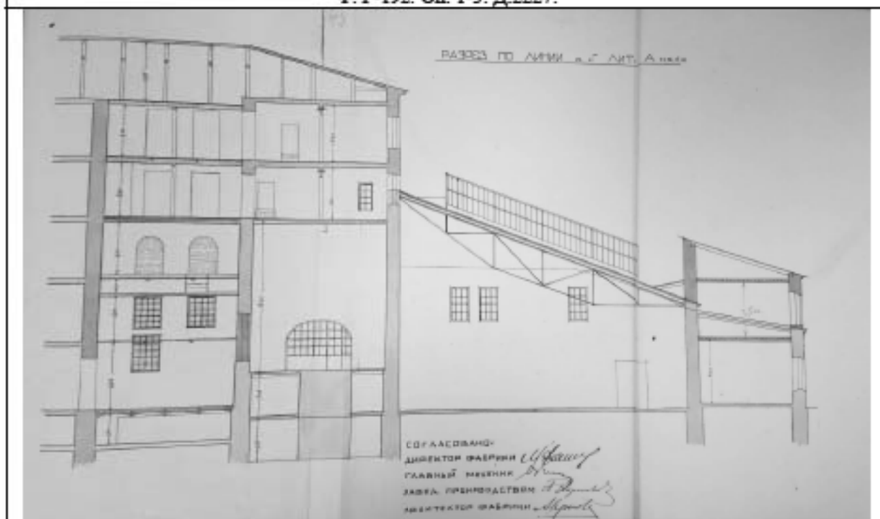
1927 г. Разрез по линии а-б корпусов А11, А12, А17, А18 (сохранились). Архитектор А.М.Арнольд. ЦГАНТД. Ф. Р-192. Оп. 1-3. Д.2227.
