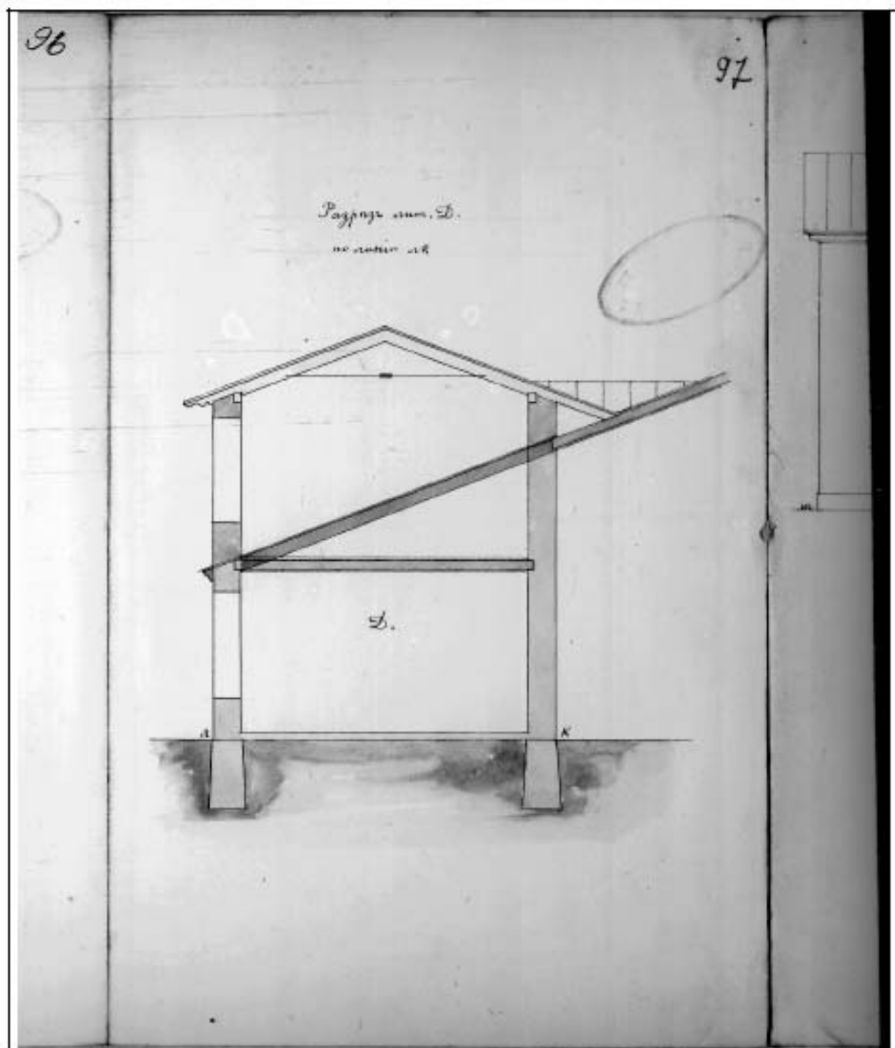
1906 г. Проект надстройки механической мастерской. Архитектор Н.П.Басин. ЦГИА СПб. Ф.513. Оп.102. Д.786.
