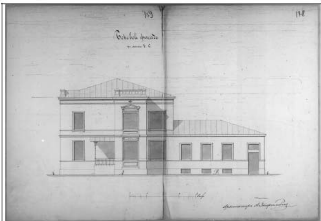
1872 г. Боковой фасад каменного жилого дома. Архитектор А. Ф. Занфглеб. ЦГИА СПб. Ф. 513. Оп. 102. Д. 784.
