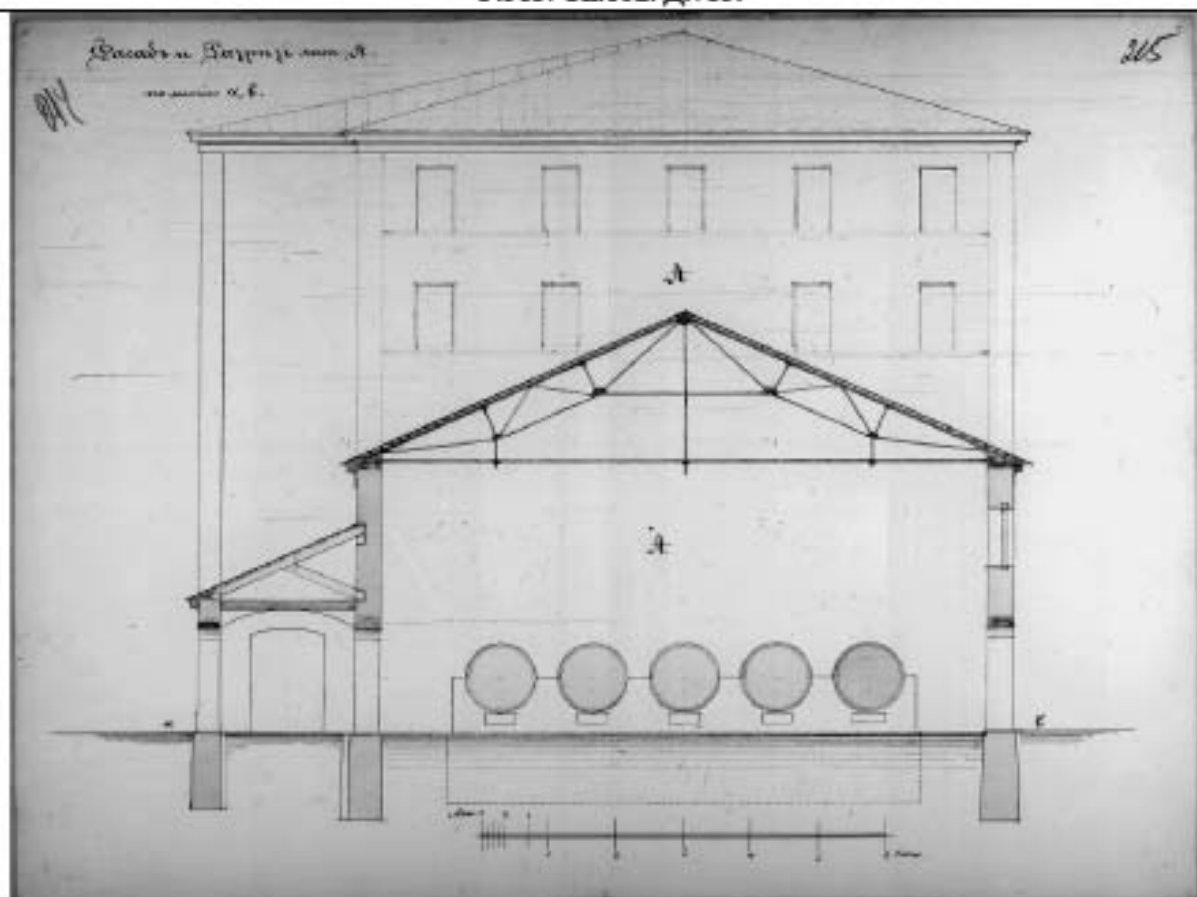
1875 г. Проект перестройки кочегарки. Разрез. Архитектор А. Ф. Занфглебен. ЦГИА СПб. Ф.513. Оп.102. Д.785.
