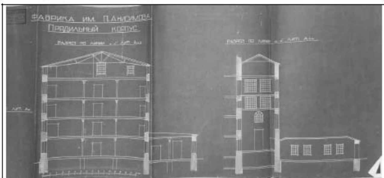
1926 г. Разрезы корпусов А3,7 и А9,10. (Утрачены) Архитектор А.М.Арнольд. ЦГАНТД Ф. Р-192. Оп. 1-3. Д.4103.
