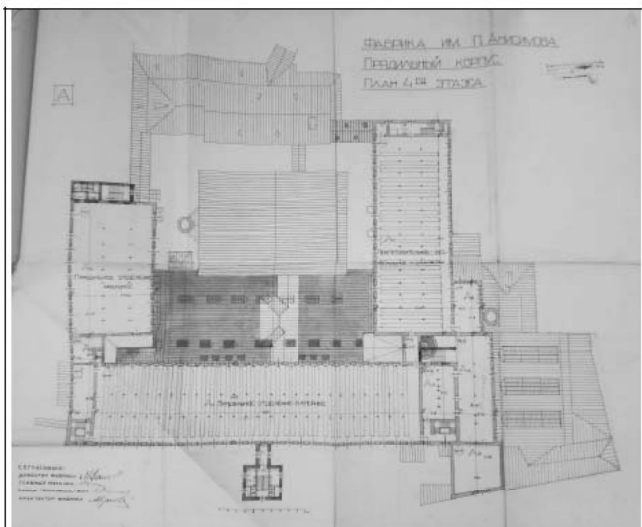
1927 г. План 4-го этажа. Архитектор А.М.Арнольд. ЦГАНТД. Ф. Р-192. Оп. 1-3. Д 2227.
