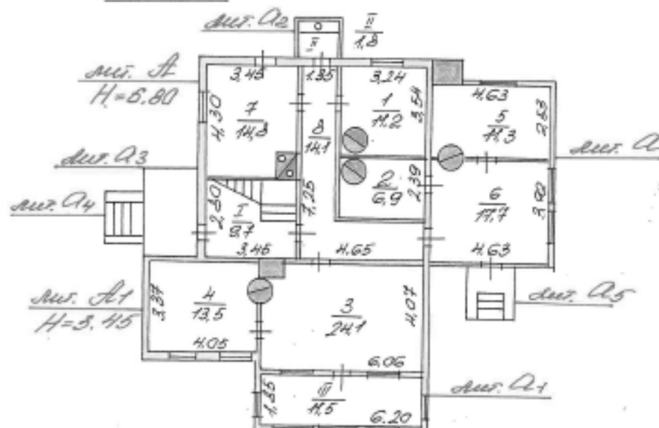
План 1 этаж
