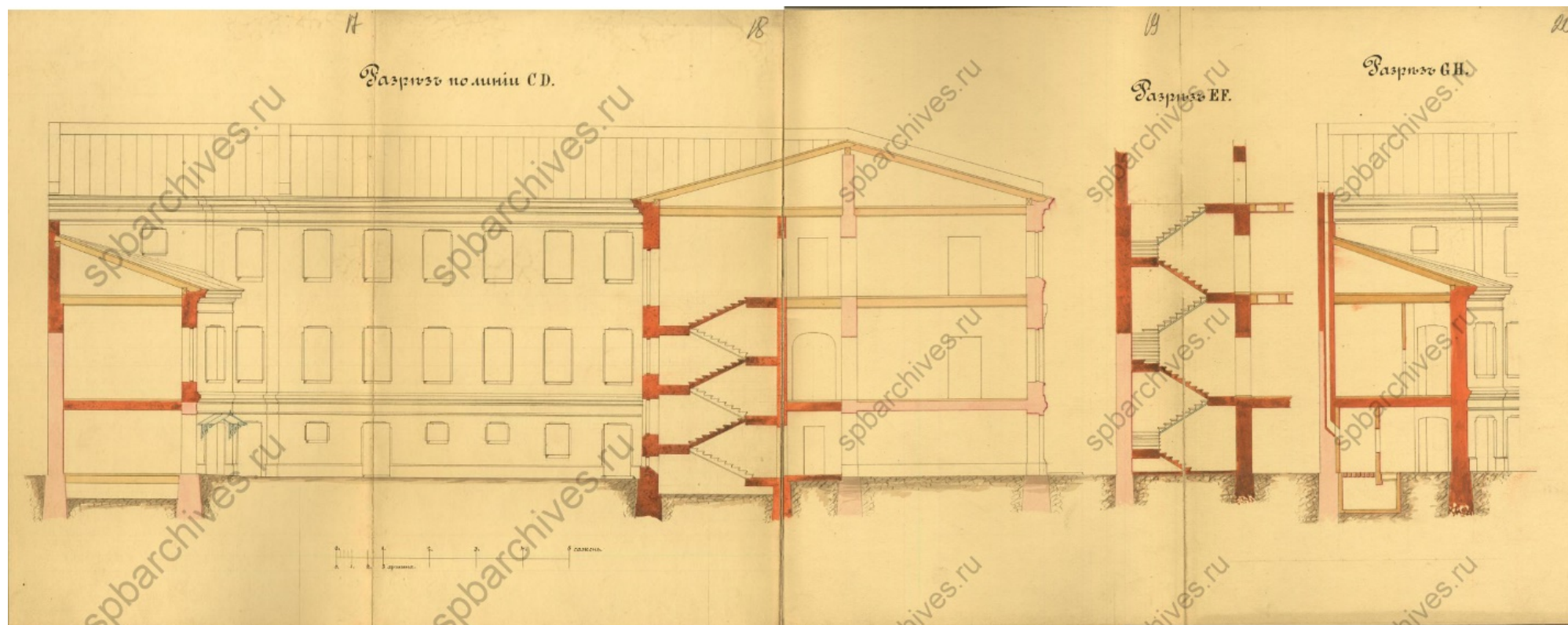
21. Разрезы. 1877 г. // Источник: ЦГИА СПб. Ф. 513. Оп. 102. Д. 57. Лл. 17-20.
