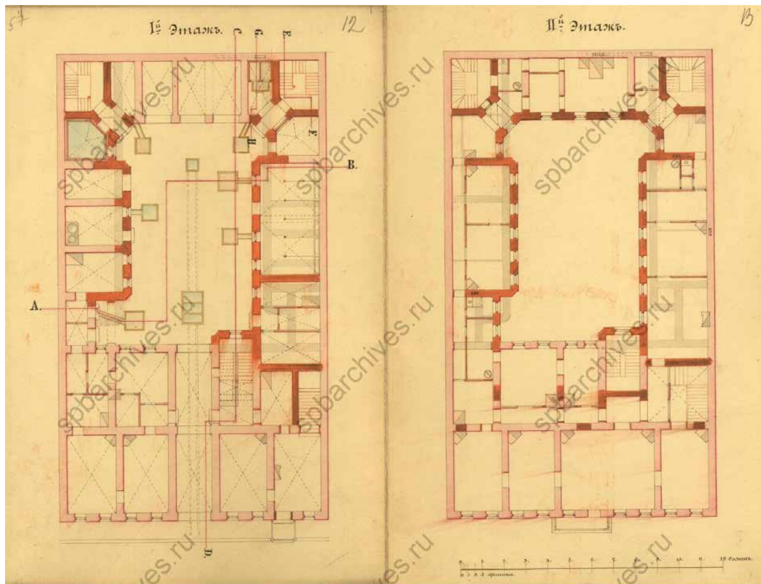
18. Планы 1 и 2 этажей. 1877 г. // Источник: ЦГИА СПб. Ф. 513. Оп. 102. Д. 57. Лл. 12-13.
