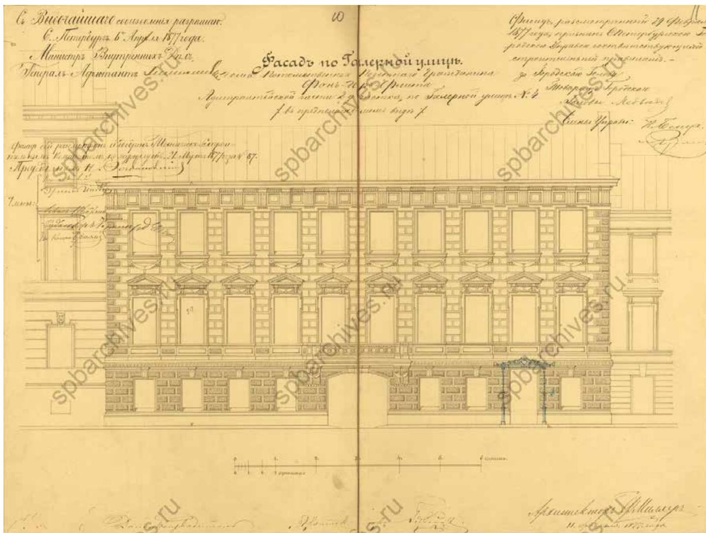
17. Фасад по Галерной улице дома потомственного почетного гражданина Фон-дер-Флита, Адмиралтейской части 2 участка, по Галерной улице №4. (в предполагаемом виде). Подпись: Архитектор Ф. Миллер. 1877 г. // Источник: ЦГИА СПб. Ф. 513. Оп. 102. Д. 57. Лл. 10-11.
