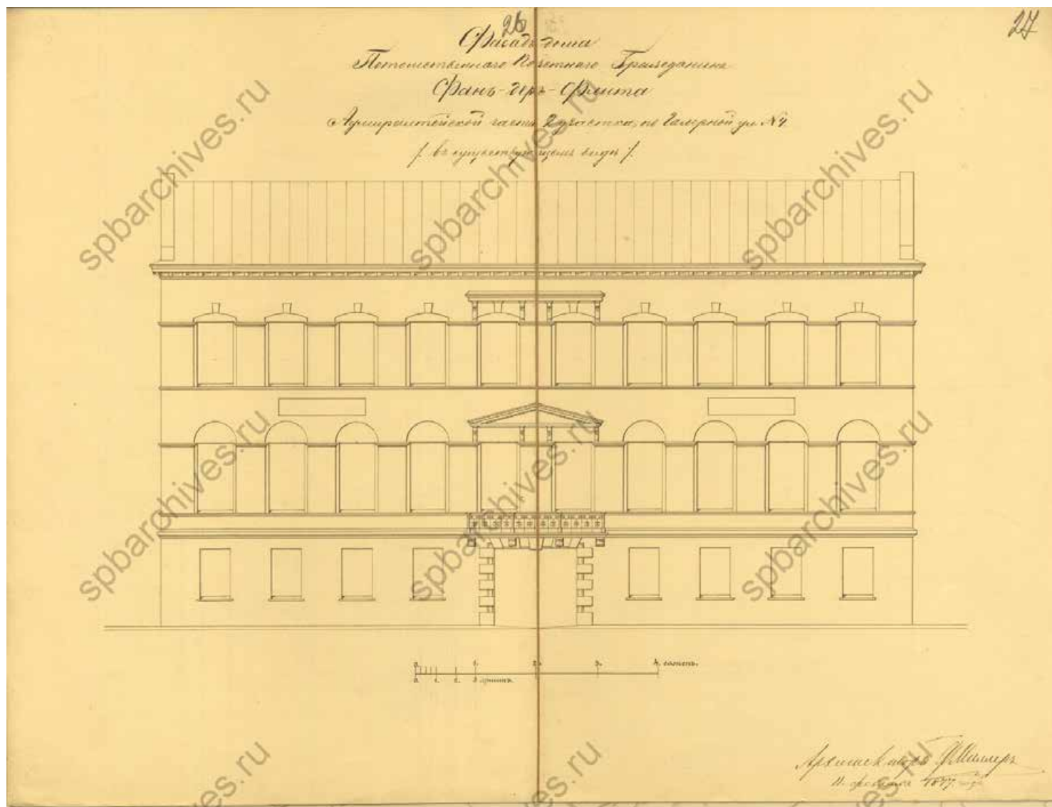
16. Фасад дома потомственного почетного гражданина Фан-дер-Флита Адмиралтейской части 2 участка, по Галерной ул. №4 (в существующем виде). Подпись: Архитектор Ф. Миллер. 1877 г. // Источник: ЦГИА СПб. Ф. 513. Оп. 102. Д. 57. Лл. 26-27.
