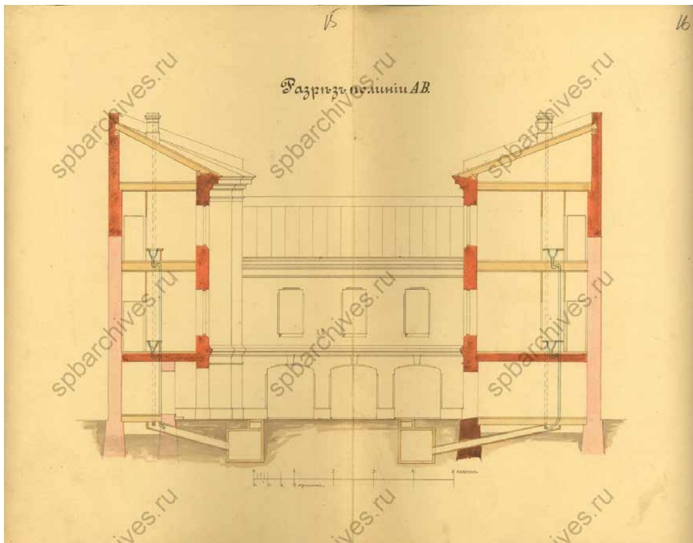
20. Разрез по линии АВ. 1877 г. // Источник: ЦГИА СПб. Ф. 513. Оп. 102. Д. 57. Лл. 15-16.
