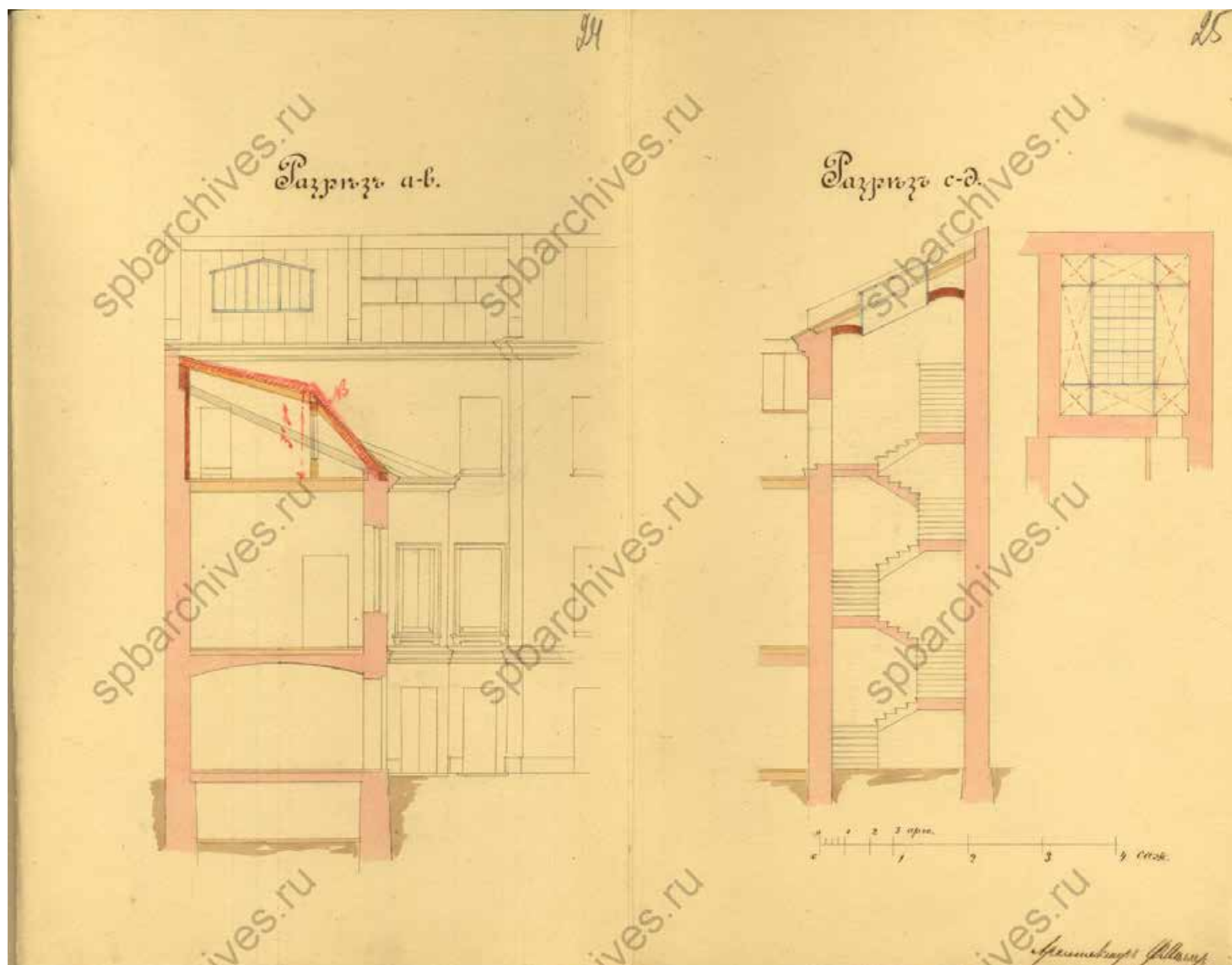
30. Разрезы. Подпись: Архитектор Ф. Миллер. 1902 г. // Источник: ЦГИА СПб. Ф. 513. Оп. 102. Д. 57. Лл. 24-25.
