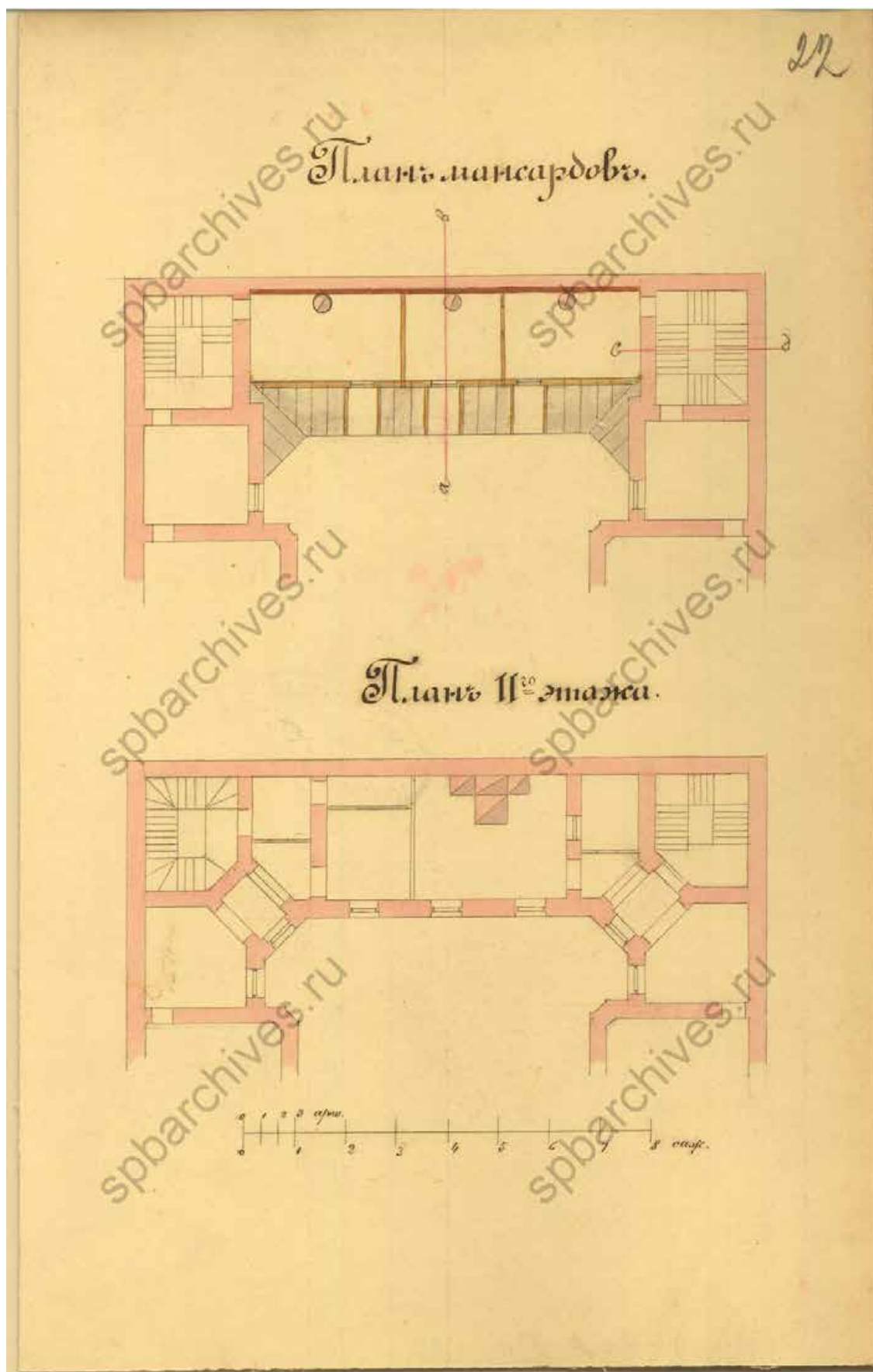
28. План мансардов и 2 этажа. 1902 г. // Источник: ЦГИА СПб. Ф. 513. Оп. 102. Д. 57. Л. 22.
