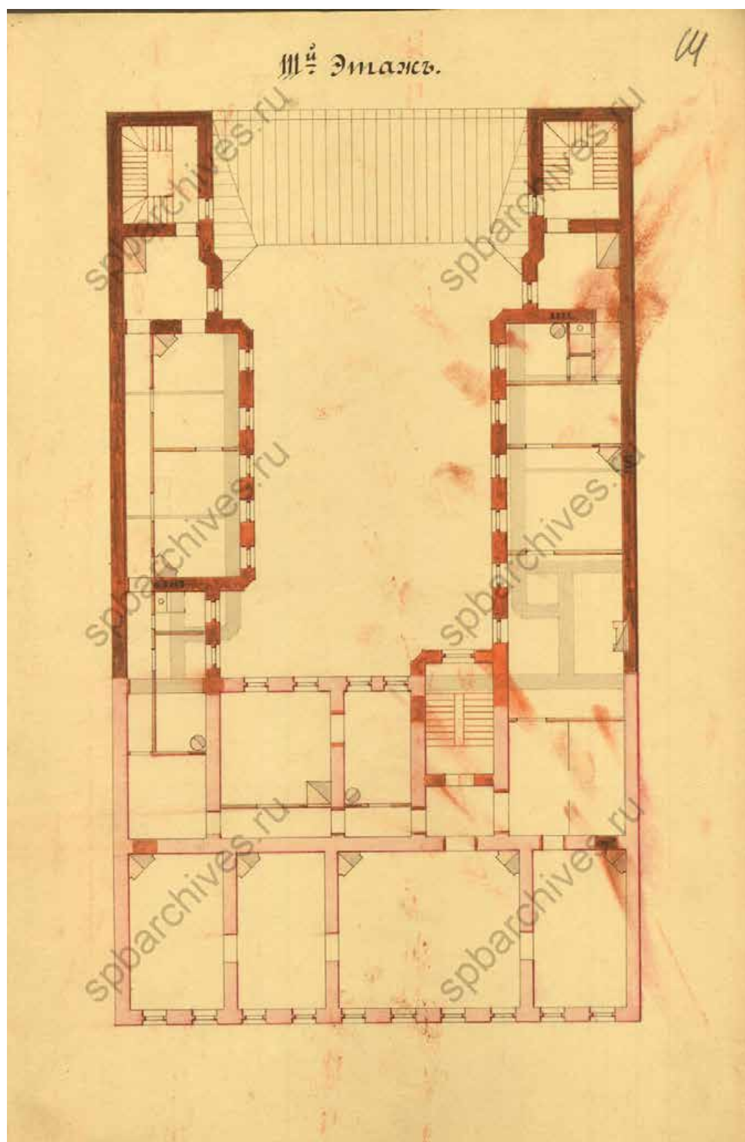
19. План 3 этажа. 1877 г. // Источник: ЦГИА СПб. Ф. 513. Оп. 102. Д. 57. Л. 14.
