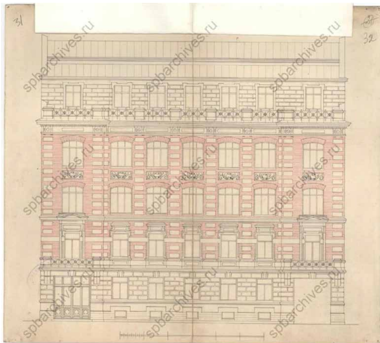
8. Фасад. 1899 г. ЦГИА СПб. Ф.513 Оп.102 Д.4297 Л. 32.
