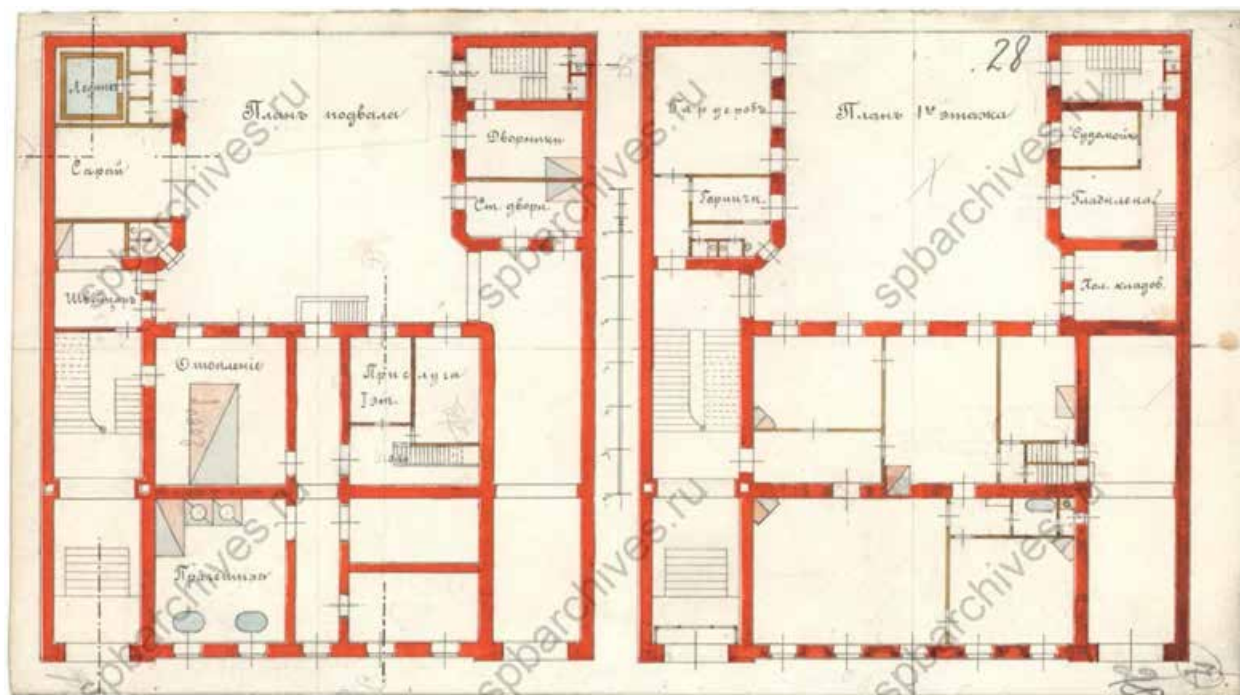
5. План подвала и 1-го этажа. 1899 г. ЦГИА СПб. Ф.513 Оп.102 Д.4297 Л. 28.
