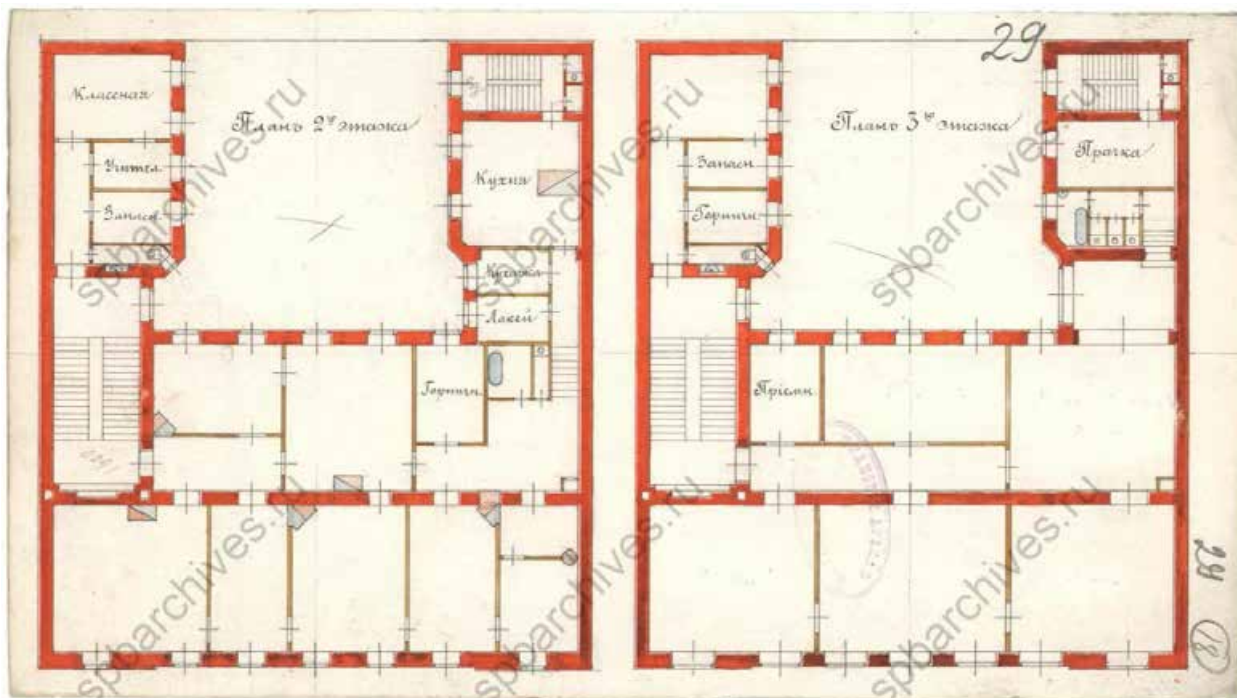
6. Планы 2-го и 3-го этажей. 1899 г. ЦГИА СПб. Ф.513 Оп.102 Д.4297 Л. 29.
