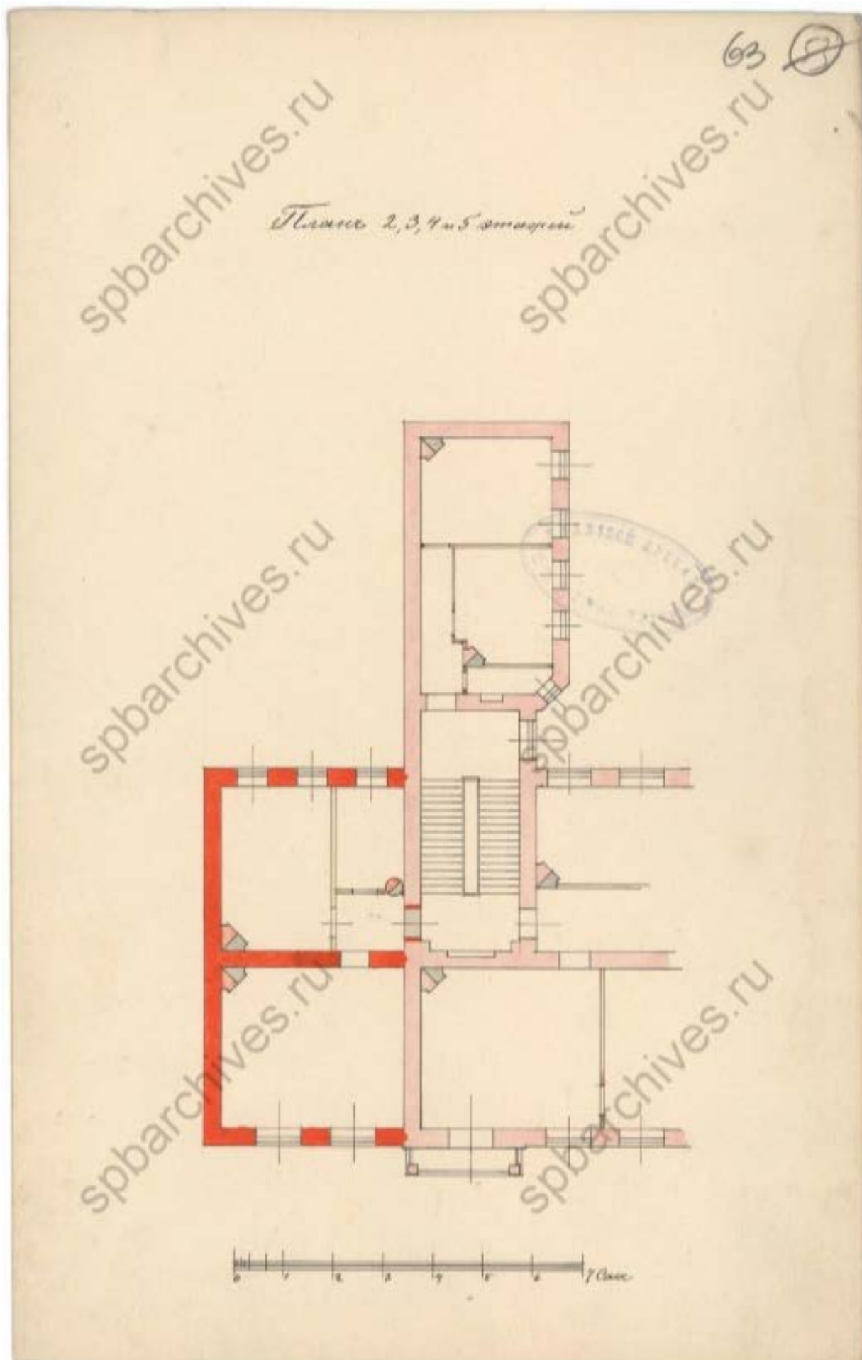
11. План 2, 3, 4, и 5 этажей. 1902 г. ЦГИА СПб. Ф.513 Оп.102 Д.4297 Л. 63.
