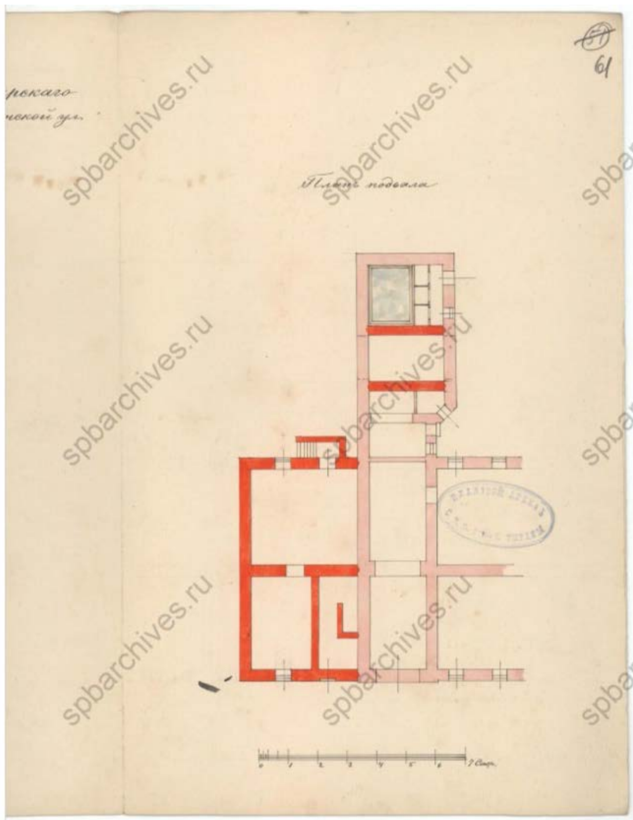
9. План подвала. 1902 г. ЦГИА СПб. Ф.513 Оп.102 Д.4297 Л. 61.
