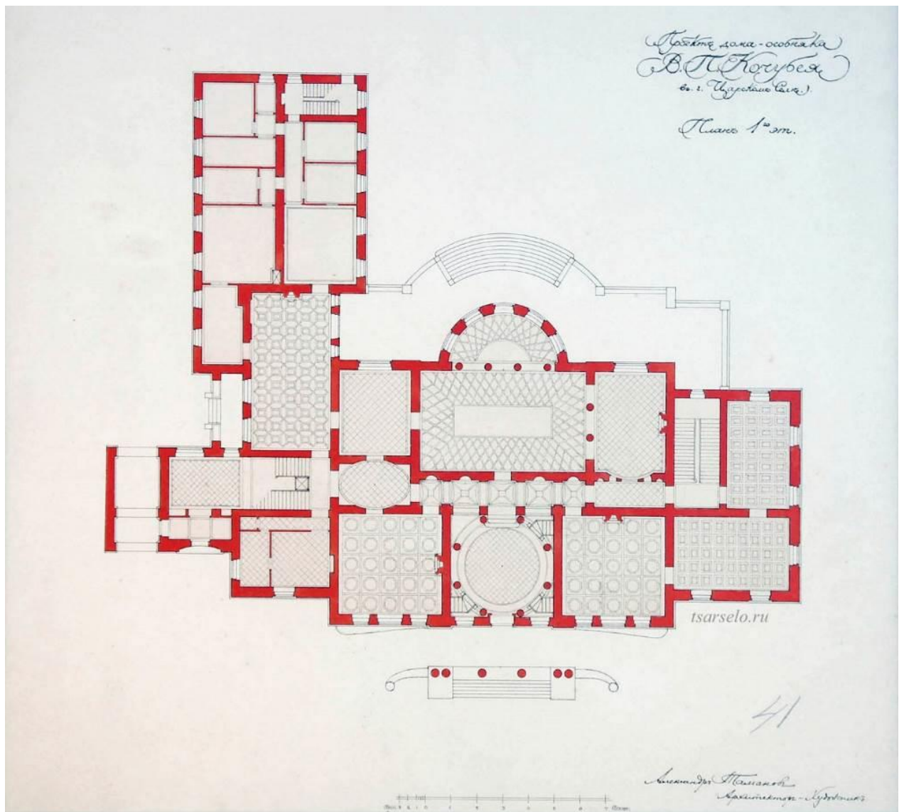
Илл. 8. Таманов Александр. План 1 этажа особняка В.П. Кочубея, 1911· ГМЗ «Царское Село».
