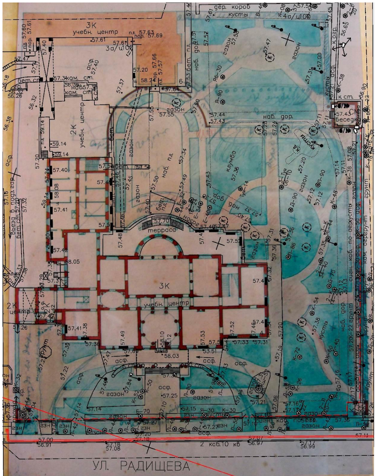
Илл. 22. Совмещённый план топосъёмки 2019 года и проектного чертежа 1914 года.
