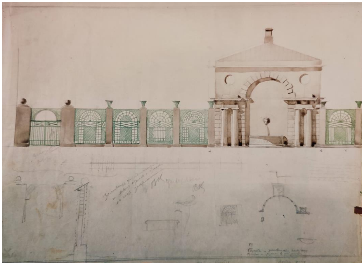
Илл. 14. Эскиз ограды между садом и хозяйственным двором с фонтаном. Арх. Н. Лансере. 1914. Из собрания ГМИ СПб.
