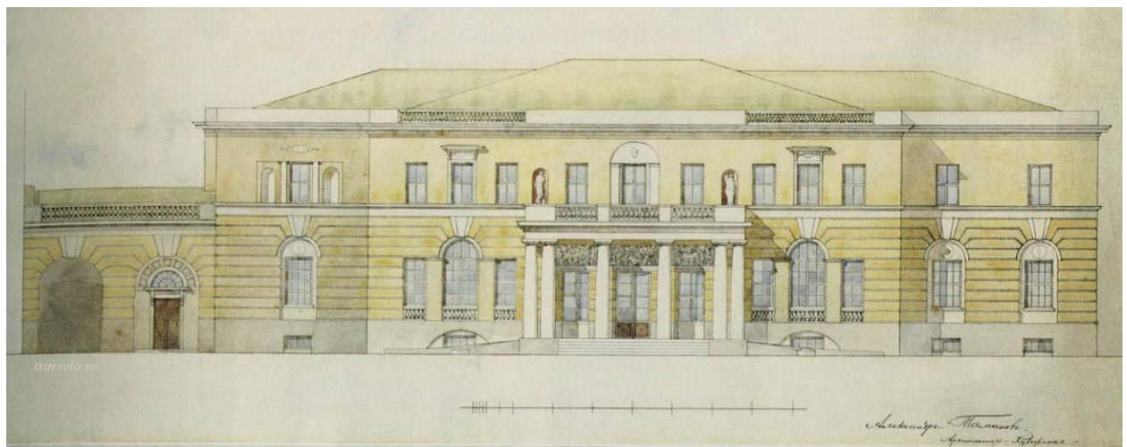
Илл. 4. Таманов Александр. Проект парадного фасада особняка Кочубея. ГМЗ Царское Село. 1911 г.
