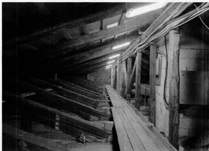
45, 46. Стропильная система
