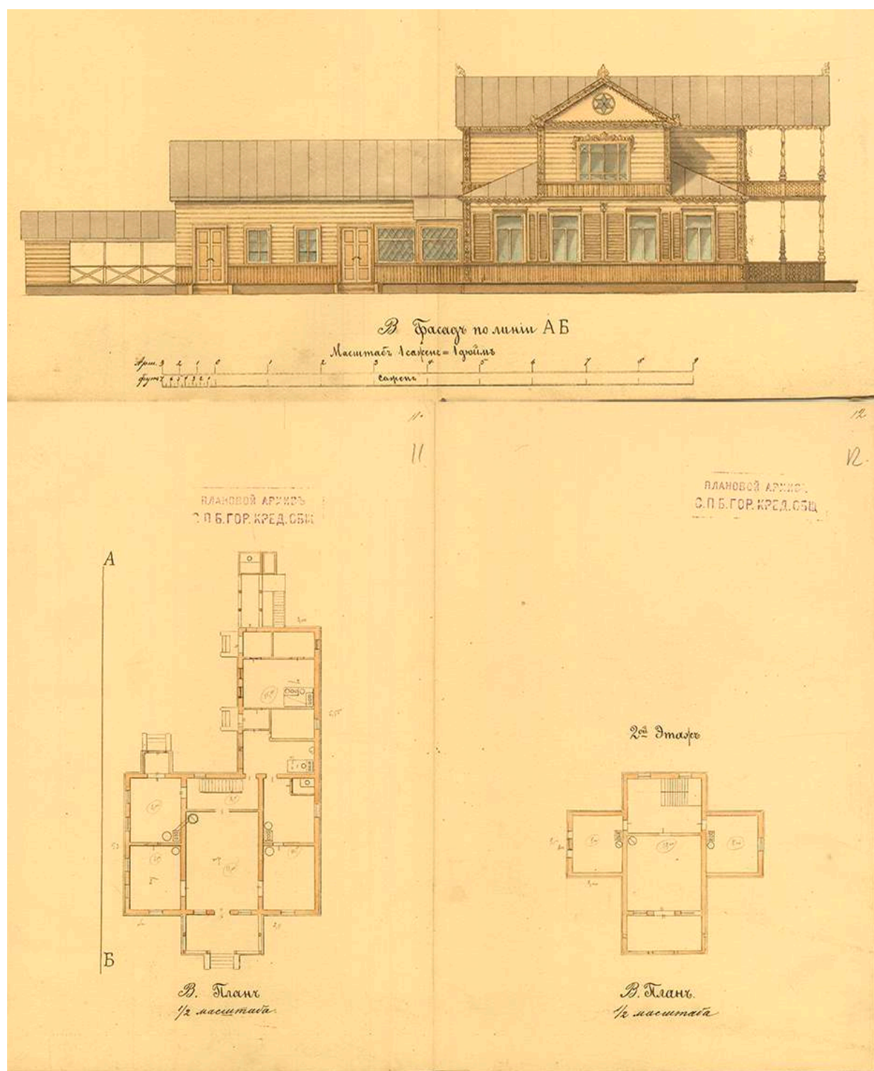
19. Фасад и планы дома Н.Н.Струка. 1884 г. //ЦГИА СПб. Ф. 515. ОП. 4. Д. 212 1. Лл. 9-11//
