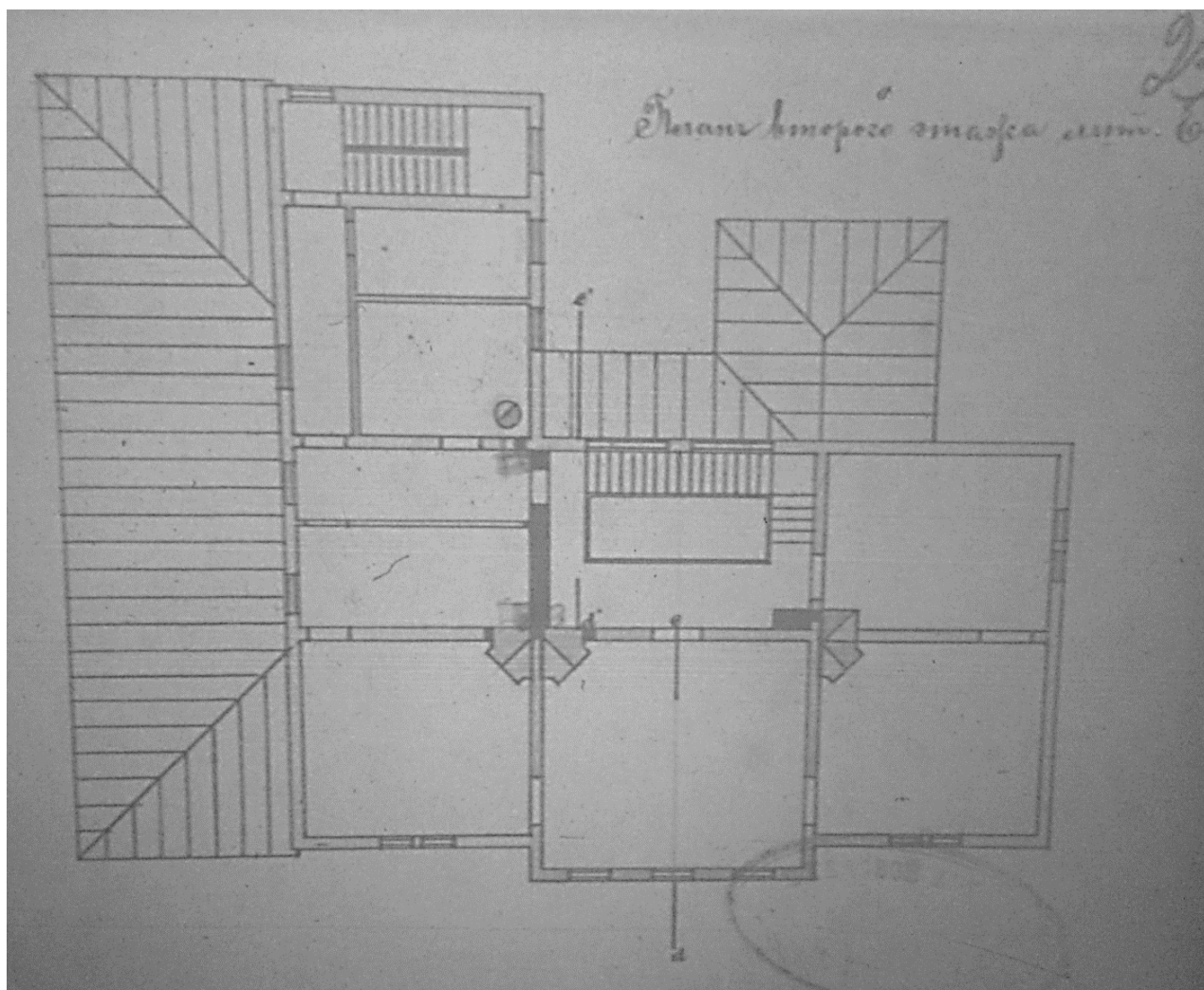
72. Проект пристройки к дому на участке Н.Н.Струка. План 2 этажа. 1908 г. //ЦГИА Ф. 515. Оп.102. Д. 2618. Л. 21//
