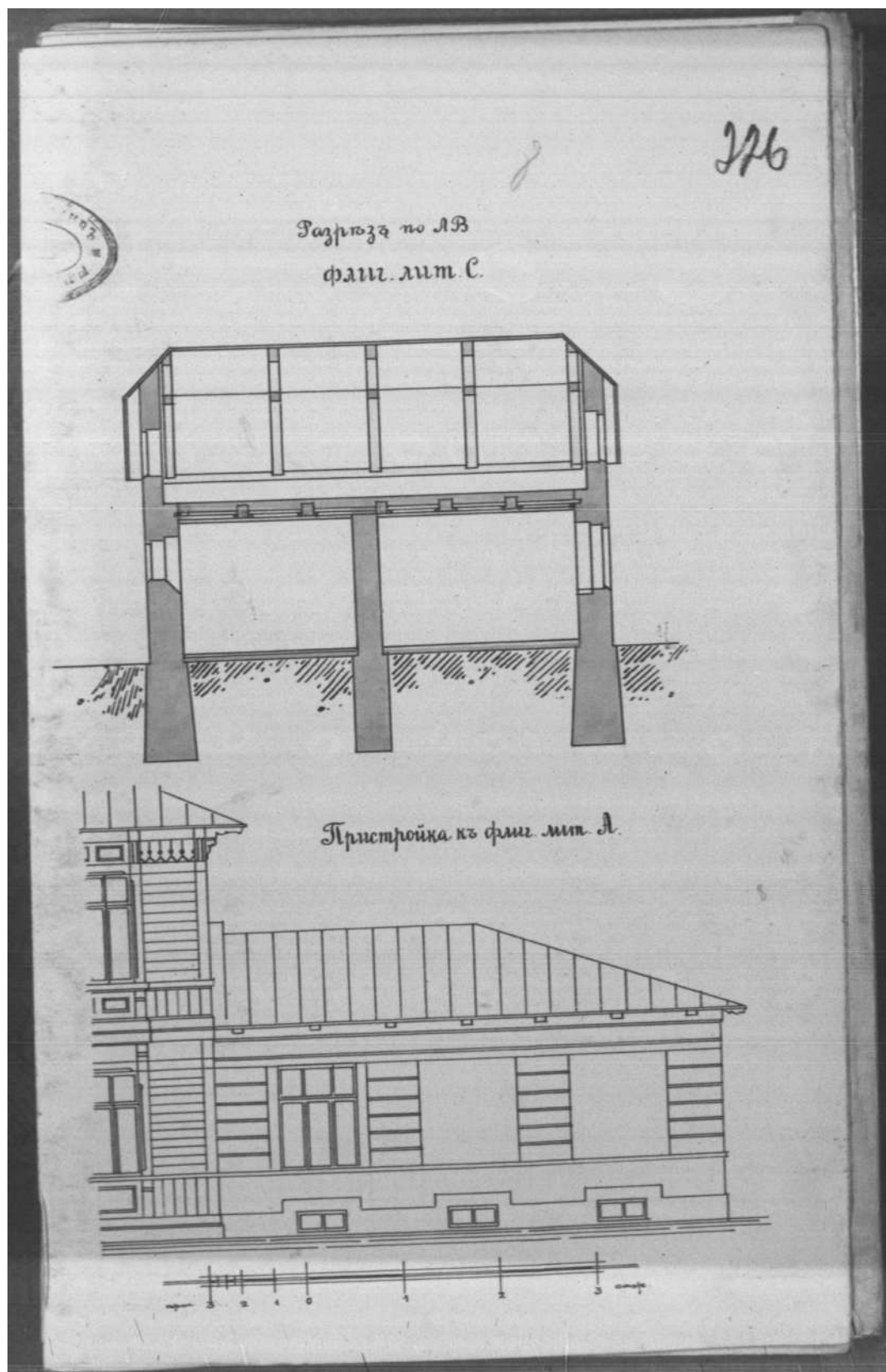
60. Проект пристройки флигеля к особняку. Фасад. 1911 г. //ЦГИА СПб. Ф. 513. ОП. 102. Д. 2664. Л. 226//
