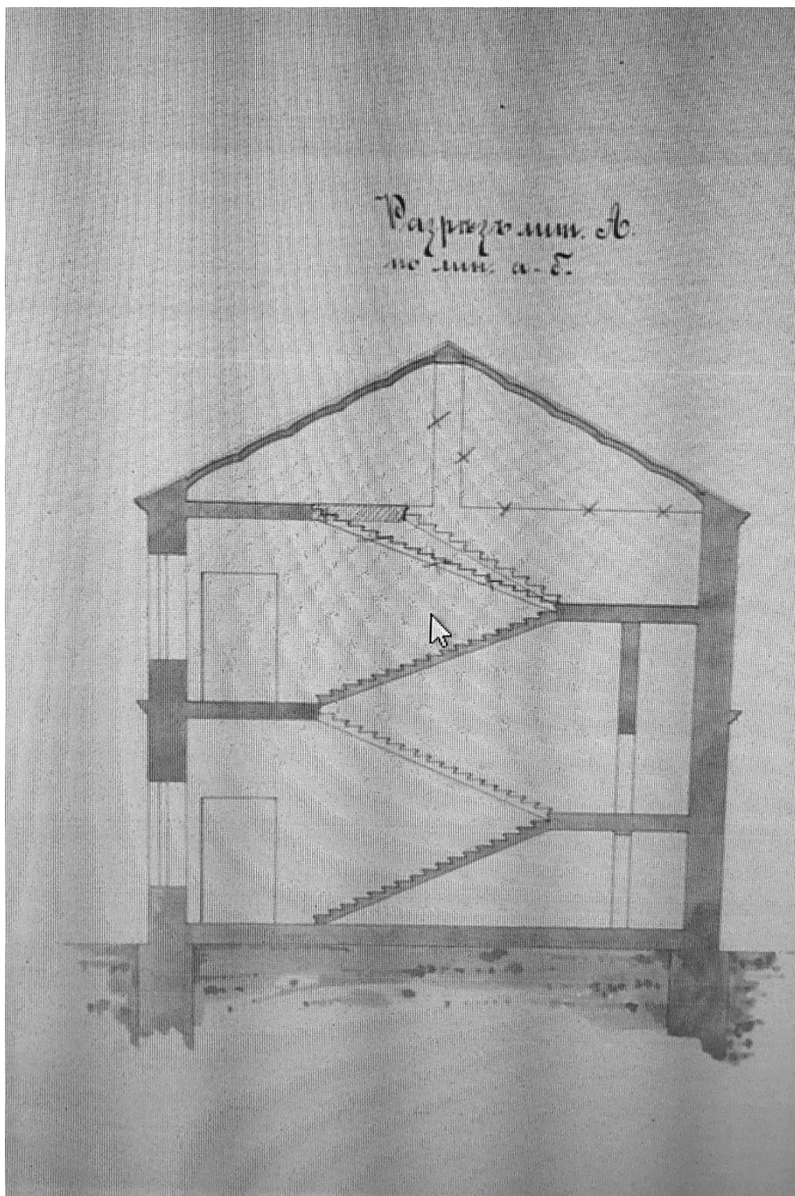
59. Проект административного корпуса. Разрез. 1900 г. //ЦГИА СПб. Ф. 513. ОП. 102. Д. 2664. Л. 137//
