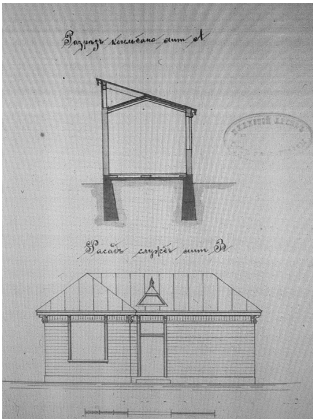
64. Проект строительства кегельбанов на участке Н.Н.Струка. Разрез. 1902 г. // Ф. 513. Оп. 102. Д. 2664. Л. 15//
