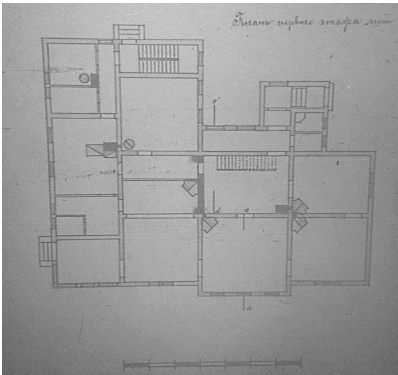
71. Проект пристройки к дому на участке Н.Н.Струка. План 1 этажа. 1908 г. //ЦГИА Ф. 515. Оп.102. Д. 2618. Л. 22//
