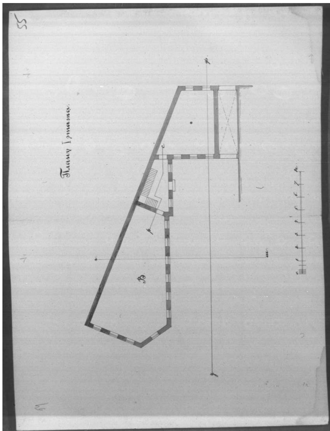
33. Проект пристройки к производственному зданию вдоль западной границы участка. План 1 этажа. 1895 г. //ЦГИА СПб. Ф. 513. Оп. 102. Д. 2664. Л. 55//
