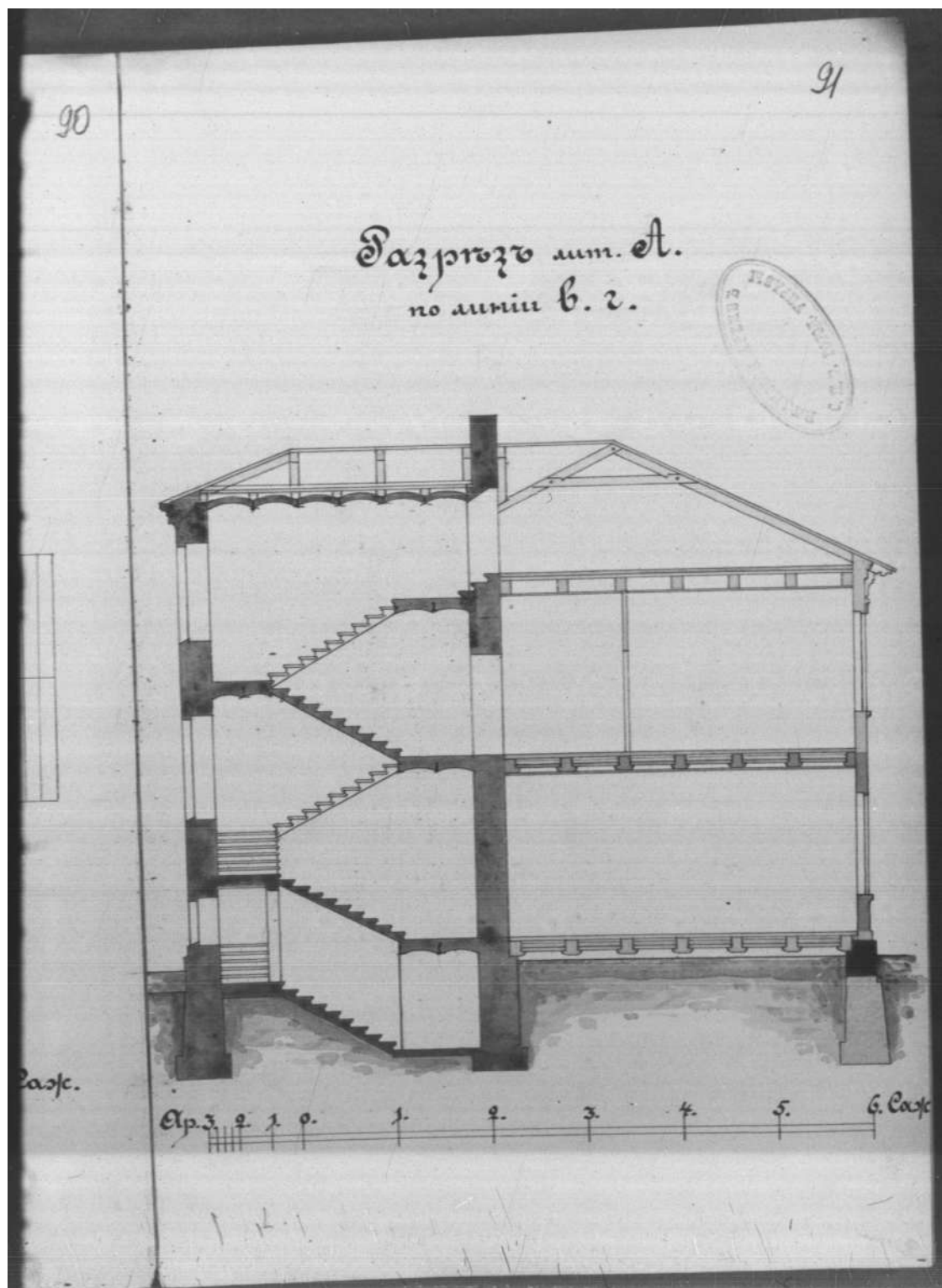
48. Проект каменной пристройки. 1897 г. Разрез // ЦГИА Ф. 513. Оп. 102. Д. 2664 Л. 89//
