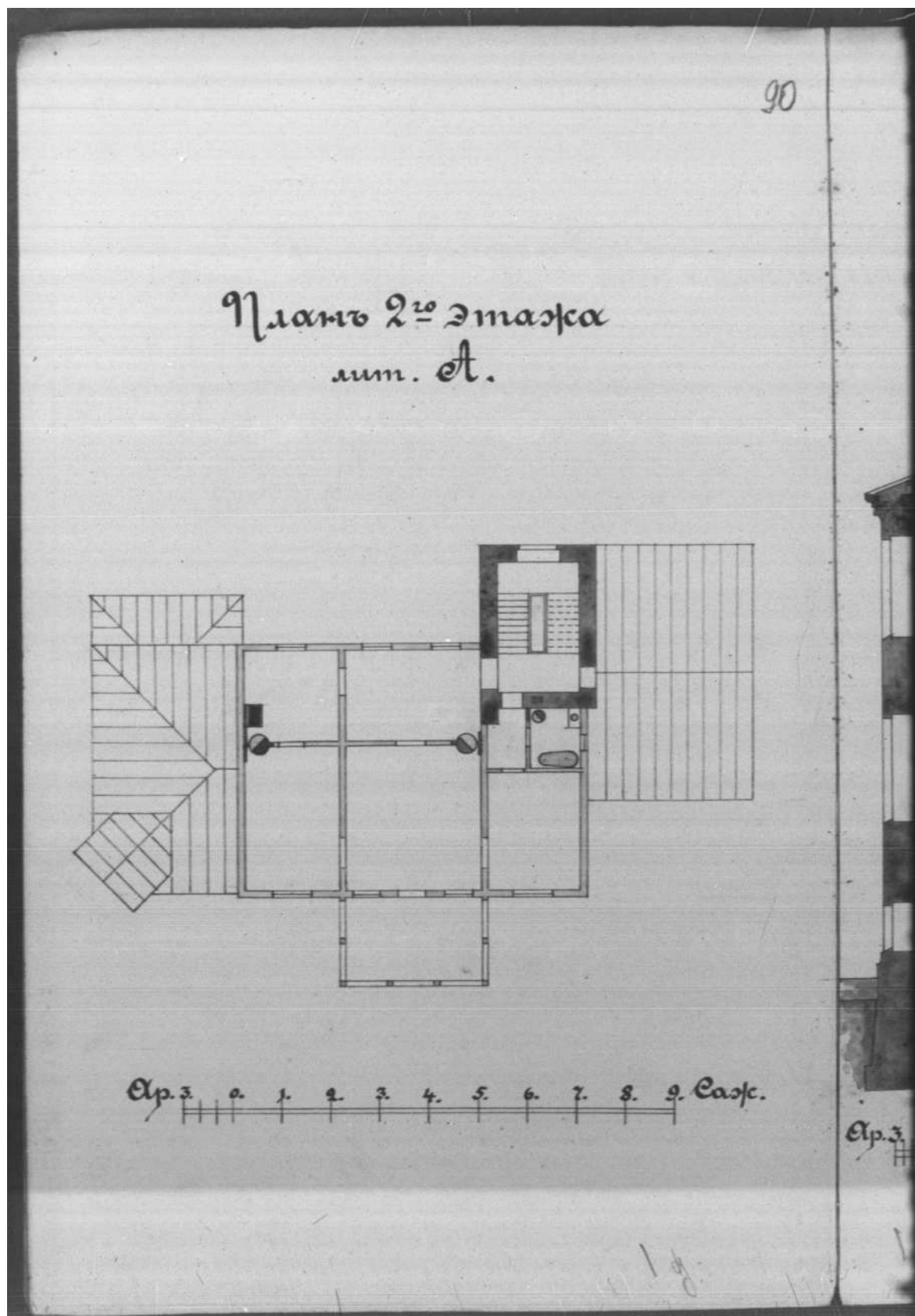
47. Проект каменной пристройки. 1897 г. План 2 этажа // ЦГИА Ф. 513. Оп. 102. Д. 2664 Л. 89//
