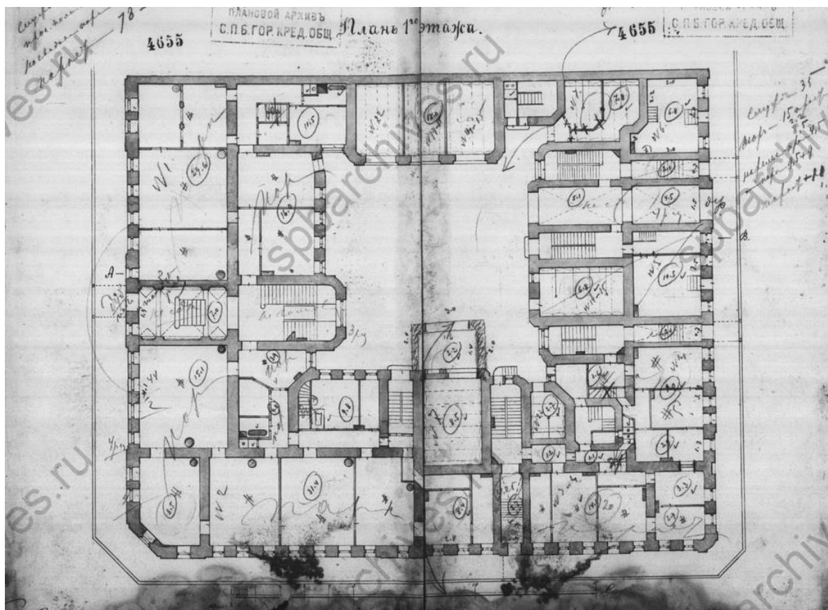
Илл. 20. План 1-го этажа. Дата: 1887 г. Источник: ГЦИА СПб, ф. 515, оп. 4, д. 4756.
