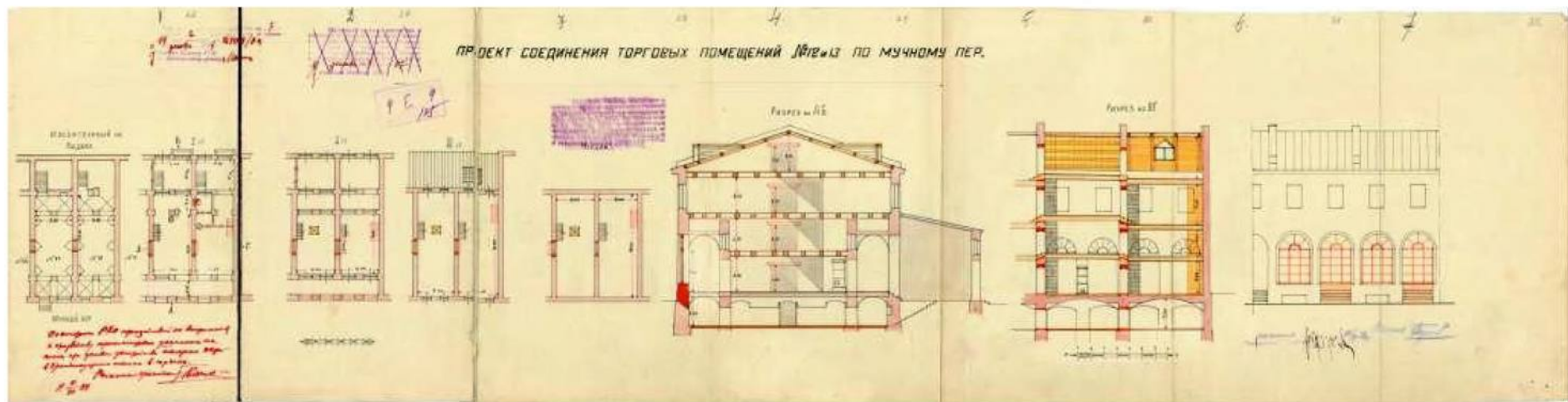
Илл. 131. Проект соединения лавок №№ 12-19. 1929 г. ЦГА НТД. Ф. 192. Оп. 31. Д. 5481. Л. 26-32.
