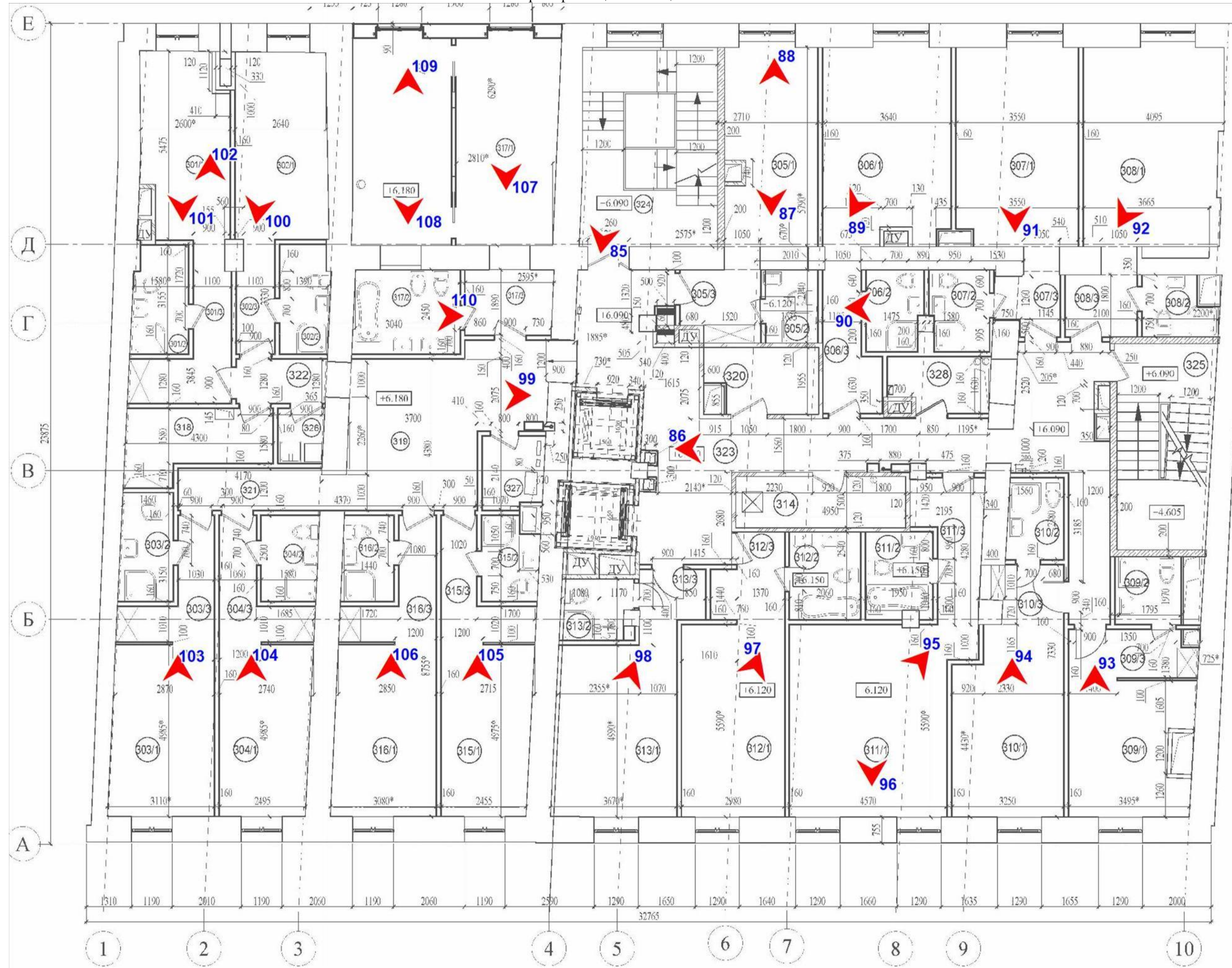
Схема фотофиксации помещений 3-го этажа
