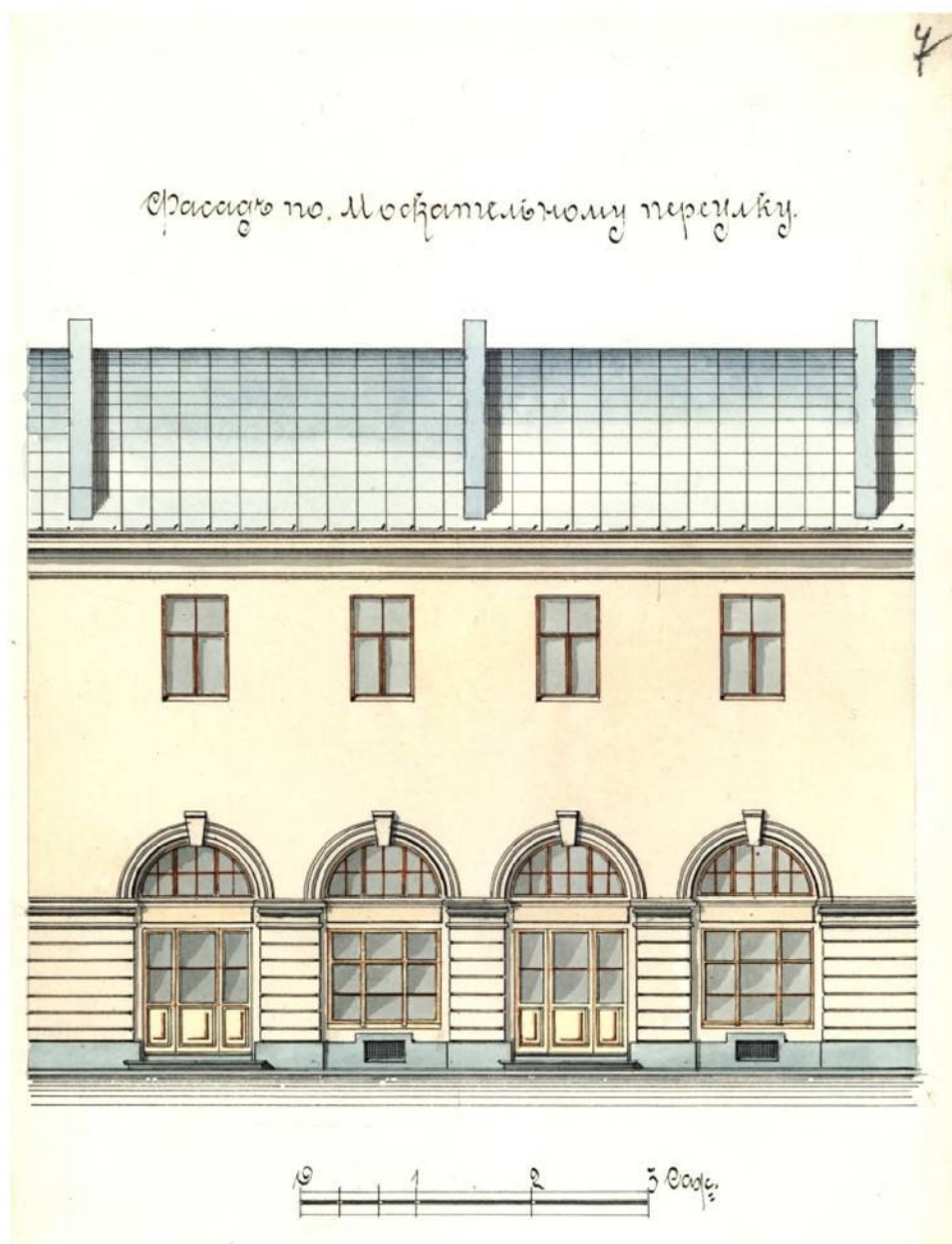
Илл. 106. Малый Гостиный двор. Большой железный ряд. Проект перестройки. Лавки № 8-10. Закрытие галерей, устройство лестницы, надстройка пристройки со стороны Москательного пер. 1903 г. Архитектор А. Ковшаров. Фасад со стороны Москательного пер. . ЦГИА СПб. Ф. 513. Оп. 115. Д. 661. Л. 7.
