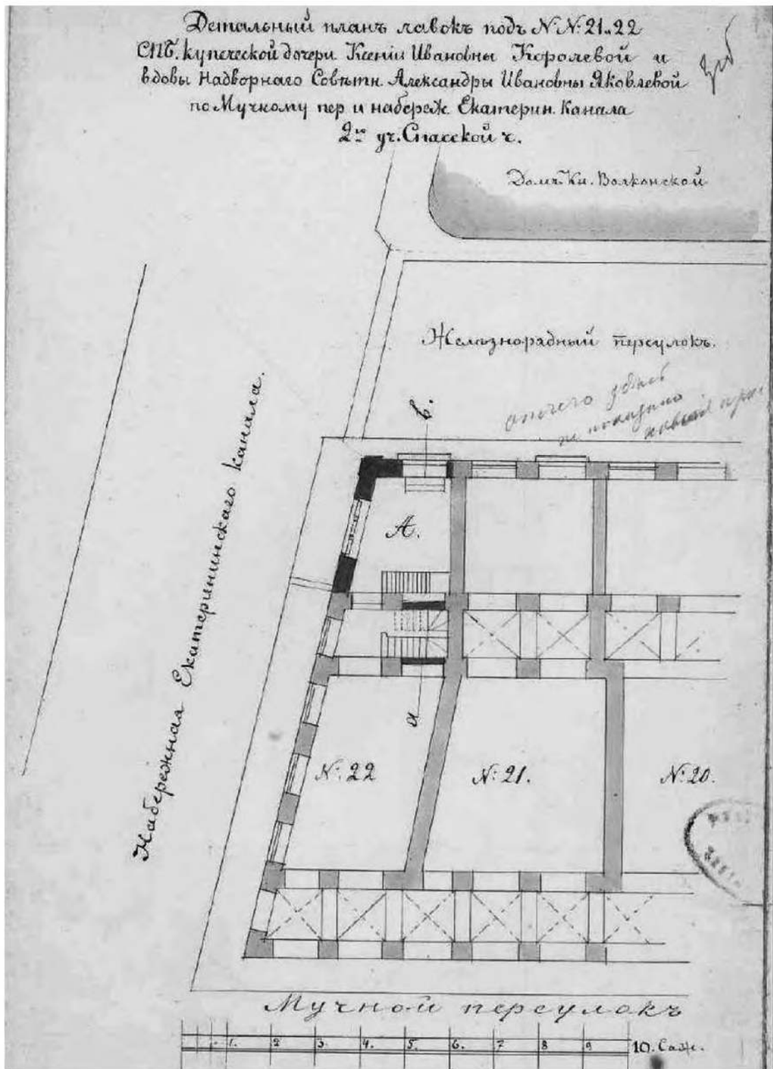
Илл. 148. Малый Гостиный двор. Большой железный ряд. 1900 г. План первого этажа лавок №№ 20-22. ЦГИА СПб. Ф. 513. Оп. 115. Д. 667. Лл. 3 об.
