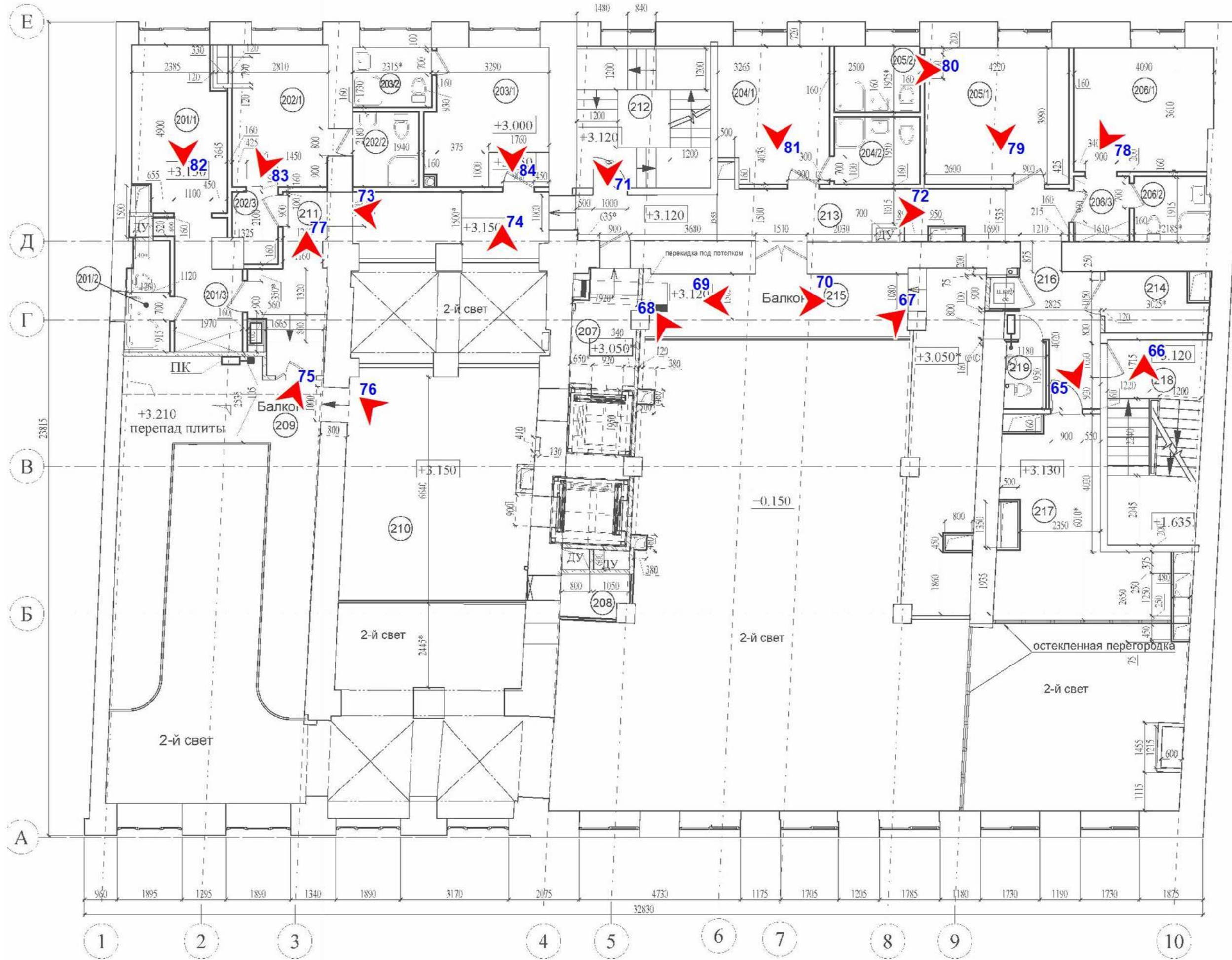
Схема фотофиксации помещений 2-го этажа
