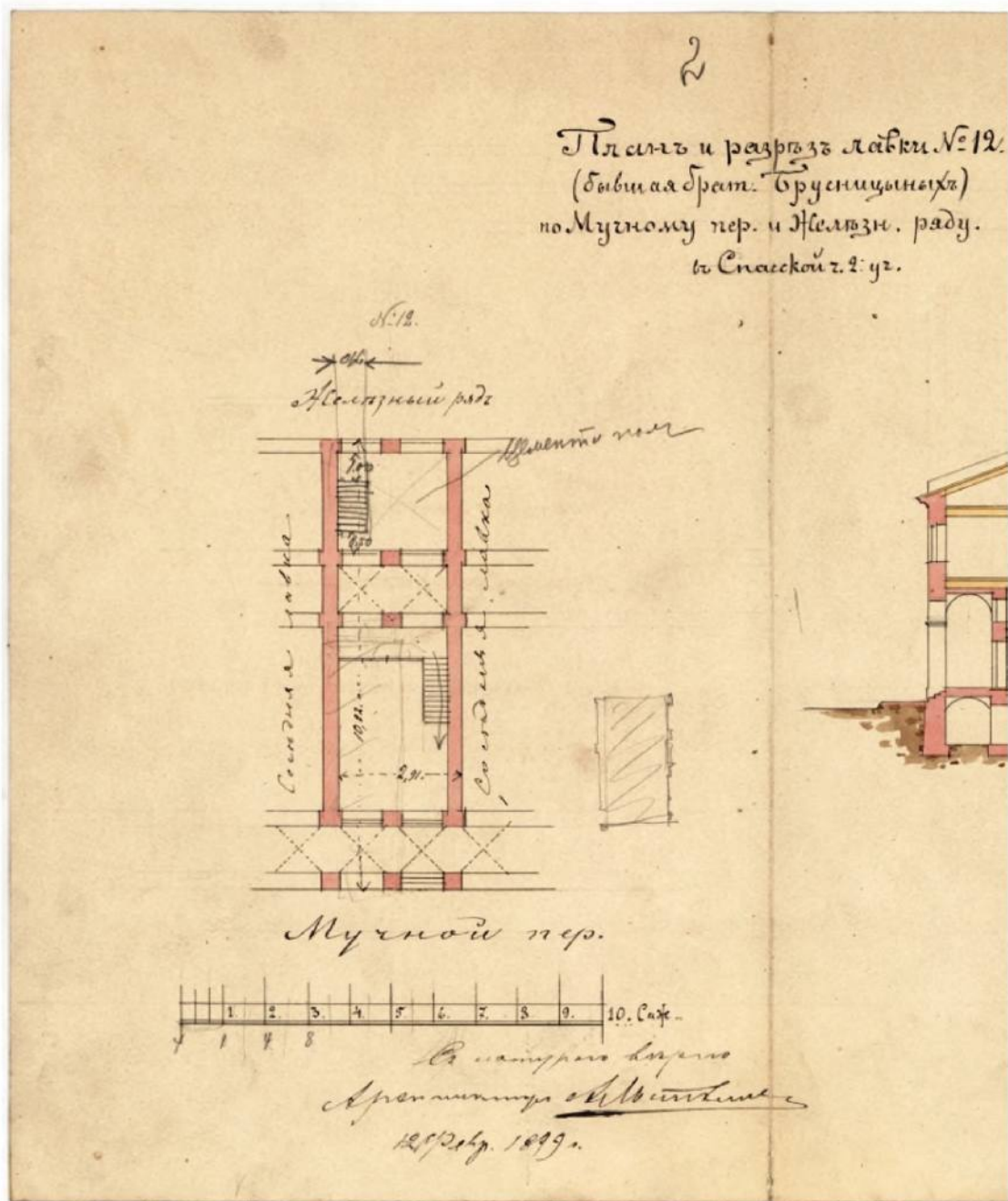
Илл. 114. Малый Гостиный двор. Большой железный ряд. Лавка № 12. План. 1899 г. ЦГИА СПб. Ф. 513. Оп. 101. Д. 595. Л. 2.
