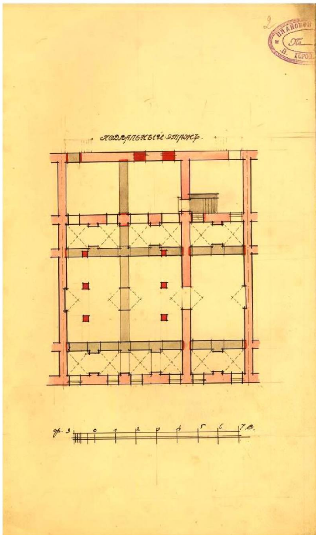
Илл. 170. План подвального этажа Торгового дома В.П. Липина. Проект. 19 февраля 1915 г. Архитектор А.А. Оль. ЦГИА СПб. Ф. 513. Оп. 173. Д.167. Л.2.
