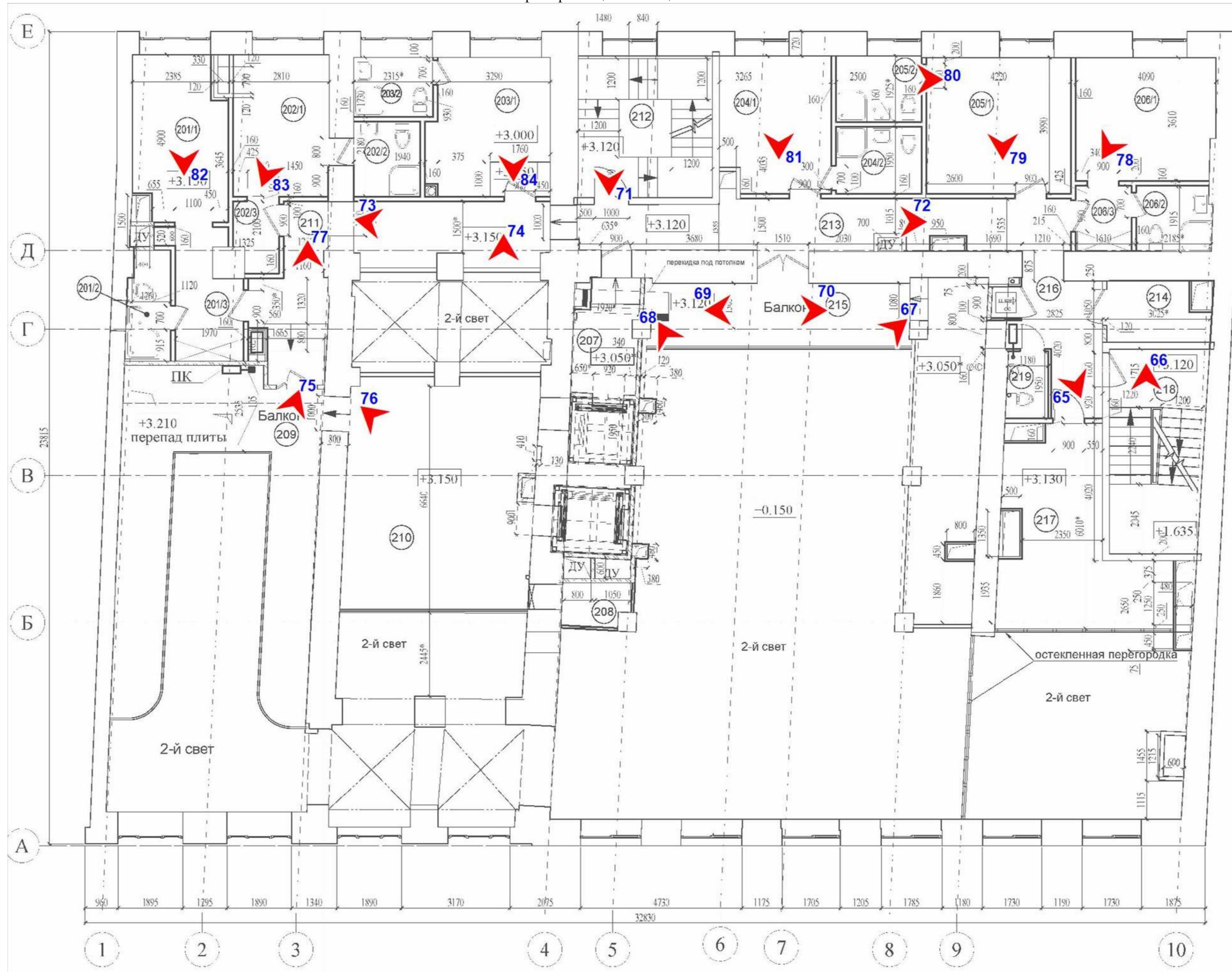
Схема фотофиксации помещений 1-го этажа
