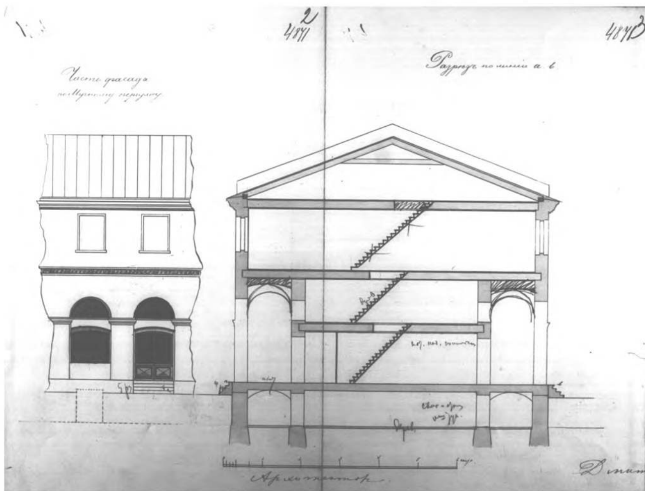
Илл. 64. Малый Гостиный двор. Большой железный ряд. Фасад и разрез лавки № 2. 1880 г. Архитектор Д.В. Знобишин. ЦГИА СПб. Ф. 515. Оп. 4. Д. 3604. Л.2-3.
