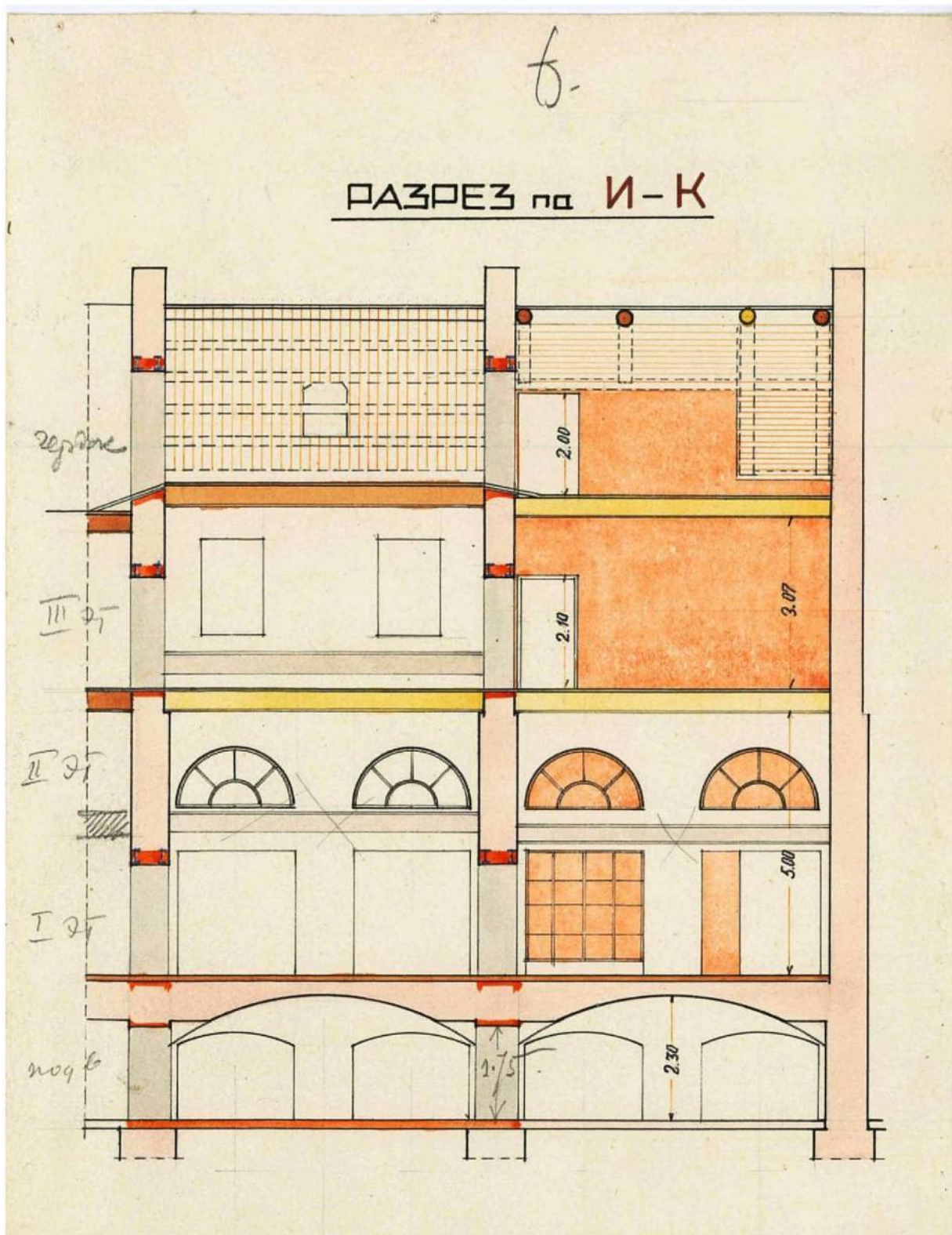
Илл. 139. Проект соединения лавок №№ 12-19. 1929 г. ЦГА НТД. Ф. 192. Оп. 31. Д. 5481. Л. 38-39.
