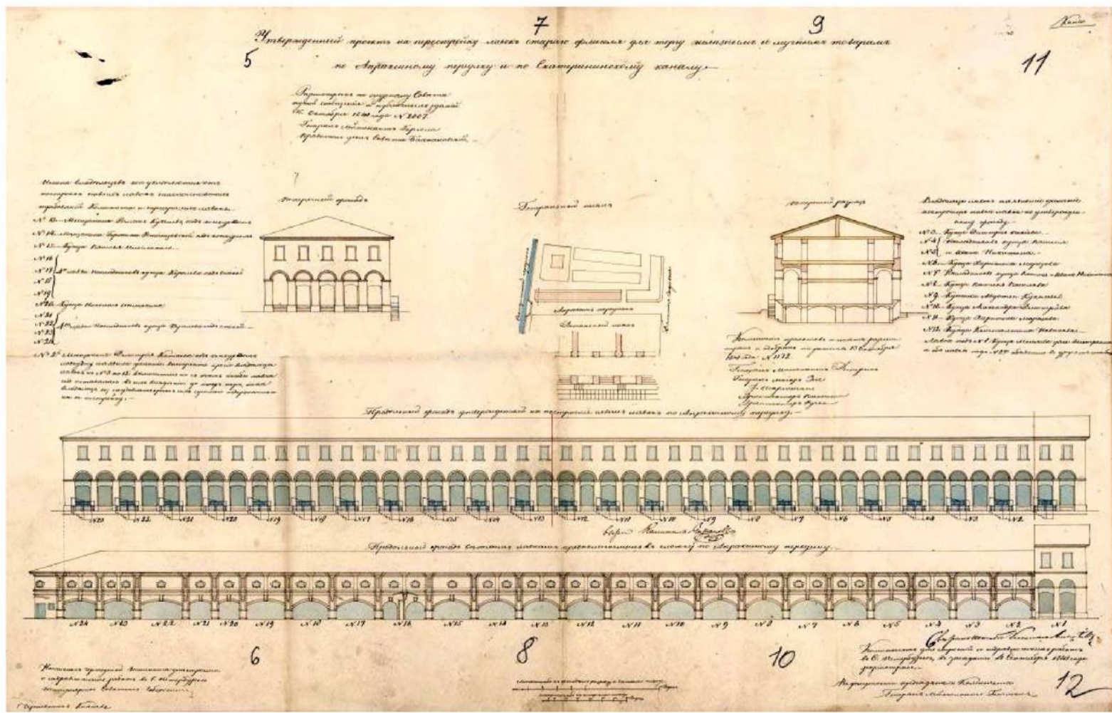
Илл. 48. Проект перестроек ветхих лавок для торгу железным и мучным товаром. Проектный и фиксационный чертежи. 1841 г. ЦГИА СПб. Ф. 513. Оп. 176. Д. 186. Лл. 5-12.
