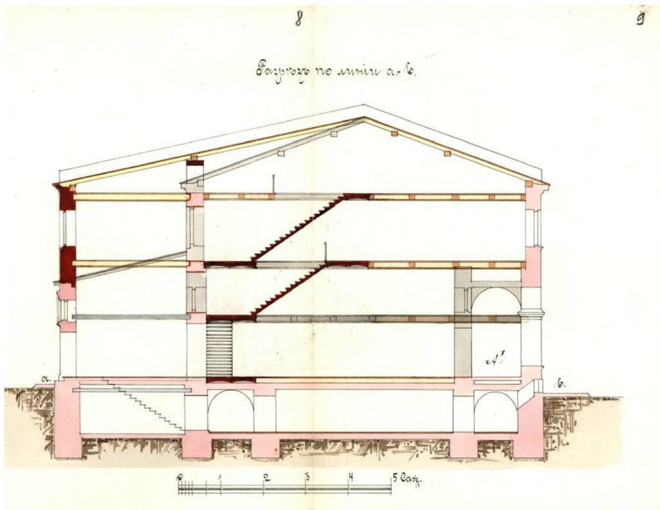
Илл. 107. Малый Гостиный двор. Большой железный ряд. Проект перестройки. Лавки № 8-10. Закрытие галерей, устройство лестницы, надстройка пристройки со стороны Москательного пер. 1903 г. Архитектор А. Ковшаров. Разрез. ЦГИА СПб. Ф. 513. Оп. 115. Д. 661. Л. 8-9.
