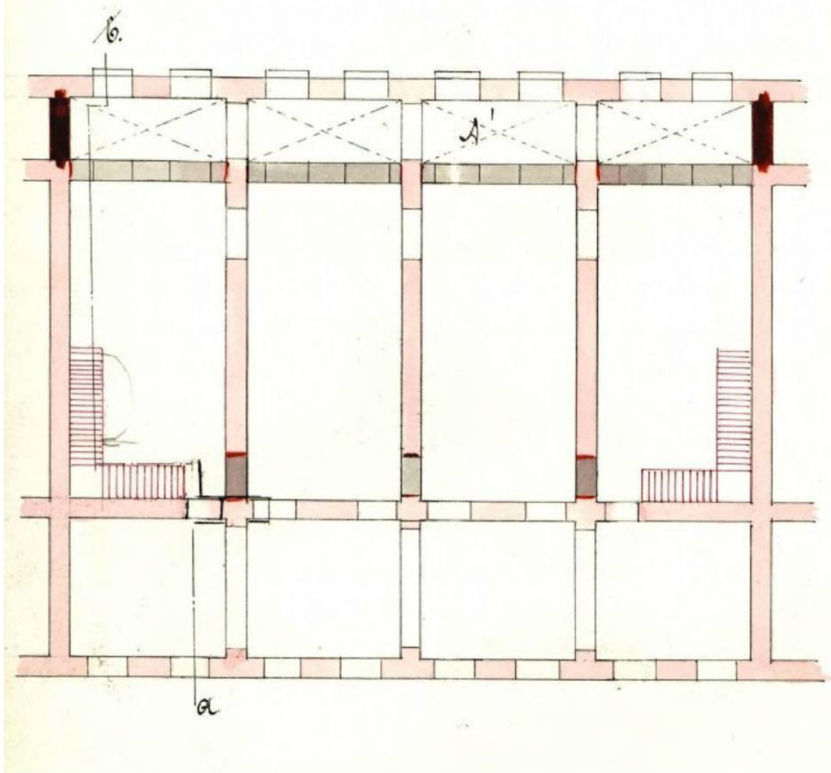
Илл. 104. Малый Гостиный двор. Большой железный ряд. Проект перестройки. Лавки № 8-10. Закрытие галерей, устройство лестницы, надстройка пристройки со стороны Москательного пер. 1903 г. Архитектор А. Ковшаров. План 1 этажа. ЦГИА СПб. Ф. 513. Оп. 115. Д. 661. Л. 5.
