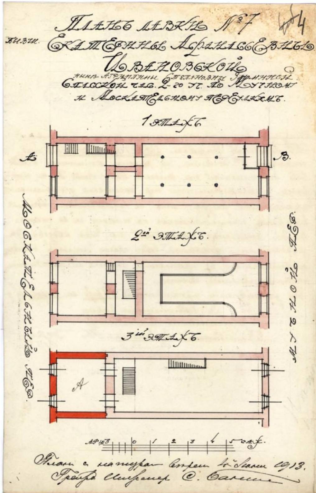
Илл. 99. Малый Гостиный двор. Большой железный ряд. Проект устройства антресоли. Лавка № 7. 1913 г. Гражданский инженер С. Баниге. Планы. ЦГИА СПб. Ф. 513. Оп. 115. Д. 660. Л. 4.
