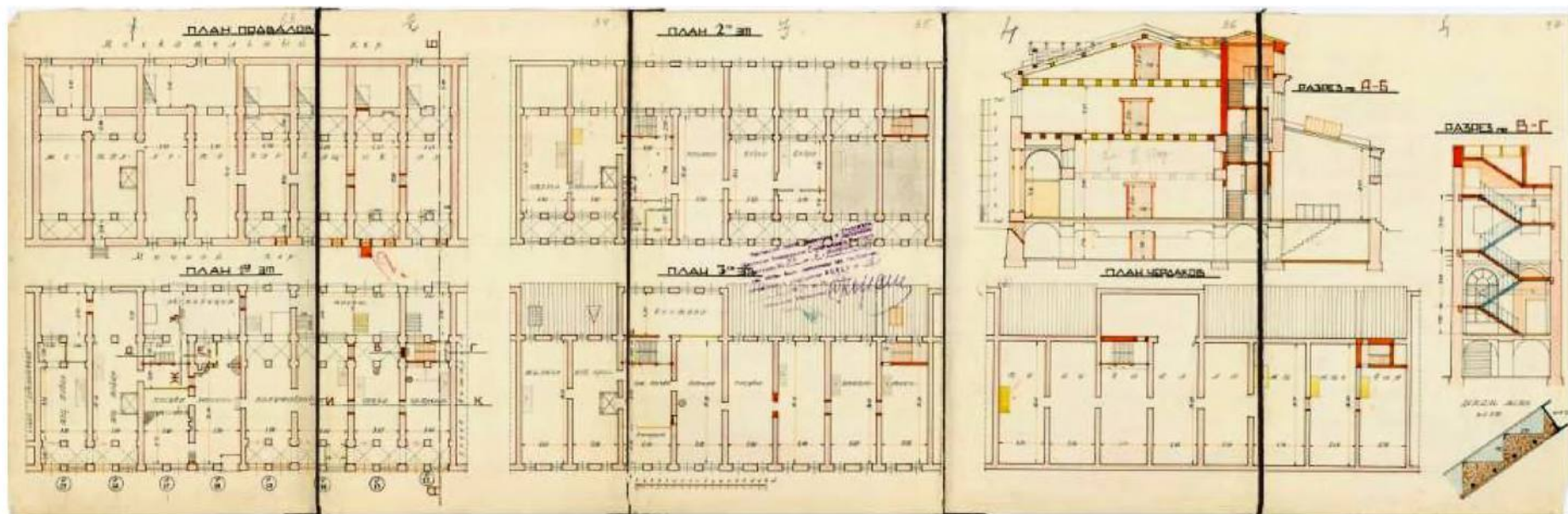
Илл. 132. Проект соединения лавок №№ 12-19. 1929 г. ЦГА НТД, Ф. 192. Оп. 31. Д. 5481. Л. 26-32. Л. 33-37
