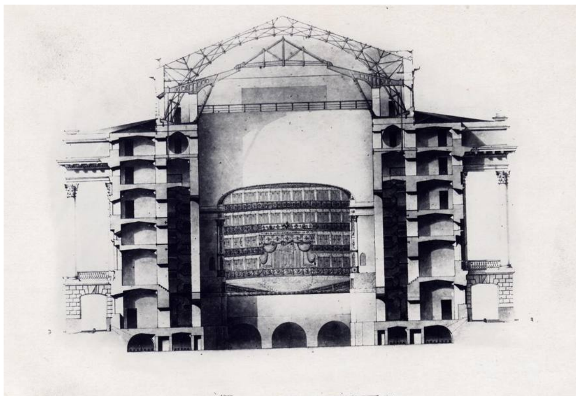
Илл. 17. Разрез зала и амфитеатра. (ФГБУК «Национальный драматический театр России (Александринский театр)», литературный отдел)
