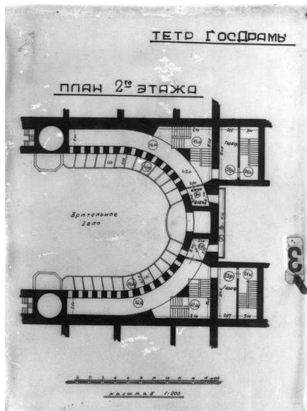
Илл. 38. План 2-го этажа. 1932 г. (ФГБУК «Национальный драматический театр России (Александринский театр)», литературный отдел)
