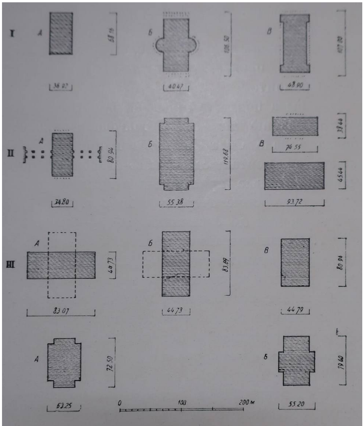
Илл. 3. Размеры здания театра по различным вариантам генерального плана и в натуре (М. Тарановская. Здание Академического театра драмы имени А.С. Пушкина (б. Александринский) в Ленинграде. Архитектор К. Росси. Государственное издательство литературы по строительству и архитектуре. Ленинград. 1956 г.)
