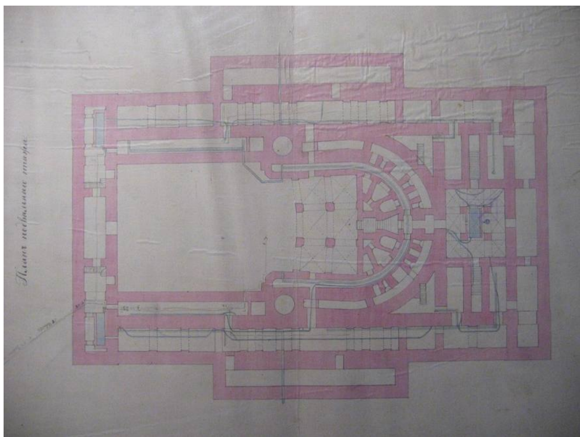
Илл. 25. План подвала. И.И. Климов. 1864 г. (Музей театрального и музыкального искусства)
