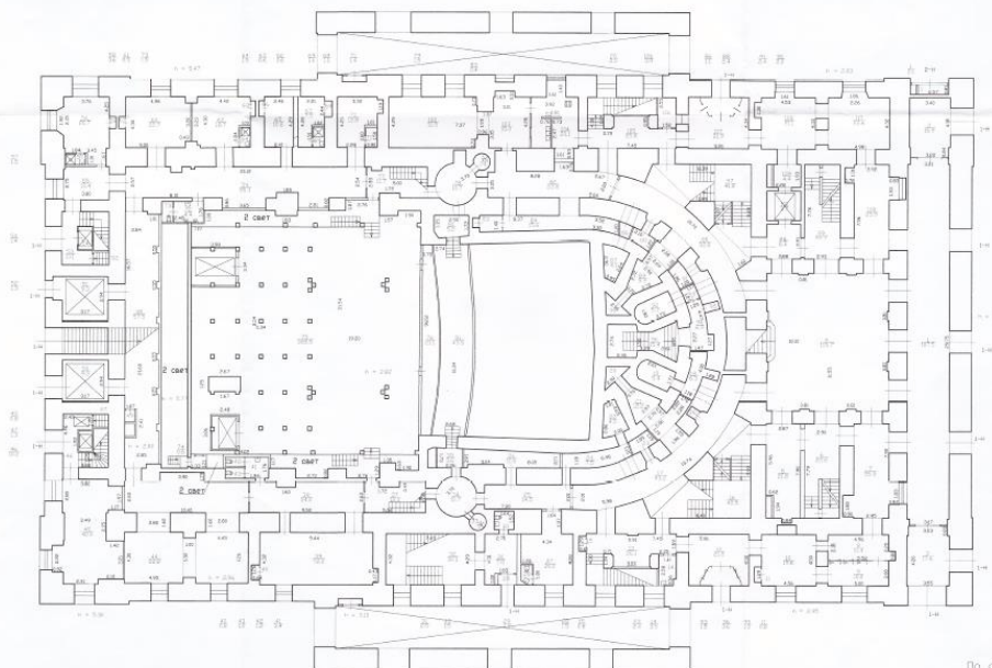
План 1 этажа
