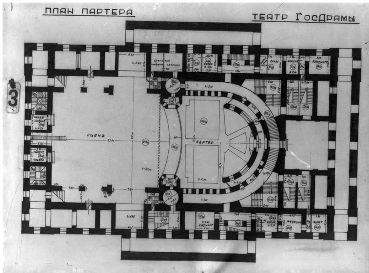
Илл. 36. План партера. 1932 г. (ФГБУК «Национальный драматический театр России (Александринский театр)»), литературный отдел
