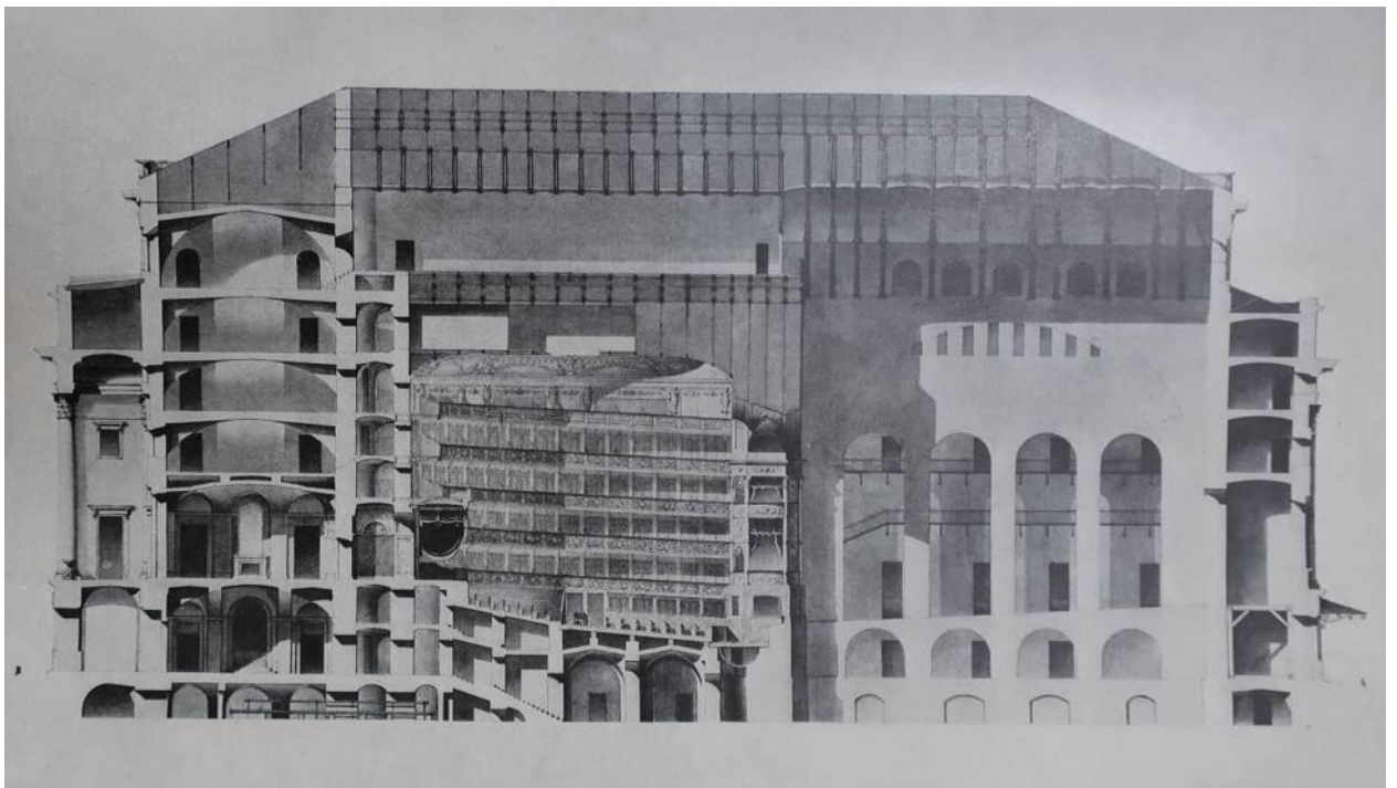
Илл. 15. Продольный разрез. Исполнительный чертёж, 1832 г. (Научно-исследовательский музей при Российской академии художеств)
