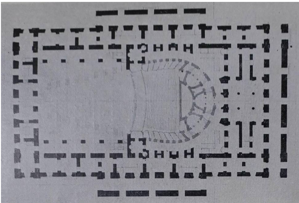
Илл. 8. План 1-го этажа, вариант, составленный в процессе строительства, 1828-1829 гг. (Научно-исследовательский музей при Российской академии художеств)
