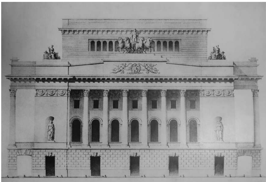
Илл. 18. Главный фасад. Исполнительный чертёж, 1832 г. (Оригинал не сохранился. Репродукция с фотографии. Фотоархив Института истории материальной культуры Российской Академии наук)
