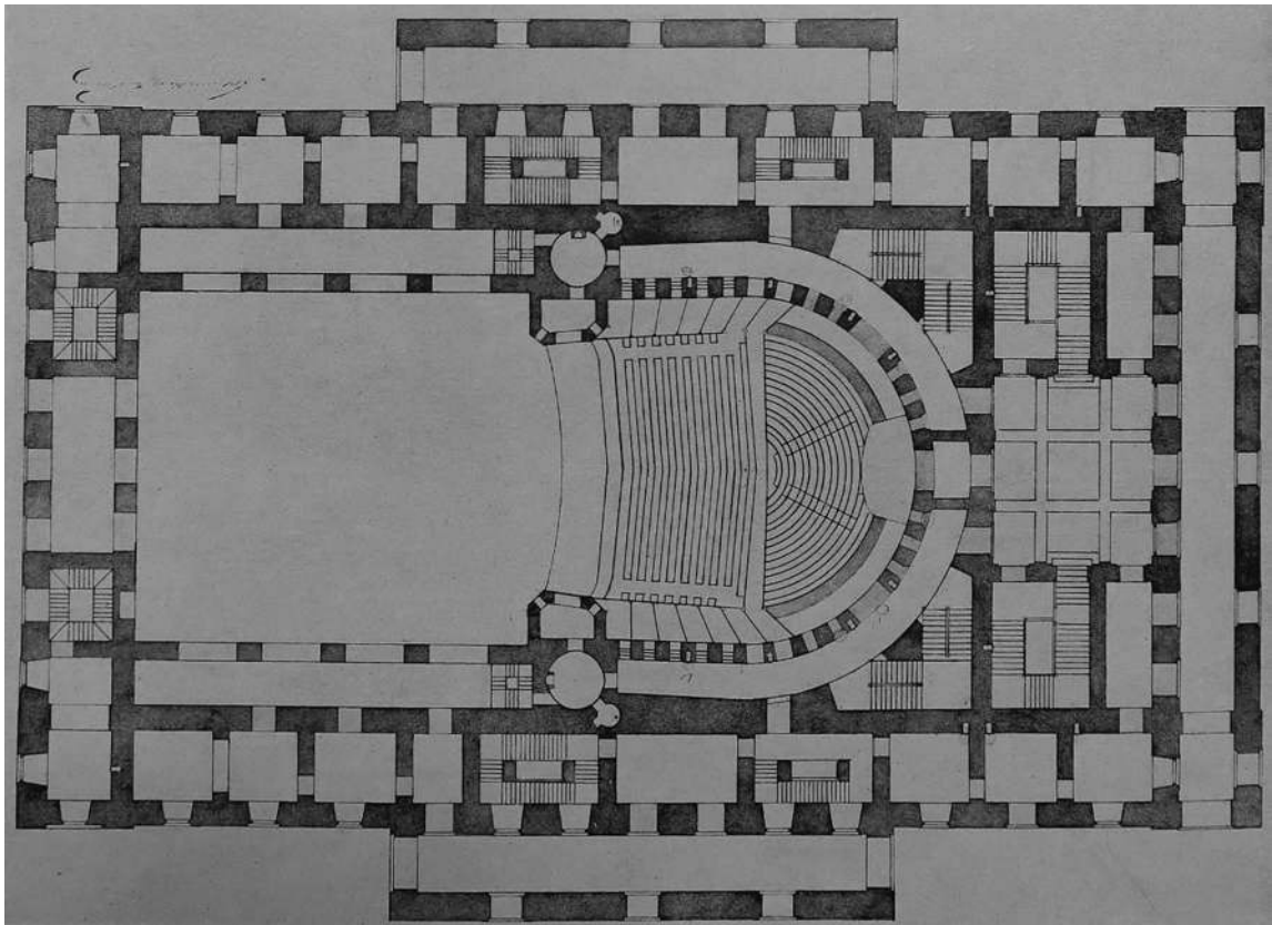
Илл. 12. План 1-го этажа. Исполнительный чертёж, 1832 г. (Научно-исследовательский музей при Российской академии художеств)
