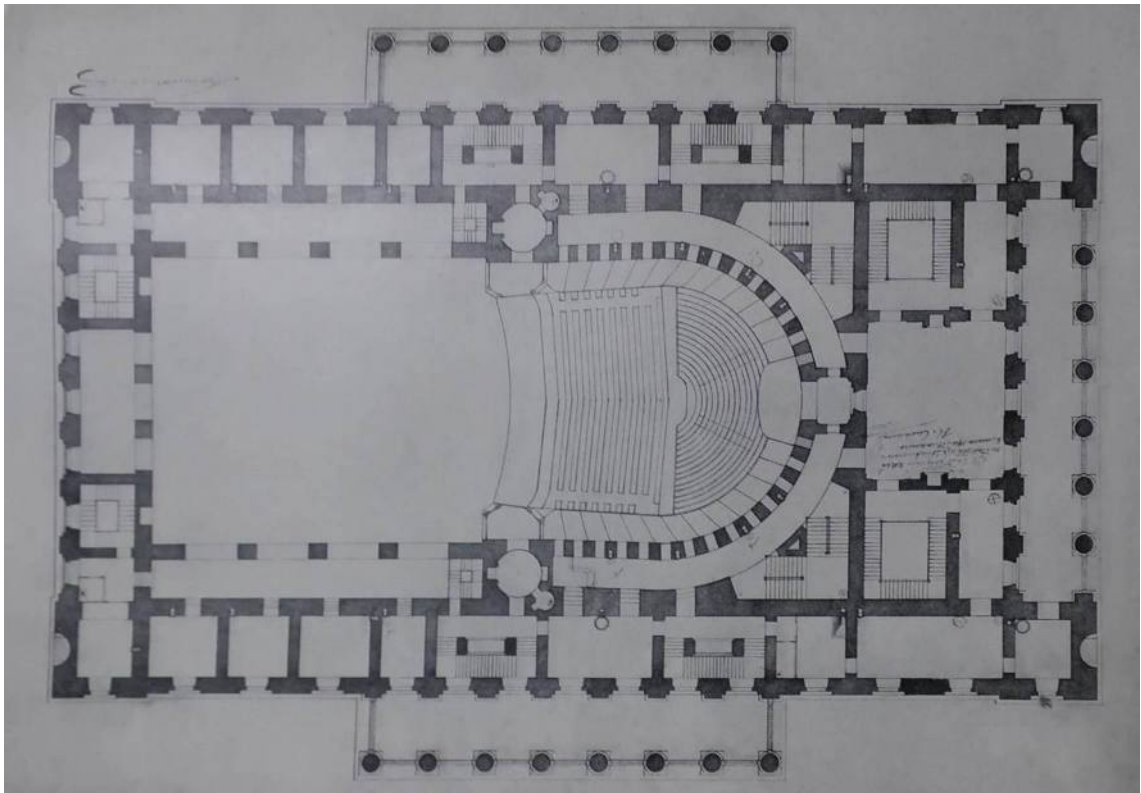
Илл. 13. План 2-го этажа. Исполнительный чертёж, 1832 г. (Научно-исследовательский музей при Российской академии художеств)
