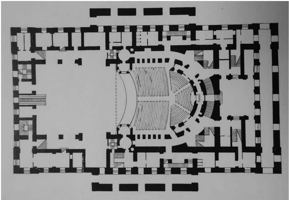
Илл. 64. План 1-го этажа и партера. Обмер, 1954 г. (М. Тарановская. Здание Академического театра драмы имени А.С. Пушкина (б. Александринский) в Ленинграде. Архитектор К. Росси. Государственное издательство литературы по строительству и архитектуре. Ленинград. 1956 г.)
