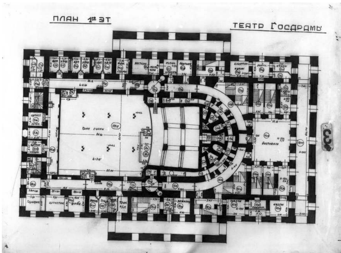
Илл. 35. План 1-го этажа. 1932 г. (ФГБУК «Национальный драматический театр России (Александринский театр)», литературный отдел)
