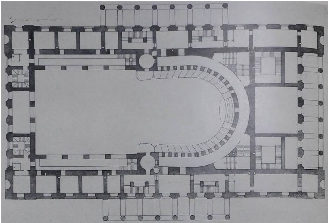
Илл. 14. План 3-го яруса лож. Исполнительный чертёж, 1832 г. (Научно-исследовательский музей при Российской академии художеств)
