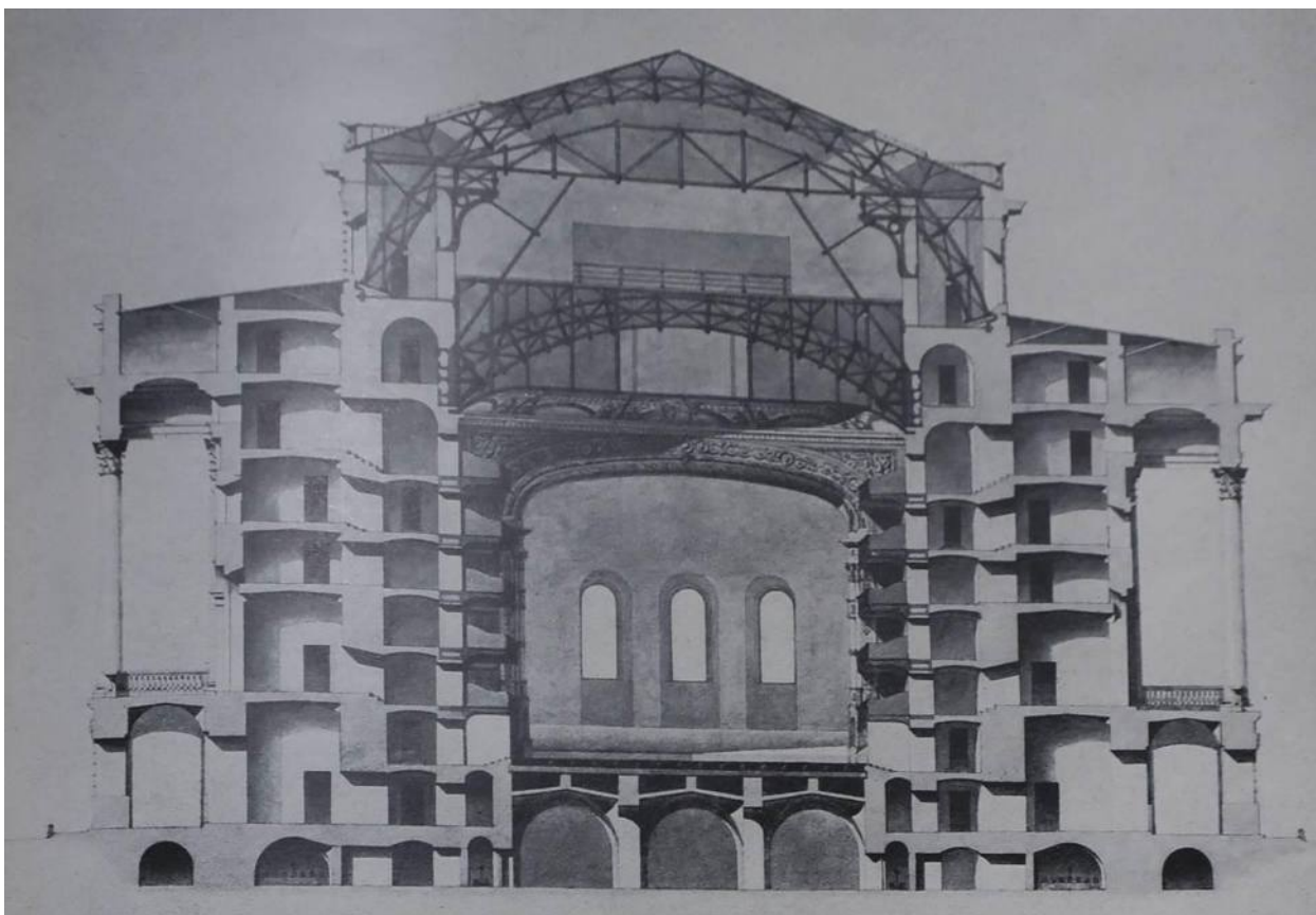
Илл. 16. Поперечный разрез. Исполнительный чертёж, 1832 г. (Научно-исследовательский музей при Российской академии художеств)
