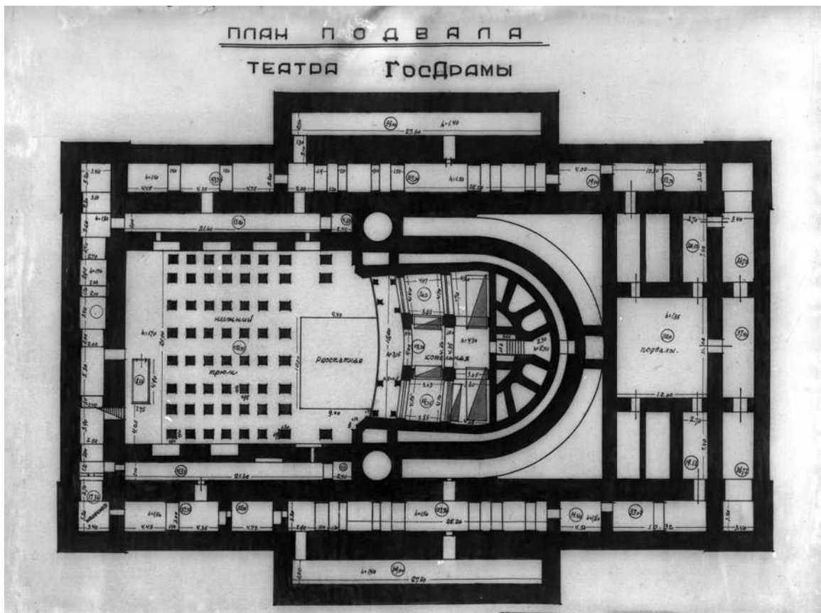
Илл. 34. План подвала. 1932 г. (ФГБУК «Национальный драматический театр России (Александринский театр)», литературный отдел)
