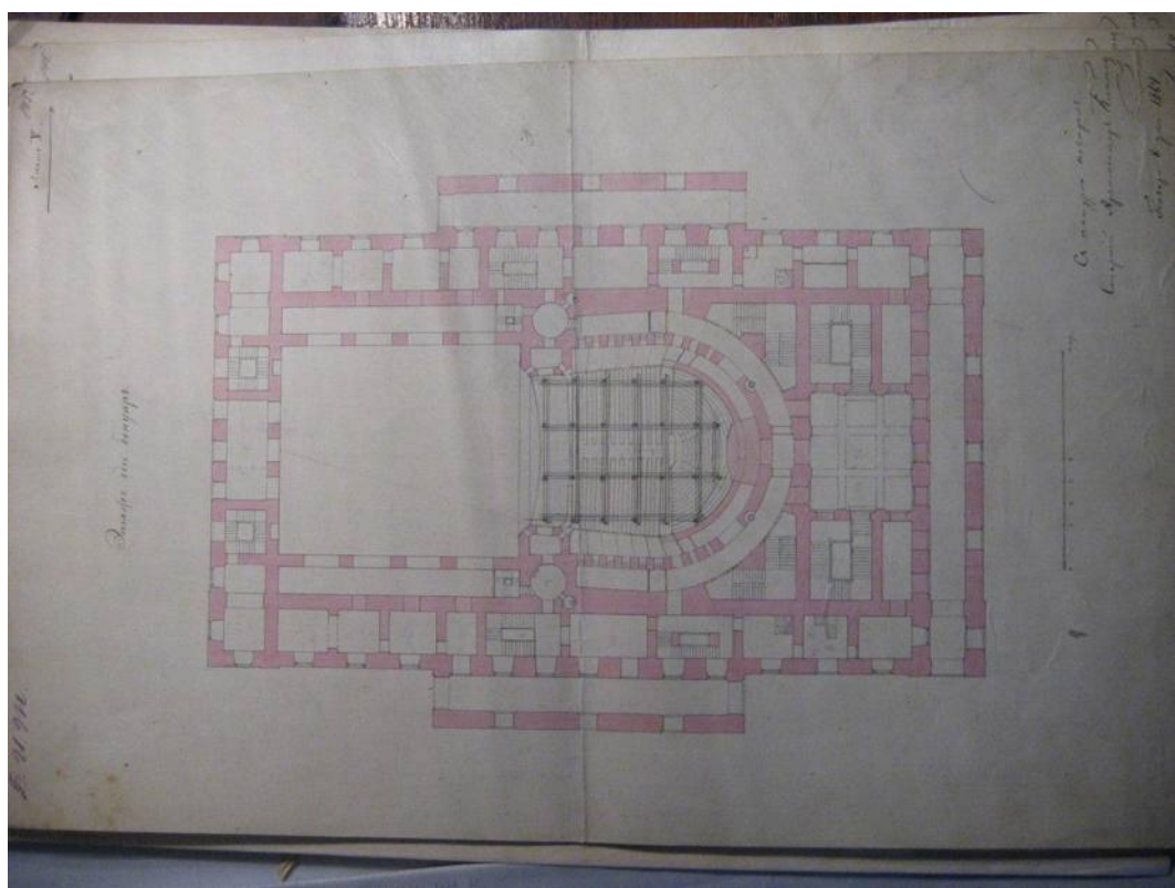
Илл. 27. План партера. И.И. Климов. 1864 г. (Музей театрального и музыкального искусства)
