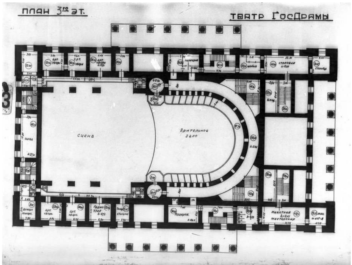
Илл. 39. План 3-го этажа. 1932 г. (ФГБУК «Национальный драматический театр России (Александринский театр)», литературный отдел)
