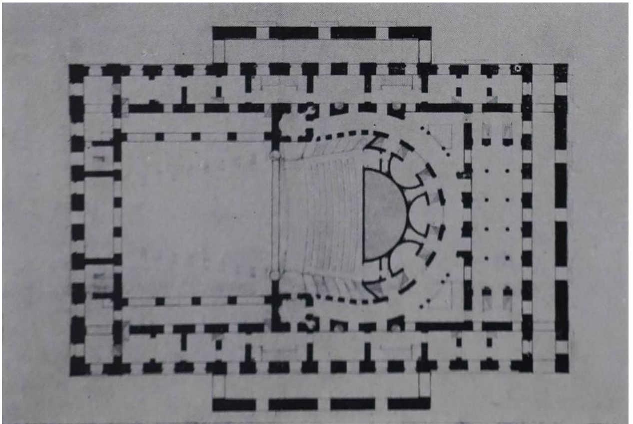
Илл. 6. План 1-го этажа, утверждённый проект, 1828 г. (РГИА)
