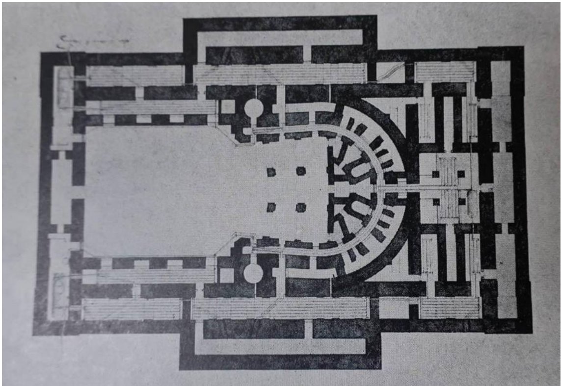
Илл. 11. План подвала с изображением системы парового отопления. Исполнительный чертёж, 1832 г. (Научно-исследовательский музей при Российской академии художеств)
