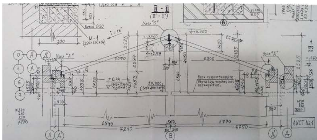
54. Разрез. Рабочий проект. 2004.
