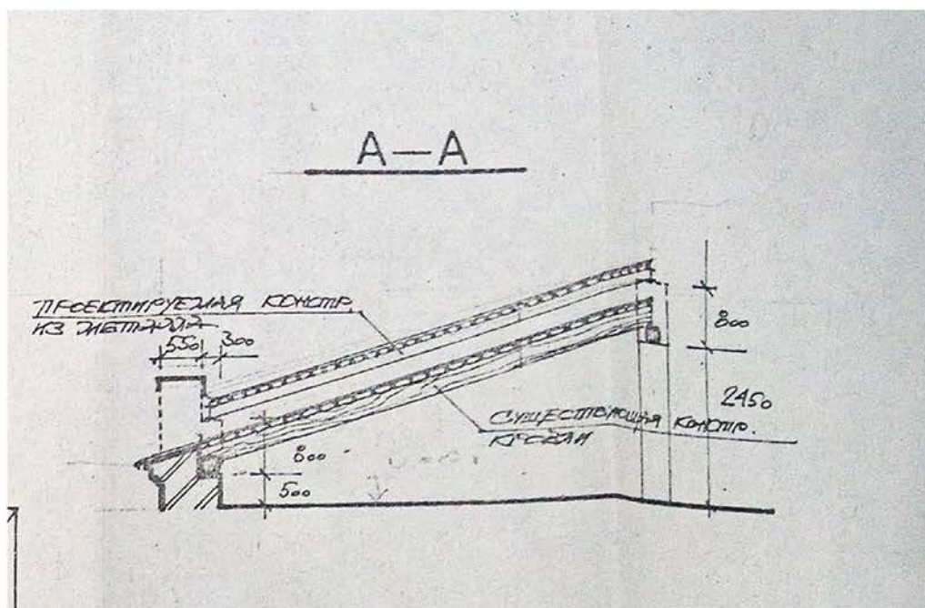
52. Разрез. Проект 1997.
