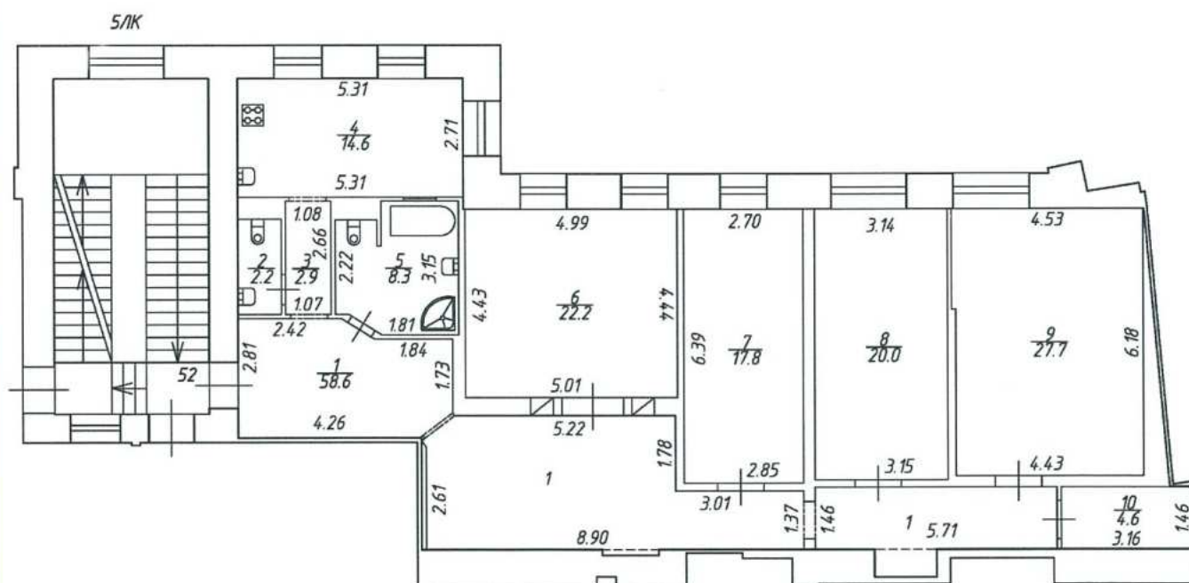
План квартиры 3 этаж
