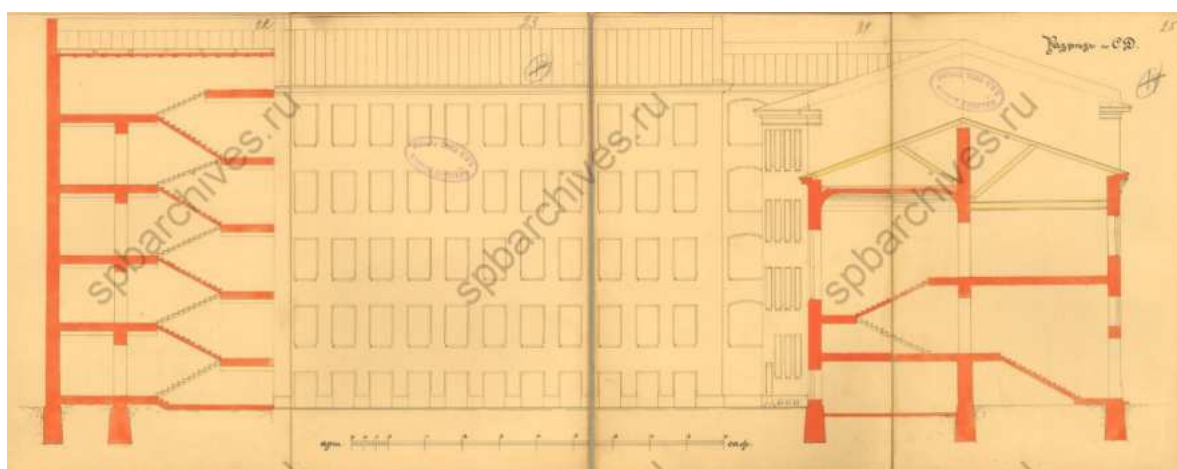
31. Чертеж дворовых фасадов, совмещенных с разрезами по линии CD. ЦГИА СПб. Фонд 513. Опись 102. Дело 7207
