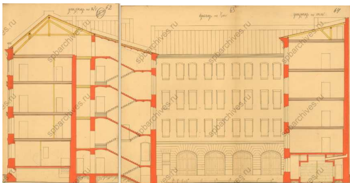
49. План дворового фасада, совмещенного с разрезом по линии к1-лм-мн. ЦГИА СПб. Фонд 513. Опись 102. Дело 7207
