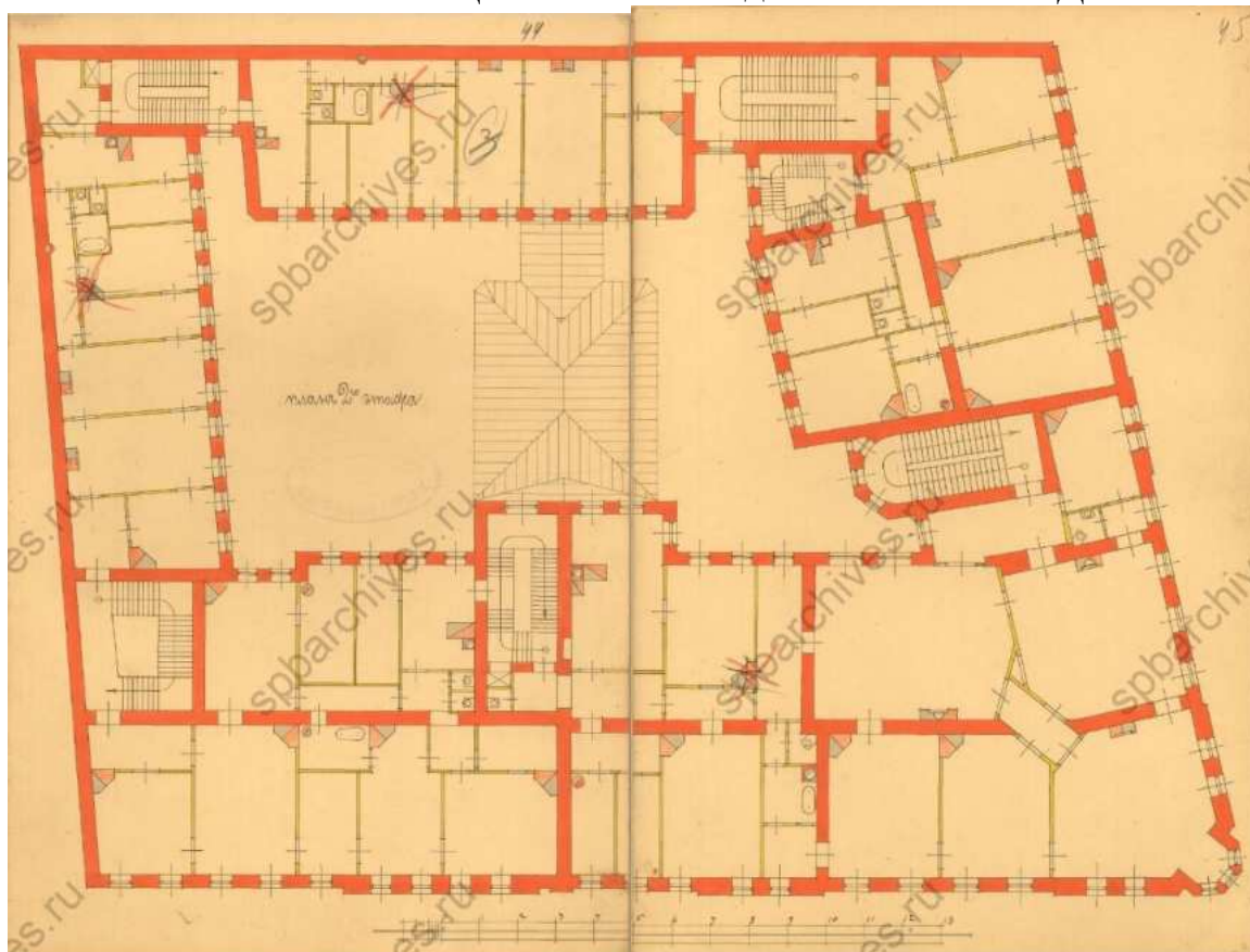
42. План 2-го этажа. ЦГИА СПб. Фонд 513. Опись 102. Дело 7207
