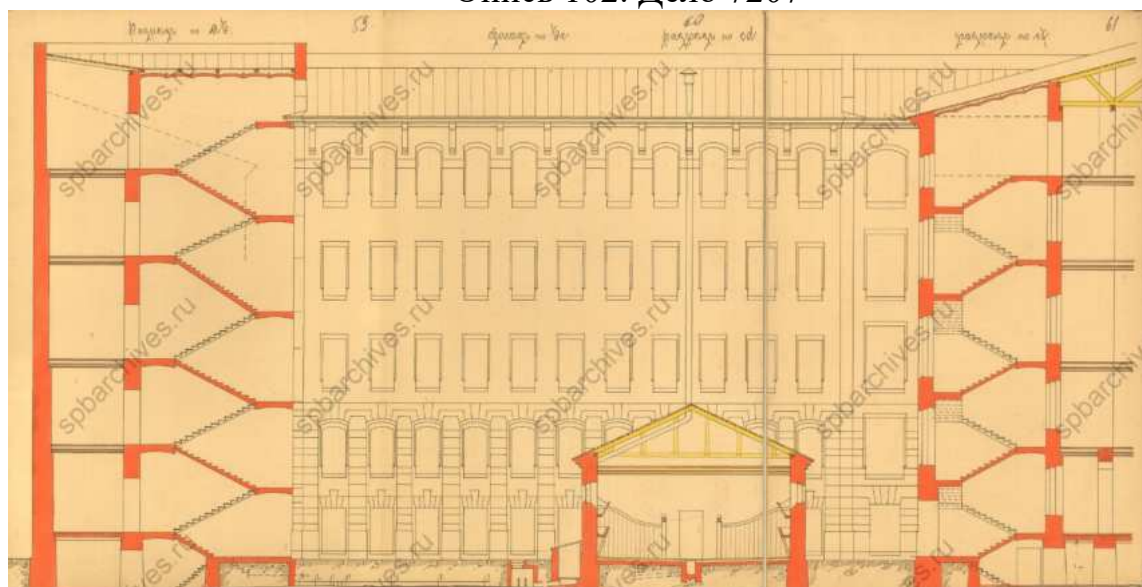
48. План дворового фасада, совмещенного с разрезом по линии а-б-вс-сд-еф. ЦГИА СПб. Фонд 513. Опись 102. Дело 7207
