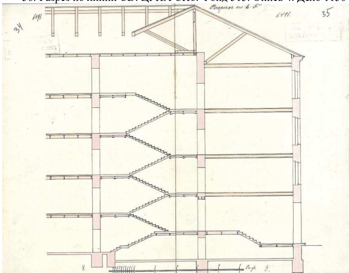
57. Разрез по линии EF. ЦГИА СПб. Фонд 515. Опись 4. Дело 1150
