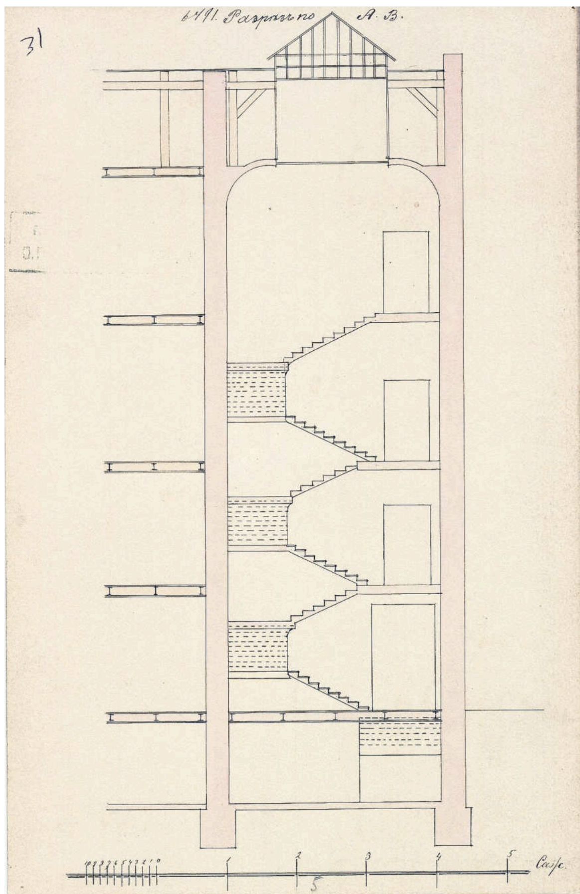
55. Разрез по линии АВ. ЦГИА СПб. Фонд 515. Опись 4. Дело 1150
