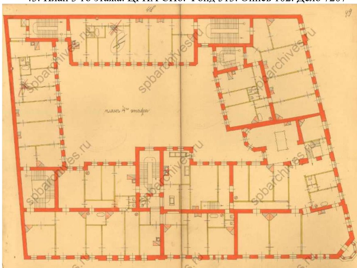
44. План 4-го этажа. ЦГИА СПб. Фонд 513. Опись 102. Дело 7207
