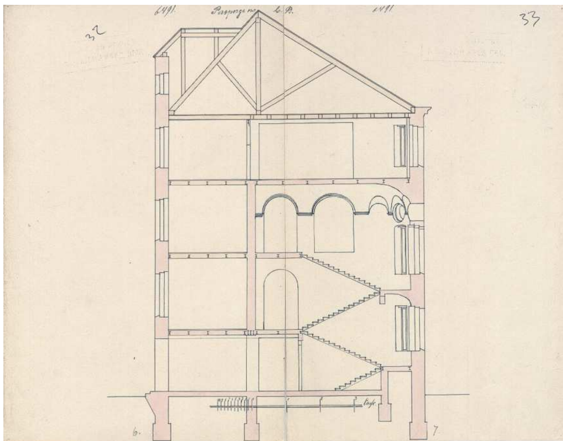
56. Разрез по линии CD. ЦГИА СПб. Фонд 515. Опись 4. Дело 1150
