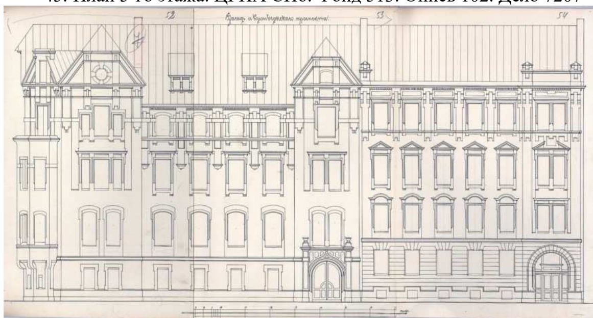
46. Фасад с Кронверкского проспекта. ЦГИА СПб. Фонд 513. Опись 102. Дело 7207
