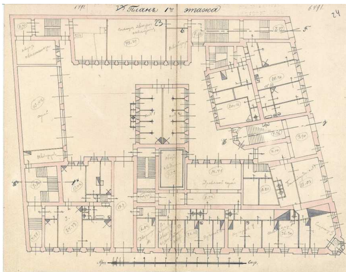
51. План 1-го этажа. ЦГИА СПб. Фонд 515. Опись 4. Дело 1150
