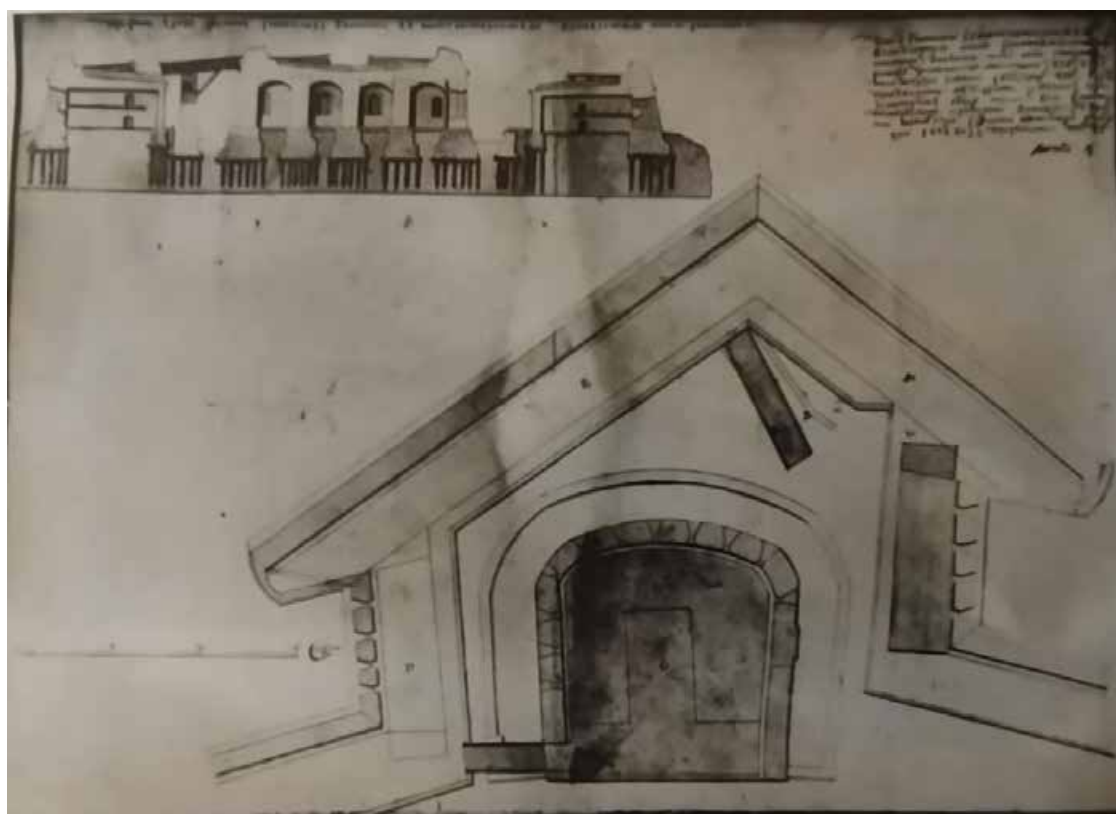
Илл.17. План и разрез бастиона с кавальером. 1750. РГА ВМФ. Копия: КГИОП, п. 90-17 (1) Н 1088.
