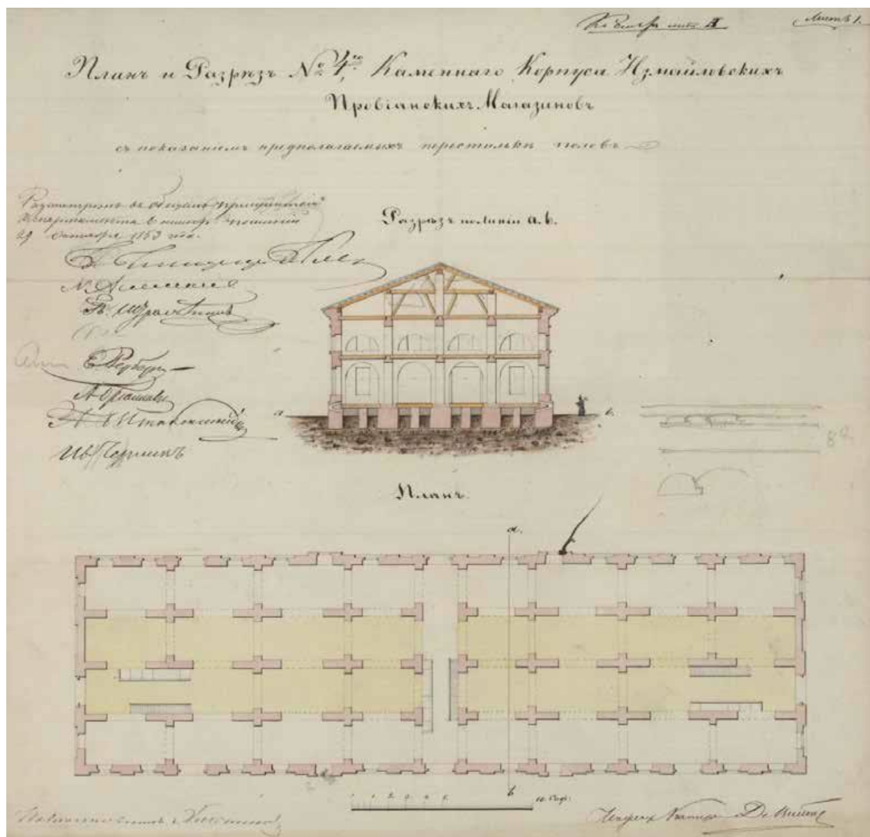
18. План и разрез № 4 каменного корпуса Измайловских провиантских магазинов. 1853 г. // РГА ВМФ. Ф. 3Л. Оп. 36. Д. 8938. Л. 1.
