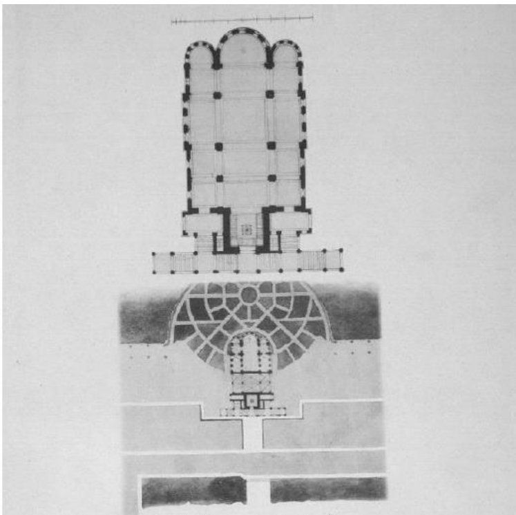
Фото 11. Проект А.А. Парланда и арх. Игнатия. Планы. Второй конкурс. 1882 г. (Зодчий. 1884. б/н. Л. 60.).
