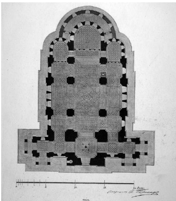
Фото 13. Храм Воскресения Христова. План. Исполнительный проект 1887 г. (Барановский В.Г. Архитектурная энциклопедия второй половины XIX века. Т.1. Архитектура исповеданий. СПб. 1902. С. 89.).
