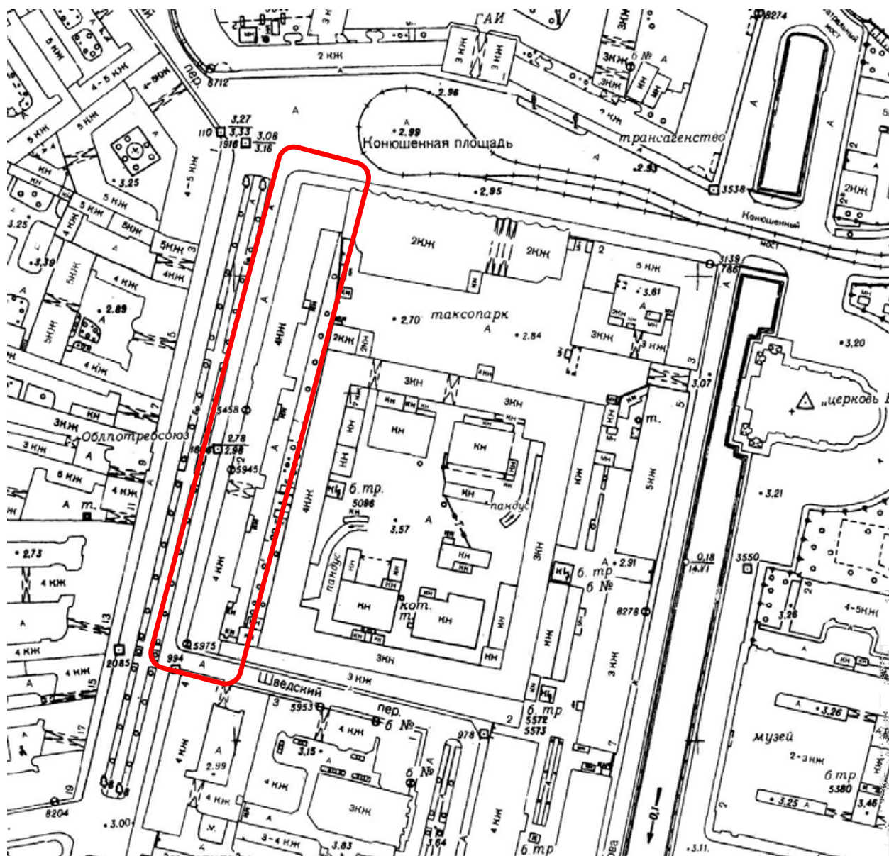
30. Топоъемка Ленинграда. 1983 г. Планшет 2429-07_83. Фрагмент.
