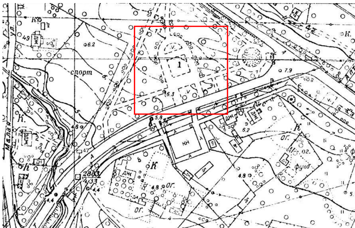
5. Топографическая съемка п. Репино. 1962 г. Архитектурно-планировочное управление исполкома Ленгорсовета. -2-XV-18. Планшет 3023-01. Архив КГА.
