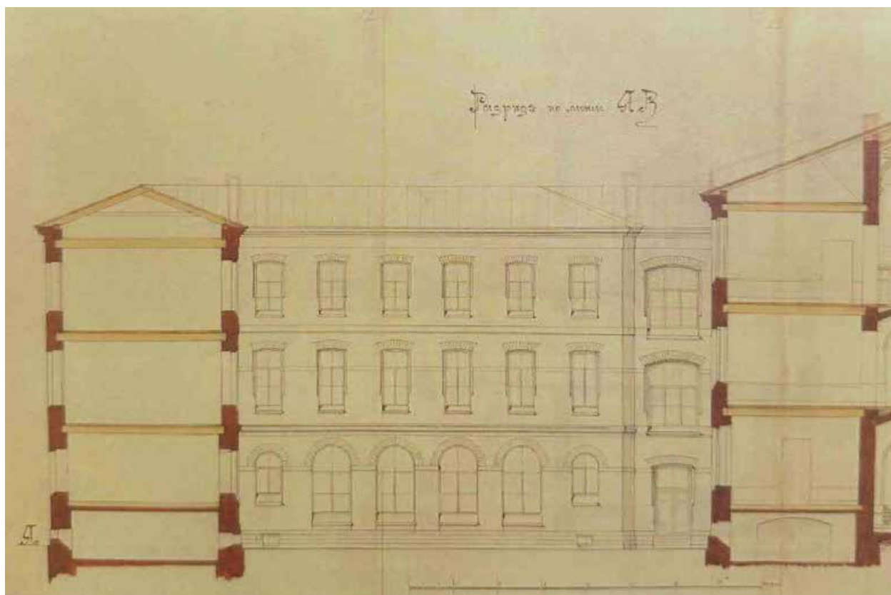
Илл.1. Разрез. Южный (дворовый) фасад. Восточный лицевой корпус. 1885 г. И.С.Китнер. ЦГИА СПб. Ф.513. Оп. 102. Д. 1218. Л. 22-23
