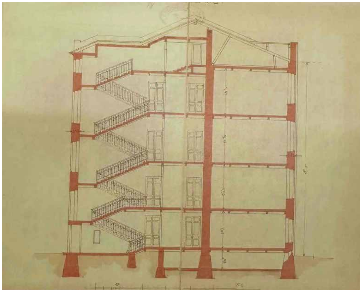
Илл. 15. Разрез лестницы южного дворового флигеля. Архитектор Г.Д. Гримм. 1913 г. ЦГИА СПб. Ф.513. Оп. 102. Д. 1218. Л.78-79
