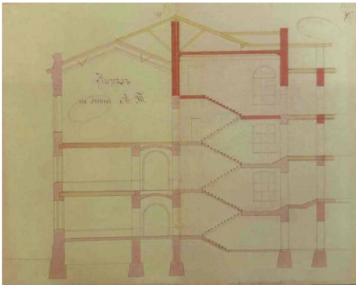
Илл.4. Разрез. Восточный лицевой корпус. 1905 г. ЦГИА СПб. Ф.513. Оп. 102. Д. 1218. Л. 44-45
