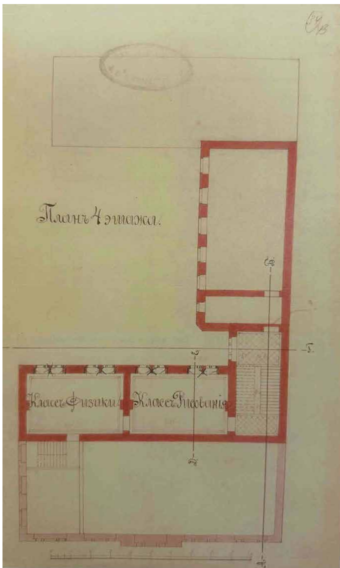
Илл.3. План 4-го этажа. Восточный лицевой корпус. 1905 г. ЦГИА СПб. Ф.513. Оп. 102. Д. 1218. Л. 43
