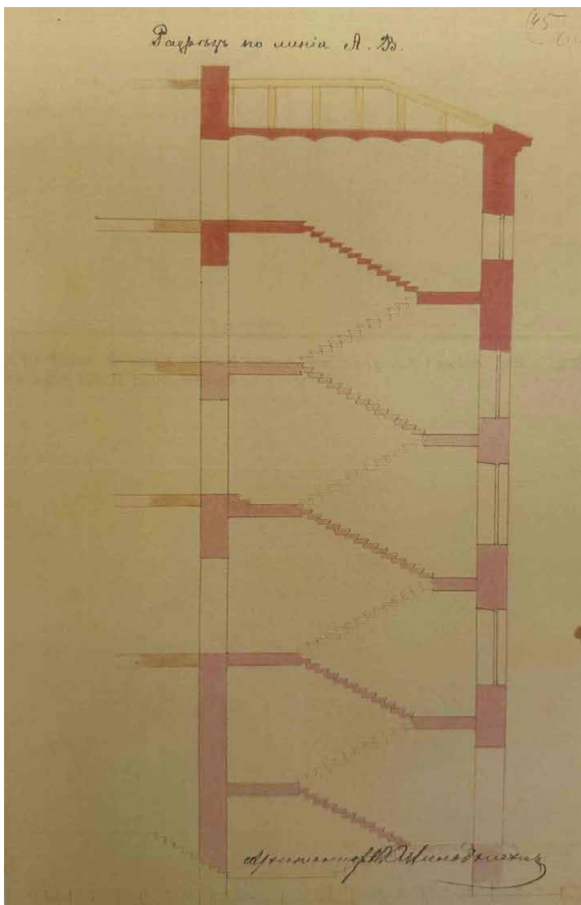
Илл.9. Разрез лестницы. Восточный лицевой корпус. [1906 г]. ЦГИА СПб. Ф.513. Оп. 102. Д. 1218. Л. 64
