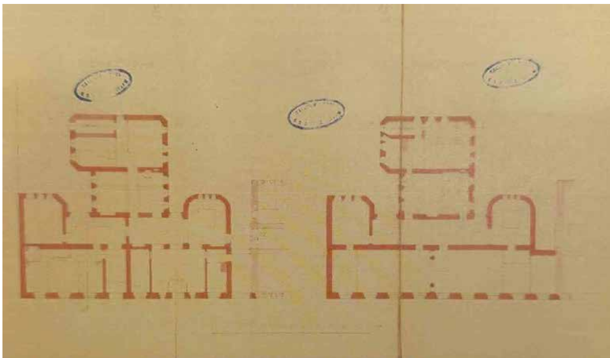
Илл.6. План 1-го и 2-го этажей. Западный лицевой корпус. Архитектор А.Р. Гавеман. 1908 г. ЦГИА СПб. Ф.513. Оп. 102. Д. 1218. Л. 55-57
