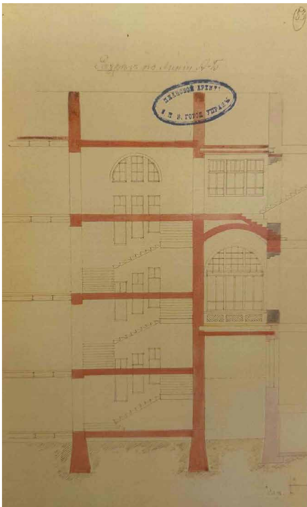
Илл.8. Разрез лестницы. Западный лицевой корпус. Архитектор А.Р. Гавеман. 1908 г. ЦГИА СПб. Ф.513. Оп. 102. Д. 1218.Л.61
