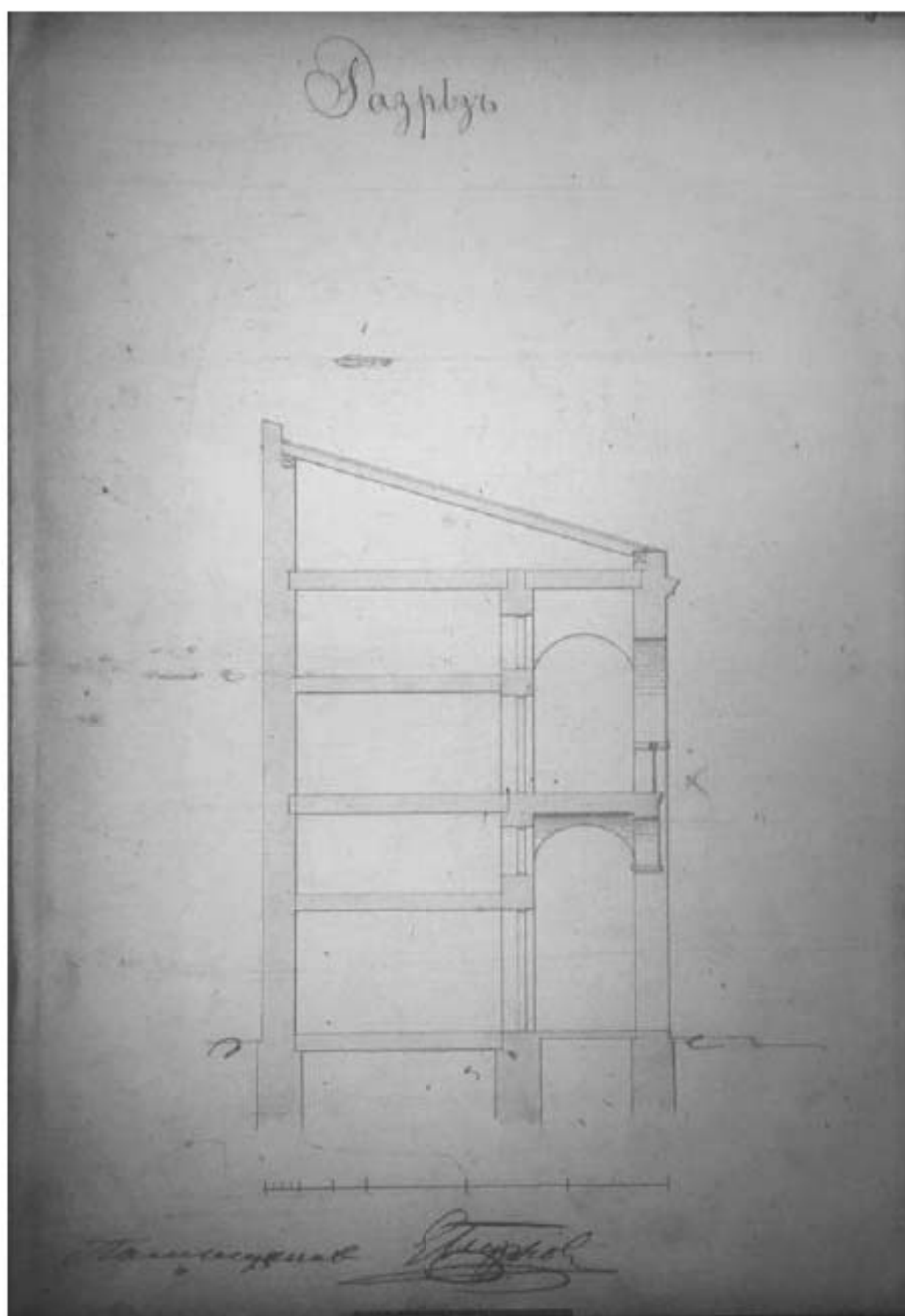
Илл. 14. Разрез лавок № 1, 2, 3. 1857 г. (источник: ЦГИА СПб. Ф. 513. Оп. 115. Д. 627).
