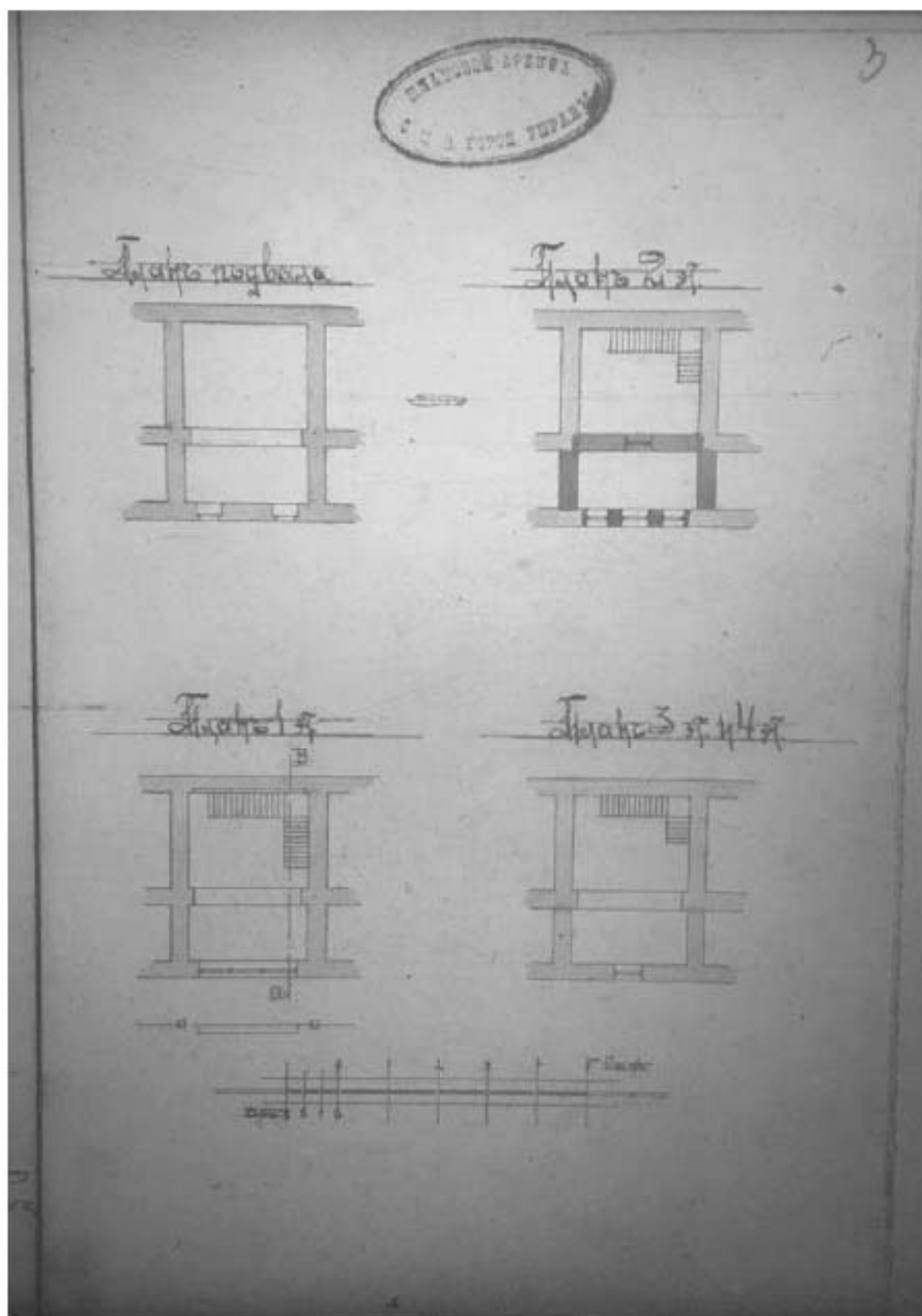
Илл. 62. Планы лавки № 12 с показанием предполагаемых к проведению работ. 1908 г. (источник: ЦГИА СПб. Ф. 513. Оп. 115. Д. 634).
