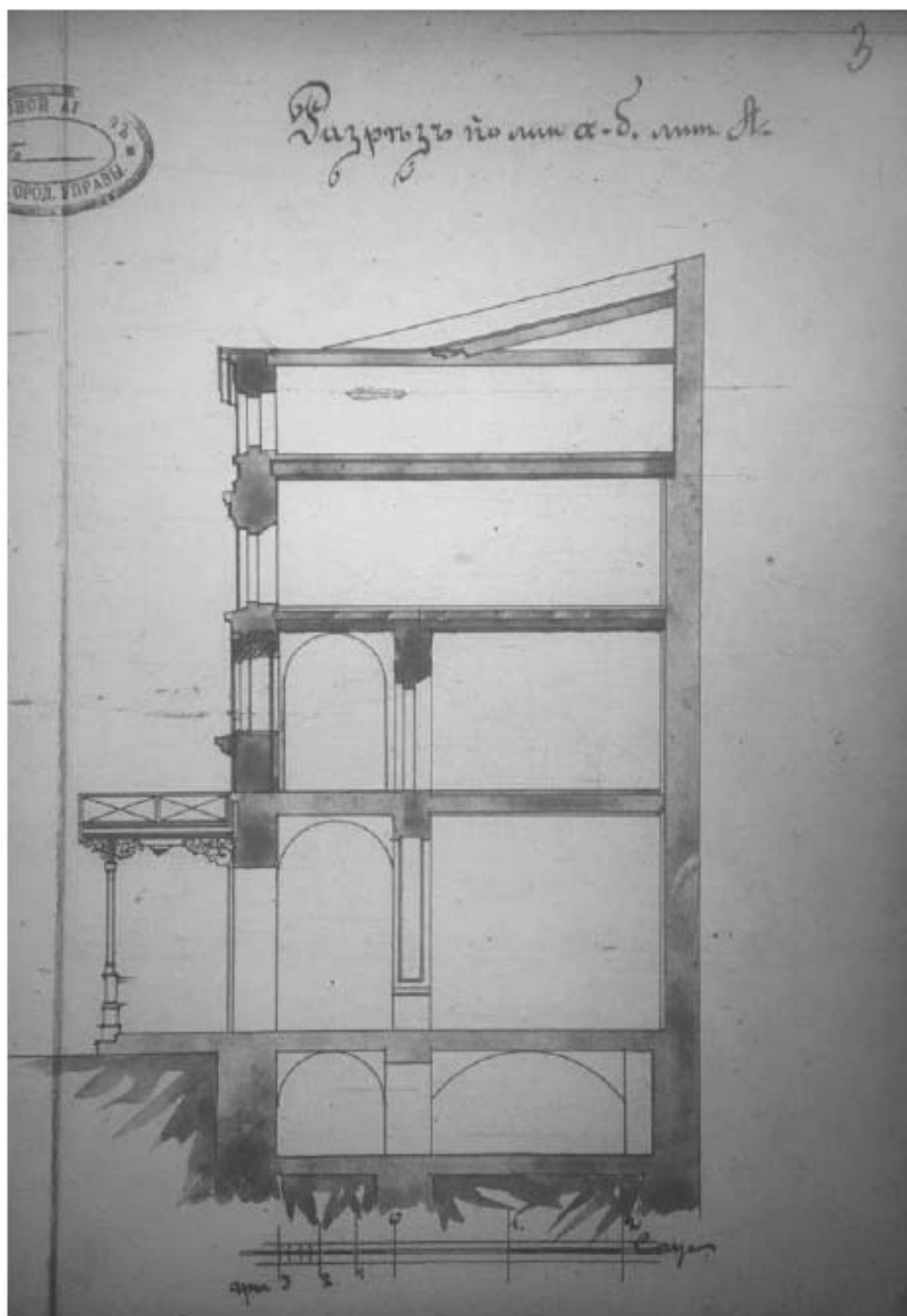
Илл. 56. Разрез лавки № 5 с показанием предполагаемых к проведению работ. 1911 г. (источник: ЦГИА СПб. Ф. 513. Оп. 115. Д. 629).
