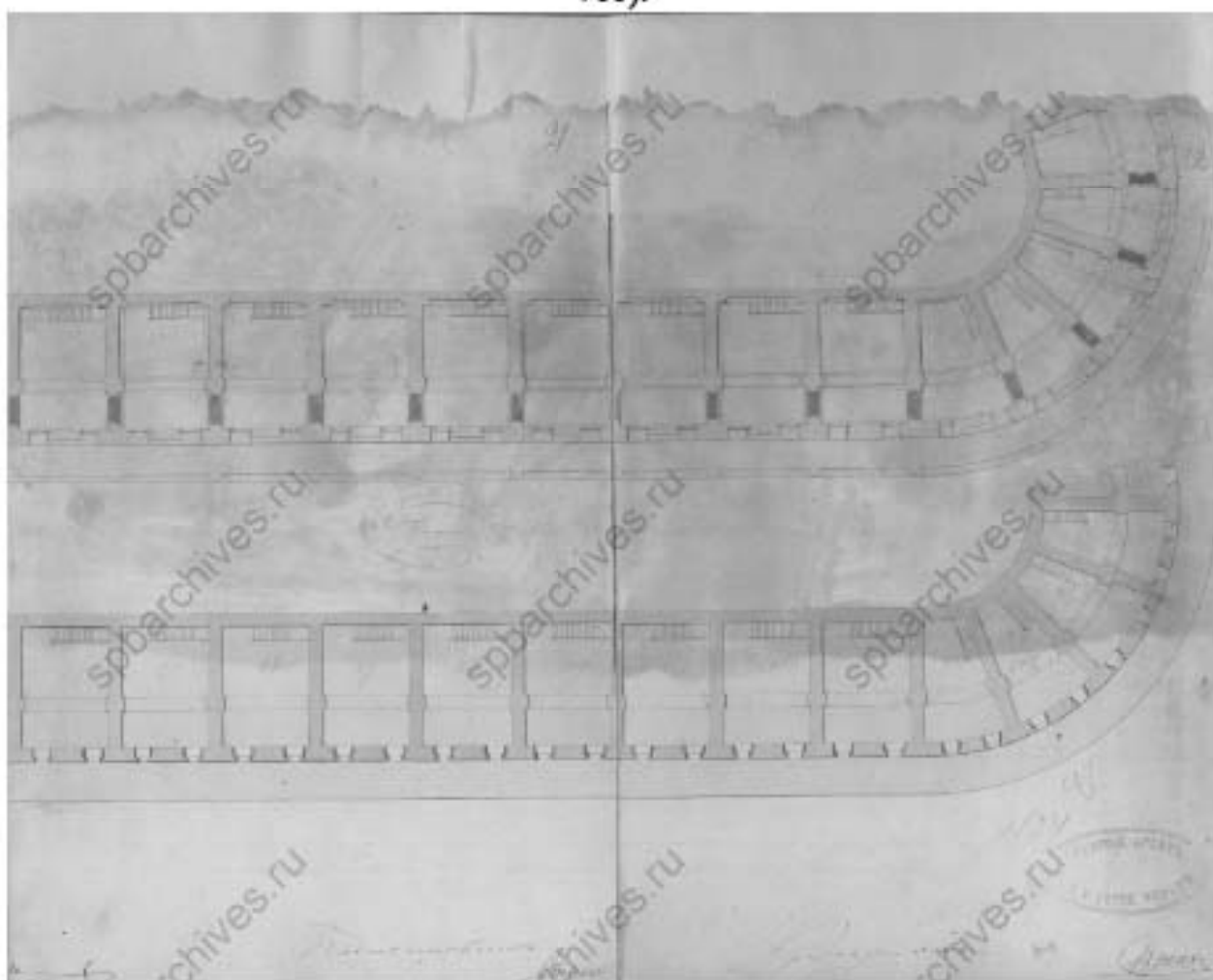
Илл. 28. План 1-го этажа и подвала лавок с показанием предполагаемых к проведению работ. Фрагмент. 1861 г. (источник: ЦГИА СПб. Ф. 513. Оп. 115. Д. 700).
