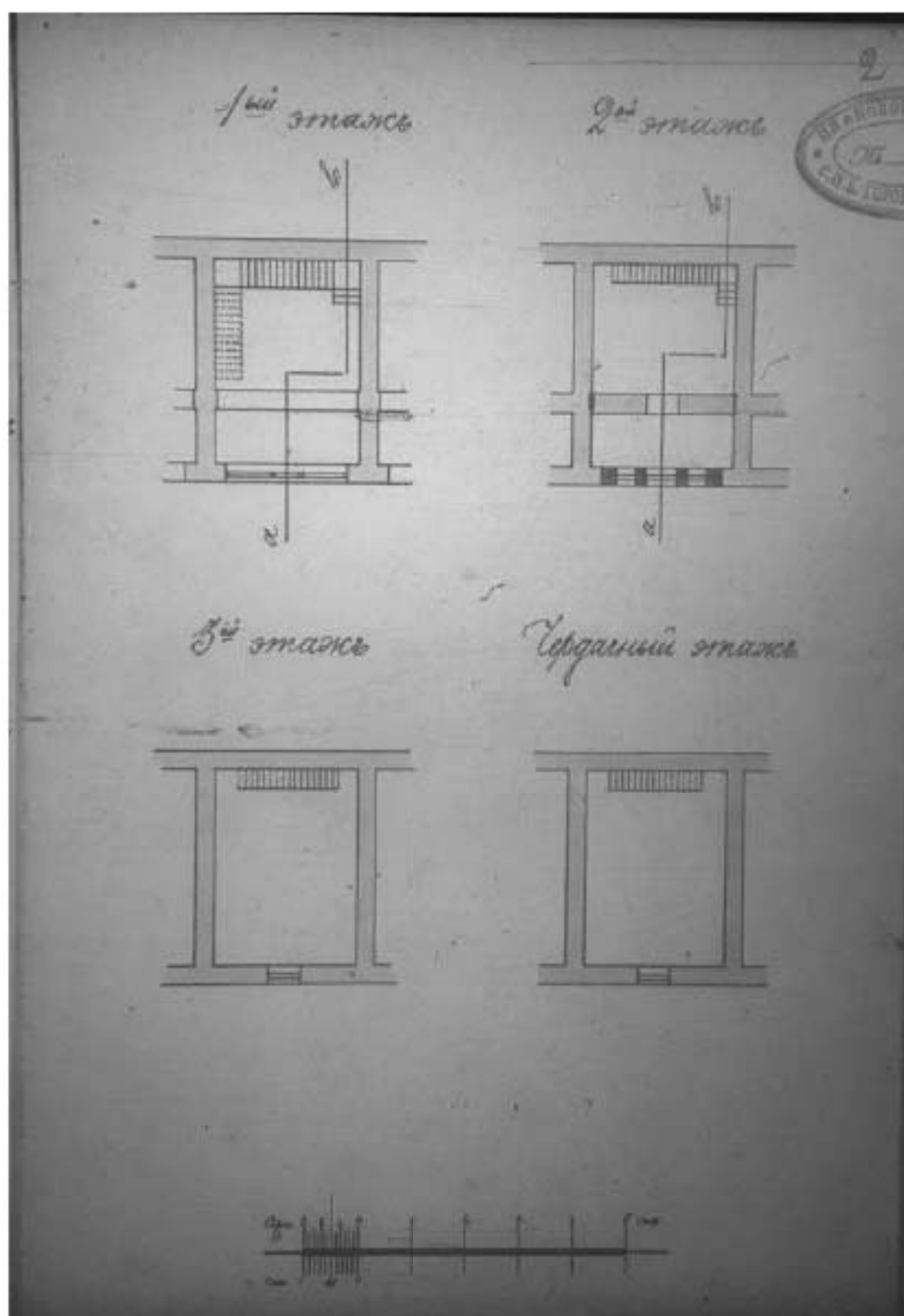
Илл. 80. План лавки № 19 с показанием предполагаемых к проведению работ. 1911 г. (источник: ЦГИА СПб. Ф. 513. Оп. 115. Д. 637).
