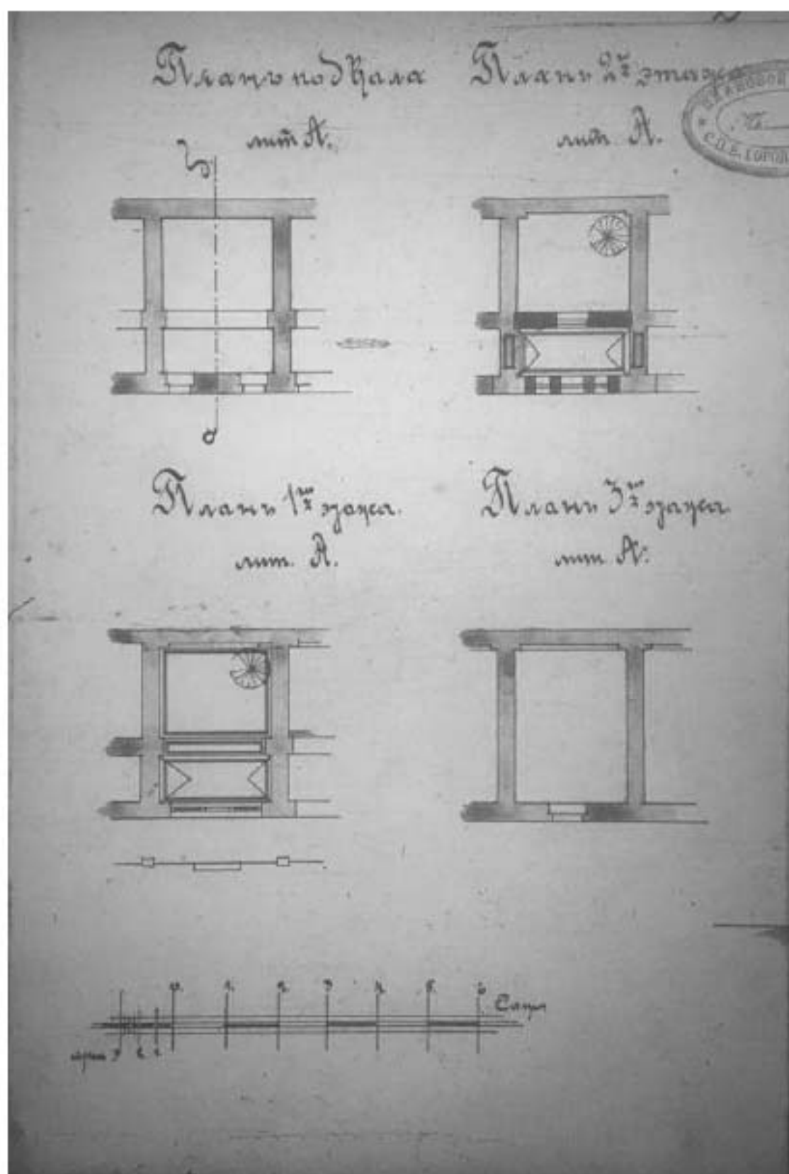
Илл. 55. План лавки № 5 с показанием предполагаемых к проведению работ. 1911 г. (источник: ЦГИА СПб. Ф. 513. Оп. 115. Д. 629).
