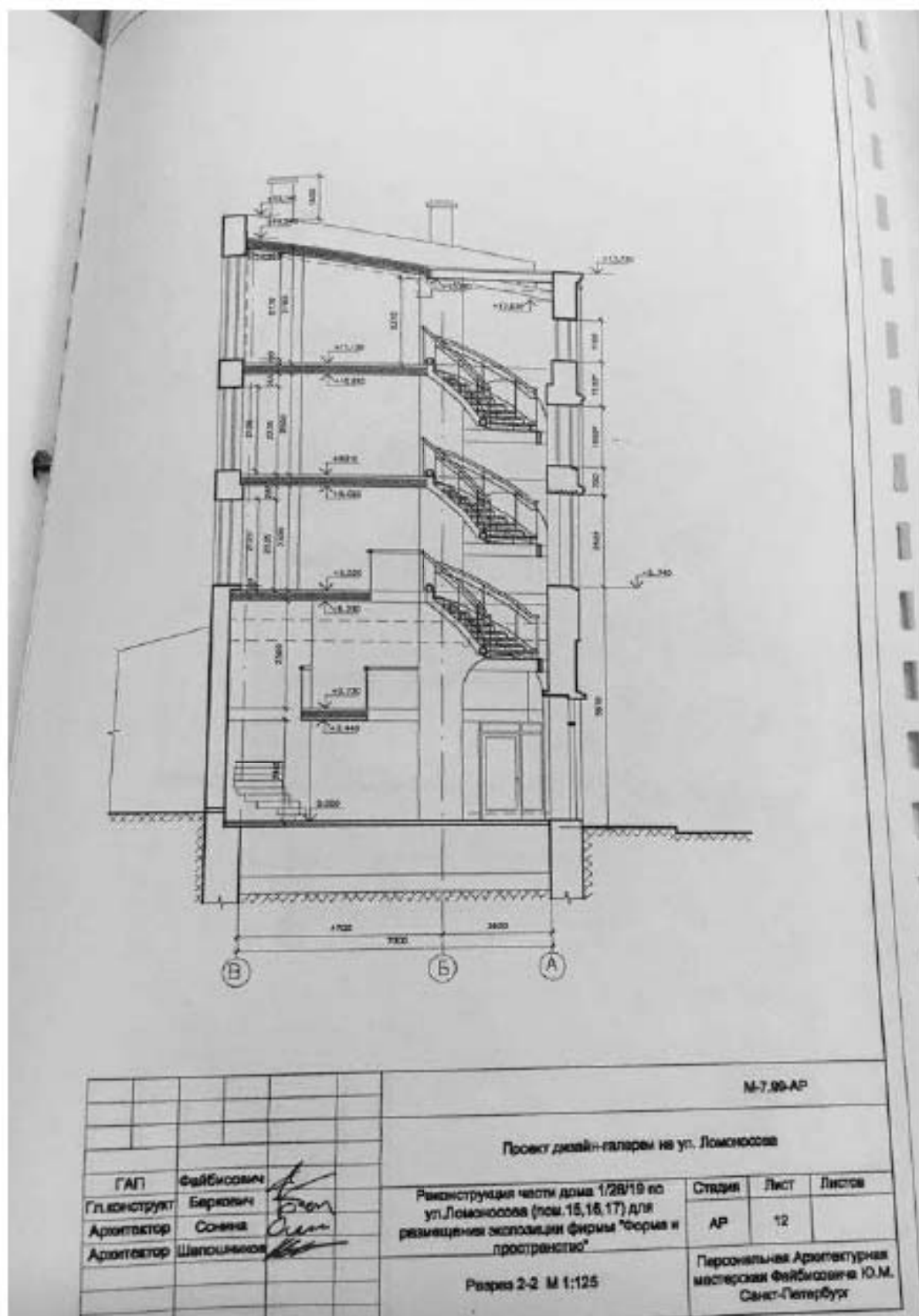
Илл. 140. Рабочий проект реконструкции помещений 15, 15 б, в, г; 16, 16 б, в, г дома 1/28/19 по ул. Ломоносова для размещения экспозиции фирмы «Форма и пространство», разработанный Персональной творческой мастерской Союза архитекторов России Ю. Файбисовича в 2001 г. (нежилые помещения 15-Н, 16-Н, 17-Н, 19-Н). Разрез 2-2 (источник: Архив КГИОП. П. 424-1. Пр-10).
