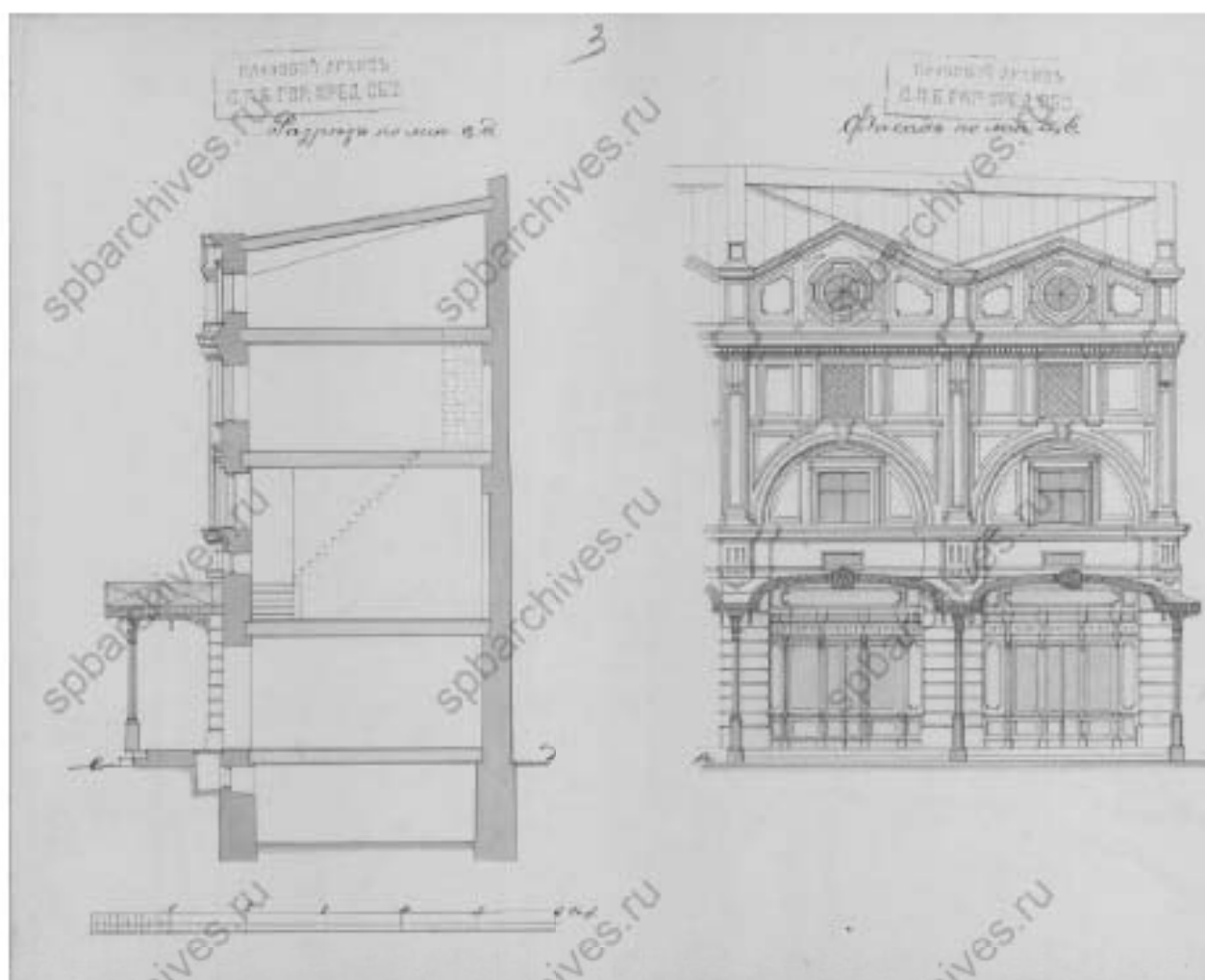
Илл. 91. Разрез и фасад лавки № 35. 6/д. Ориентировочно 1874-1895 гг. (источник: ЦГИА СПб. Ф. 515. Оп. 4. Д. 5794А).
