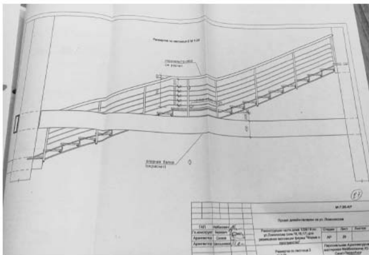
Илл. 147. Рабочий проект реконструкции помещений 15, 15 б, в, г; 16, 16 б, в, г дома 1/28/19 по ул. Ломоносова для размещения экспозиции фирмы «Форма и пространство», разработанный Персональной творческой мастерской Союза архитекторов России Ю. Файбисовича в 2001 г. (нежилые помещения 15-Н, 16-Н, 17-Н, 19-Н). Развертка по лестнице 2 (источник: Архив КГИОП. П. 424-1. Пр-10).
