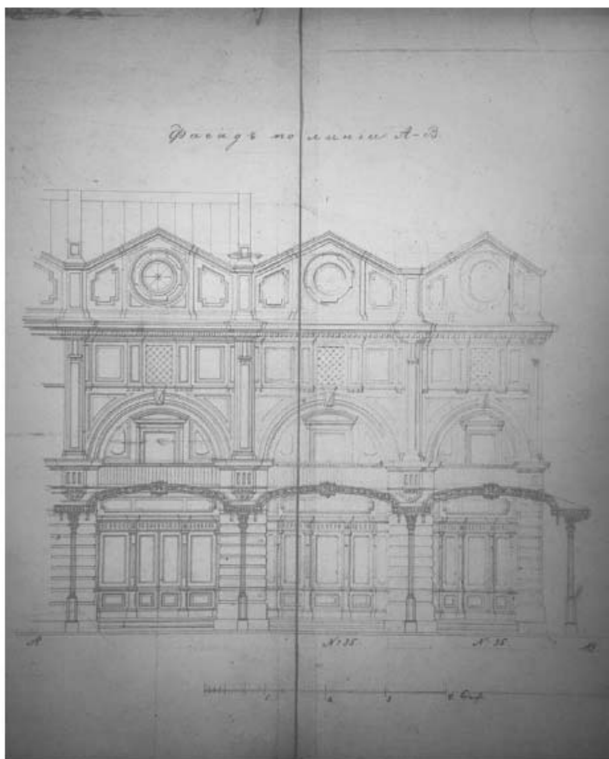
Илл. 89. Фасад лавки № 35 в предполагаемом виде. 1873 г. (источник: ЦГИА СПб. Ф. 513. Оп. 115. Д. 642).
