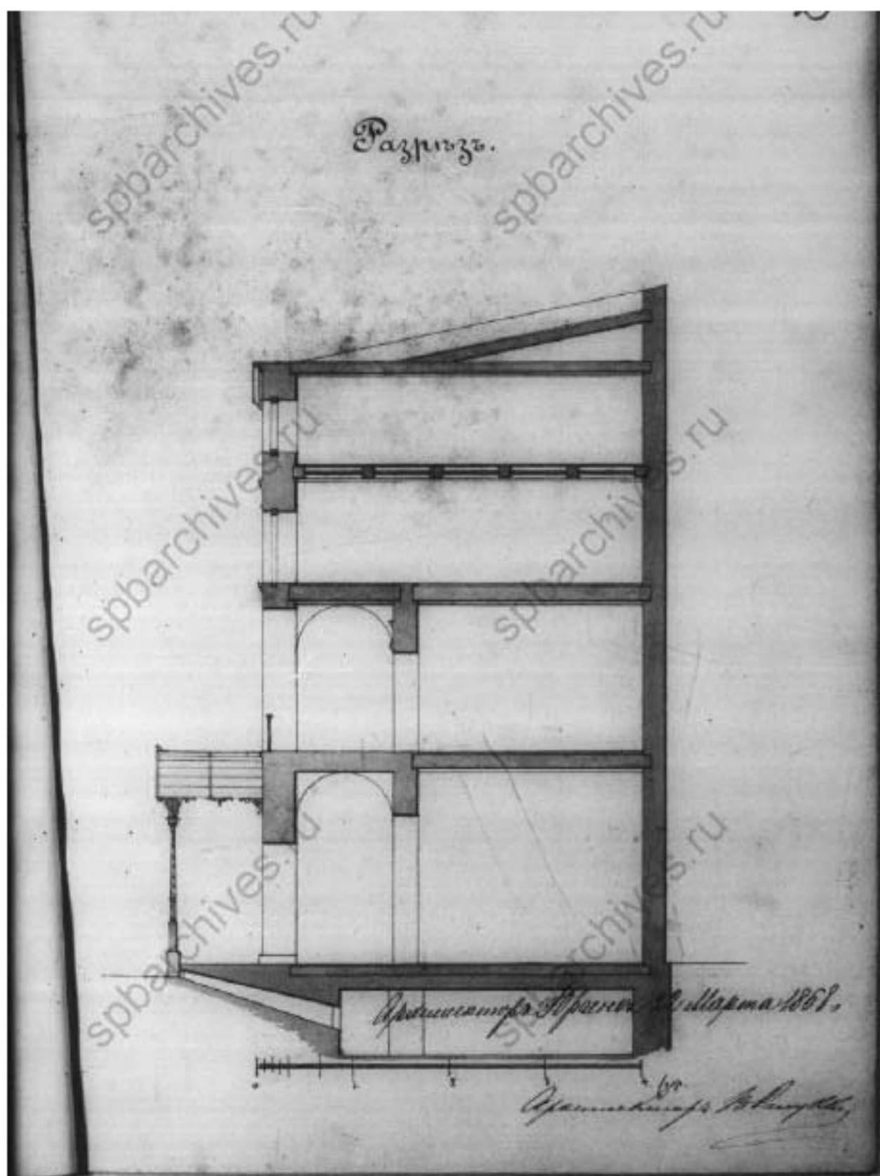
Илл. 84. Разрез лавки № 27. 1868 г. (источник: ЦГИА СПб. Ф. 515. Оп. 4. Д. 127).
