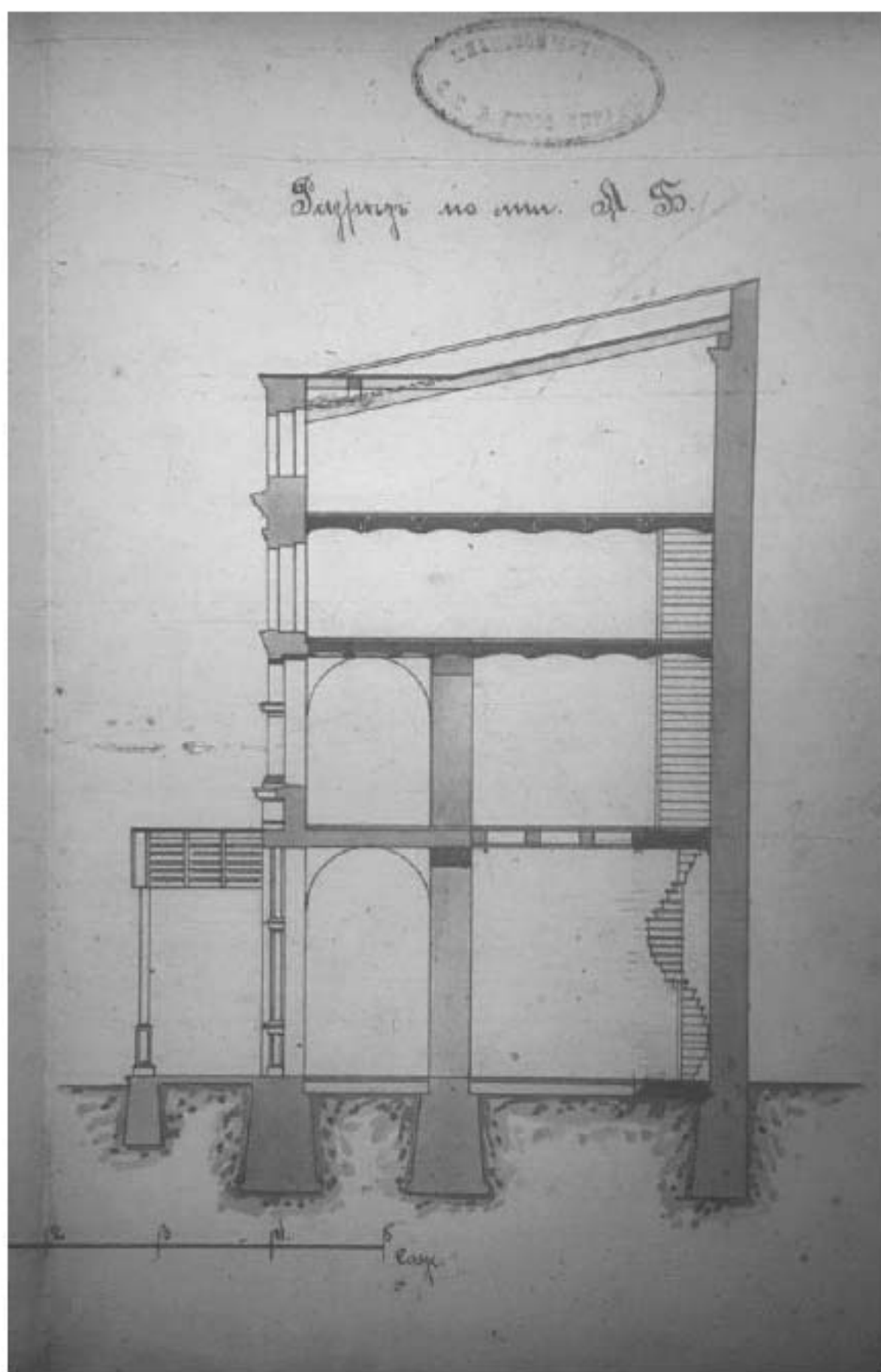
Илл. 53. Разрез лавки № 4 с показанием предполагаемых к проведению работ. 1908 г. (источник: ЦГИА СПб. Ф. 513. Оп. 115. Д. 628).
