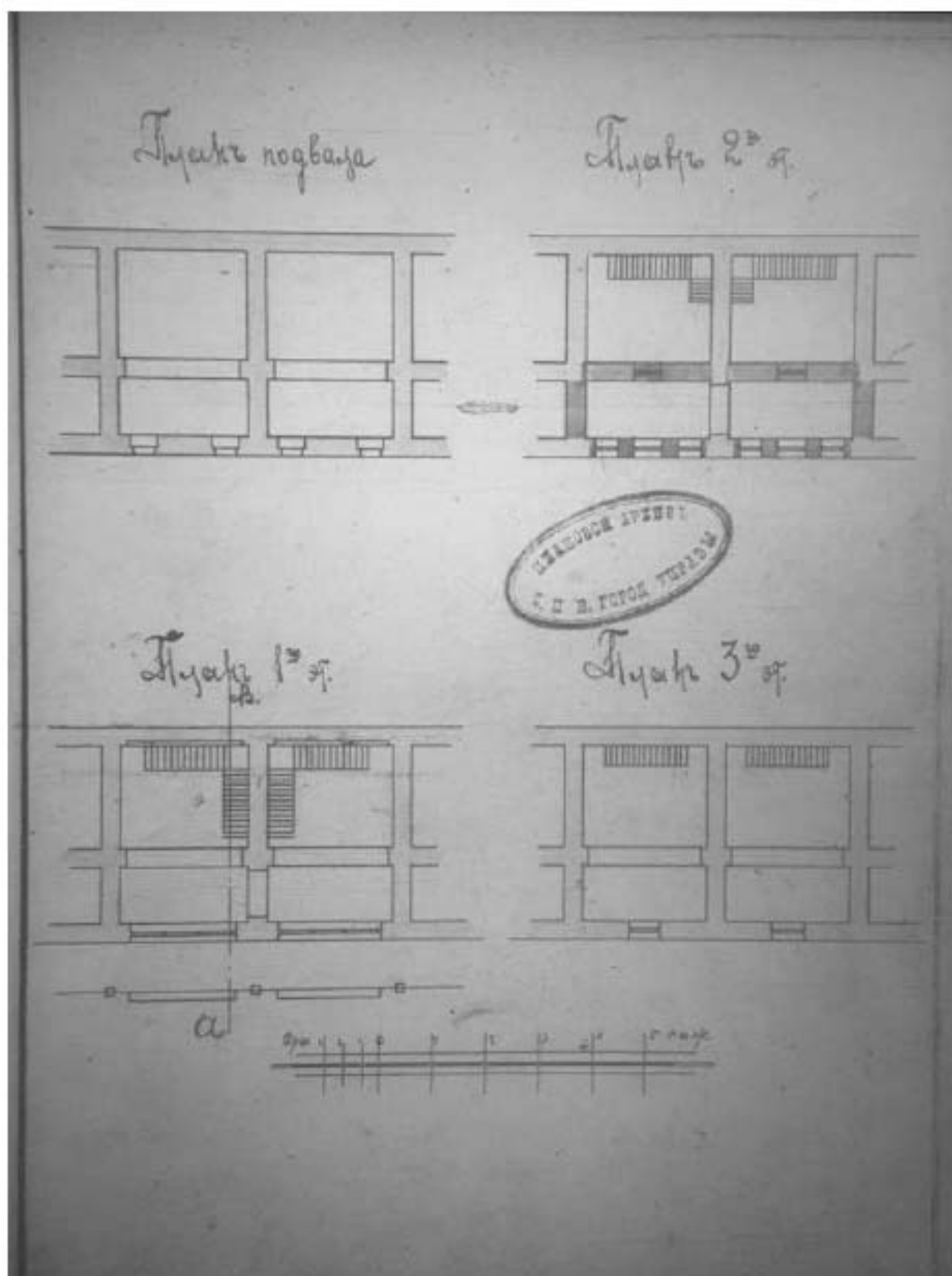
Илл. 67. План лавок № 13 и № 14 с показанием предполагаемых к проведению работ. 1908 г. (источник: ЦГИА СПб. Ф. 513. Оп. 115. Д. 635).
