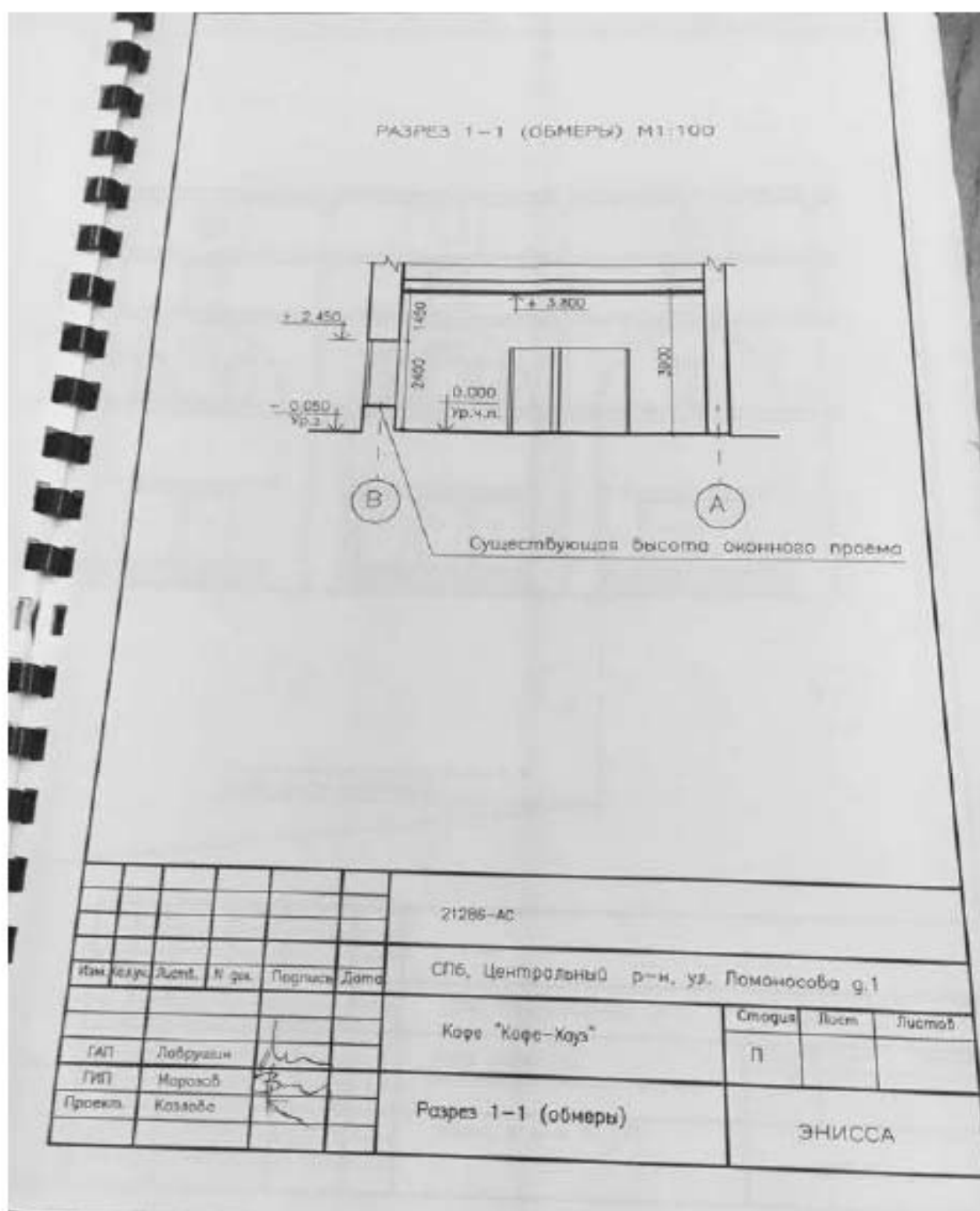
Илл. 149. Проект воссоздания оконных проемов кафе «Кофе Хаус», разработанный ООО «Энисса» в 2004 г. (нежилое помещение 31-Н). Разрез 1-1. (источник: Архив КГИОП. П. 424-1. Пр-9).
