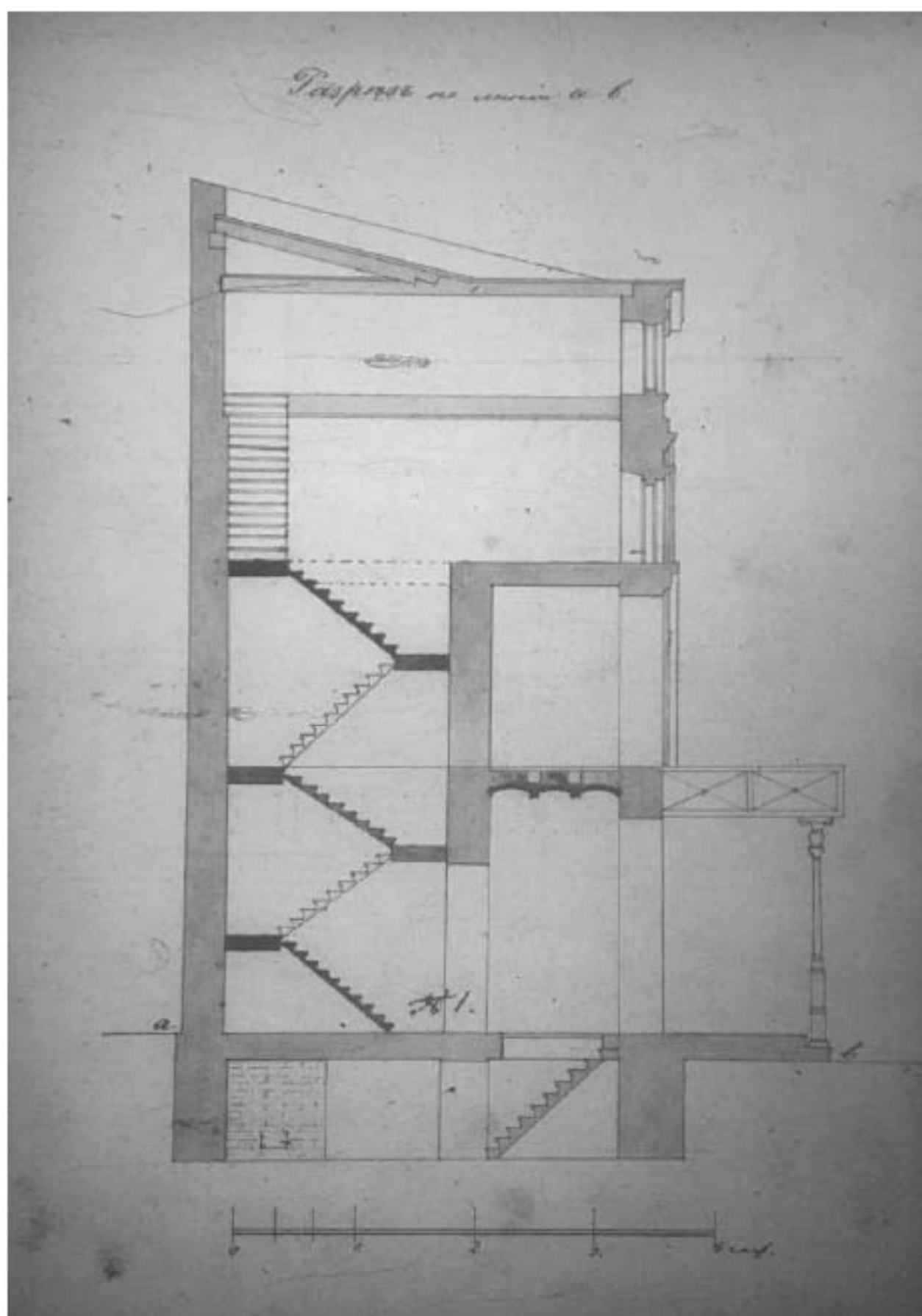
Илл. 43. Разрез лавок № 1 и № 2, принадлежащих СПб 2-й гильдии купцу Ивану Ивановичу Смирнову, с показанием предполагаемых к проведению работ. 1873 г. (источник: ЦГИА СПб. Ф. 513. Оп. 115. Д. 627).
