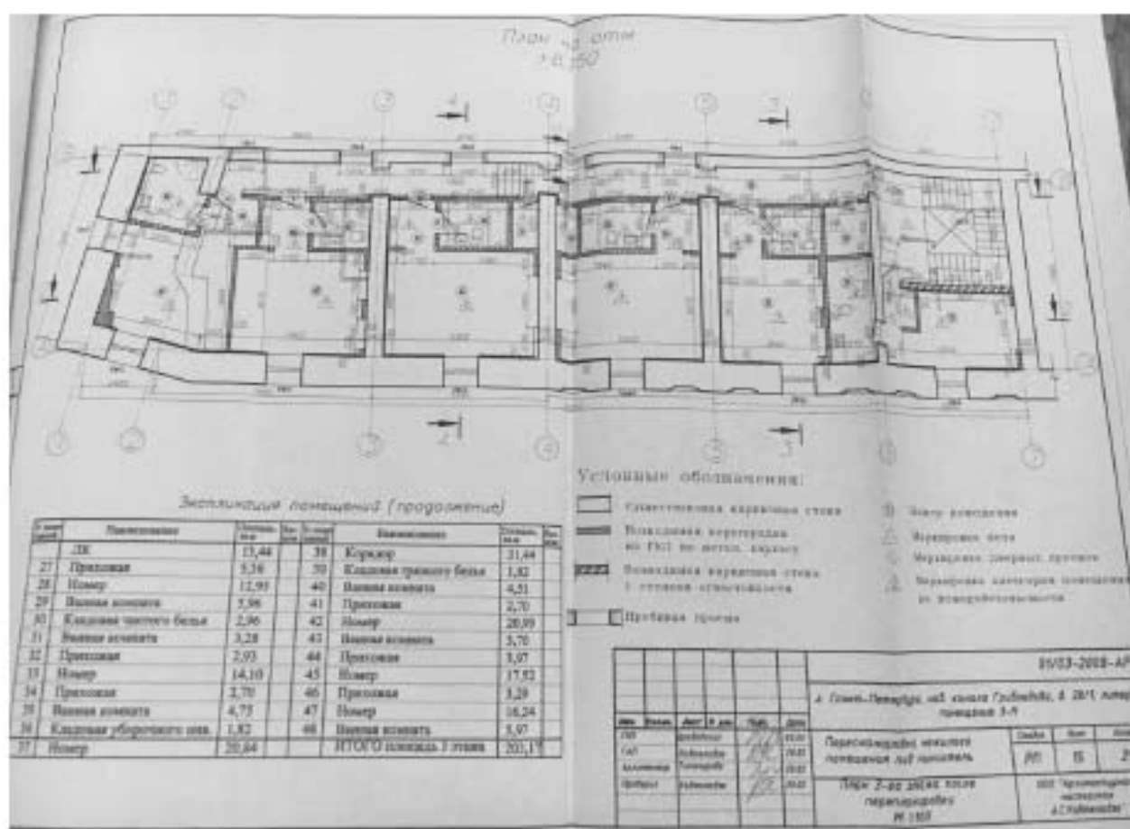
Илл. 108. Рабочий проект перепланировки нежилого помещения под миниотель по адресу: г. Санкт-Петербург, наб. канала Грибоедова, д. 28/1, лит. А, пом. 3-Н, разработанный ООО «Архитектурная мастерская А.С. Кавтеладзе» в 2008 г. (нежилое помещение 3-Н). План 3-го этажа после перепланировки (источник: Архив КГИОП. П. 424-1. Пр-14).
