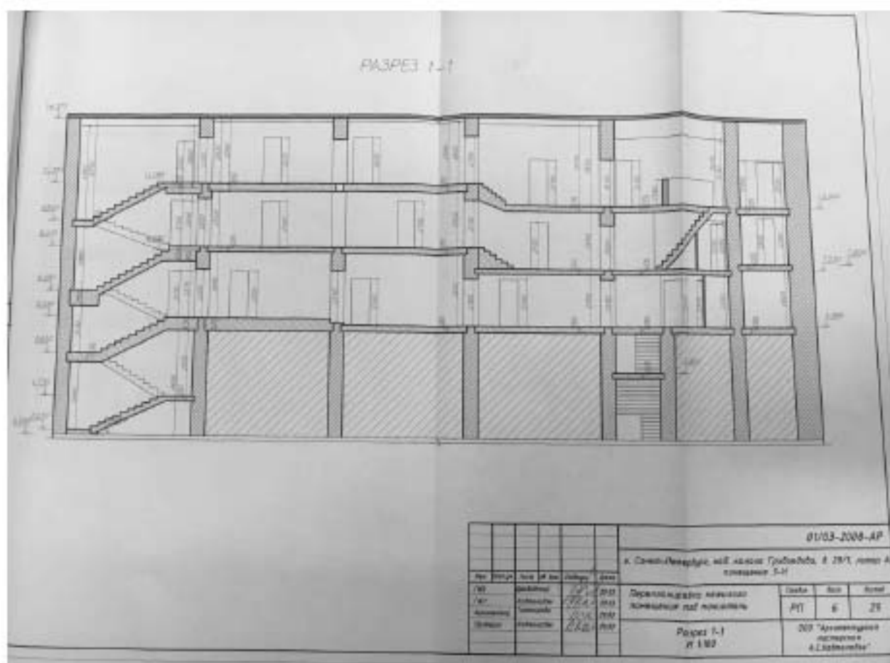
Илл. 99. Рабочий проект перепланировки нежилого помещения под миниотель по адресу: г. Санкт-Петербург, наб. канала Грибоедова, д. 28/1, лит. А, пом. 3-Н, разработанный ООО «Архитектурная мастерская А.С. Кавталадзе» в 2008 г. (нежилое помещение 3-Н). Разрез 1-1 (источник: Архив КГИОП. П. 424-1. Пр-14).
