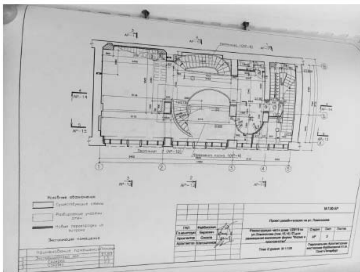
Илл. 133. Рабочий проект реконструкции помещений 15, 15 б, в, г; 16, 16 б, в, г дома 1/28/19 по ул. Ломоносова для размещения экспозиции фирмы «Форма и пространство», разработанный Персональной творческой мастерской Союза архитекторов России Ю. Файбисовича в 2001 г. (нежилые помещения 15-Н, 16-Н, 17-Н, 19-Н). План 2-го уровня (источник: Архив КГИОП. П. 424-1. Пр-10).
