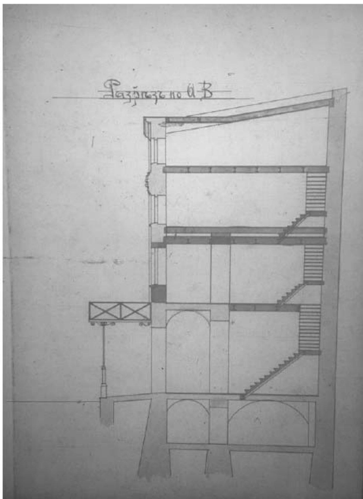
Илл. 64. Разрез лавки № 12 с показанием предполагаемых к проведению работ. 1908 г. (источник: ЦГИА СПб. Ф. 513. Оп. 115. Д. 634).
