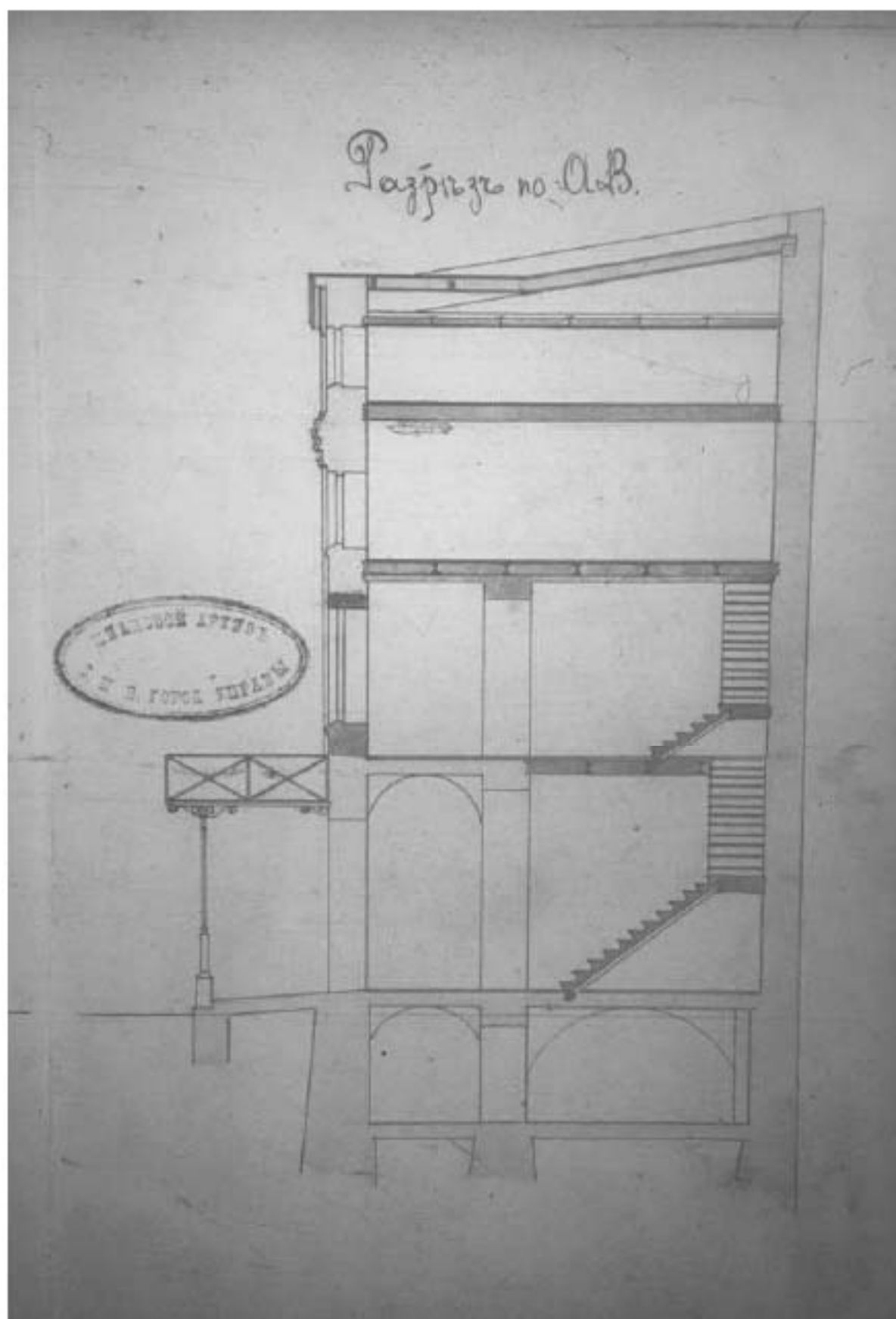
Илл. 69. Разрез лавок № 13 и № 14 с показанием предполагаемых к проведению работ. 1908 г. (источник: ЦГИА СПб. Ф. 513. Оп. 115. Д. 635).
