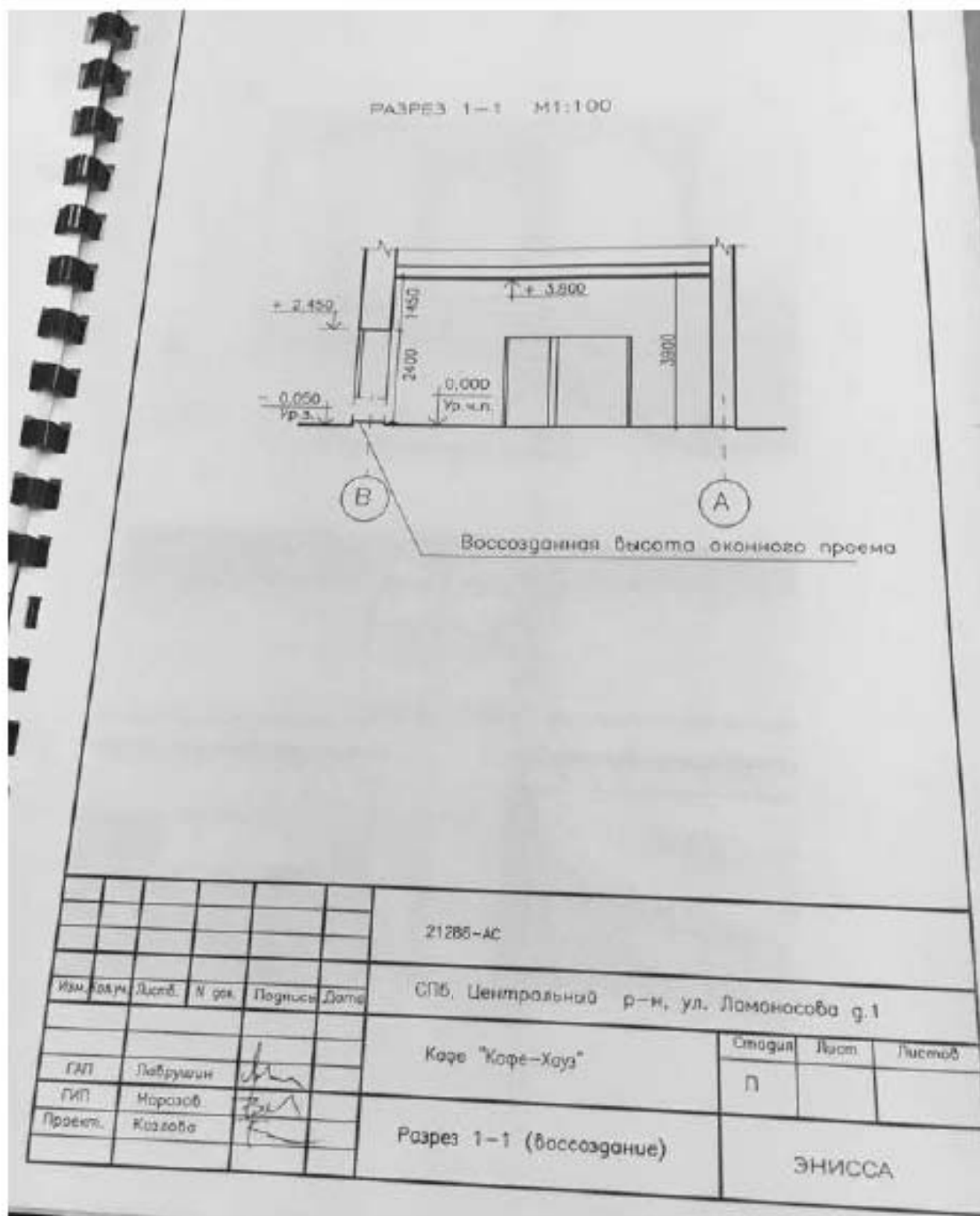
Илл. 151. Проект воссоздания оконных проемов кафе «Кофе Хаус», разработанный ООО «Энисса» в 2004 г. (нежилое помещение 31-Н). Разрез 1-1 воссоздание (источник: Архив КГИОП. П. 424-1. Пр-9).
