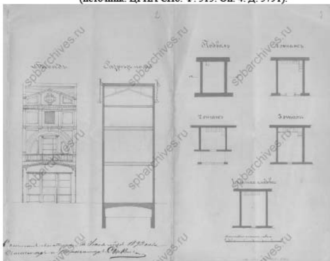
Илл. 71. Фасад, разрез и планы лавки № 15, принадлежащей СПБ купцу Дойникову. 1892 г. (источник: ЦГИА СПб. Ф. 515. Оп. 4. Д. 5791).
