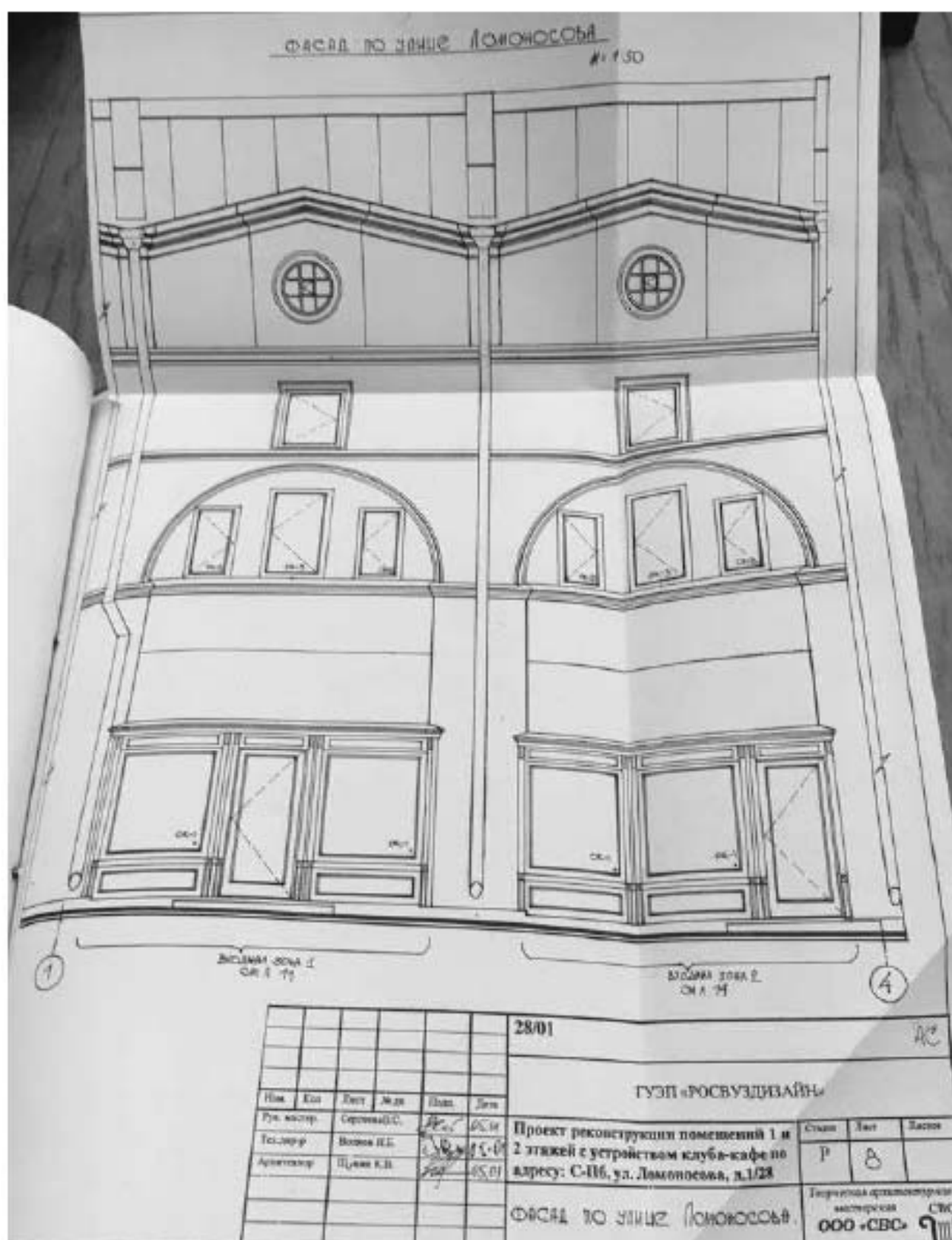
Илл. 167. Проект реконструкции помещений 1 и 2 этажей с устройством клуба-кафе по адресу: С-Пб, ул. Ломоносова, д. 1/28, разработанный ООО «СВС» в 2001 г. (нежилое помещение 16-Н). Фасад по улице Ломоносова (источник: Архив КГИОП. П. 424-1. Пр-2).
