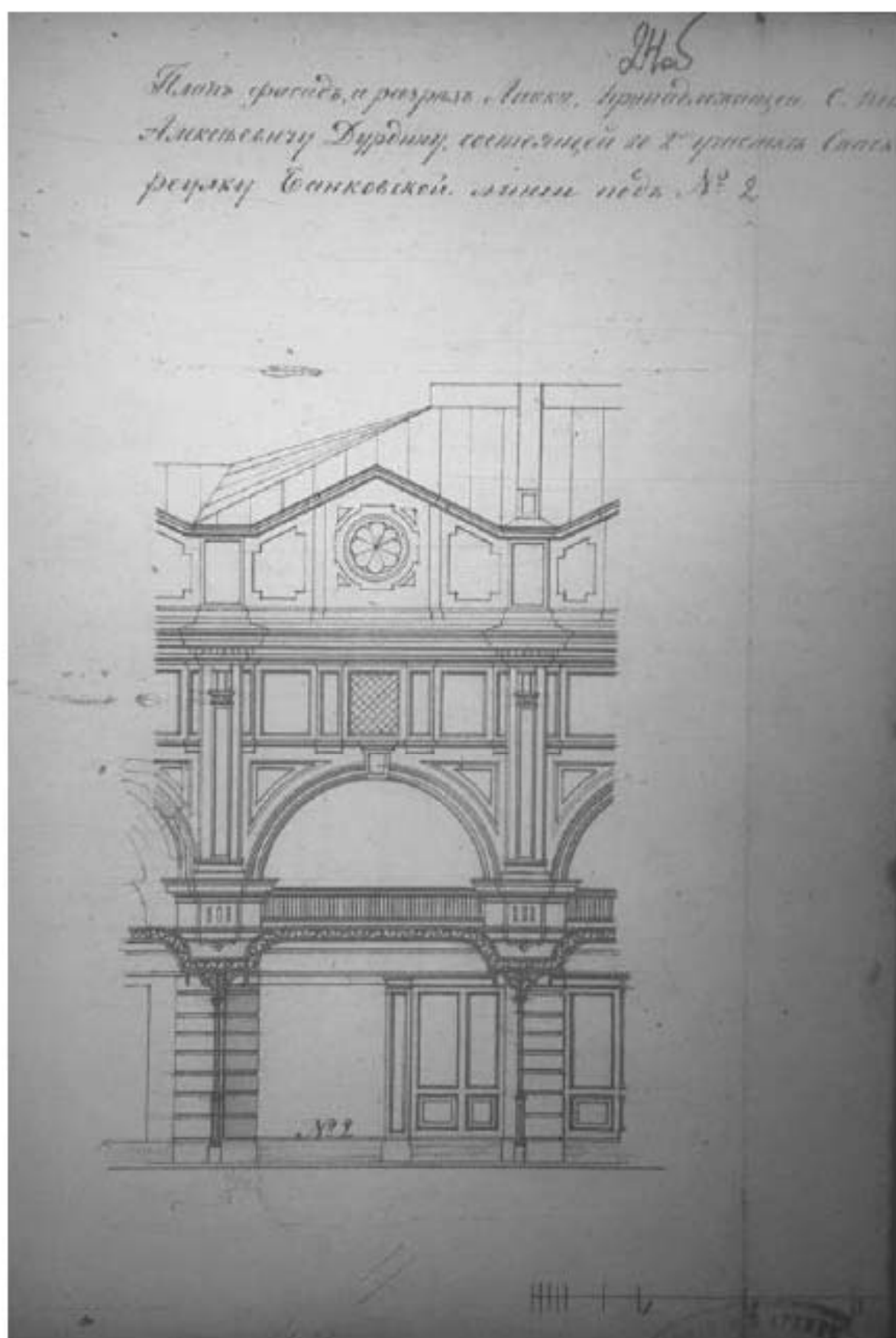
Илл. 44. Фасад лавки № 2, принадлежащей С-Петербургскому купцу Александру Алексеевичу Дурдину, в предполагаемом виде. 1889 г. (источник: ЦГИА СПб. Ф. 513. Оп. 115. Д. 627).
