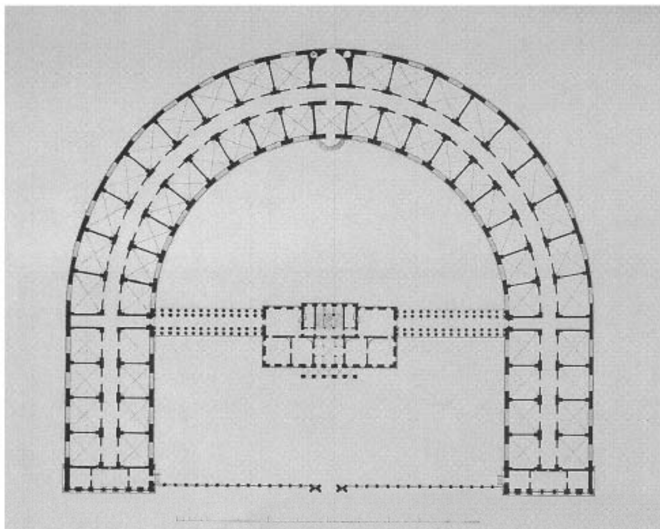
4. План первого этажа.
