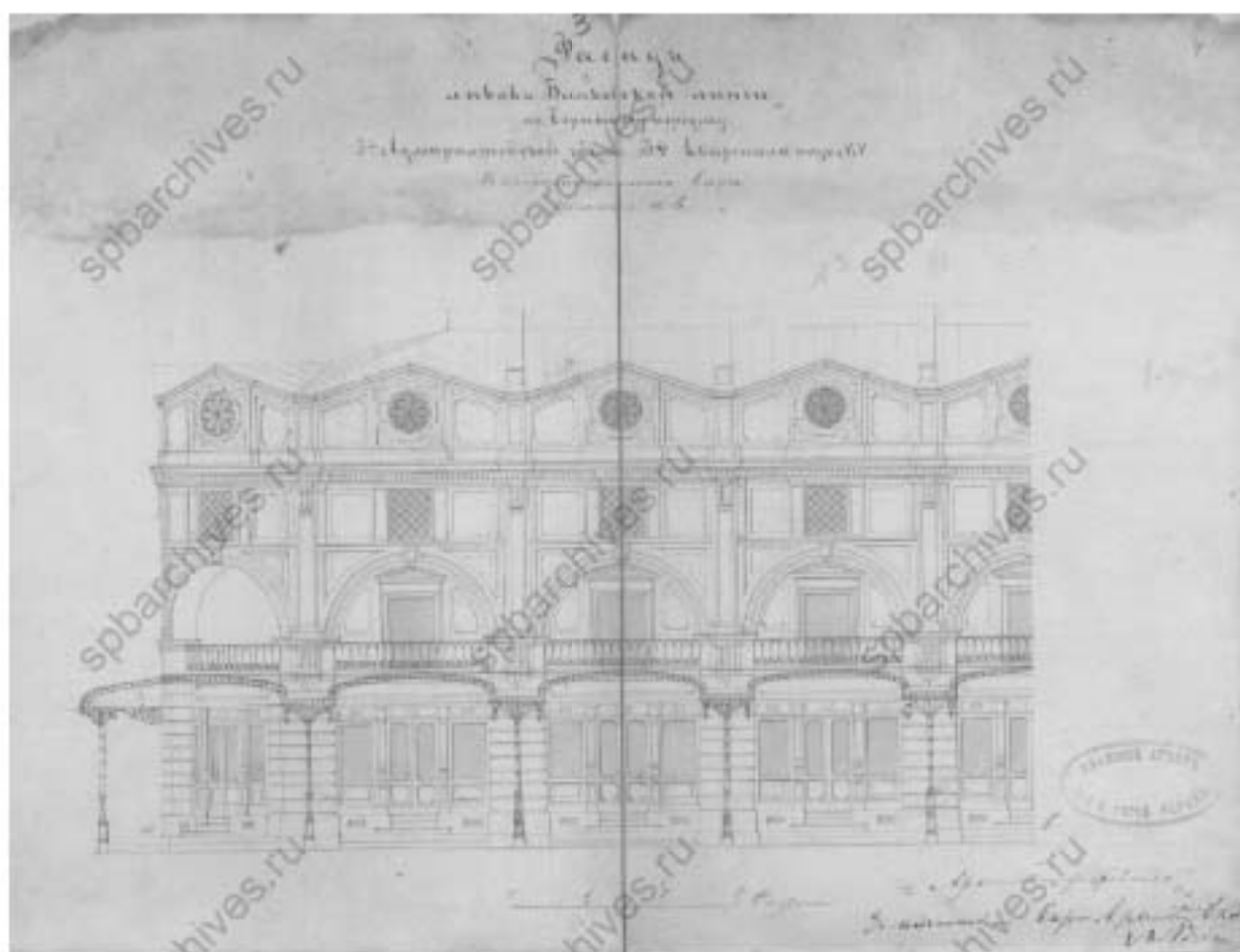
Илл. 25. Фасад лавок в предполагаемом виде. 1861 г. (источник: ЦГИА СПб. Ф. 513. Оп. 115. Д. 700).
