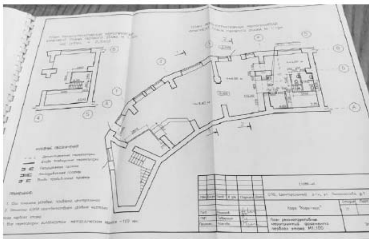
Илл. 154. Документация: «Кафе «Кофе Хаус». Общая пояснительная записка. Архитектурно-строительные решения», разработанная ООО «Энисса-2001» в 2004 г. (нежилое помещение 31-Н). План реконструктивных мероприятий фрагмента первого этажа (источник: Архив КГИОП. П. 424-1. Пр-8).
