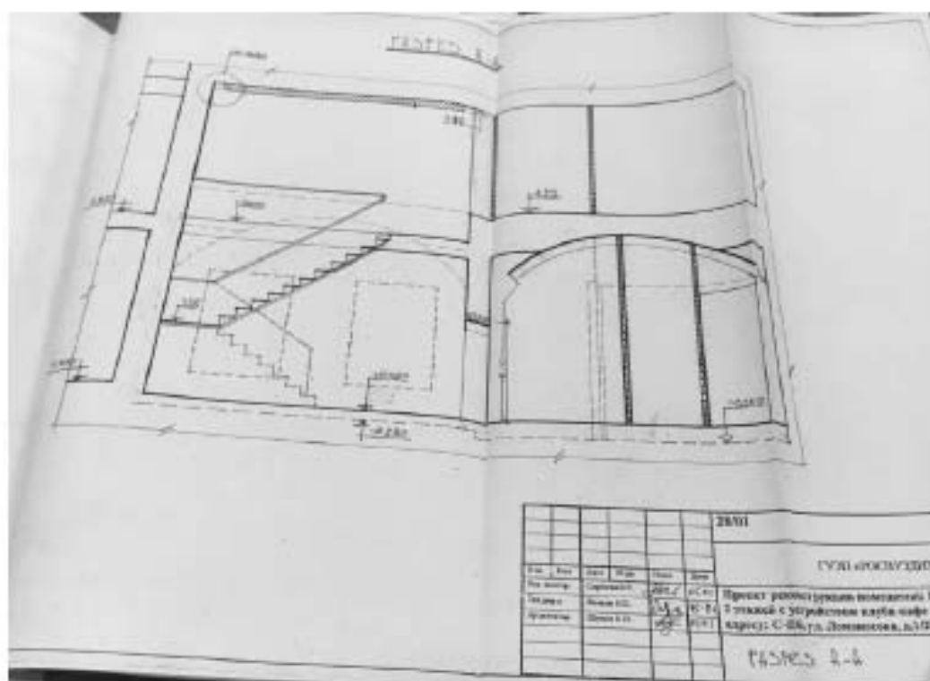
Илл. 168. Проект реконструкции помещений 1 и 2 этажей с устройством клуба-кафе по адресу: С-Пб, ул. Ломоносова, д. 1/28, разработанный ООО «СВС» в 2001 г. (нежилое помещение 16-Н). Разрез А-А (источник: Архив КГИОП. П. 424-1. Пр-2).
