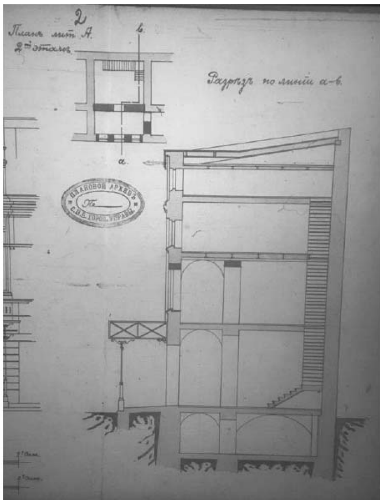
Илл. 76. План и разрез лавки № 15 с показанием предполагаемых к проведению работ 1914 г. (источник: ЦГИА СПб. Ф. 513. Оп. 115. Д. 636).
