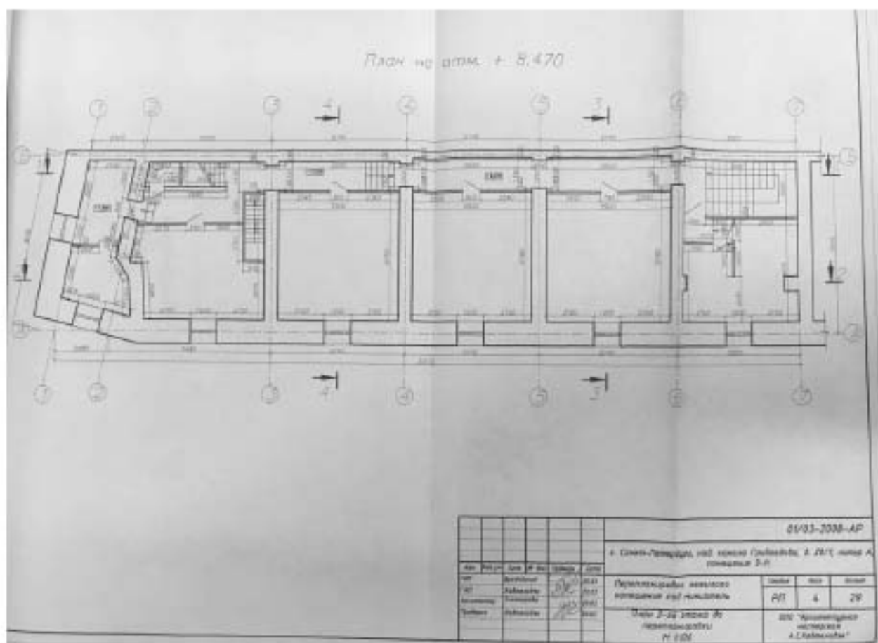
Илл. 97. Рабочий проект перепланировки нежилого помещения под миниотель по адресу: г. Санкт-Петербург, наб. канала Грибоедова, д. 28/1, лит. А, пом. 3-Н, разработанный ООО «Архитектурная мастерская А.С. Кавтеладзе» в 2008 г. (нежилое помещение 3-Н). План 3-го этажа до перепланировки (источник: Архив КГИОП. П. 424-1. Пр-14).
