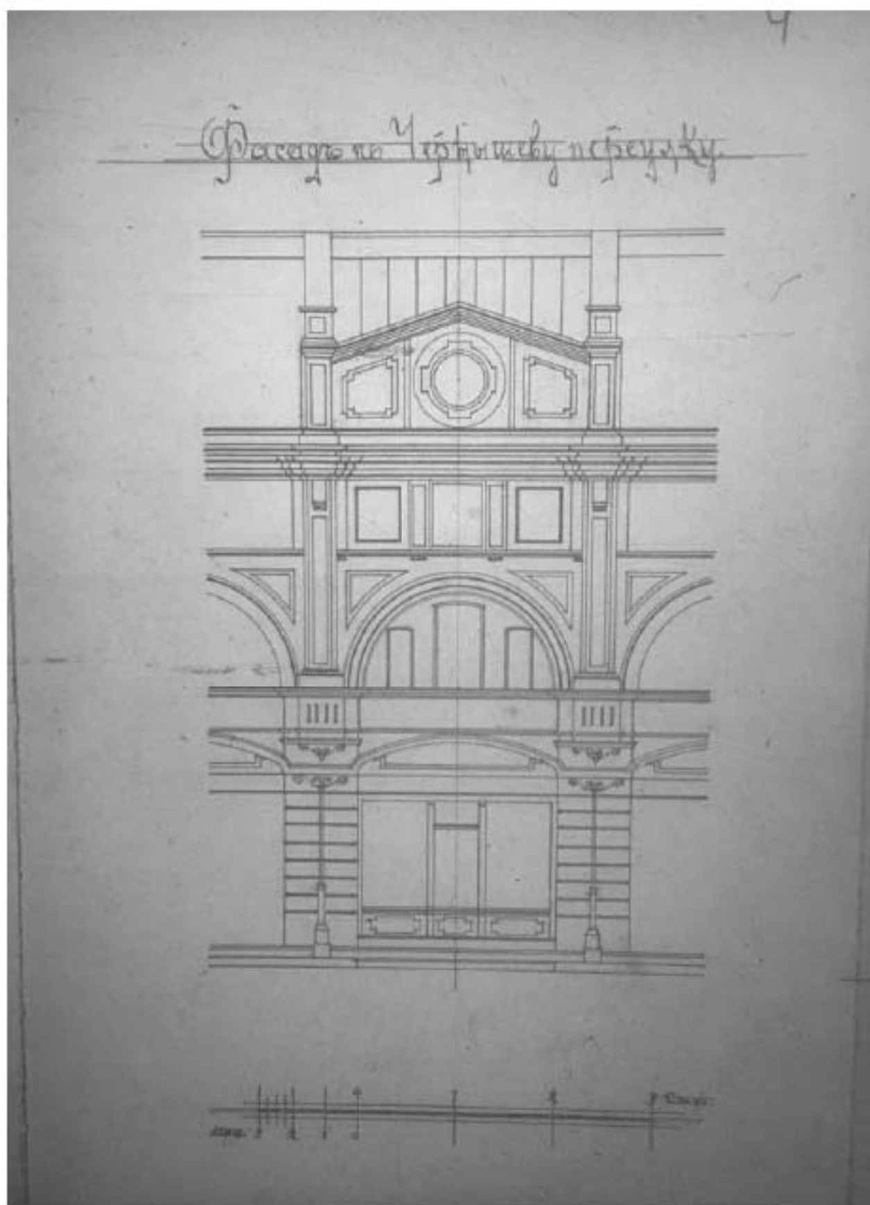
Илл. 63. Фасад лавки № 12 в предполагаемом виде. 1908 г. (источник: ЦГИА СПб. Ф. 513. Оп. 115. Д. 634)
