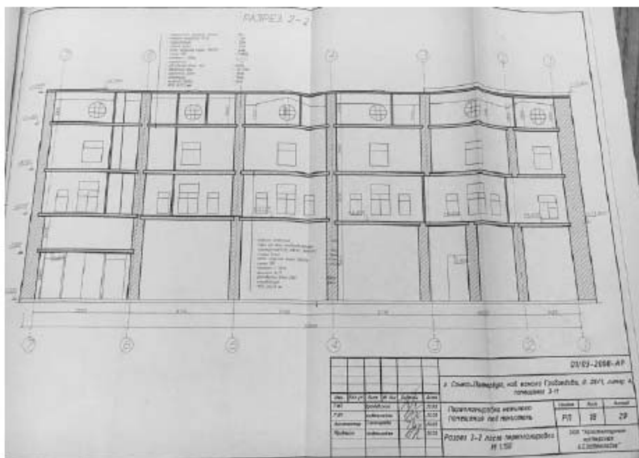
Илл. 111. Рабочий проект перепланировки нежилого помещения под миниотель по адресу: г. Санкт-Петербург, наб. канала Грибоедова, д. 28/1, лит. А, пом. 3-Н, разработанный ООО «Архитектурная мастерская А.С. Кавталадзе» в 2008 г. (нежилое помещение 3-Н). Разрез 2-2 после перепланировки (источник: Архив КГИОП. П. 424-1. Пр-14).
