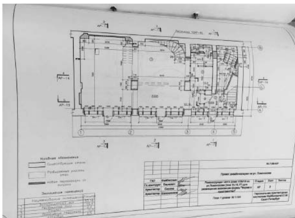
Илл. 132. Рабочий проект реконструкции помещений 15, 15 б, в, г; 16, 16 б, в, г дома 1/28/19 по ул. Ломоносова для размещения экспозиции фирмы «Форма и пространство», разработанный Персональной творческой мастерской Союза архитекторов России Ю. Файбисовича в 2001 г. (нежилые помещения 15-Н, 16-Н, 17-Н, 19-Н). План 1-го уровня (источник: Архив КГИОП. П. 424-1. Пр-10).
