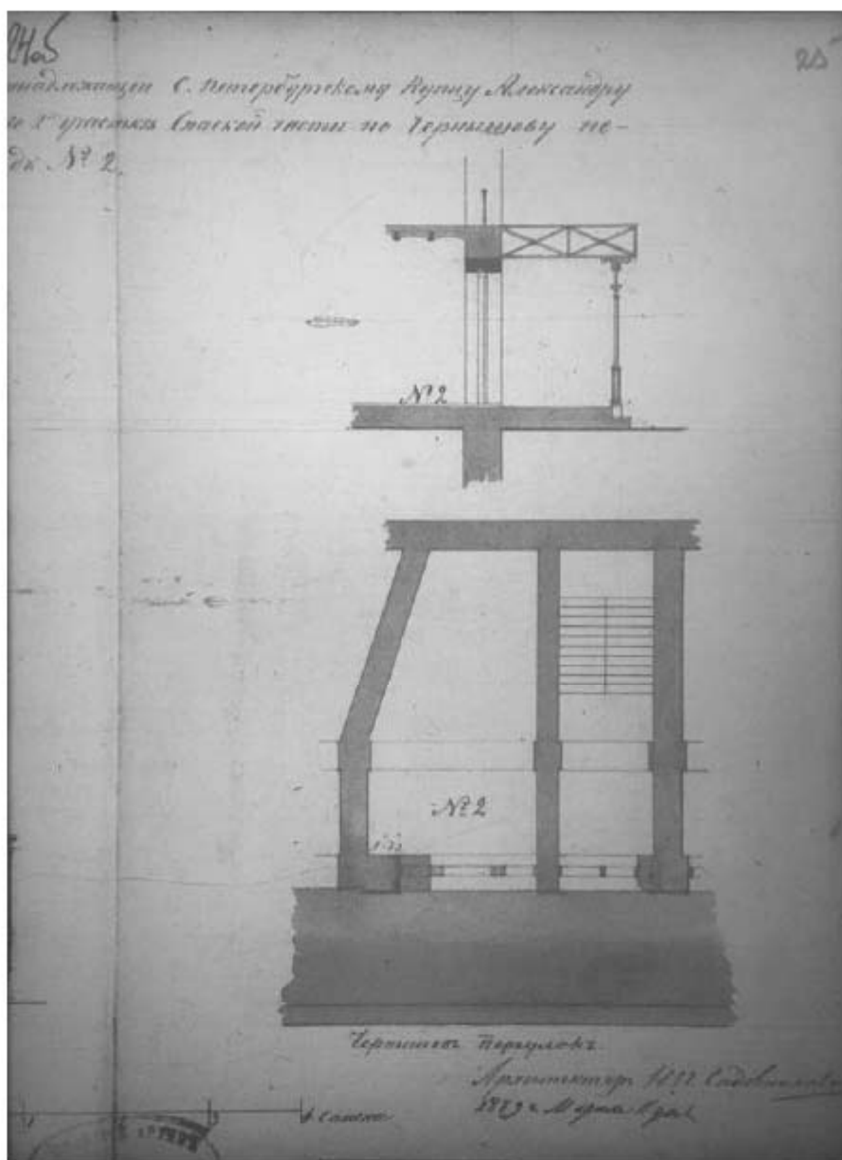
Илл. 45. План и разрез лавки № 2, принадлежащей С-Петербургскому купцу Александру Алексеевичу Дурдину, с указанием предполагаемых к проведению работ. 1889 г. (источник: ЦГИА СПб. Ф. 513. Оп. 115. Д. 627).
