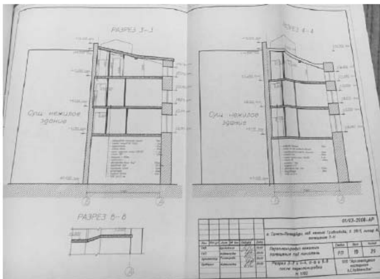
Илл. 112. Рабочий проект перепланировки нежилого помещения под миниотель по адресу: г. Санкт-Петербург, наб. канала Грибоедова, д. 28/1, лит. А, пом. 3-Н, разработанный ООО «Архитектурная мастерская А.С. Кавтеладзе» в 2008 г. (нежилое помещение 3-Н). Разрез 3-3 и 4-4 после перепланировки (источник: Архив КГИОП. П. 424-1. Пр-14).
