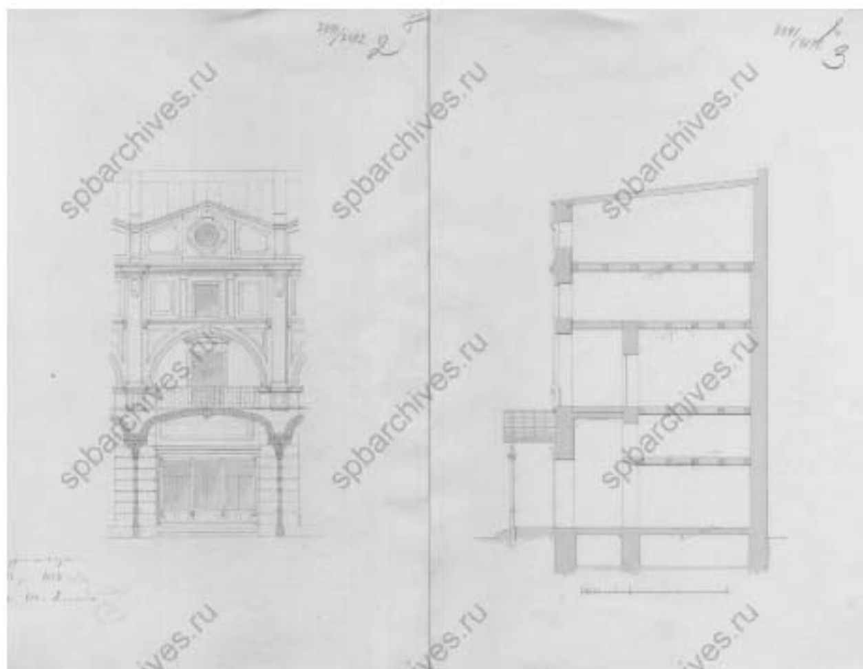
Илл. 59. Фасад и разрез лавки № 10 Николая Васильевича Набилкова. 1874 г. (источник: ЦГИА СПб. Ф. 515. Оп. 4. Д. 5792).
