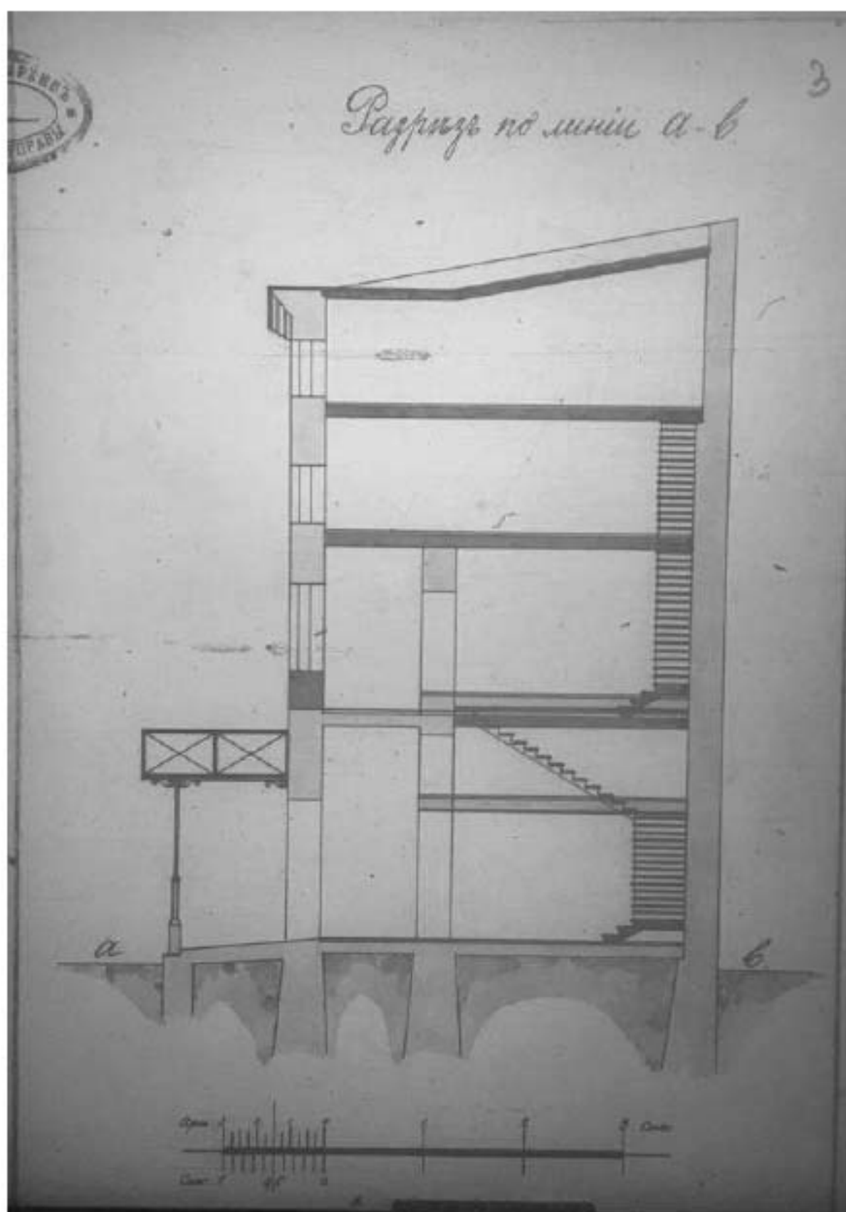
Илл. 81. Разрез лавки № 19 с показанием предполагаемых к проведению работ. 1911 г. (источник: ЦГИА СПб. Ф. 513. Оп. 115. Д. 637).
