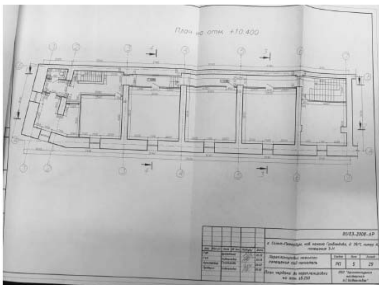
Илл. 98. Рабочий проект перепланировки нежилого помещения под миниготель по адресу: г. Санкт-Петербург, наб. канала Грибоедова, д. 28/1, лит. А, пом. 3-Н, разработанный ООО «Архитектурная мастерская А.С. Кавталадзе» в 2008 г. (нежилое помещение 3-Н). План чердака до перепланировки (источник: Архив КГИОП. П. 424-1. Пр-14).
