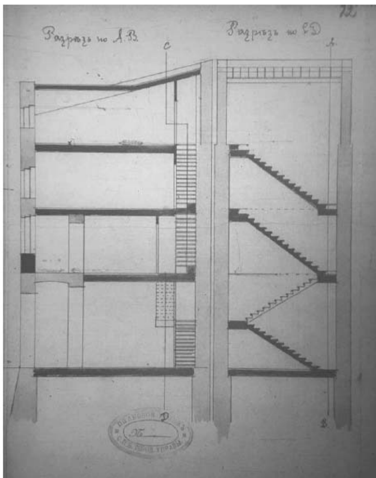
Илл. 47. Разрезы лавки № 3, принадлежащей В.В. Залеману, с показанием предполагаемых к проведению работ. 1909 г. (источник: ЦГИА СПб. Ф. 513. Оп. 115. Д. 627).
