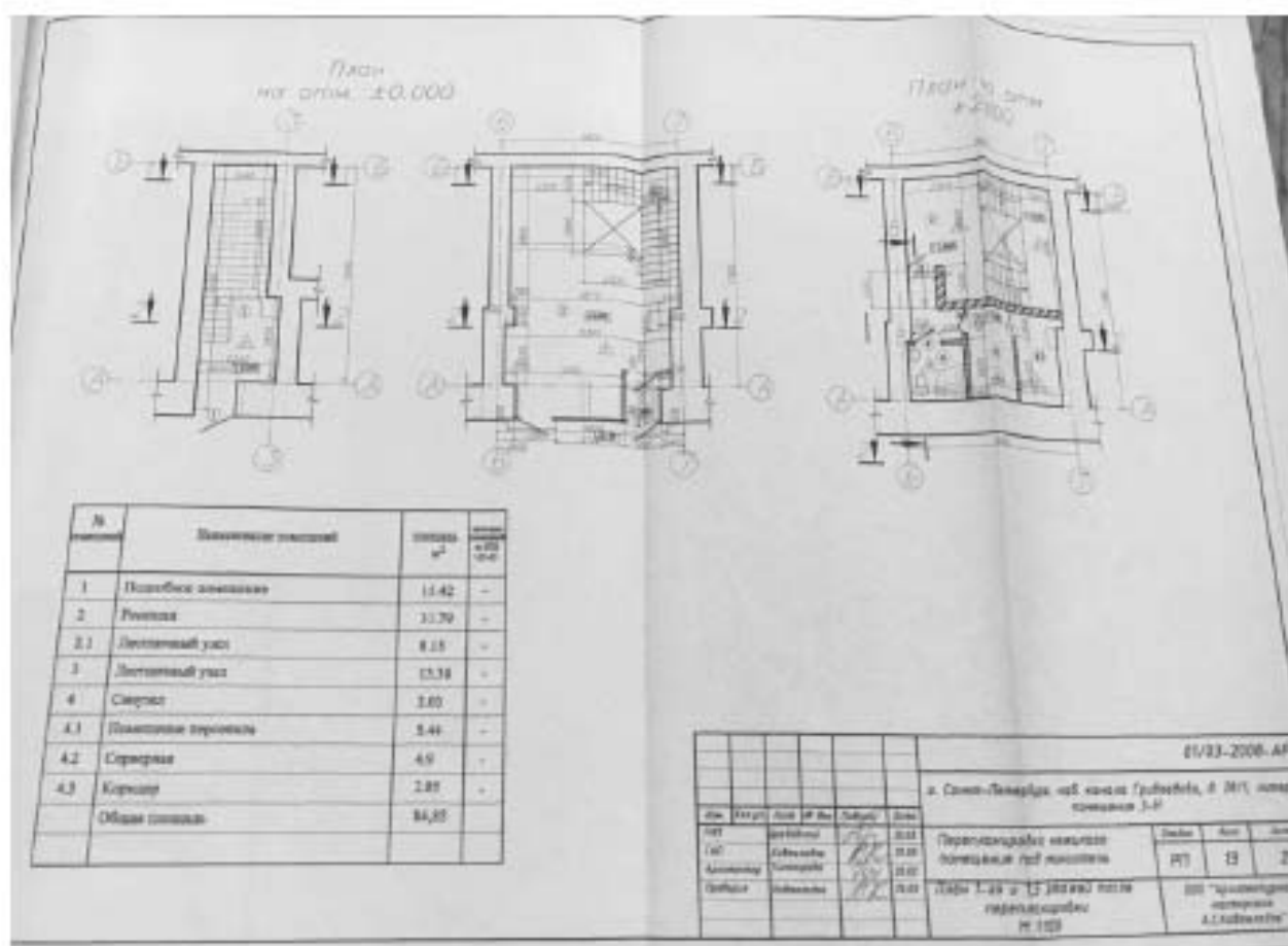
Илл. 106. Рабочий проект перепланировки нежилого помещения под миниотель по адресу: г. Санкт-Петербург, наб. канала Грибоедова, д. 28/1, лит. А, пом. 3-Н, разработанный ООО «Архитектурная мастерская А.С. Кавтеладзе» в 2008 г. (нежилое помещение 3-Н). План 1-го и 1,5-го этажей после перепланировки (источник: Архив КГИОП. П. 424-1. Пр-14).
