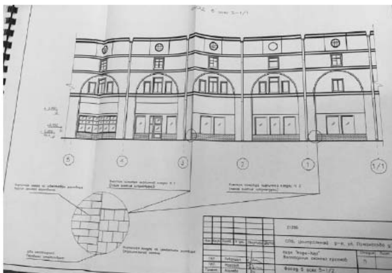
Илл. 150. Проект восстановления оконных проемов кафе «Кофе Хаус», разработанный ООО «Энниса» в 2004 г. (нежилое помещение 31-Н). Фасад. (источник: Архив КГИОП. П. 424-1. Пр-9).
