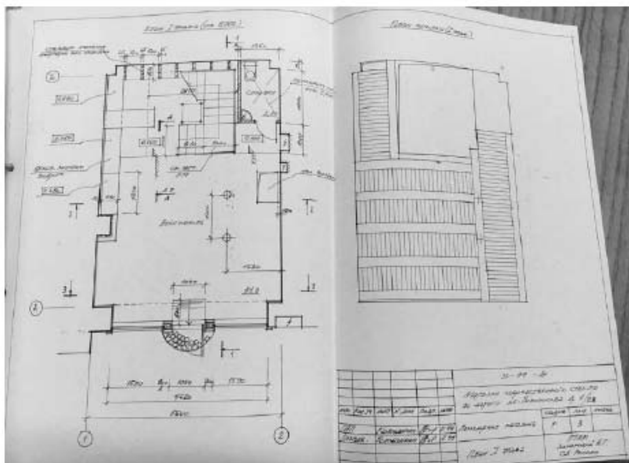
Илл. 118. Проект ремонта и перепланировки части помещений магазина художественного стекла по адресу: ул. Ломоносова, дом 1/28, пом. 21-Н, разработанный Персональной творческой архитектурной мастерской под руководством Захаровой Н.Г. в 1999 г. (нежилое помещение 61-Н). План 1-го этажа (источник: Архив КГИОП. П. 424-1. Пр-13).
