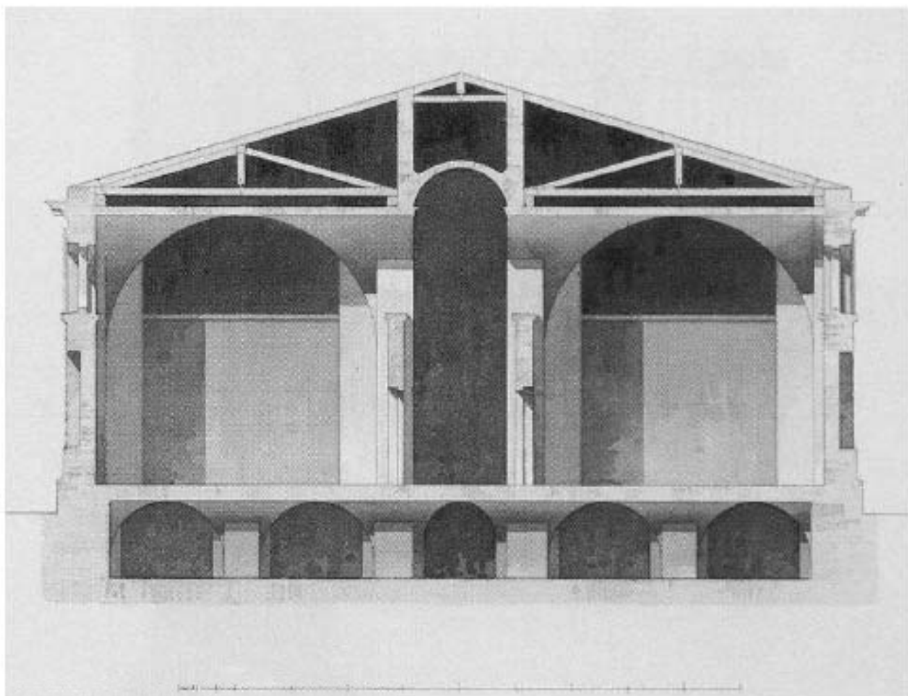
11. Поперечный разрез здания кладовых.
