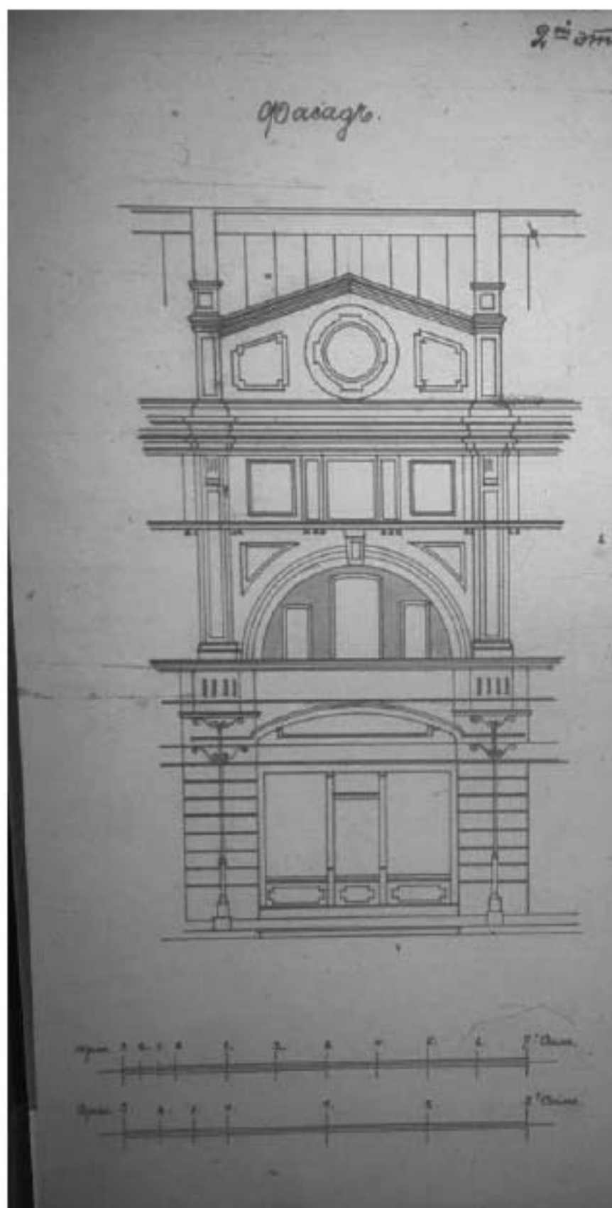
Илл. 75. Фасад лавки № 15 в предполагаемом виде. 1914 г. (источник: ЦГИА СПб. Ф. 513. Оп. 115. Д. 636).
