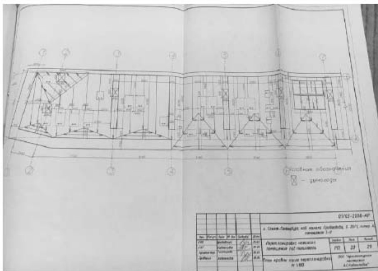
Илл. 113. Рабочий проект перепланировки нежилого помещения под миниотель по адресу: г. Санкт-Петербург, наб. канала Грибоедова, д. 28/1, лит. А, пом. 3-Н, разработанный ООО «Архитектурная мастерская А.С. Кавтеладзе» в 2008 г. (нежилое помещение 3-Н). План кровли после перепланировки (источник: Архив КГИОП. П. 424-1. Пр-14).
