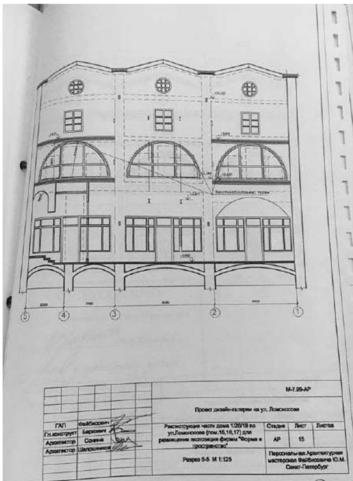
Илл. 143. Рабочий проект реконструкции помещений 15, 15 б, в, г; 16, 16 б, в, г дома 1/28/19 по ул. Ломоносова для размещения экспозиции фирмы «Форма и пространство», разработанный Персональной творческой мастерской Союза архитекторов России Ю. Файбисовича в 2001 г. (нежилые помещения 15-Н, 16-Н, 17-Н, 19-Н). Разрез 5-5 (источник: Архив КГИОП. П. 424-1. Пр-10).
