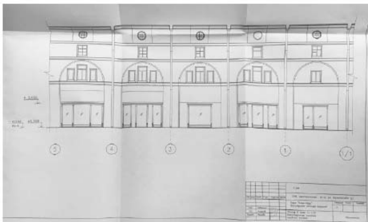
Илл. 152. Проект воссоздания оконных проемов кафе «Кофе Хаус», разработанный ООО «Энисса» в 2004 г. (нежилое помещение 31-Н). Воссозданные проемы первого этажа (источник: Архив КГИОП. П. 424-1. Пр-9).
