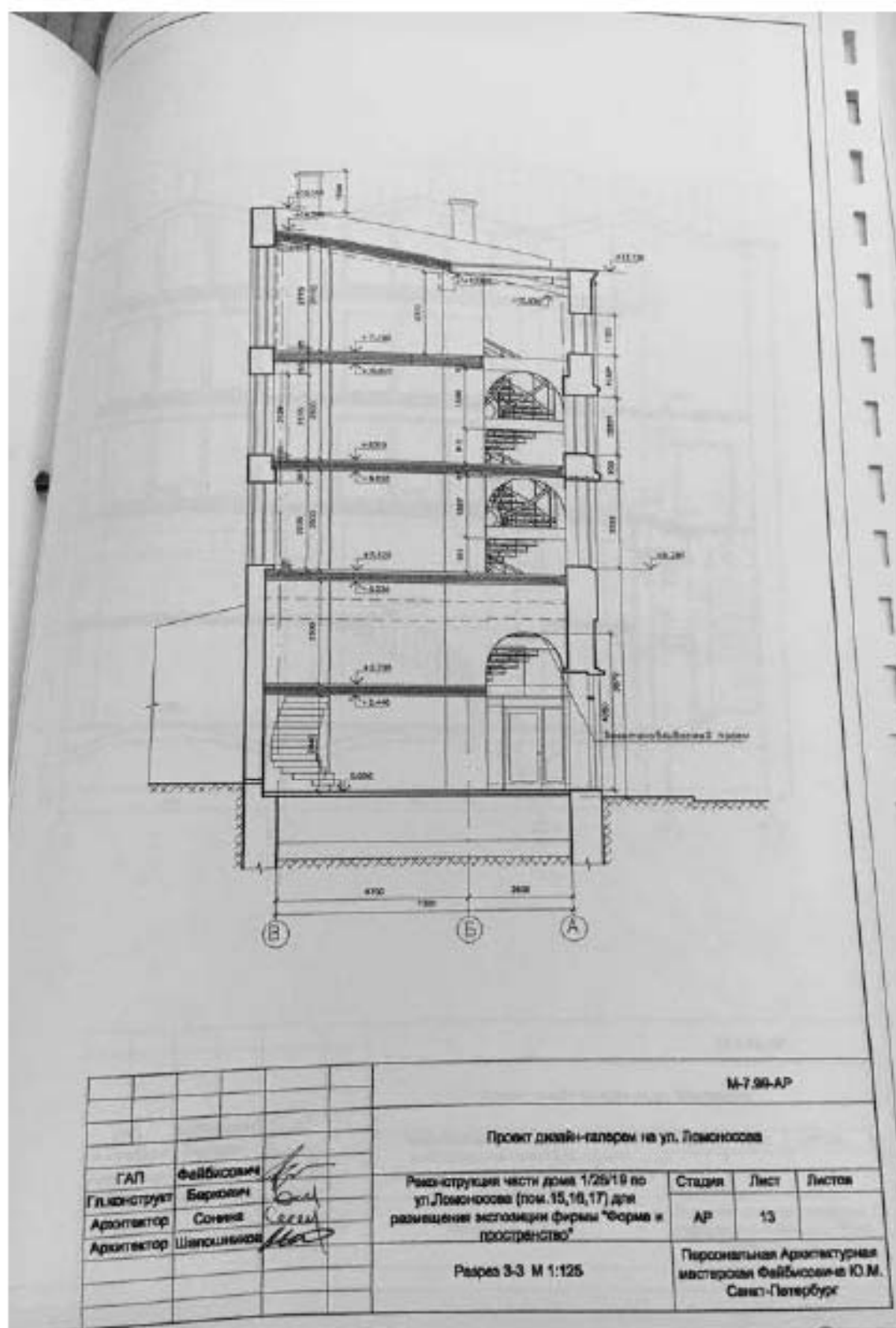
Илл. 141. Рабочий проект реконструкции помещений 15, 15 б, в, г; 16, 16 б, в, г дома 1/28/19 по ул. Ломоносова для размещения экспозиции фирмы «Форма и пространство», разработанный Персональной творческой мастерской Союза архитекторов России Ю. Файбисовича в 2001 г. (нежилые помещения 15-Н, 16-Н, 17-Н, 19-Н). Разрез 3-3 (источник: Архив КГИОП. П. 424-1. Пр-10).
