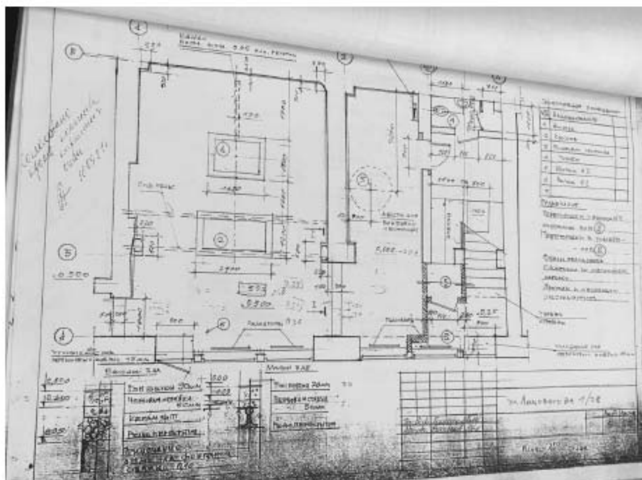
Илл. 157. Проект реконструкции помещений с устройством на 1 этаже магазина и на 2-4 этажах офисных помещений по адресу: С-Пб, ул. Ломоносова, д. 1/28, разработанный ЗАО «Проект М» в 2001 г. (нежилое помещение 66-Н). План 1-го этажа (источник: Архив КГИОП. П. 424-1. Пр-5).
