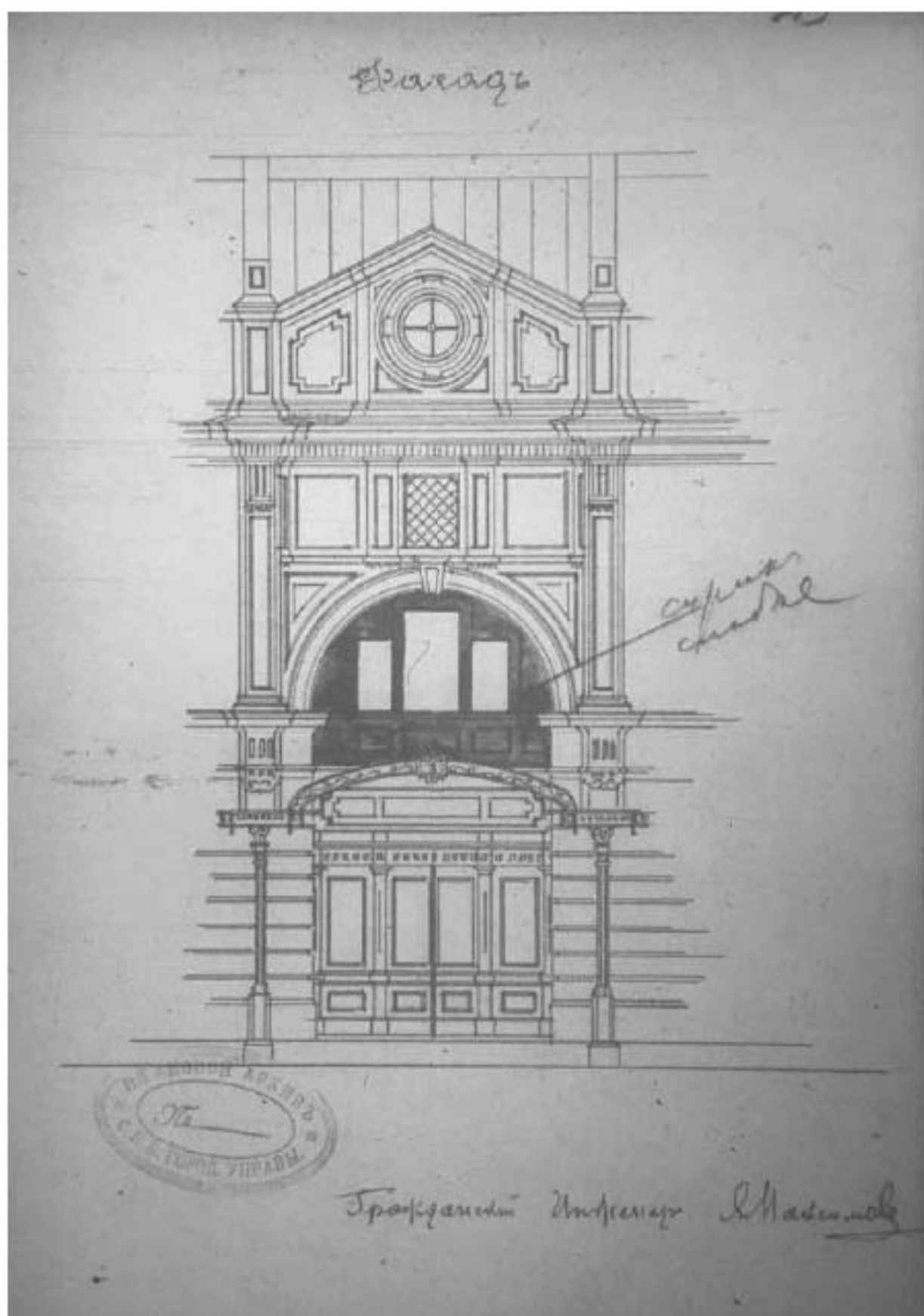
Илл. 48. Фасад лавки № 3, принадлежащей В.В. Залеману, с показанием предполагаемых к проведению работ. 1909 г. (источник: ЦГИА СПб. Ф. 513. Оп. 115. Д. 627).
