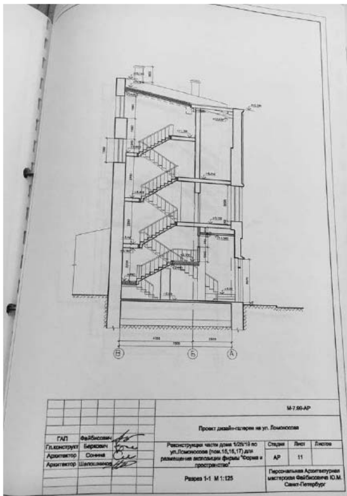
Илл. 139. Рабочий проект реконструкции помещений 15, 15 б, в, г; 16, 16 б, в, г дома 1/28/19 по ул. Ломоносова для размещения экспозиции фирмы «Форма и пространство», разработанный Персональной творческой мастерской Союза архитекторов России Ю. Файбисовича в 2001 г. (нежилые помещения 15-Н, 16-Н, 17-Н, 19-Н). Разрез 1-1 (источник: Архив КГИОП. П. 424-1. Пр-10).
