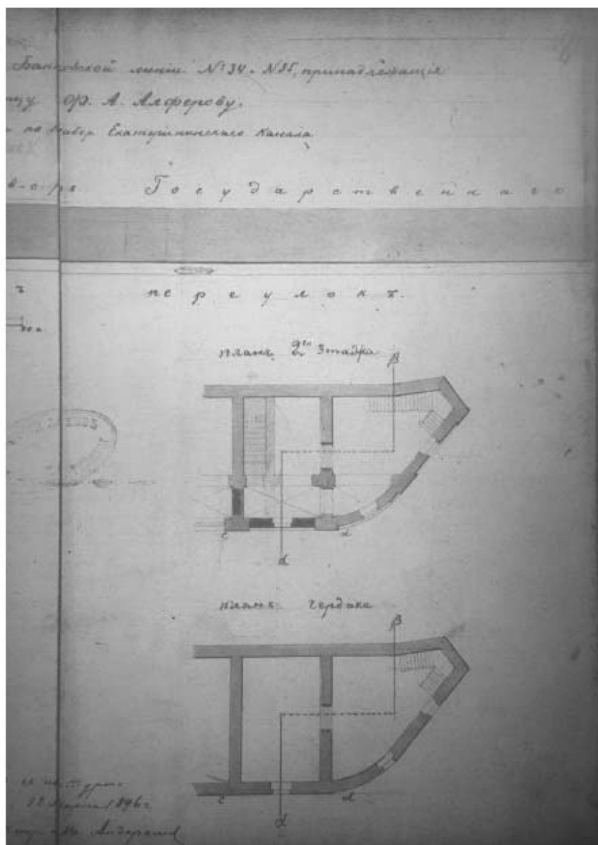
Илл. 94. Генеральный план и планы лавок № 34 и № 35, принадлежащих С.-Петербургского купцу Ф.А. Алферову с показанием предполагаемых к проведению работ. Фрагмент 1896 г. (источник: ЦГИА СПб. Ф. 513. Оп. 115. Д. 642).
