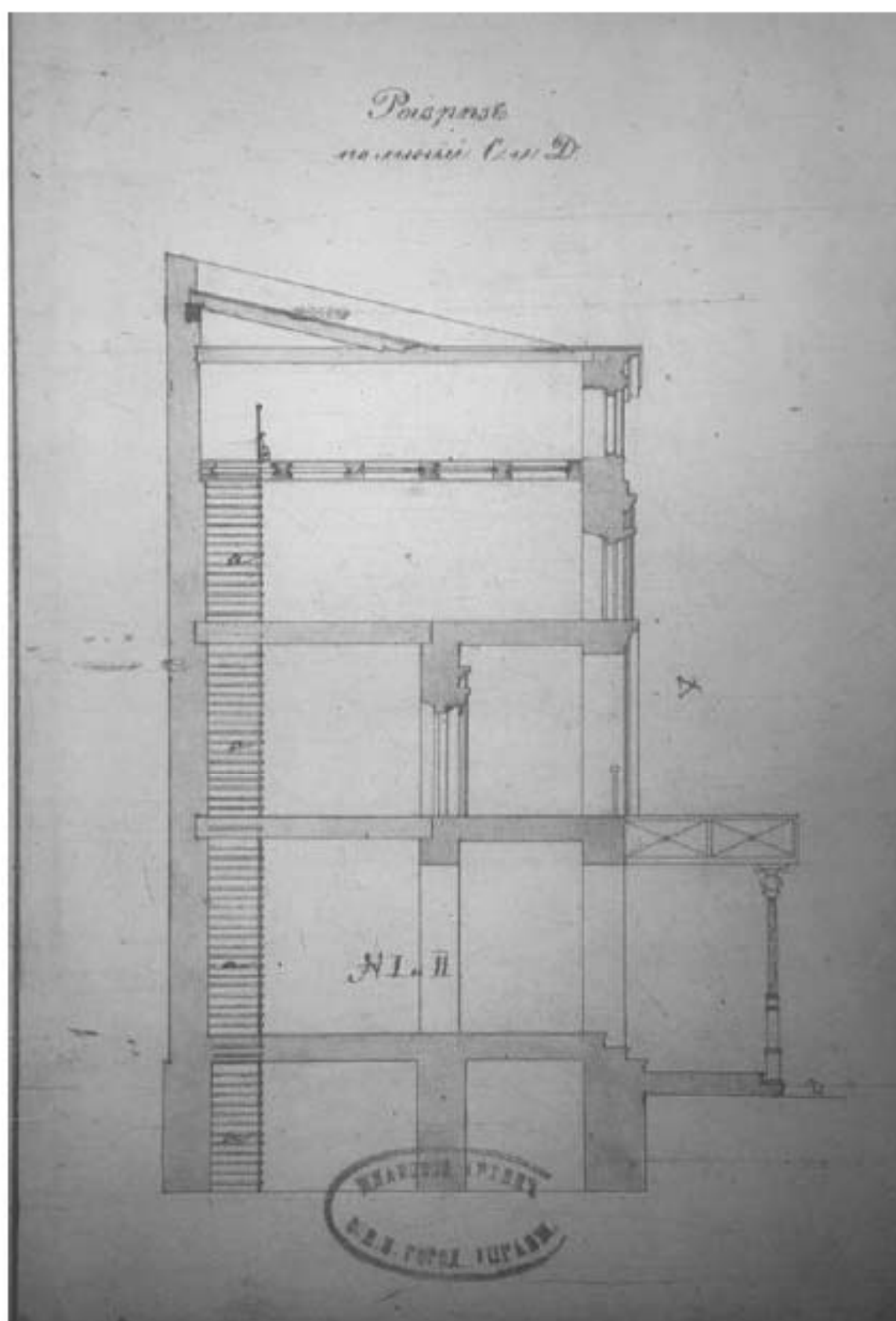
Илл. 38. Разрез лавок № 1 и № 2, принадлежащих СПб 2-й гильдии купцу Ивану Ивановичу Смирнову. 1868 г. (источник: ЦГИА СПб. Ф. 513. Оп. 115. Д. 627).
