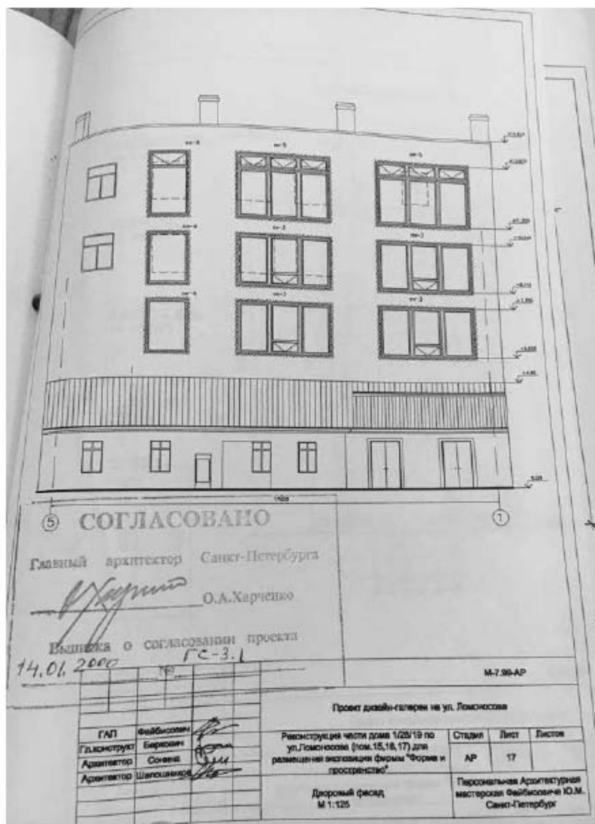
Илл. 145. Рабочий проект реконструкции помещений 15, 15 б, в, г; 16, 16 б, в, г дома 1/28/19 по ул. Ломоносова для размещения экспозиции фирмы «Форма и пространство», разработанный Персональной творческой мастерской Союза архитекторов России Ю. Файбисовича в 2001 г. (нежилые помещения 15-Н, 16-Н, 17-Н, 19-Н). Дворовый фасад (источник: Архив КГИОП. П. 424-1. Пр-10).
