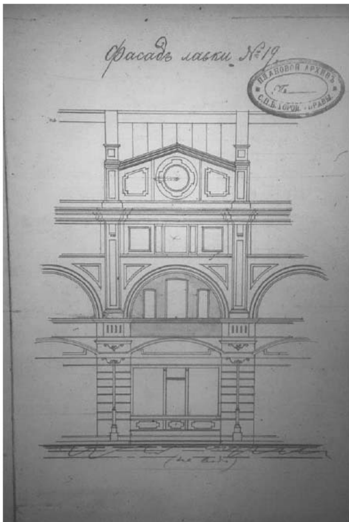
Илл. 82. Фасад лавки № 19 с показанием предполагаемых к проведению работ. 1911 г. (источник: ЦГИА СПб. Ф. 513. Оп. 115. Д. 637).
