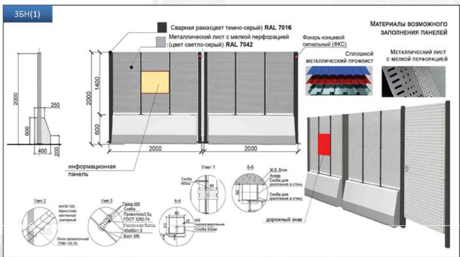
ТИП 3: ЗАЩИТНО-ОХРАННОЕ ОГРАЖДЕНИЕ
