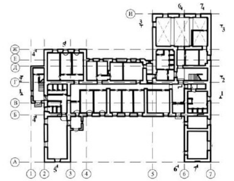
План-схема 1 этажа
