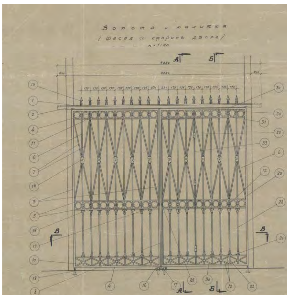
Рис. 27. Рабочие обмерно-реставрационные чертежи. Ограда и ворота между домами № 46 и 48. Фрагменты ограда и ворот. ЦГАНТД СПб. Ф. Р-36. Оп. 32. Д. 581.
