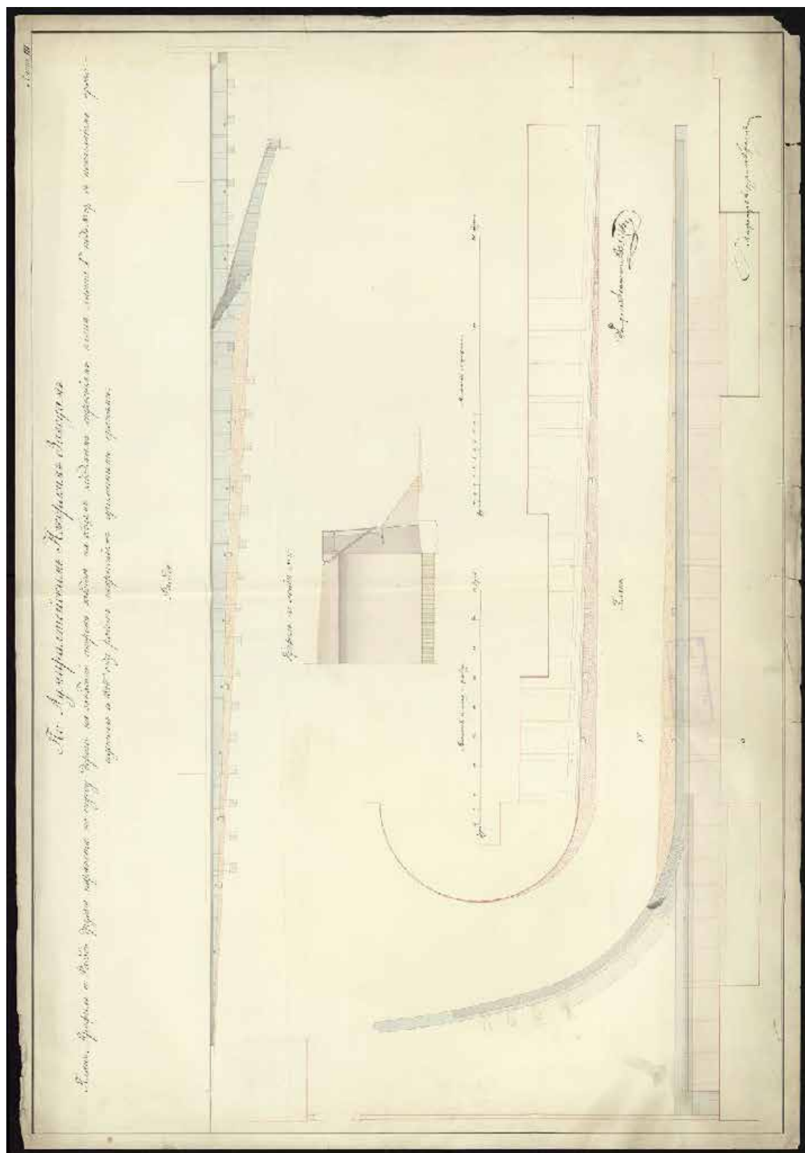
Илл. 49. План, профиль и фасад парапета по спуску дороги на западной стороне заводов с показанием произведённых работ в 1846г. РГАВМФ. Ф. 326. Оп. 1
