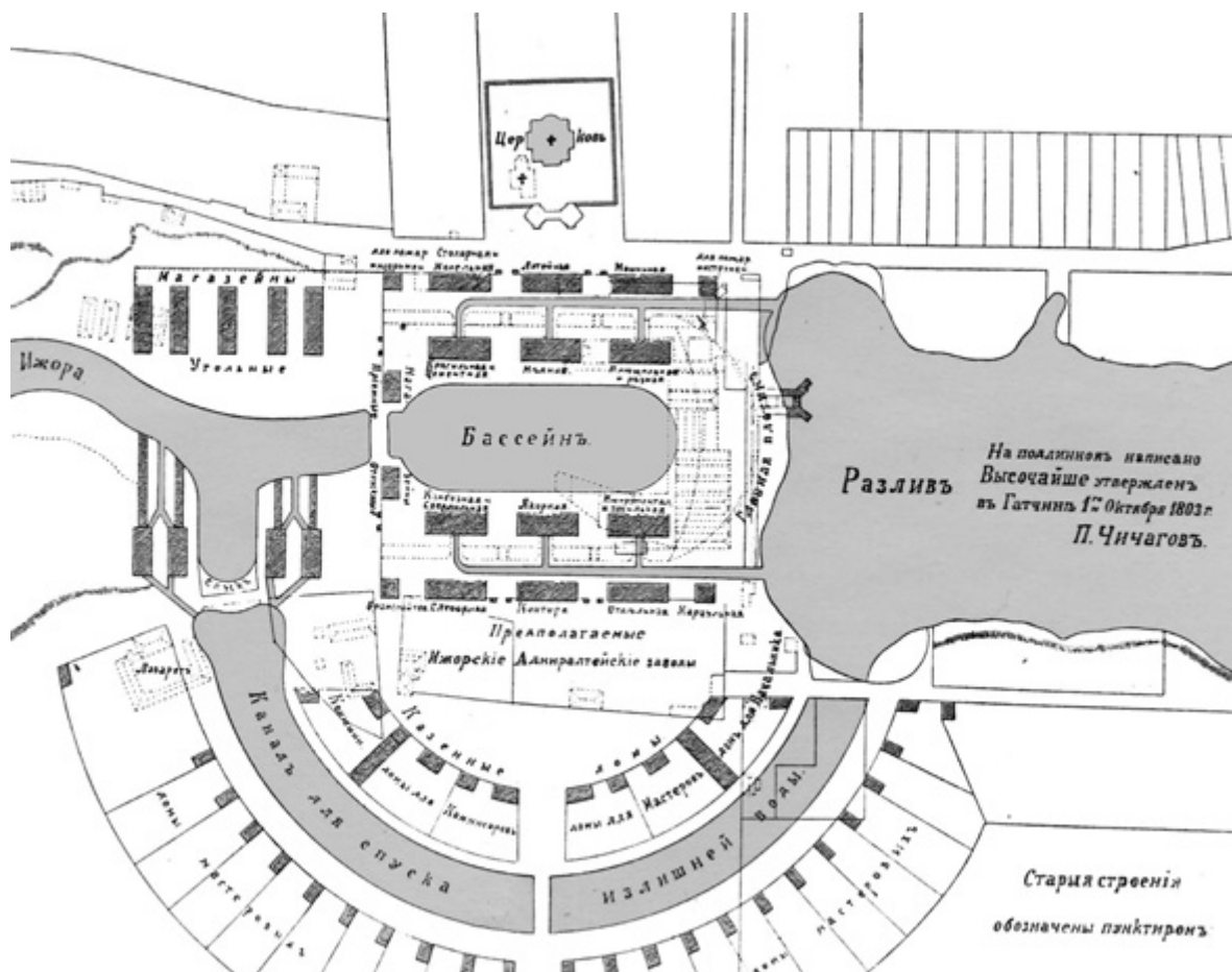
Илл. 2. Проект реконструкции заводов 1803 г. Городков Г. И. Адмиралтейские Ижорские за- воды. СПб, 1903. С.39, 49.
