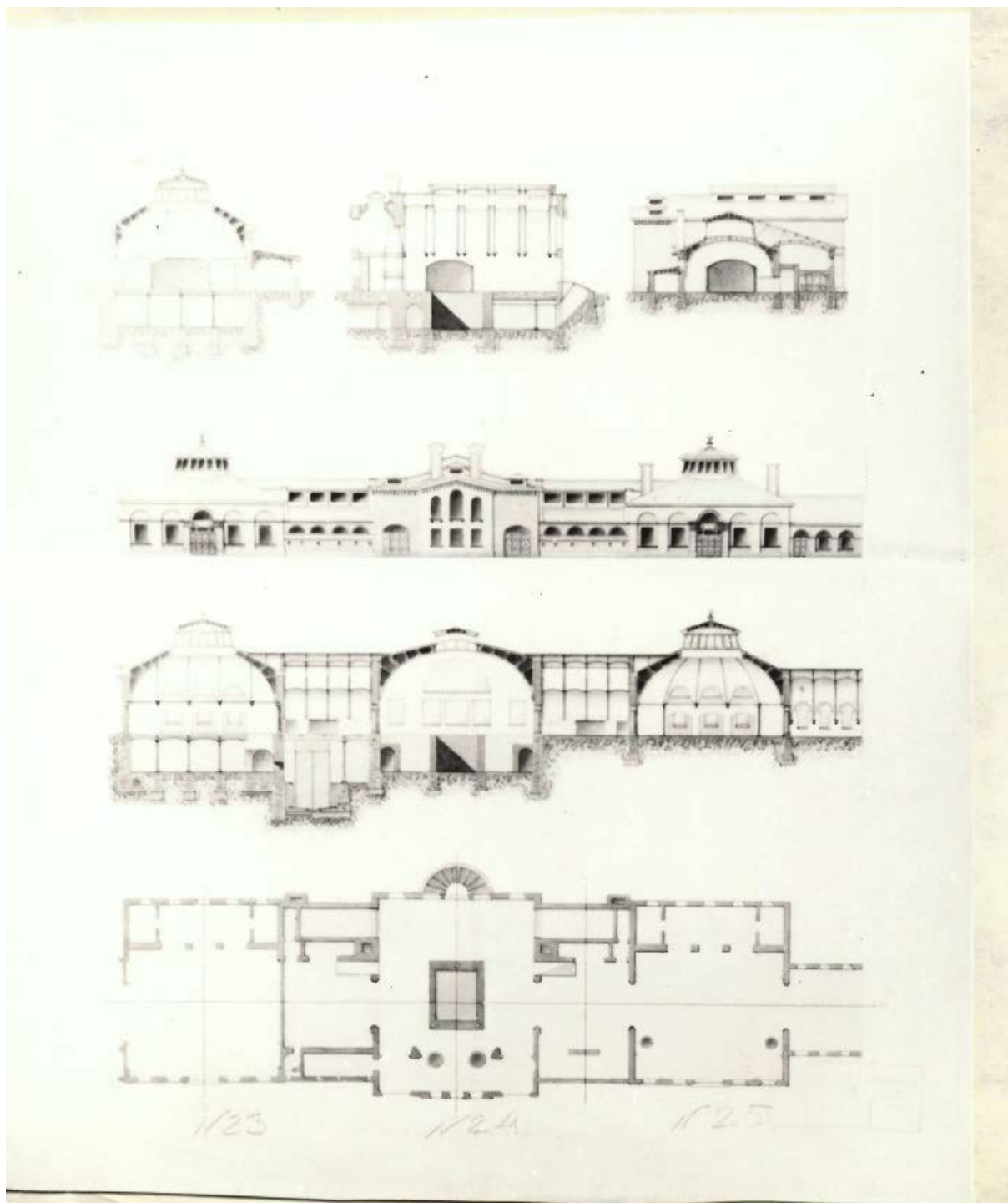
Илл. 17. Чугунолитейный завод. Фиксационный чертеж к неосуществленному проекту реконструкции 1877 г. КГИОП, № Н-4518/2, 1985. С. 59
