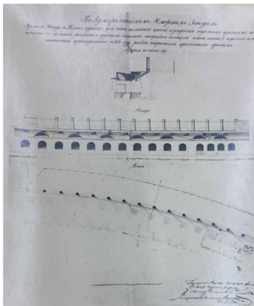
Илл. 9. Чертеж цепных кузниц 1831 г. Зельтен Л.В. Историческая справка по зданиям Ижорского завода, КГИОП, № Н-802/1, 1954, С. 21
