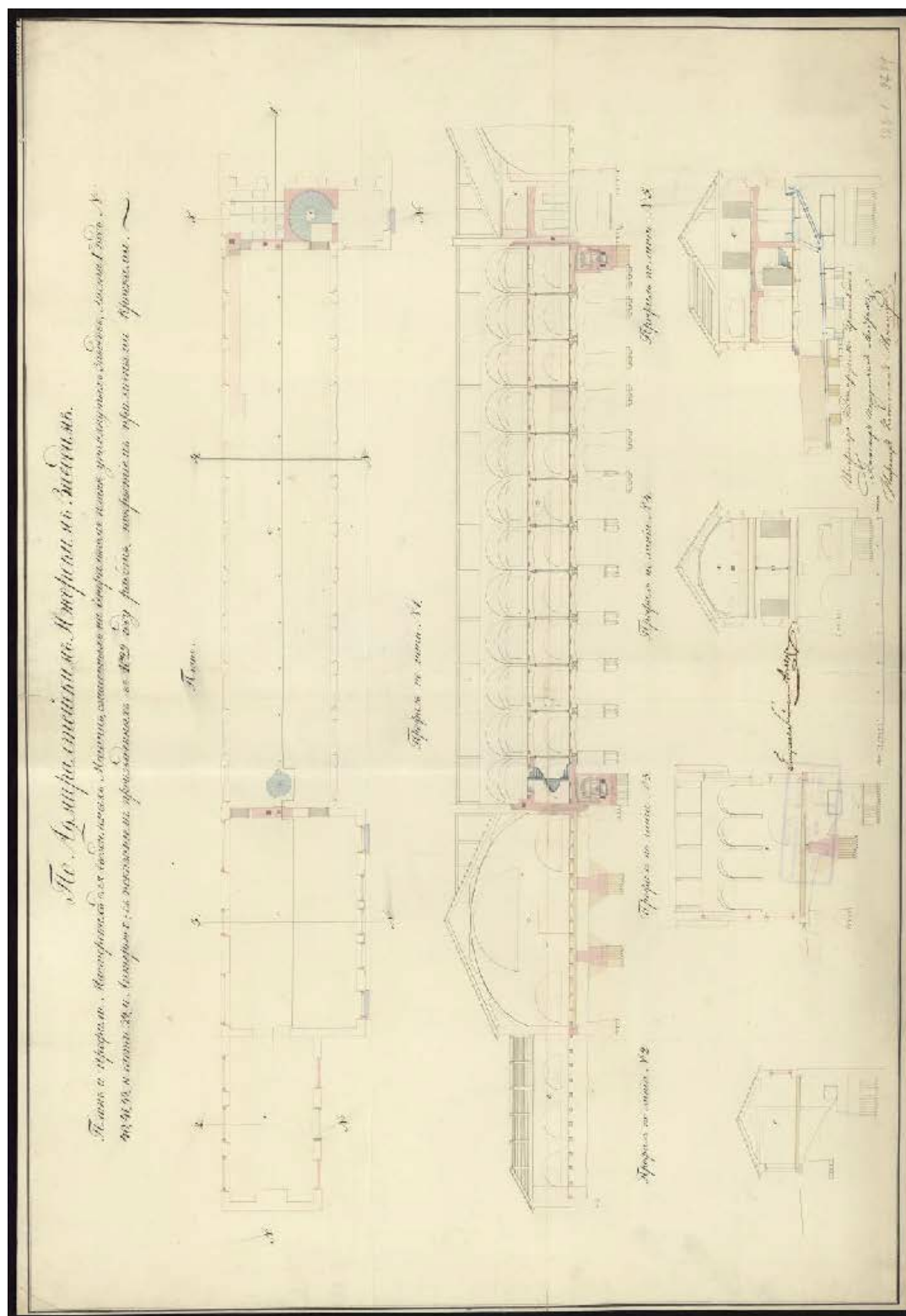
Илл. 32. План, профили гвоздильной мастерской. 1829 г. РГАВМФ. Ф. 326. Оп. 1 Д. 9744
