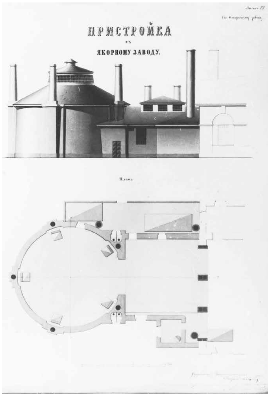
Илл. 13. Чертежи пристройки к якорному заводу для хвостовых молотов. (Фасад, план). КГИОП, № Н-4518/2, 1985, С. 32
