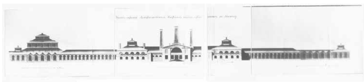
Фасад заводов (западный). Проект чугунолитейного производства. Осуществлено.
