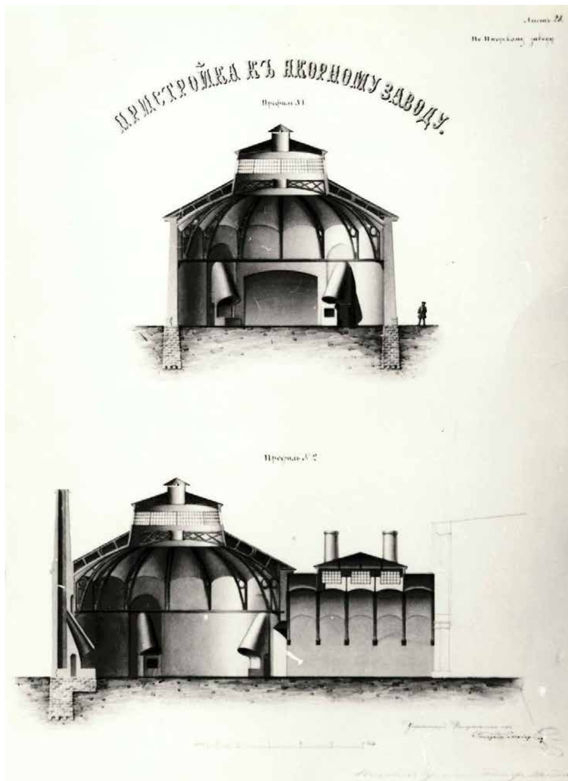
Илл. 12. Чертежи пристройки к якорному заводу для хвостовых молотов. (Разрезы, фасад, план). КГИОП, № Н-4518/2, 1985, С. 30, 31
