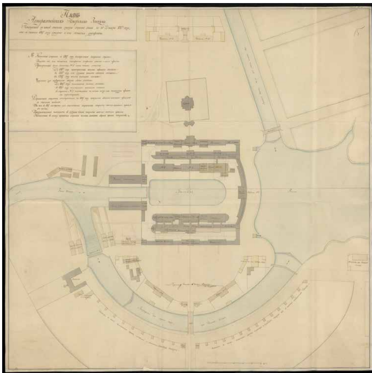
Илл. 30. План Адмиралтейских Ижорских заводов. 1819 г. РГА ВМФ. Ф. 326. Оп. 1. Д. 9397.
