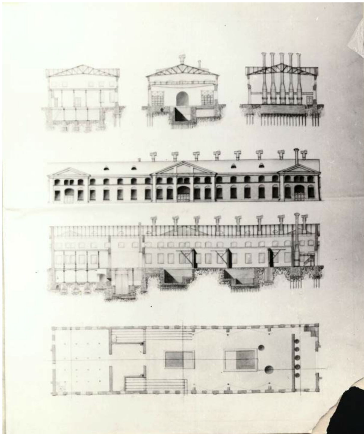
Илл. 18. Чугунолитейный завод. Фиксационный чертеж к неосуществленному проекту реконструкции 1877 г. КГИОП, № Н-4518/2, 1985. С. 59
