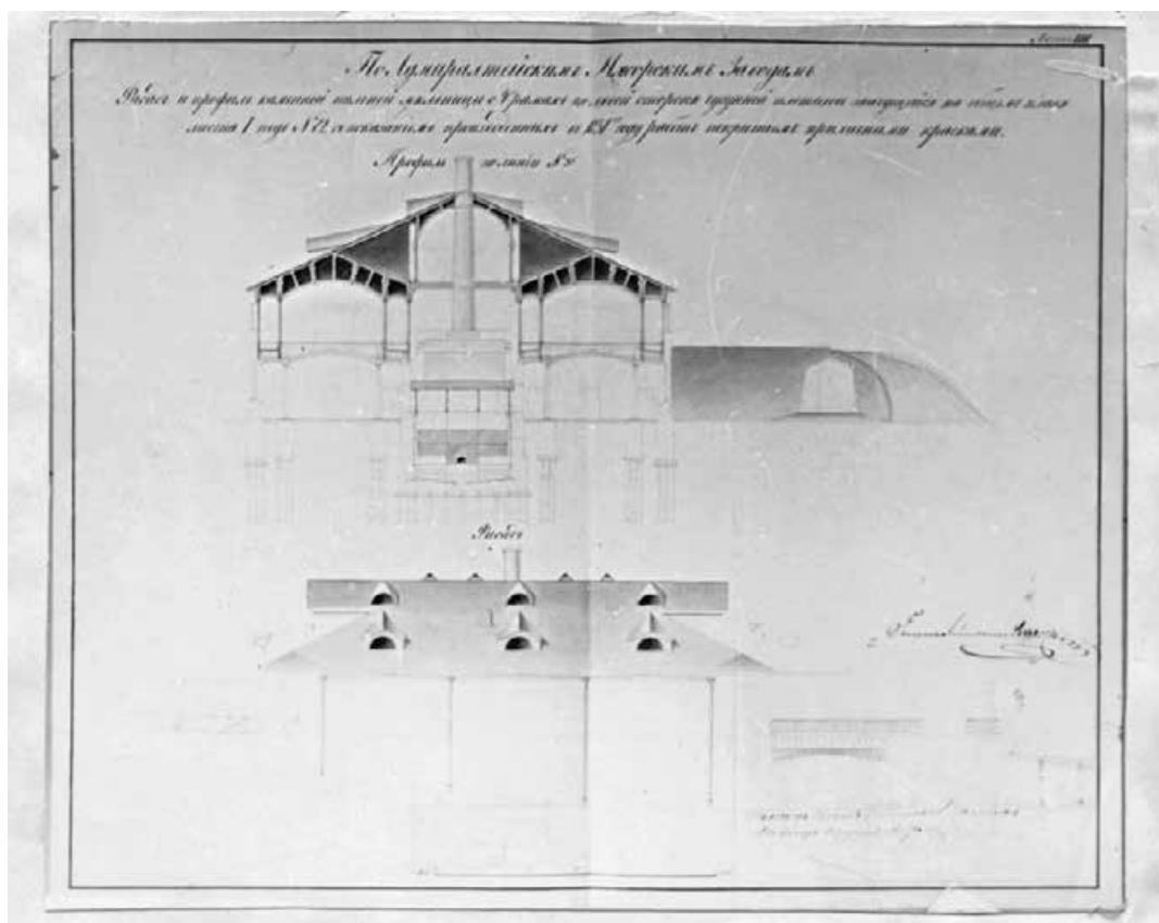
Илл. 6. Проект пильной мельницы. КГИОП № Н-4518/2, 1985, С. 73
