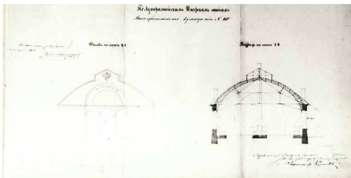
Илл. 20. Паровая кузница проект 1858 г., арх. А.С. Кудинов. КГИОП, № Н-4518/2, 1985. С.62, 63
