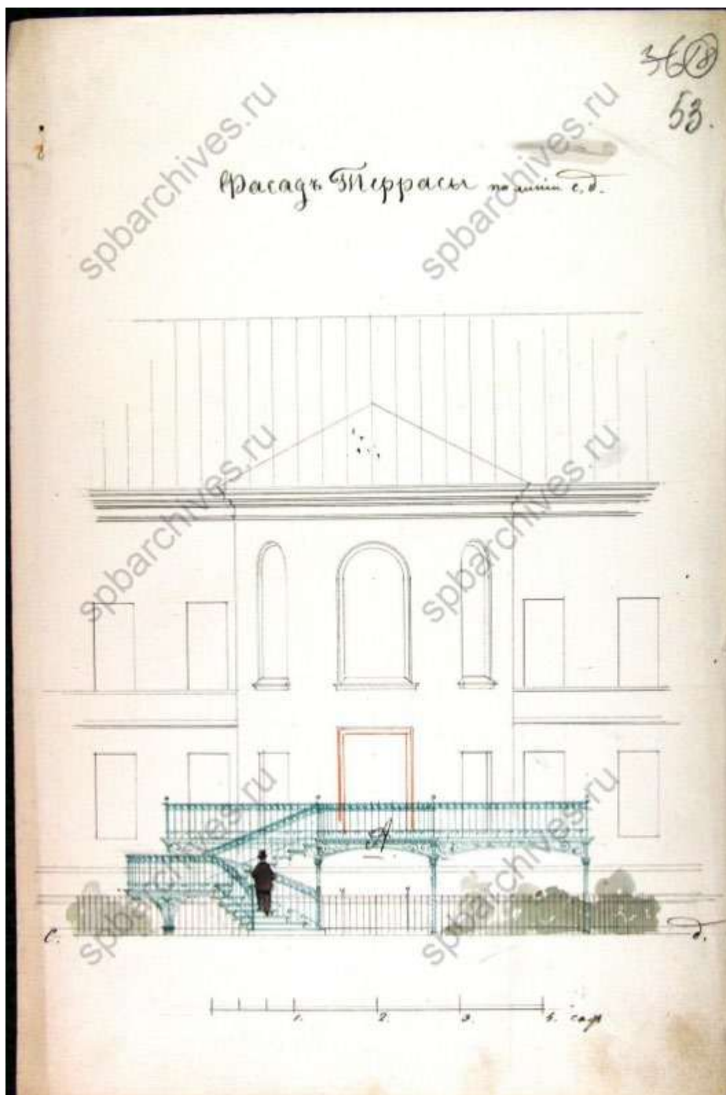
4.Фасад Террасы. ЦГАЛИ СПб
