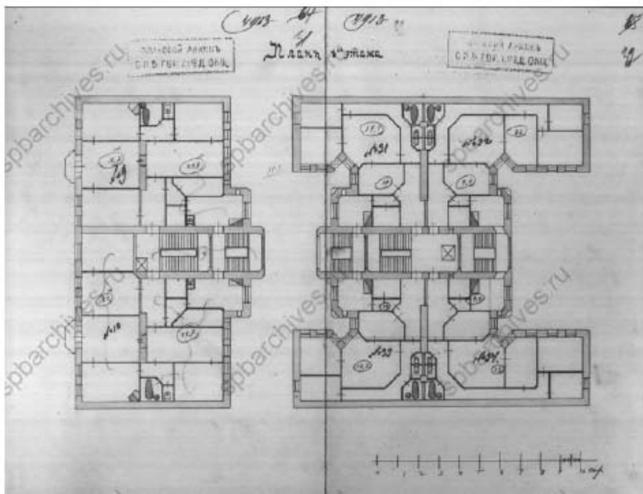
37. 1910 г. План шестого этажа. ЦГИА СПб, ф. 515, оп. 4, д. 5230, лл. 31-32.
