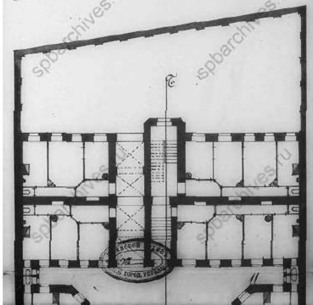
18. 1909 г. План первого этажа (фрагмент). ЦГИА СПб, ф. 513, оп. 102, д. 9517, л. 10.
