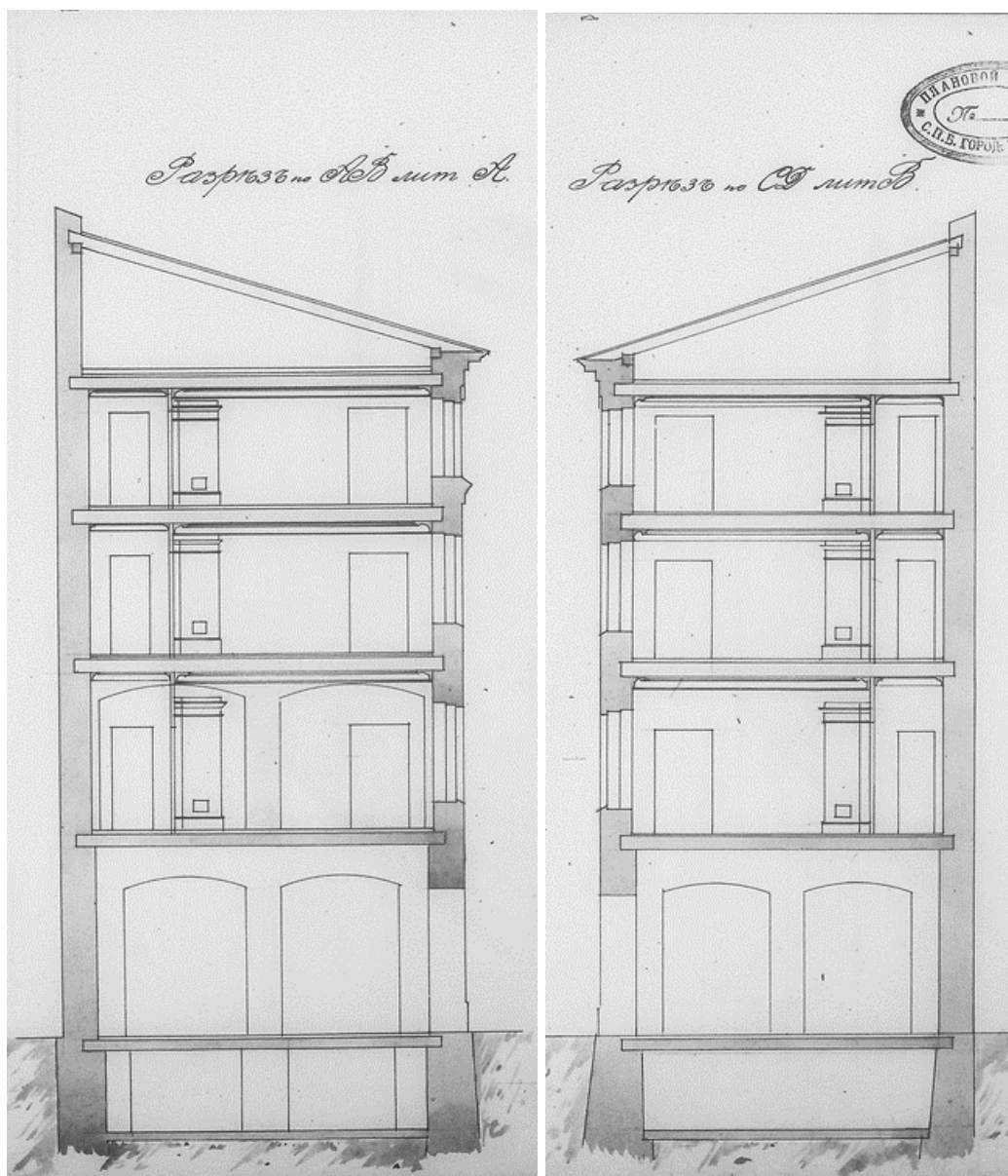
54. ЦГИА СПб. Ф. 513. Оп. 102. Д. 9709. Разрезы боковых флигелей В.А. Максимовича. 1913 г.
