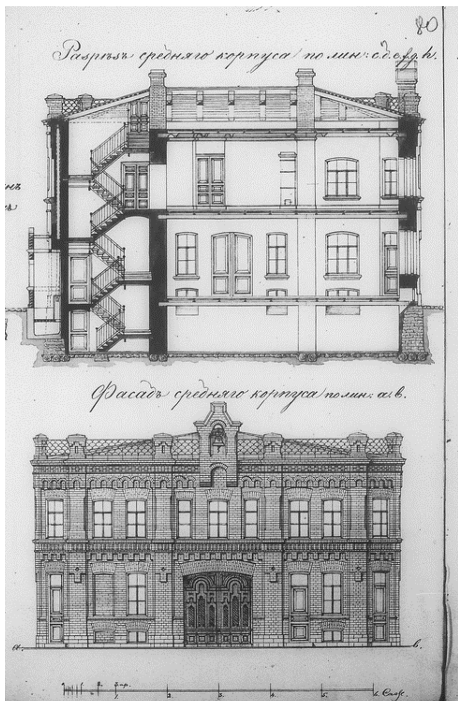
40. ЦГИА СПб. Ф. 513. Оп. 102. Д. 9709. Разрез и фасад среднего флигеля потомственного почетного гражданина Георгия Матвеевича Ландрина. 1881 г.
