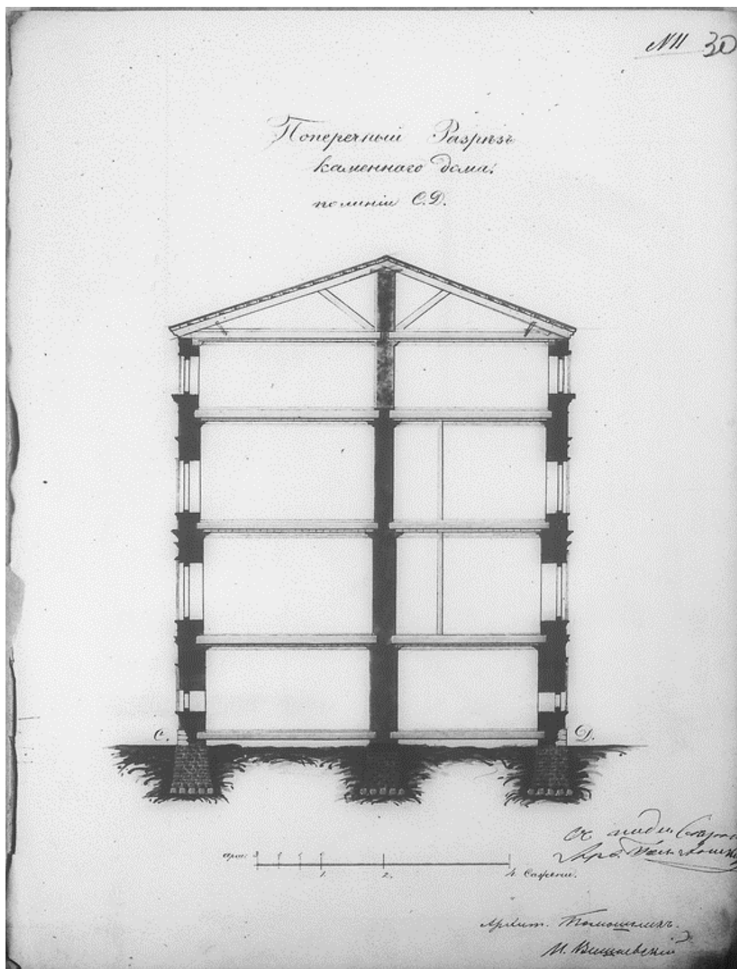
19. ЦГИА СПб. Ф. 513. Оп. 102. Д. 9709. Н.П. Гребенка. Разрез дома дворянина Станислава Вишневецкого. 1850 г.
