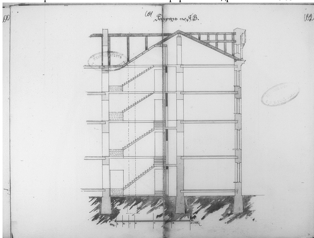
50. ЦГИА СПб. Ф. 513. Оп. 102. Д. 9709. Разрез лицевого дома В.А. Максимовича фирмы «Ландрин и Ко». 1905 г.
