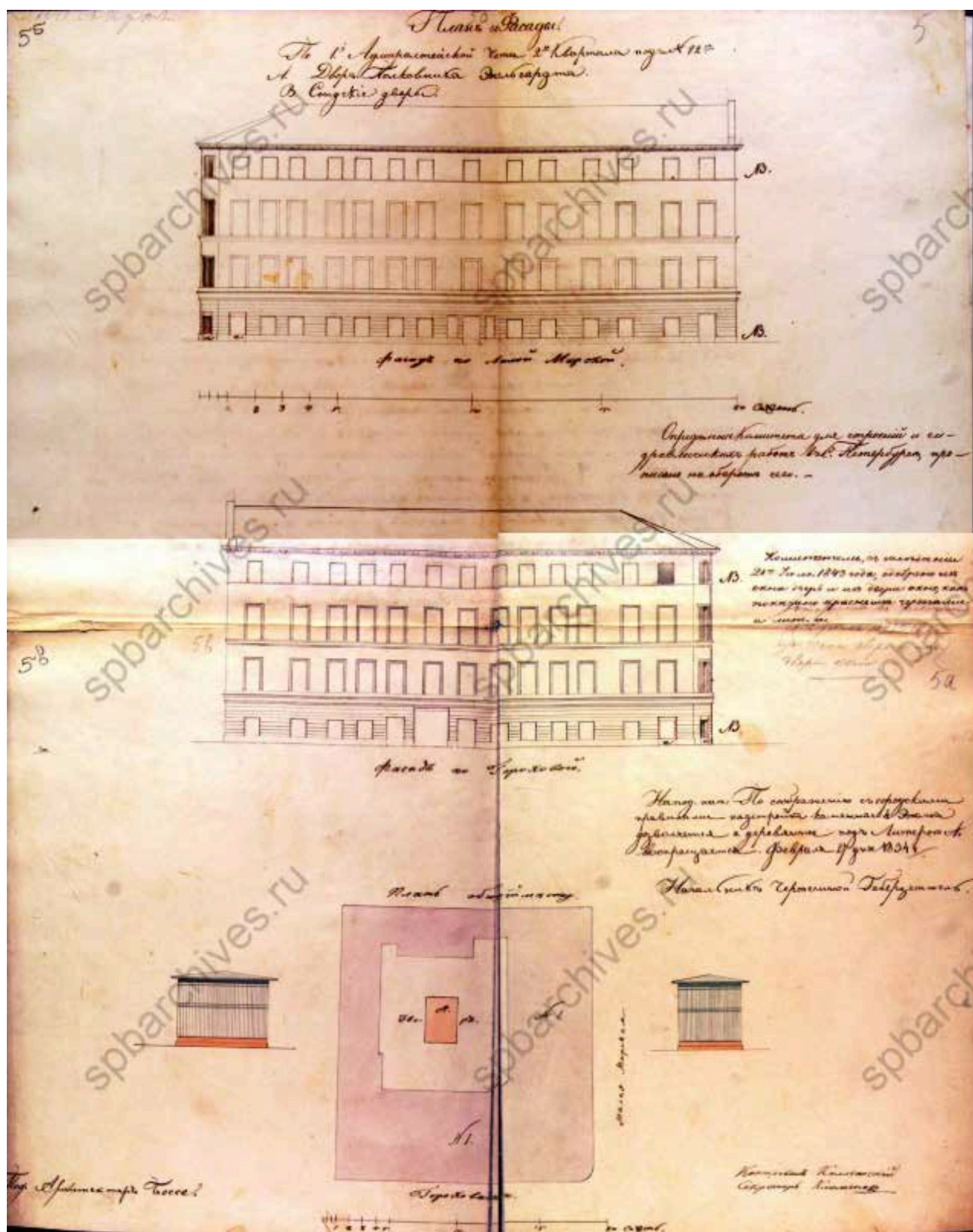
2. План и фасады по 1-й Адмиралтейской части 2-го квартала под №82. Двор полковника Энгельгардта. 1834 г. // Источник: ЦГИА СПб. Фонд 513.
