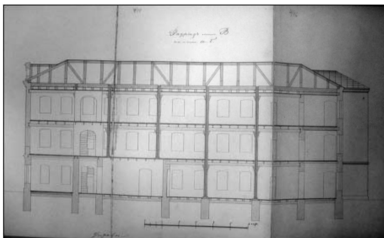
19. Разрез по линии а-б производственного корпуса (в настоящее время – корпус лит. В). 1895 г. // Архив фабрики «Свечо» . Папка № 29. Л. 4/14-4/16
