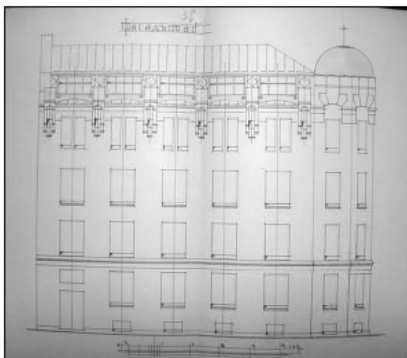
88. Фасад по 2-6 производственного корпуса (в настоящее время – лит. Е) с показанием надстройки мансардного этажа. Гр. инж. Л.П. Андреев. 1911 г. // ЦГИА СПб. Ф. 513. Оп. 102. Д. 7562. Л. 38-39.
