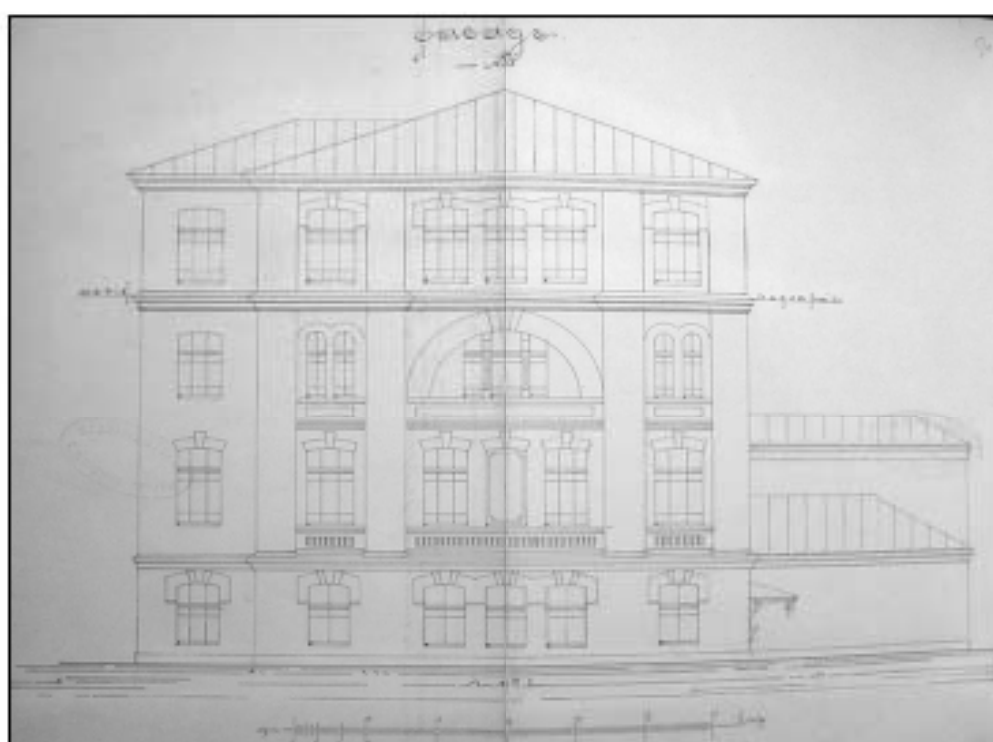
33. Фасад производственного корпуса (в настоящее время – корпус лит. В) с показанным надстройкой 4-го этажа. Гр. инж. Л.П. Андреев. 1902 г. // ЦГИА СПб. Ф. 513. Оп. 102. Д. 8363. Л. 55-56.
