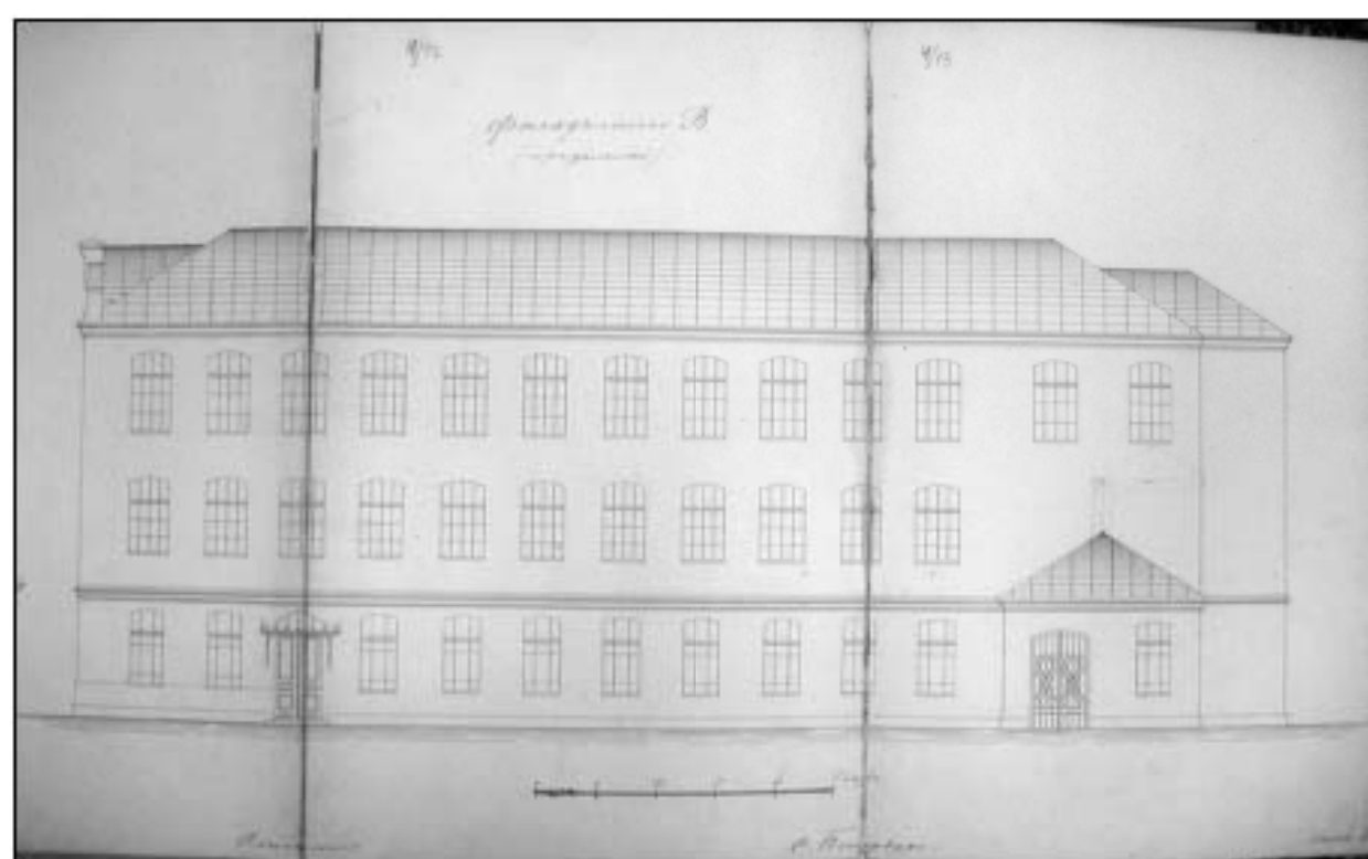
18. Фасад (продольный) производственного корпуса (в настоящее время – корпус лит. В). 1895 г. // Архив фабрики «Свечи». Папка № 60. Л. 4/11-4/13.
