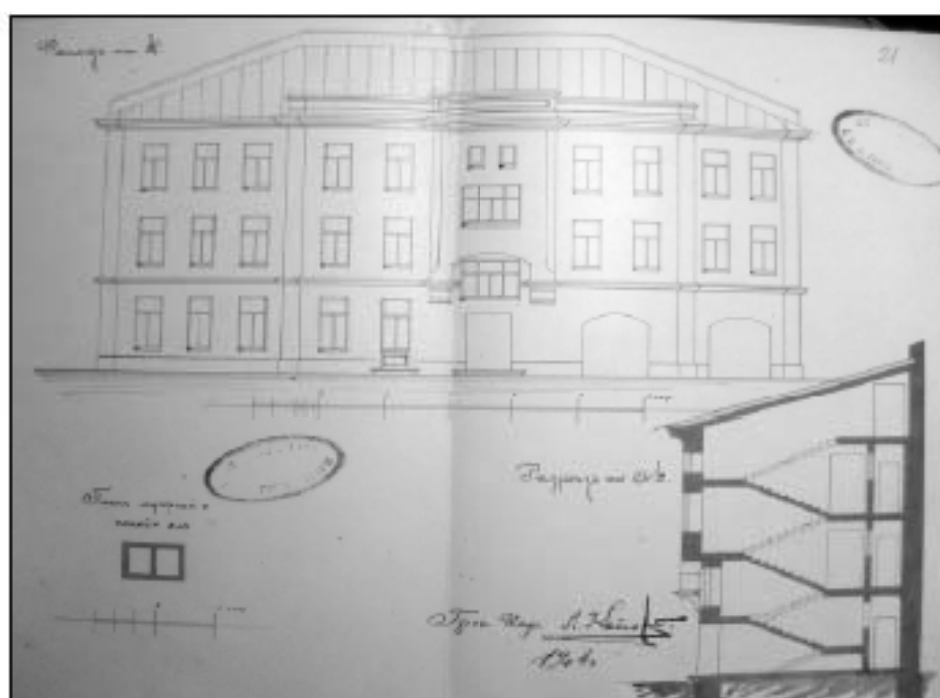
48. Фасад, разрез по а-б каменного дома Шустовой (в настоящее время — часть корпуса лит. 3), план мусорной и помойной ям. Гр. инж. Л. Котов. 1904 г. // ЦГИА СПб. Ф. 513. Оп. 102. Д. 8362. Лл. 20-21.
