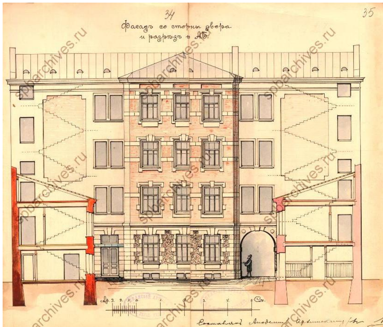
Илл. 10. Фасад со стороны двора и разрез. 1901 г. Акад. арх. В. Прусаков. ЦГИА СПб. Ф. 513. Оп. 102. Д. 1501. Л. 34, 35.
