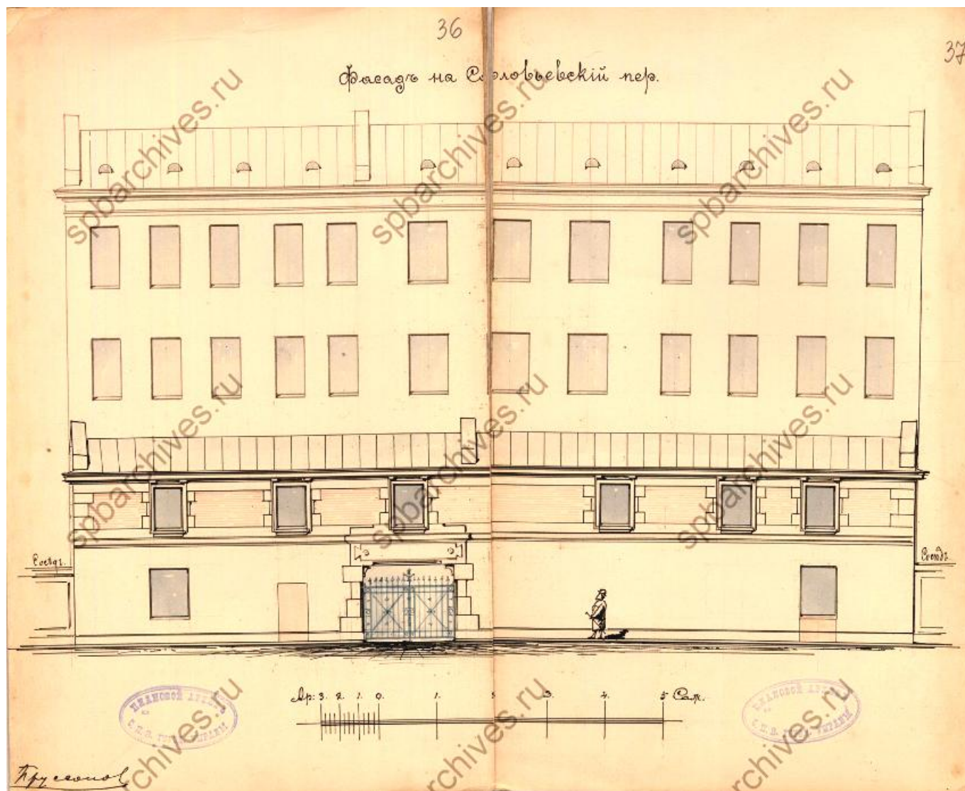
Илл. 11. Фасад по Соловьёвскому переулку. 1901 г. Акад. арх. В. Пруссаков. ЦГИА СПб. Ф. 513. Оп. 102. Д. 1501. Л. 36, 37..
