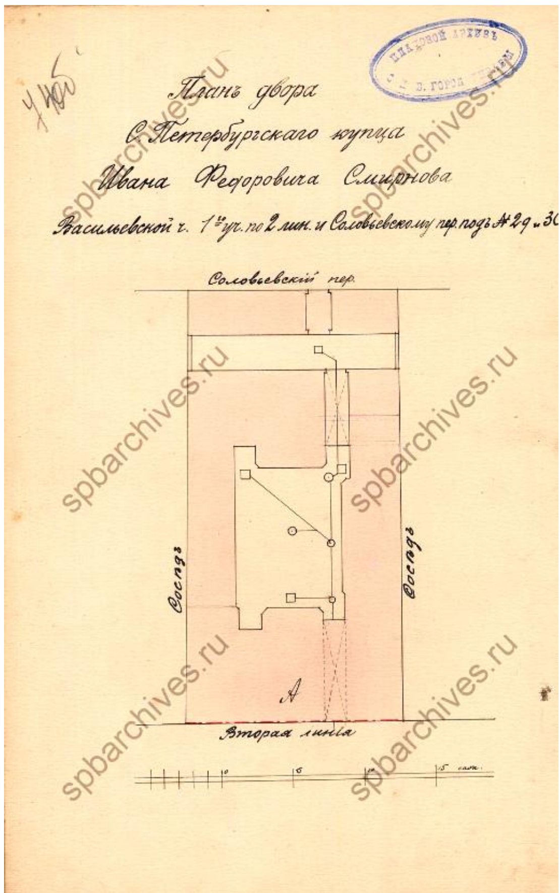
Илл. 17. План двора С.-Петербургскаго купца Ивана Федоровича Смирнова. Васильевской части, 1-го участка по 2-й линии и Соловьевскому переулку под № 29 и 30. 1906 г. Арх. Ф.Ф. фон Постельс. ЦГИА СПб. Ф. 513. Оп. 102. Д. 1501. Л. 74об.
