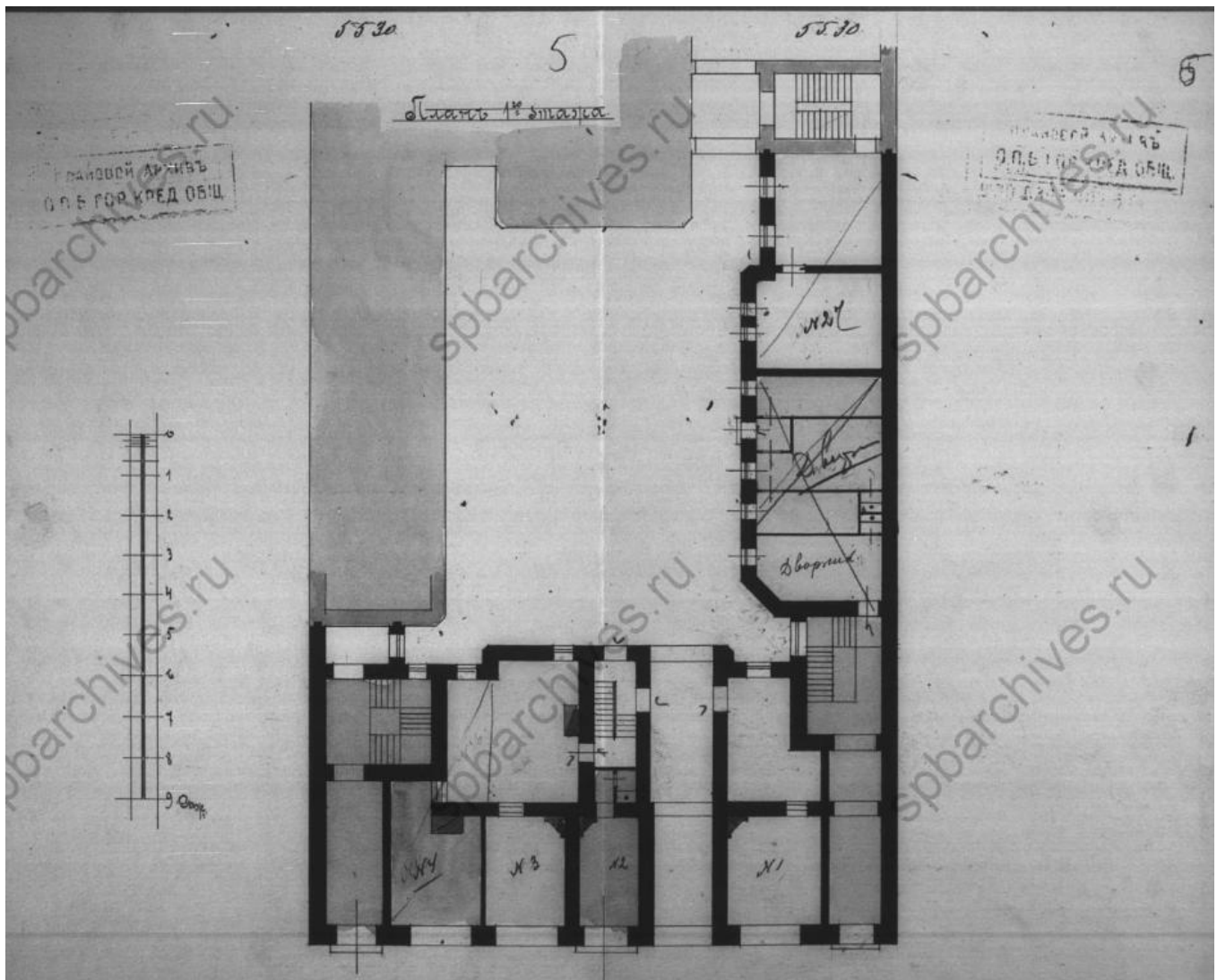
Илл. 22. План 1 этажа. ЦГИА СПб. Ф. 515. Оп. 4. Д. 2671. Л. 5, 6.
