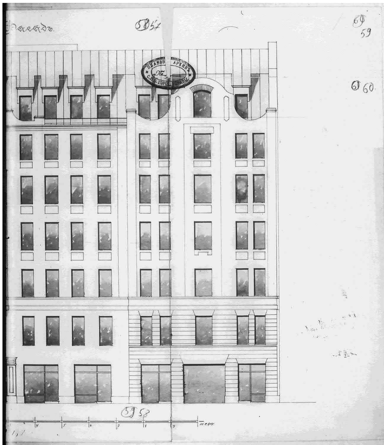
Илл.15. Лицевой фасад дома Э. Э. Арнольда (правая часть). ЦГИА СПб. Ф. 513. Оп. 102. Д. 9449
