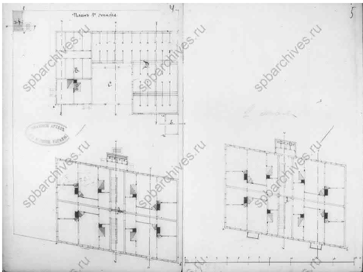
Илл.3. План деревянного дома П. С. Платонова. www.spbarchives.ru
