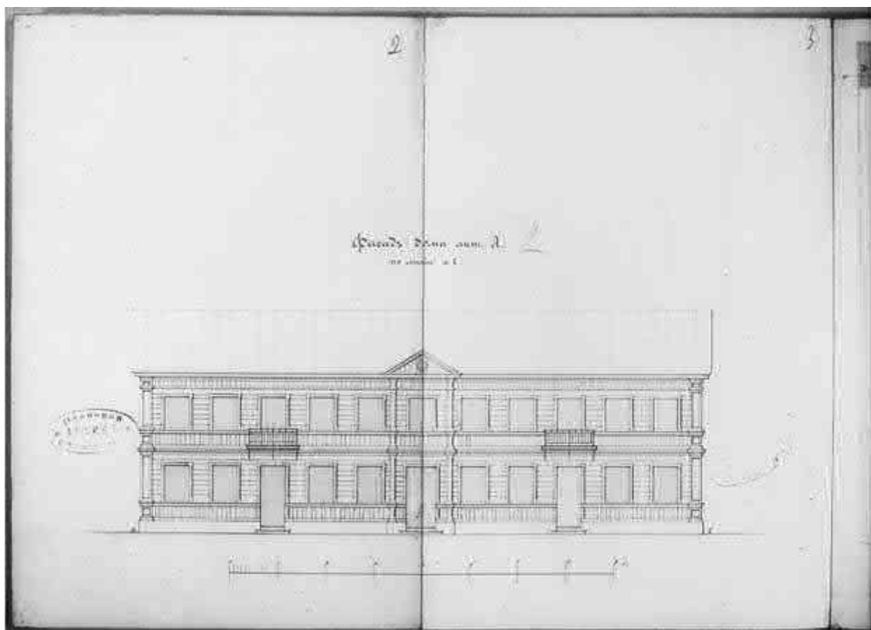
Илл.1. Фасад дома П. С. Платонова. ЦГИА СПб. Ф. 513. Оп. 102. Д. 9449
