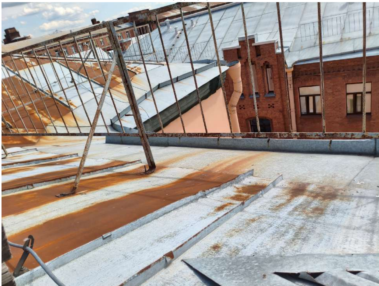
Фото 28. Общее состояния кровельного покрытия лицевого корпуса. Дата фотофиксации: 26.09.2025г.
