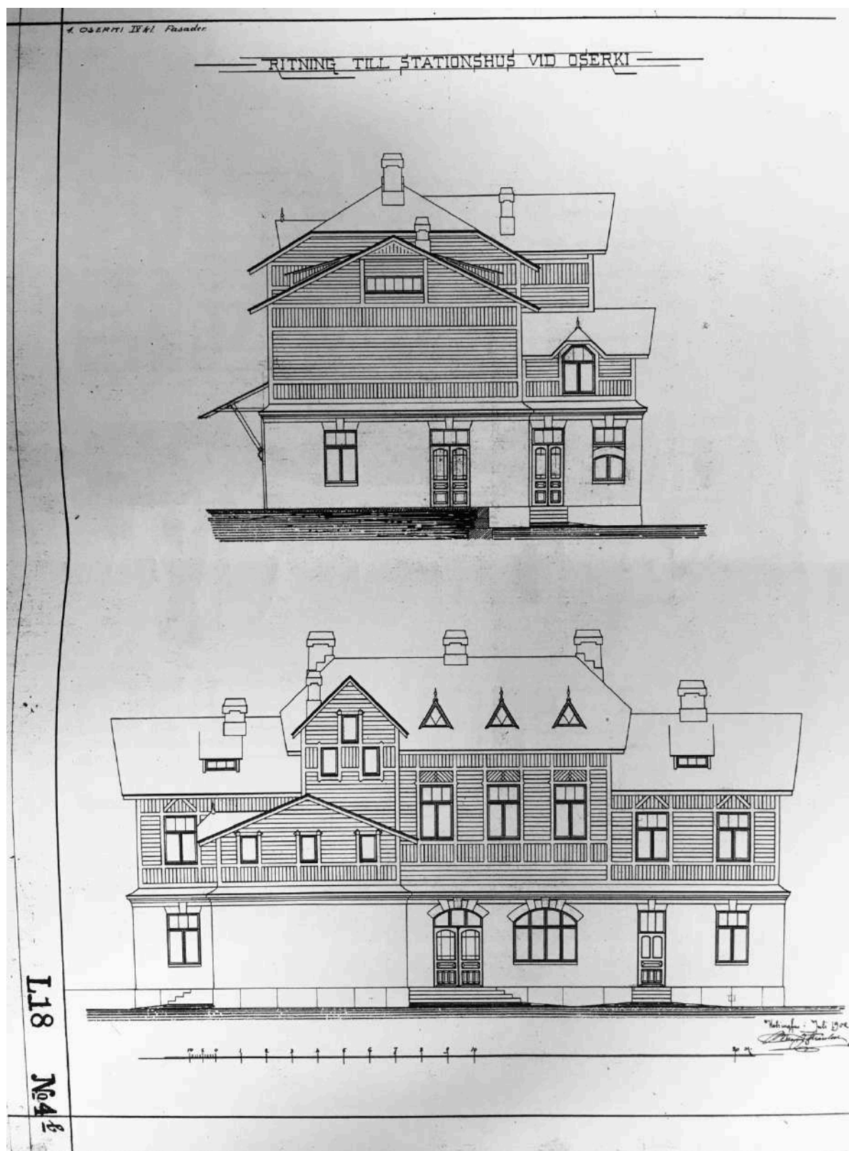
16. Б.Ф. Гранхольм. Проект вокзала на станции Озерки. 1902 г. Южный фасад. Восточный фасад. В. Н. Свешникова. ЛИНИЯ РИХИМЯКИ - САНКТ-ПЕТЕРБУРГ ФИНЛЯНДСКОЙ ЖЕЛЕЗНОЙ ДОРОГИ (от Санкт-Петербурга до Белоострова).
