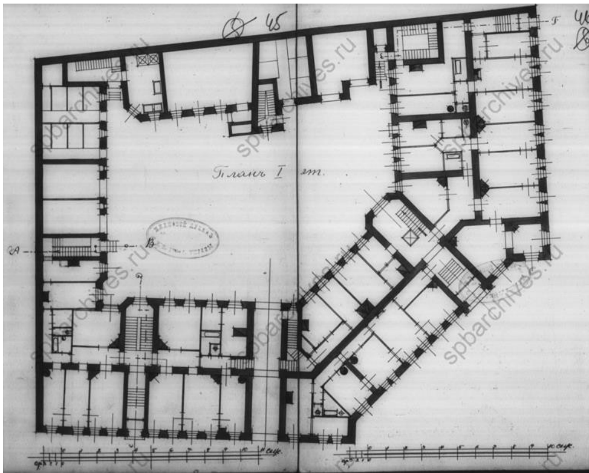
Илл. 33. «План I этажа». 1902 г.
