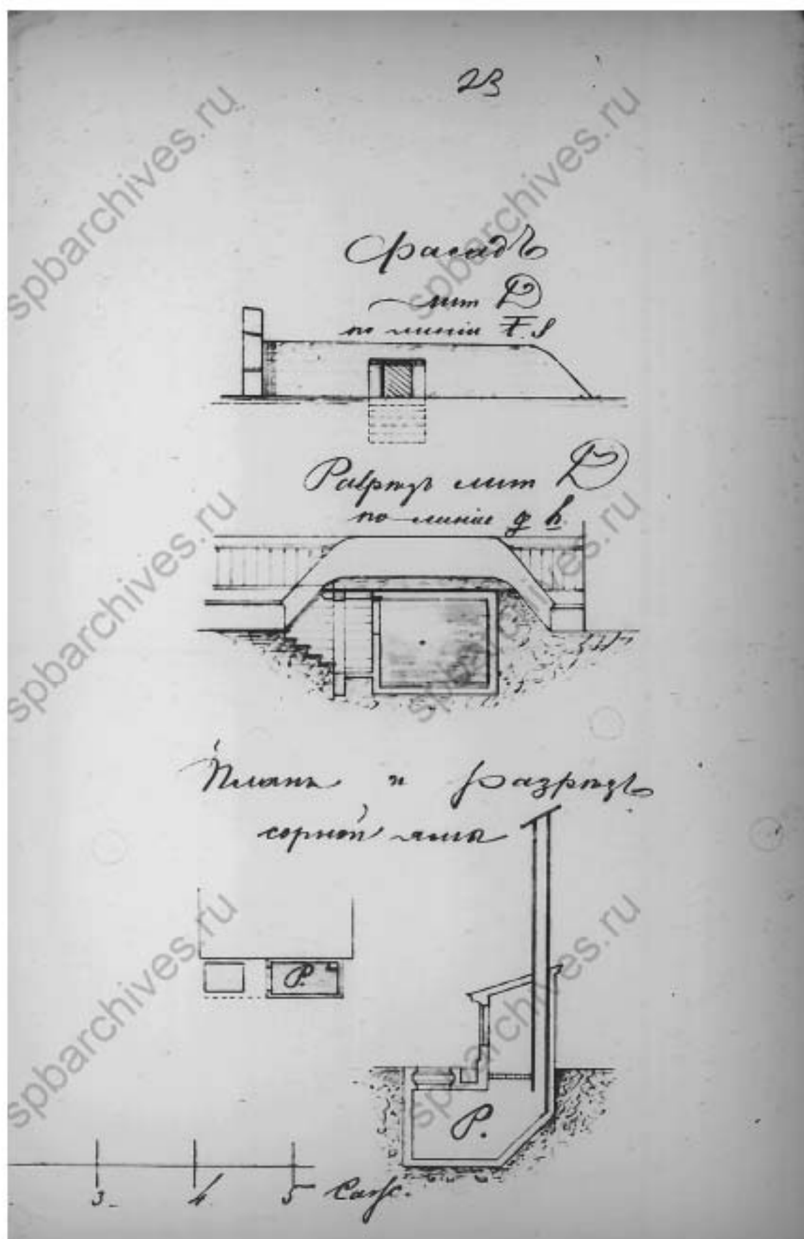
18. Фасадъ лит. D. Разрѣзъ лит. D. Планъ и разрѣзъ сорной ямы. 1876 г. // Источник: ЦГИА СПб Ф.513 Оп.102 Д.1870 Л.23.
