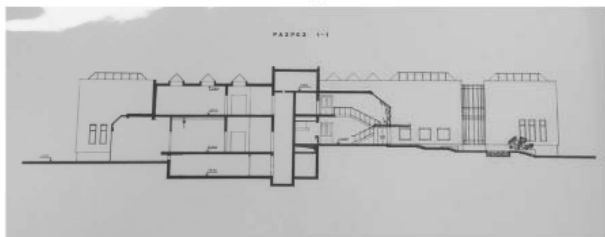
18. Проект реставрации главного здания Академии художеств 1989 г. Разрез I-I. ЦГАНТД СПб. Ф. Р-398. Оп. 35. Д. 582.
