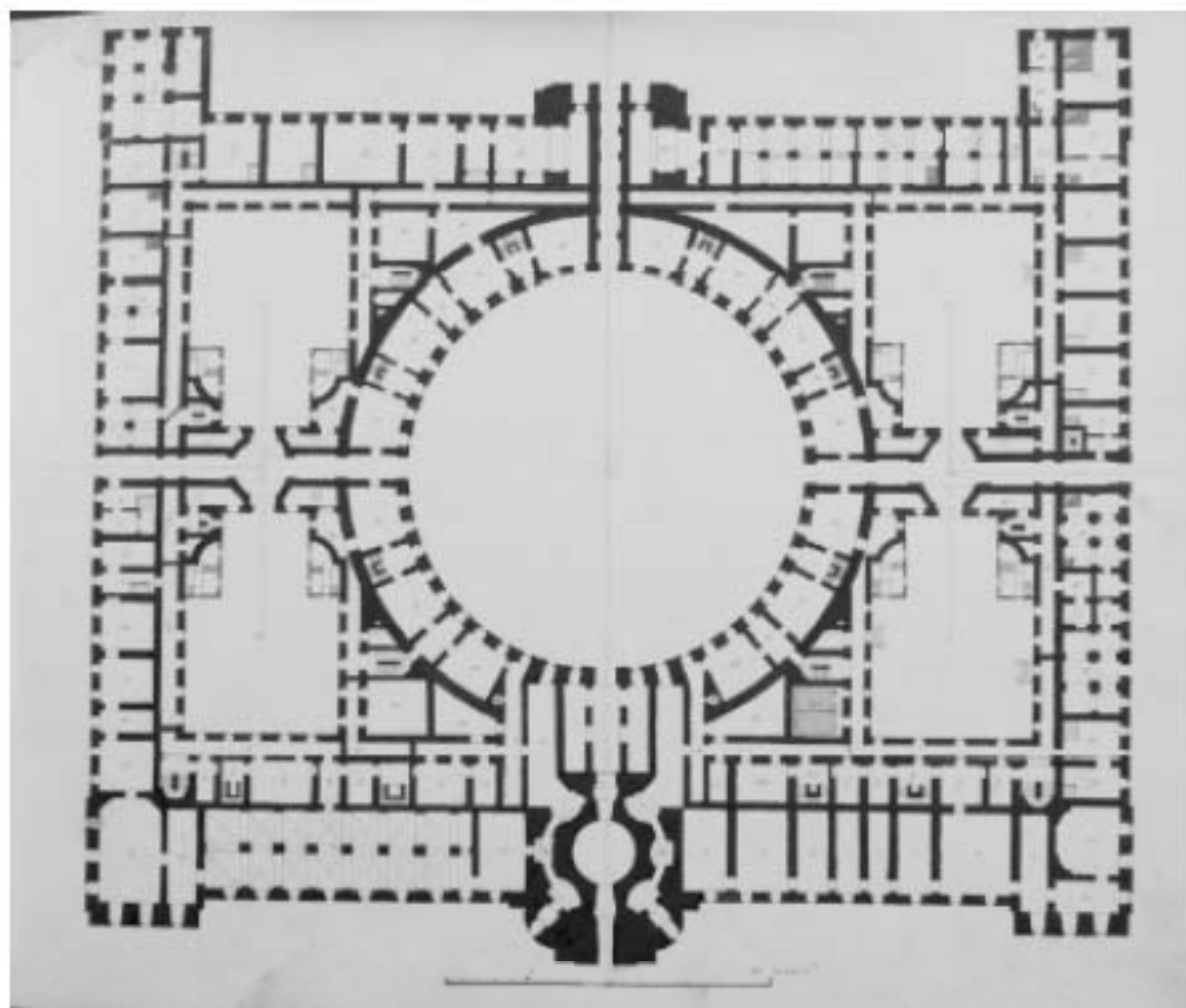
7. План подвального этажа здания Академии художеств, 1820-е гг. Музей НИИМРАХ, А-21717.
