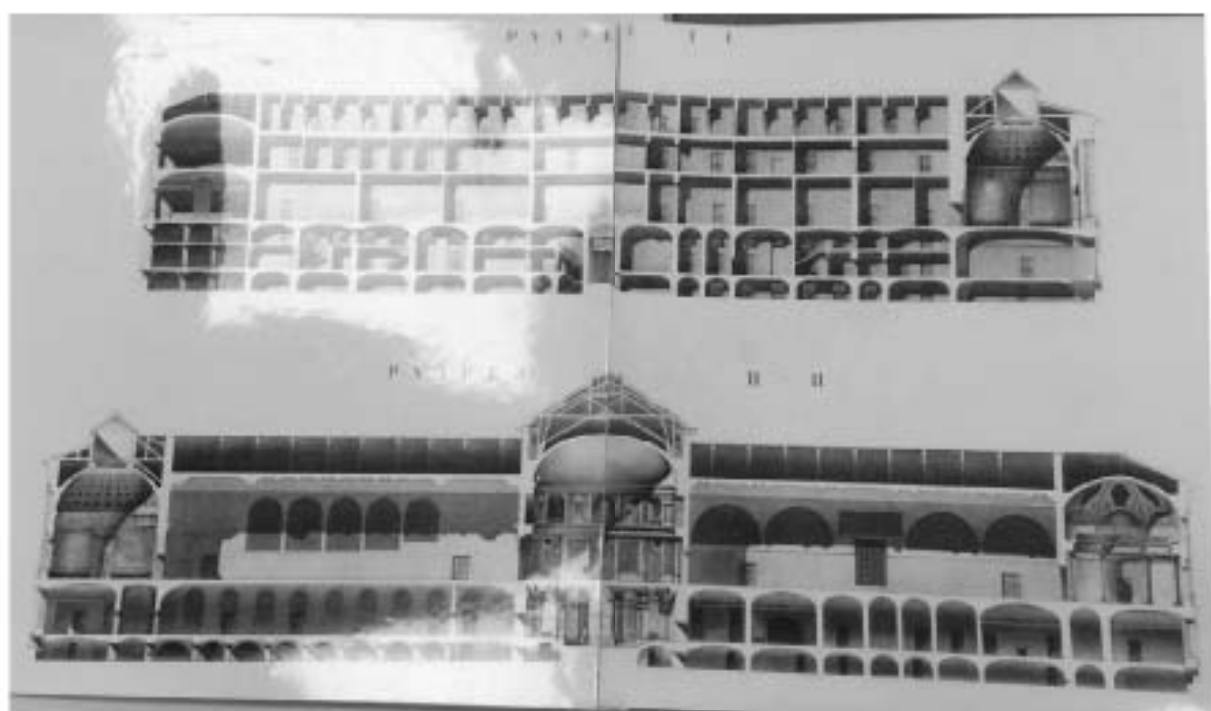
19. Проект реставрации главного здания Академии художеств 1989 г. Разрез I-I и II-II. ЦГАНТД СПб. Ф. Р-398. Оп. 35. Д. 582.
