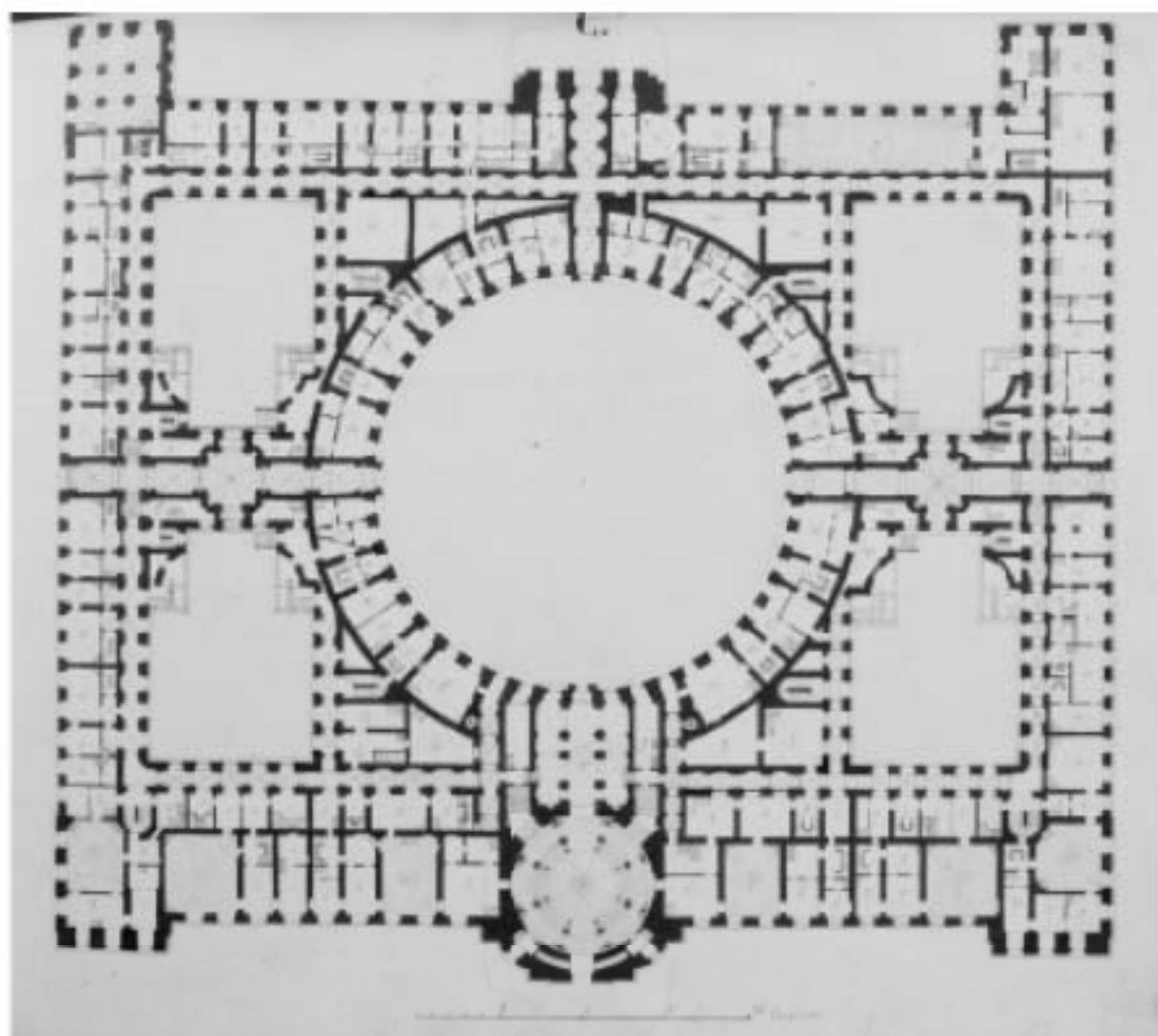
8. План 1-го этажа здания Академии художеств, 1820-е гг. Музей НИИМРАХ, А-21718.
