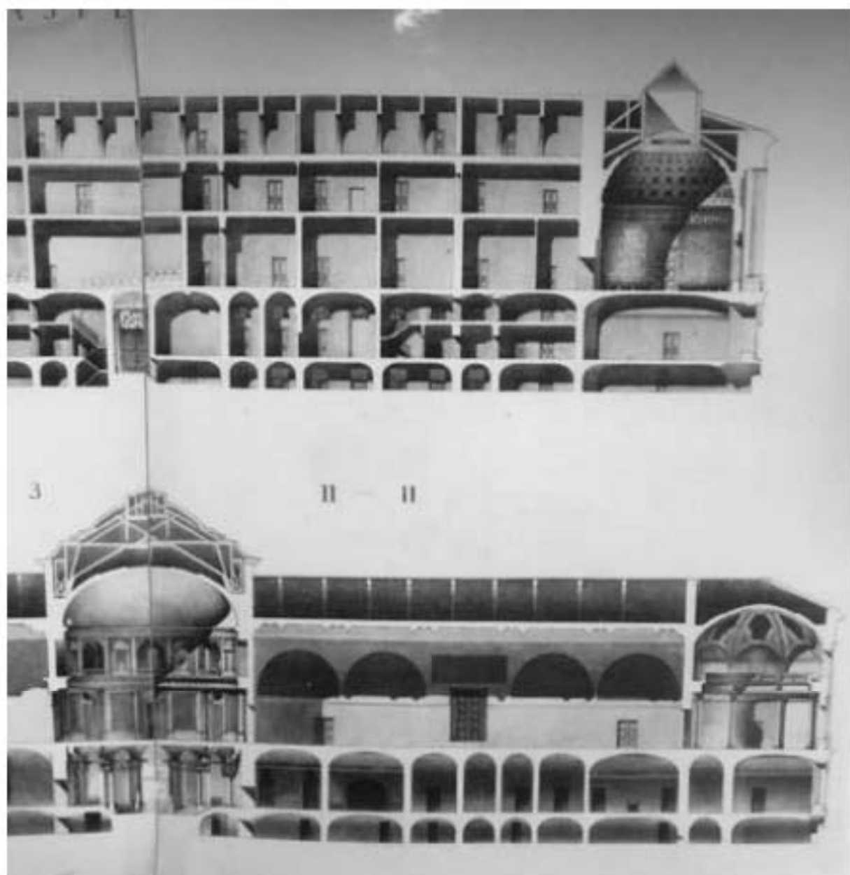
21. Проект реставрации главного здания Академии художеств 1989 г. Разрез I-I и II-II. Фрагмент. Правая часть. ЦГАНТД СПб. Ф. Р-398. Оп. 35. Д. 582.
