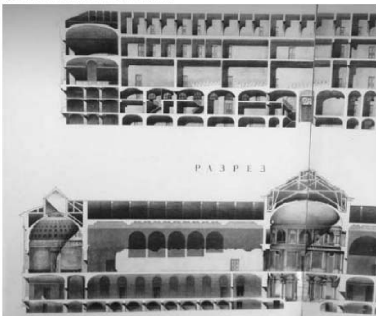
20. Проект реставрации главного здания Академии художеств 1989 г. Разрез I-I и II-II. Фрагмент. Левая часть. ЦГАНТД СПб. Ф. Р-398. Оп. 35. Д. 582.
