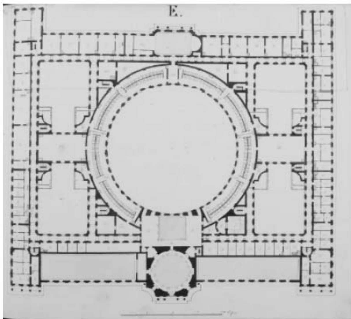
10. План 3-го этажа здания Академии художеств, 1820-е гг. Музей НИИМРАХ, А-21720.
