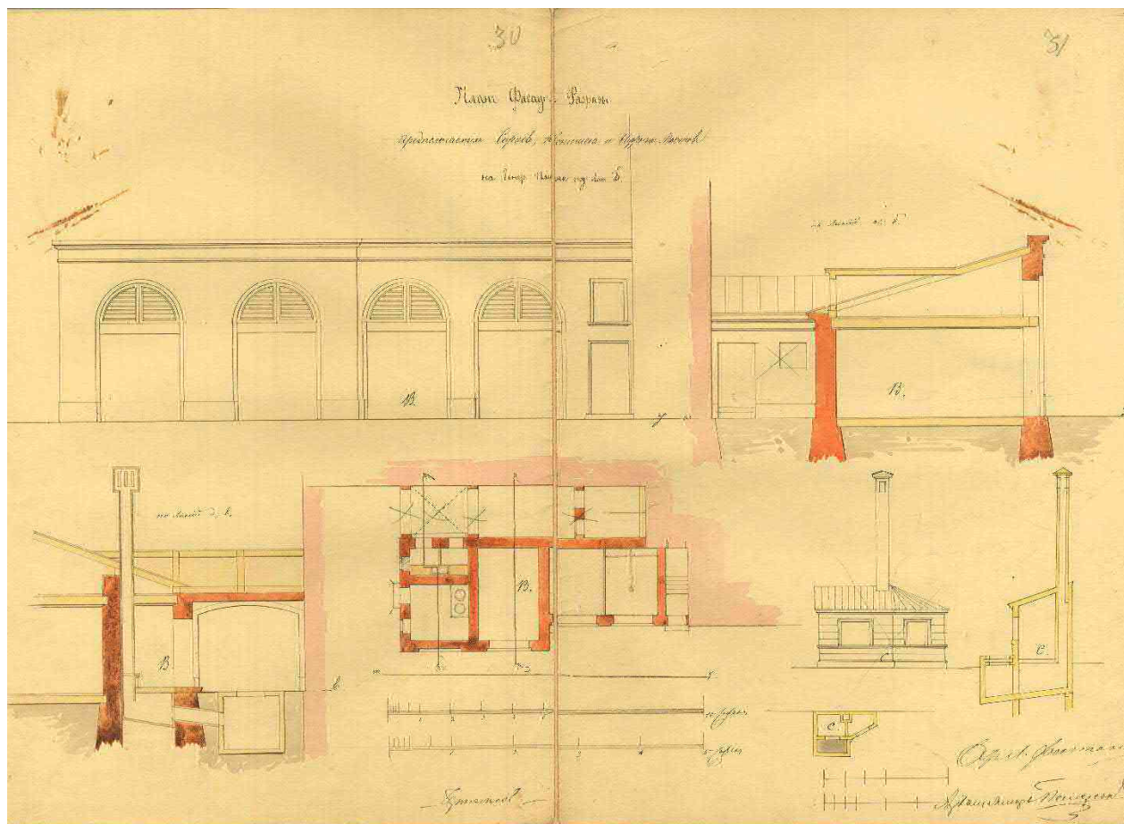
Илл. 8. К.К.Рахау. Особняк И.Ф.Громова. Проект перестройки. Генеральный план. Двор.план и разрез предлагаемых сараев, конюшни и нужных мостов. 1875г. ЦГИА СПб. Ф.513. Оп.102. Д.88. Л.26
